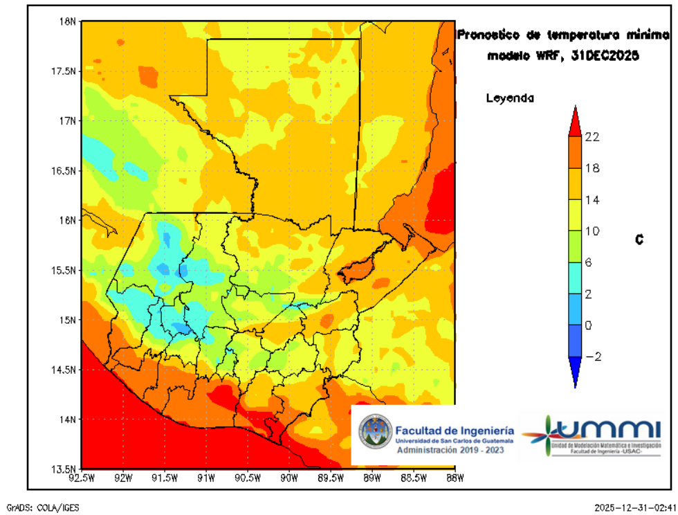
Figura 7: Pronóstico de temperatura mínima diaria del 01 de January
