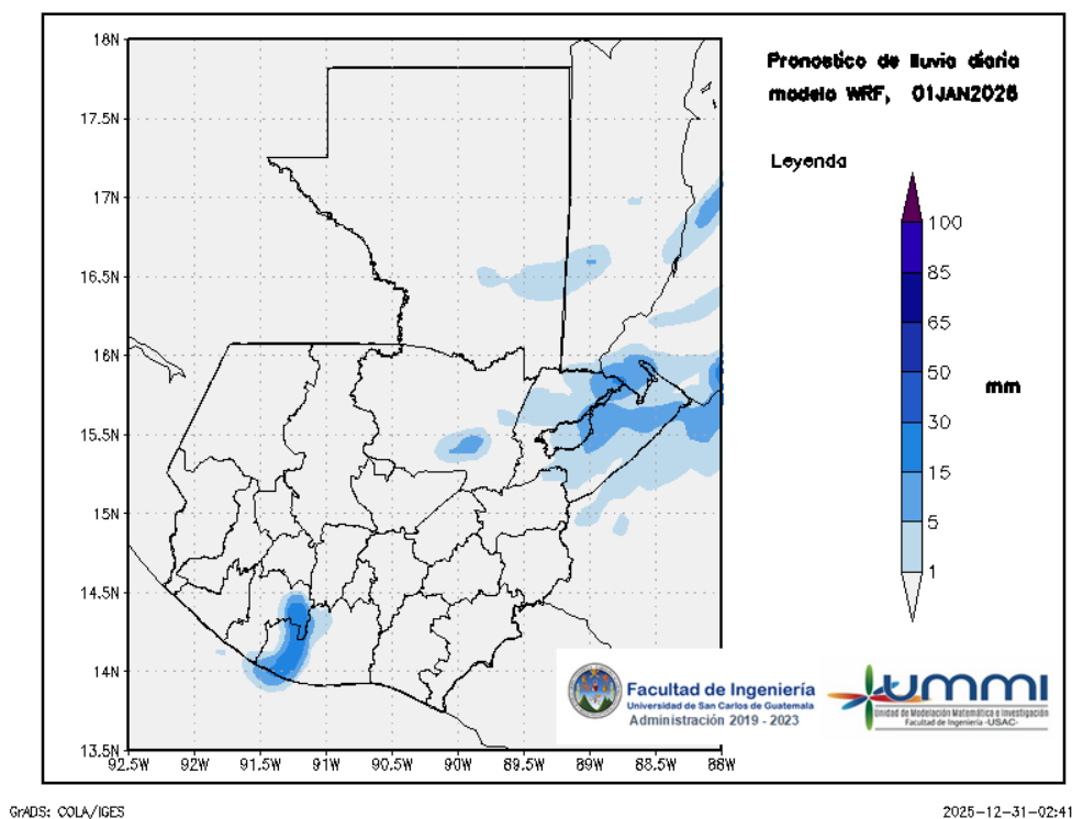
Figura 2: Pronóstico de lluvia diaria del 01 de January
