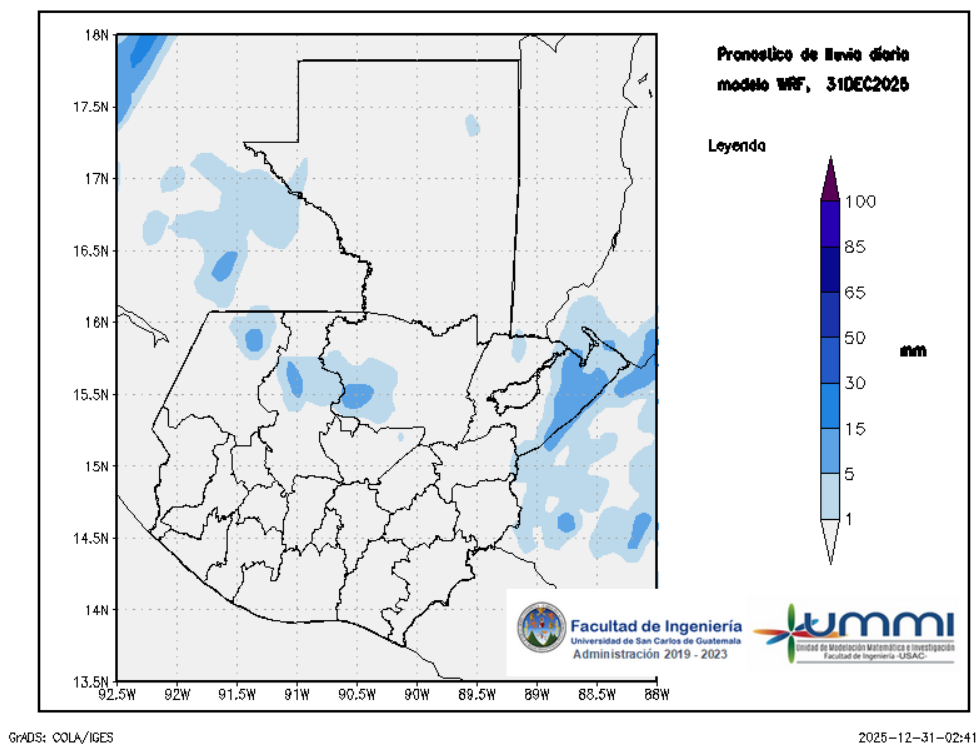
Figura 1: Pronóstico de lluvia diaria del 31 de December
