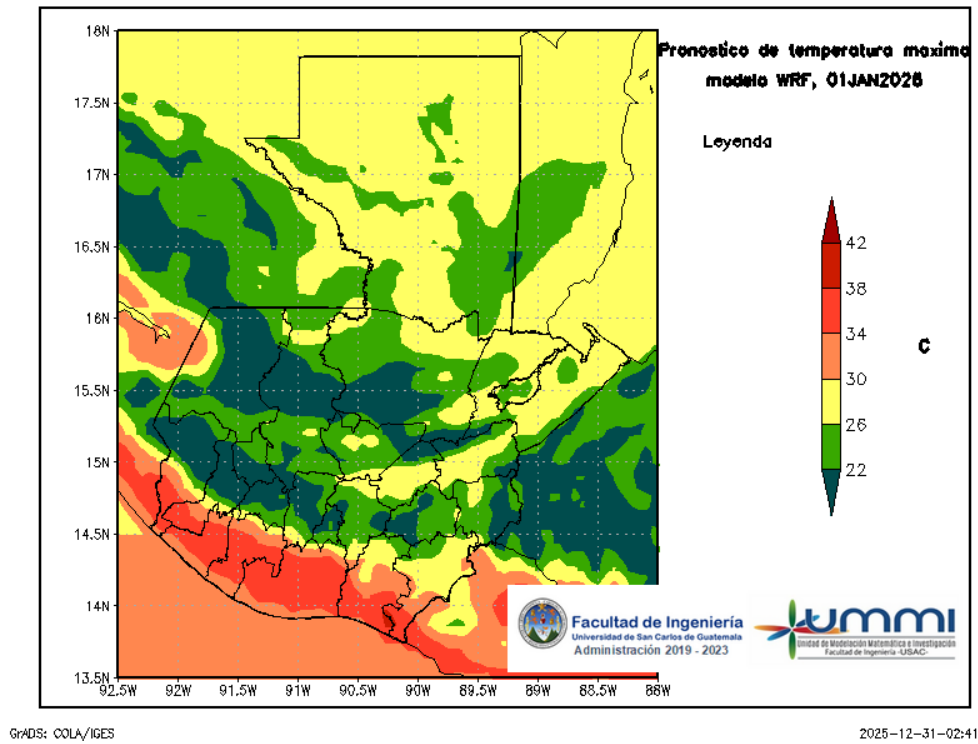
Figura 5: Pronóstico de temperatura máxima diaria del 01 de January
