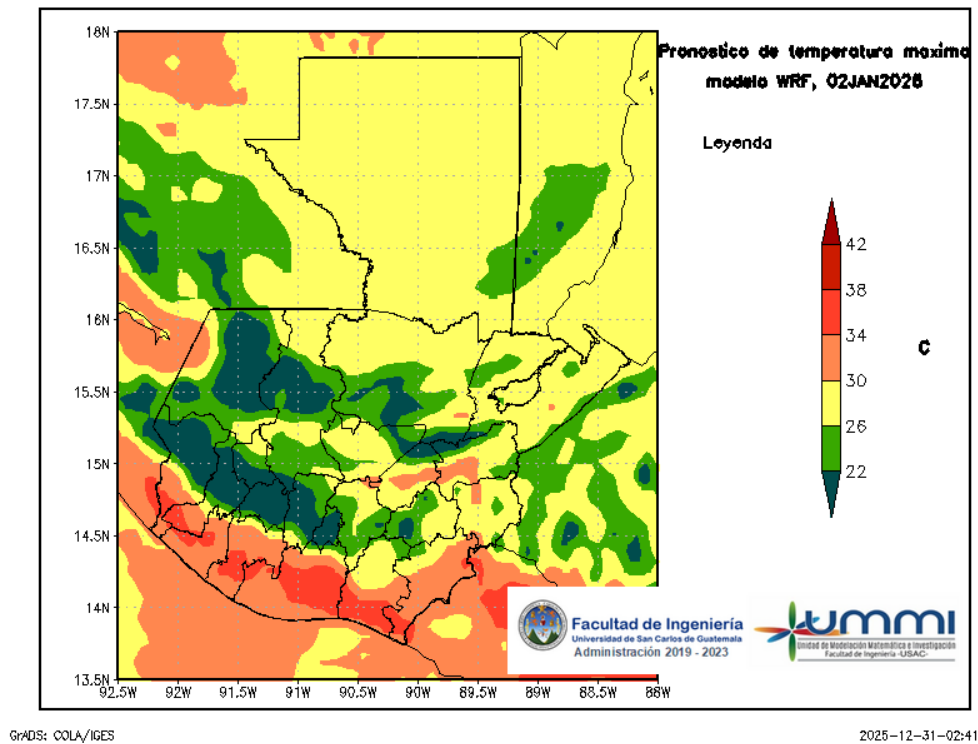
Figura 6: Pronóstico de temperatura máxima diaria del 02 de January
