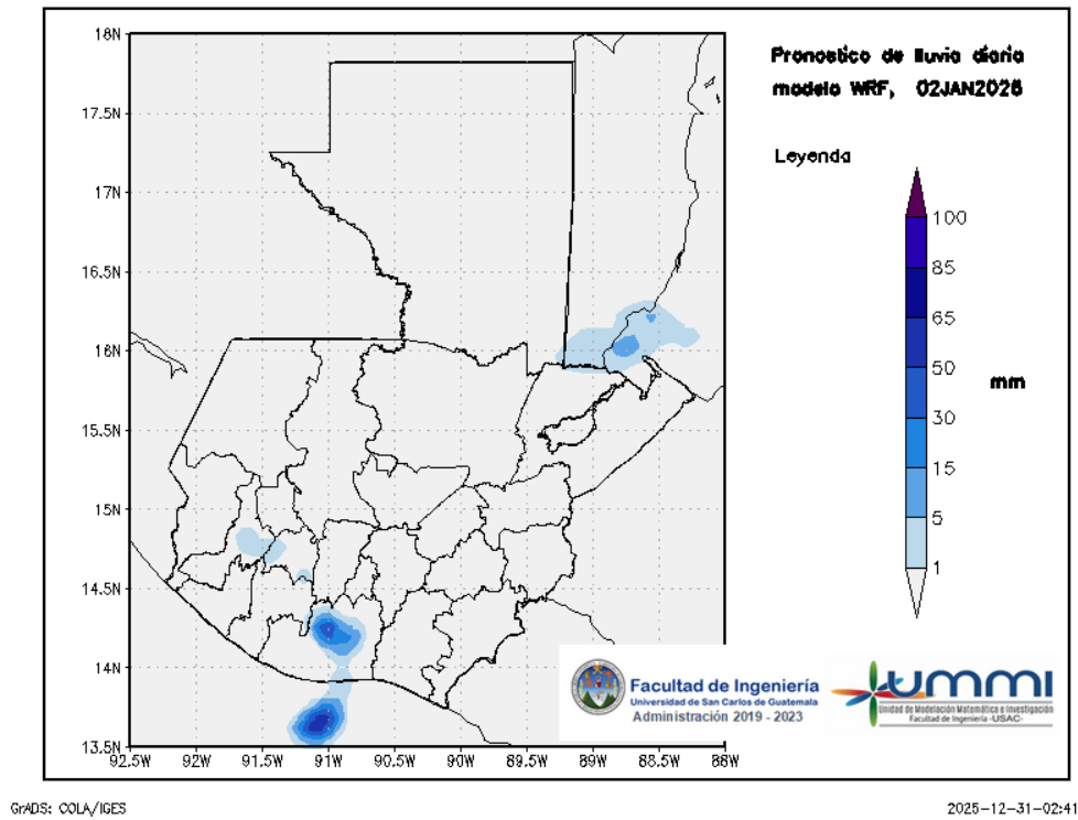
Figura 3: Pronóstico de lluvia diaria del 02 de January
