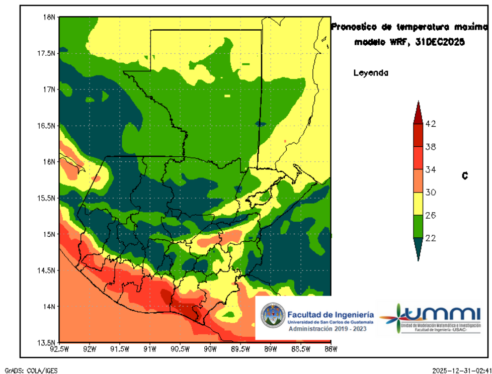
Figura 4: Pronóstico de temperatura máxima diaria del 31 de December
