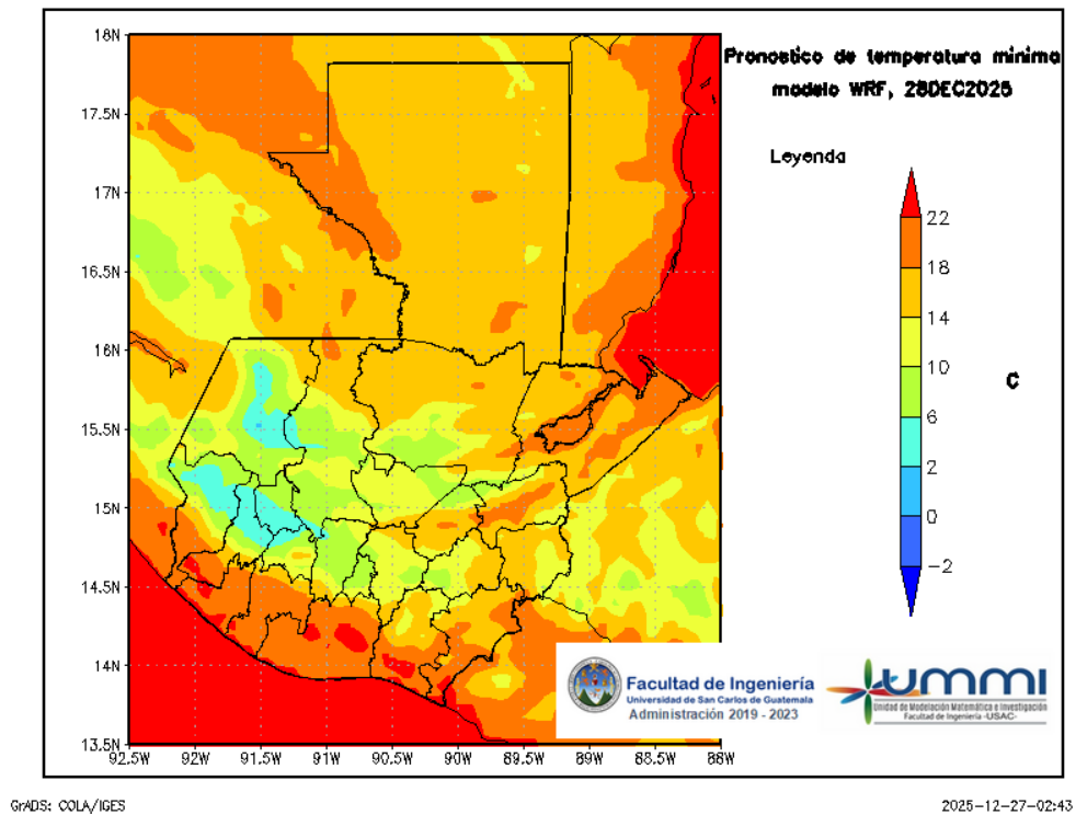
Figura 8: Pronóstico de temperatura mínima diaria del 29 de December
