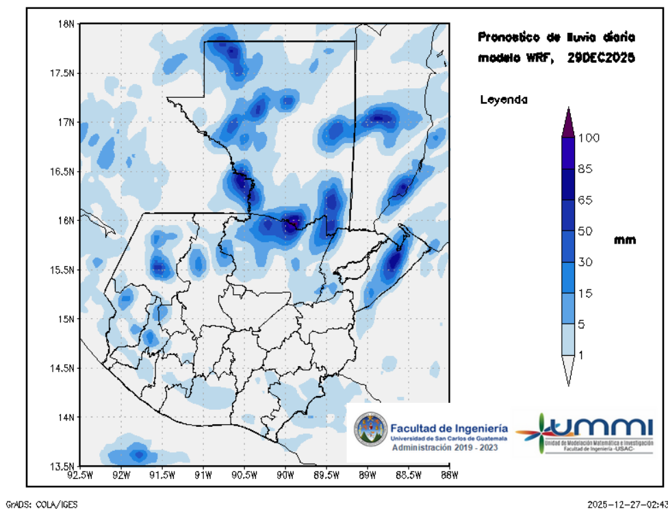
Figura 3: Pronóstico de lluvia diaria del 29 de December
