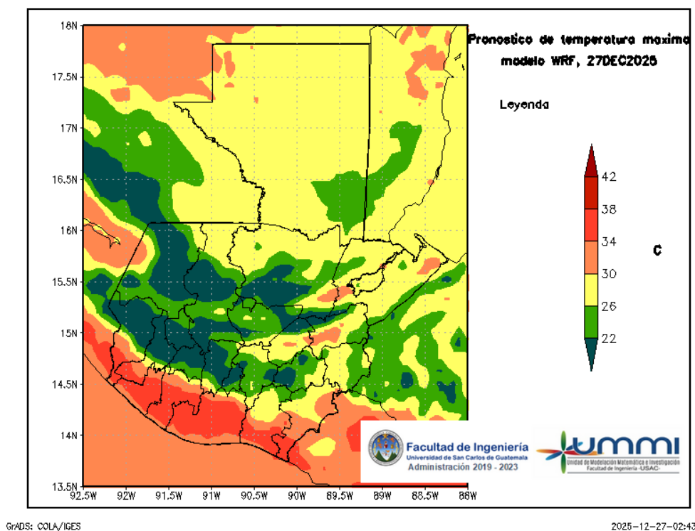
Figura 4: Pronóstico de temperatura máxima diaria del 27 de December
