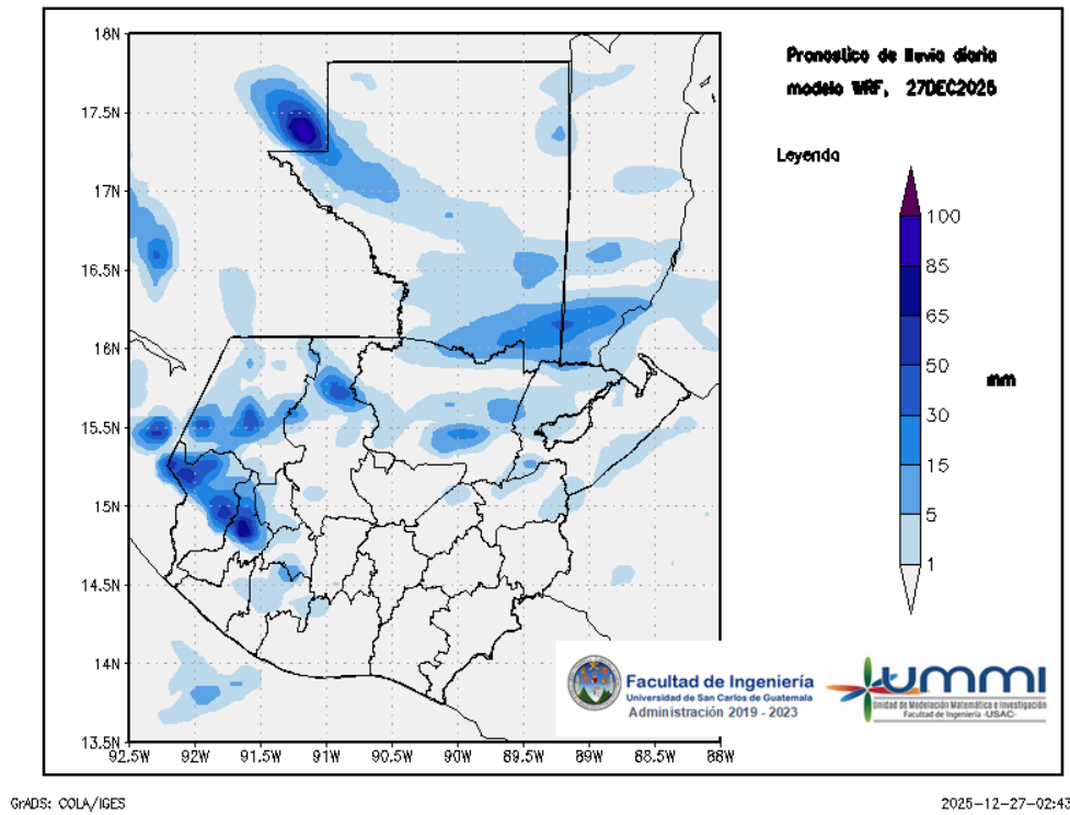
Figura 1: Pronóstico de lluvia diaria del 27 de December
