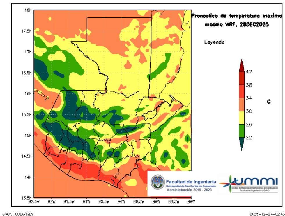
Figura 5: Pronóstico de temperatura máxima diaria del 28 de December
