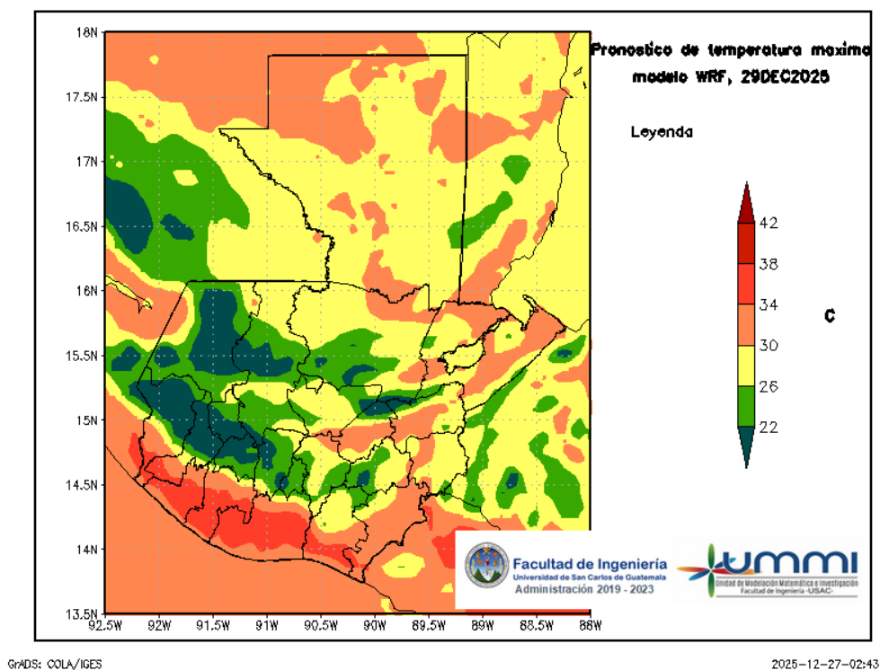
Figura 6: Pronóstico de temperatura máxima diaria del 29 de December
