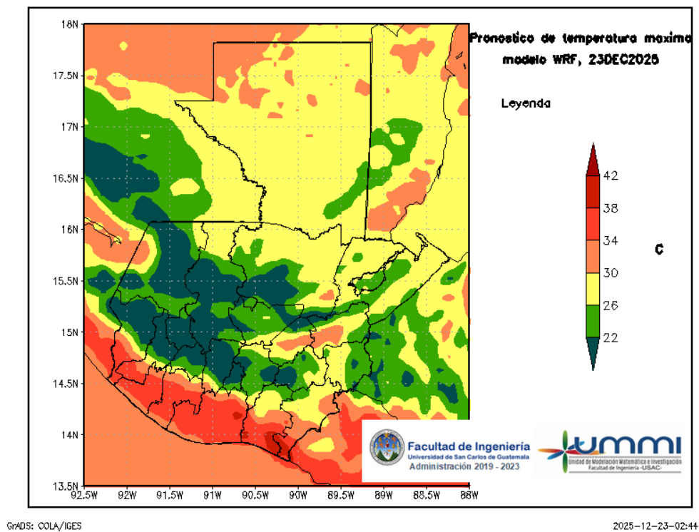
Figura 4: Pronóstico de temperatura máxima diaria del 23 de December
