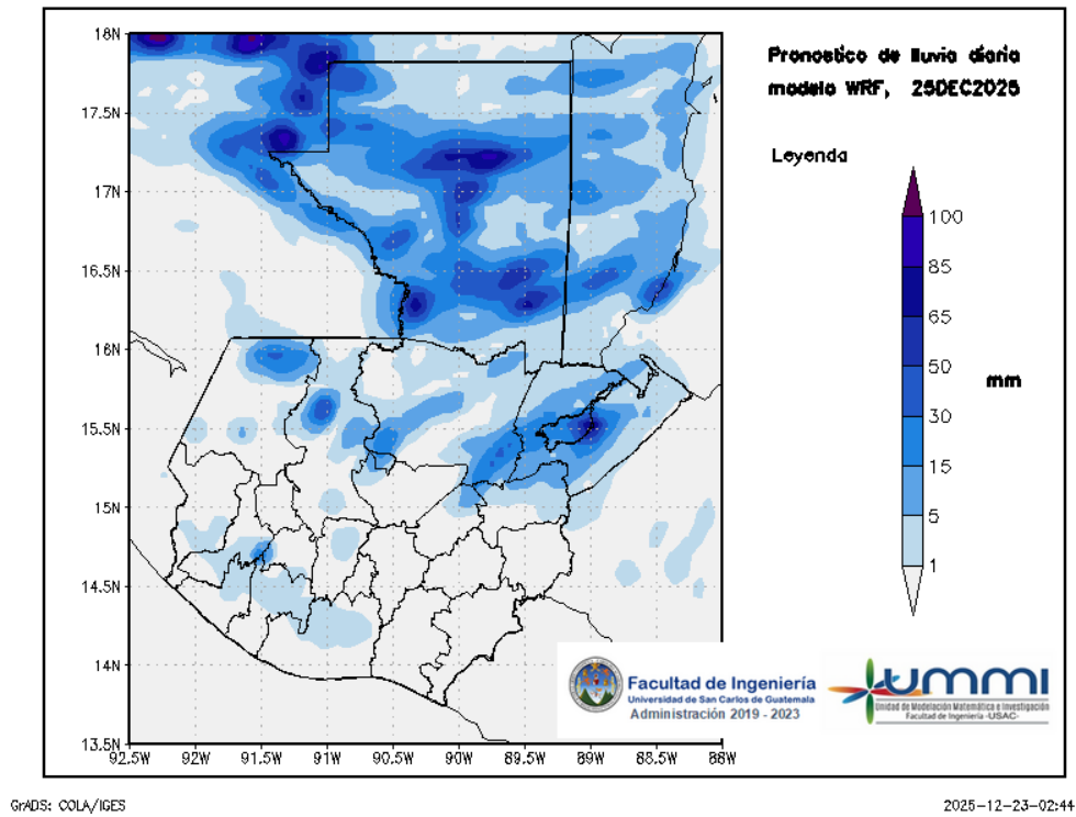
Figura 3: Pronóstico de lluvia diaria del 25 de December
