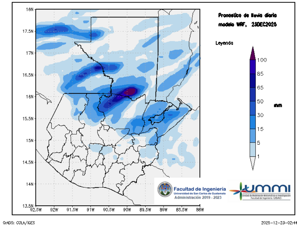
Figura 1: Pronóstico de lluvia diaria del 23 de December
