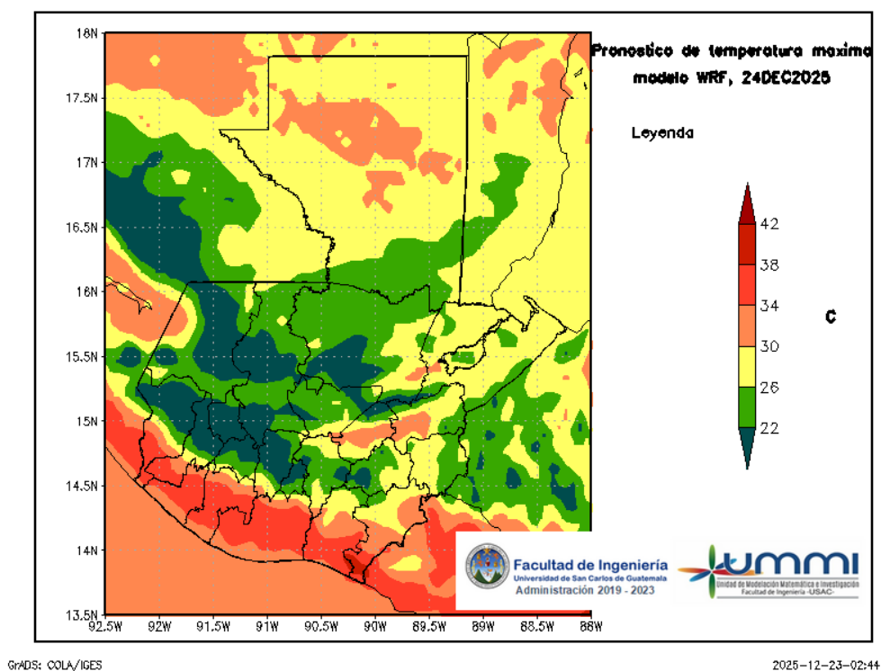
Figura 5: Pronóstico de temperatura máxima diaria del 24 de December
