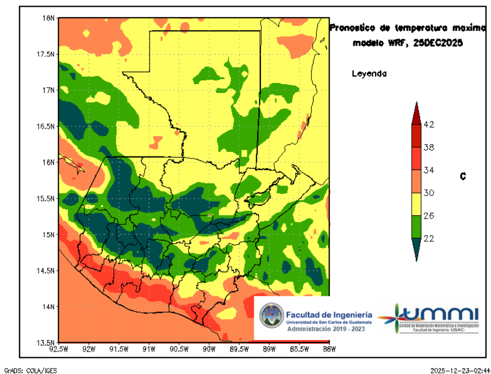
Figura 6: Pronóstico de temperatura máxima diaria del 25 de December
