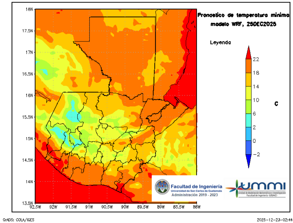
Figura 9: Pronóstico de temperatura mínima diaria del 26 de December
