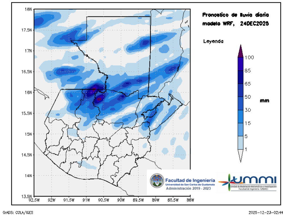
Figura 2: Pronóstico de lluvia diaria del 24 de December
