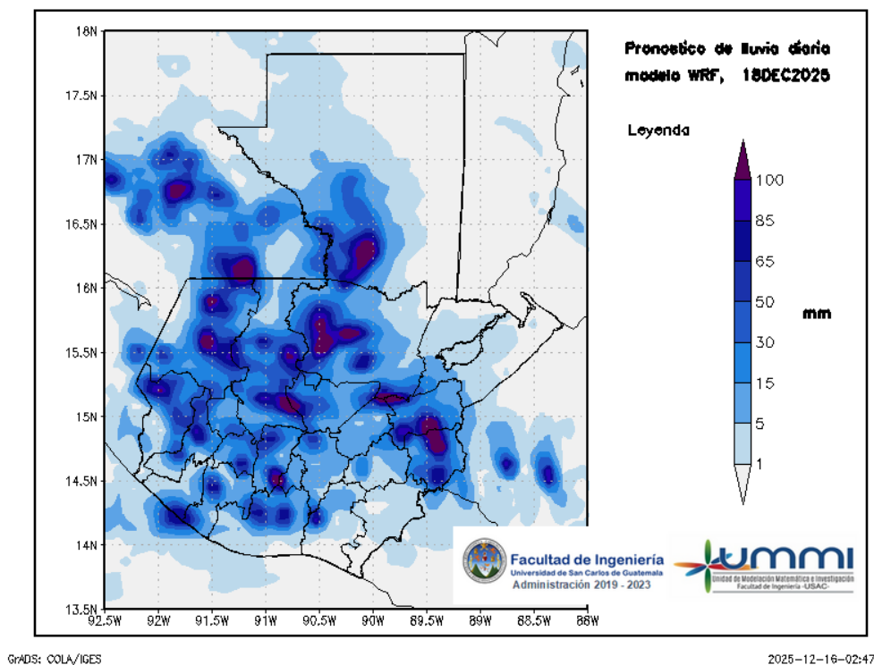
Figura 3: Pronóstico de lluvia diaria del 18 de December
