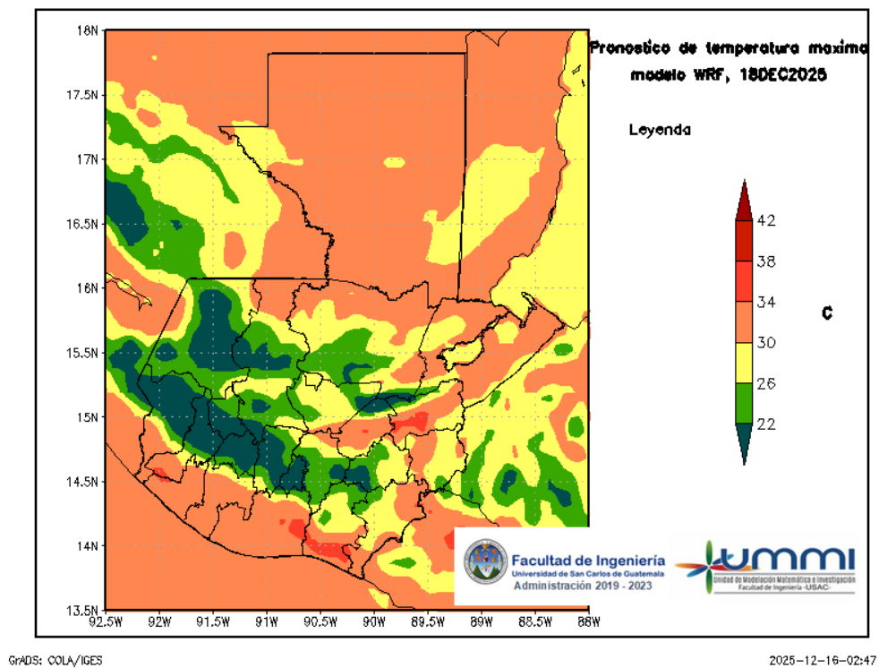
Figura 6: Pronóstico de temperatura máxima diaria del 18 de December
