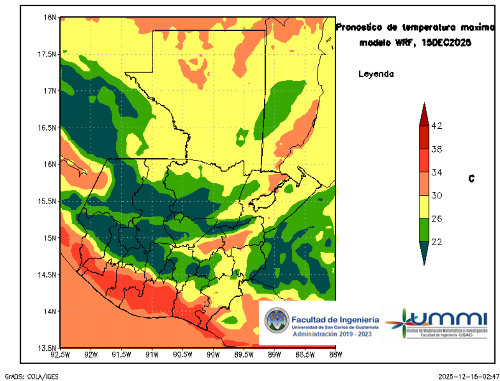
Figura 4: Pronóstico de temperatura máxima diaria del 15 de December
