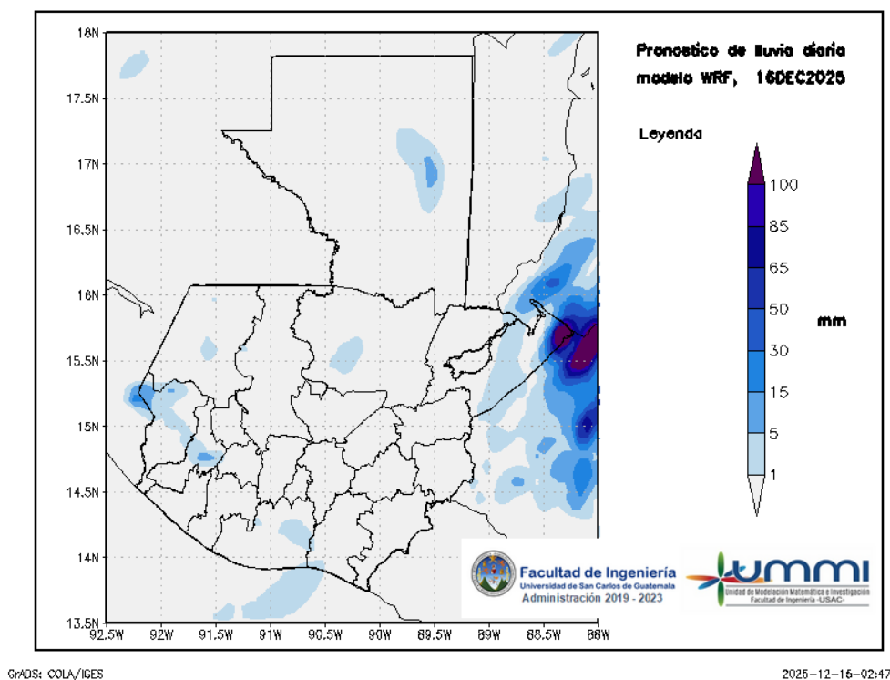
Figura 2: Pronóstico de lluvia diaria del 16 de December
