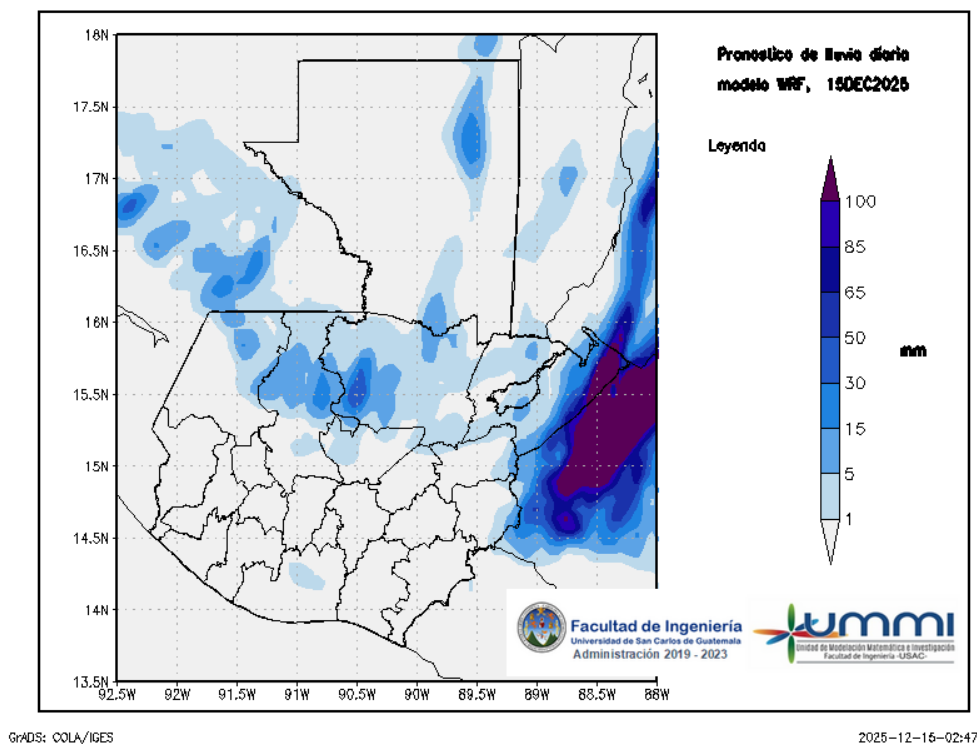
Figura 1: Pronóstico de lluvia diaria del 15 de December
