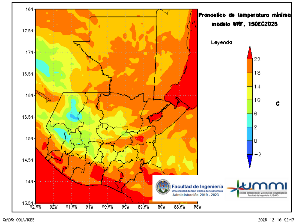
Figura 7: Pronóstico de temperatura mínima diaria del 16 de December
