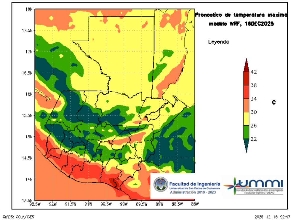
Figura 5: Pronóstico de temperatura máxima diaria del 16 de December
