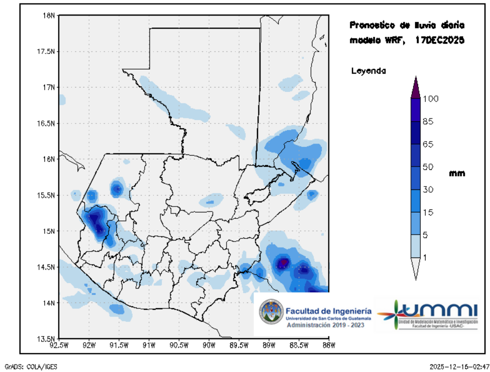
Figura 3: Pronóstico de lluvia diaria del 17 de December
