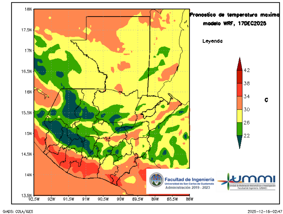
Figura 6: Pronóstico de temperatura máxima diaria del 17 de December
