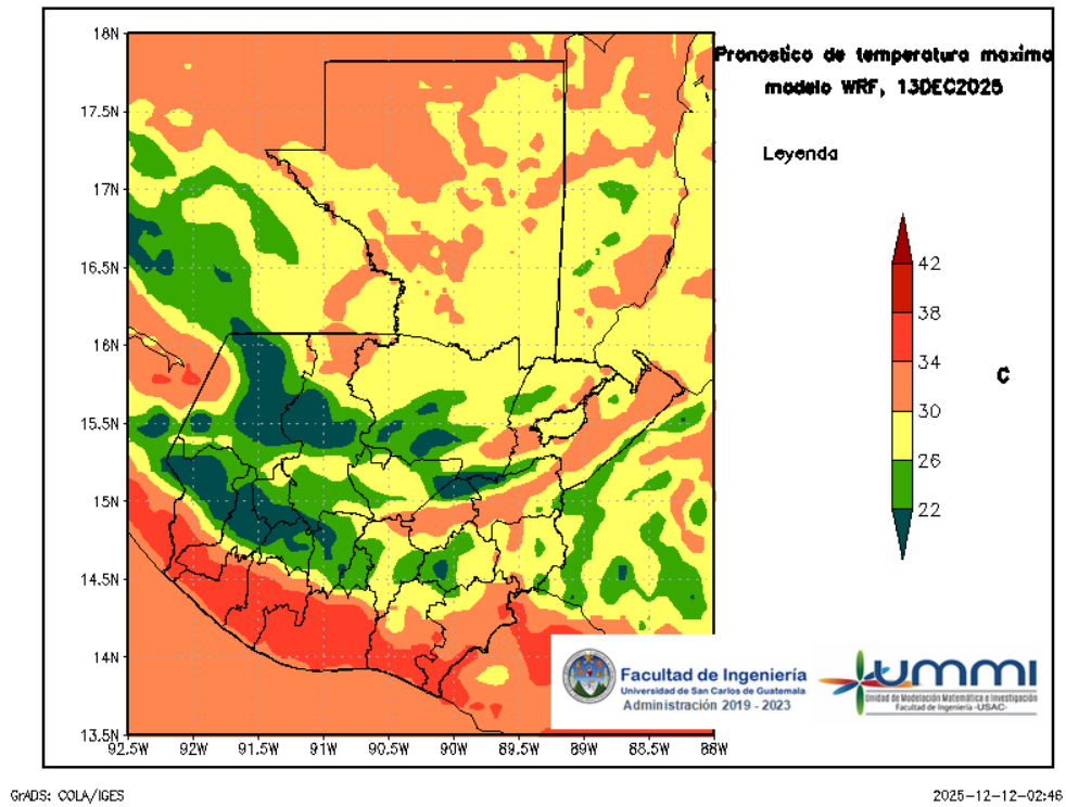
Figura 5: Pronóstico de temperatura máxima diaria del 13 de December
