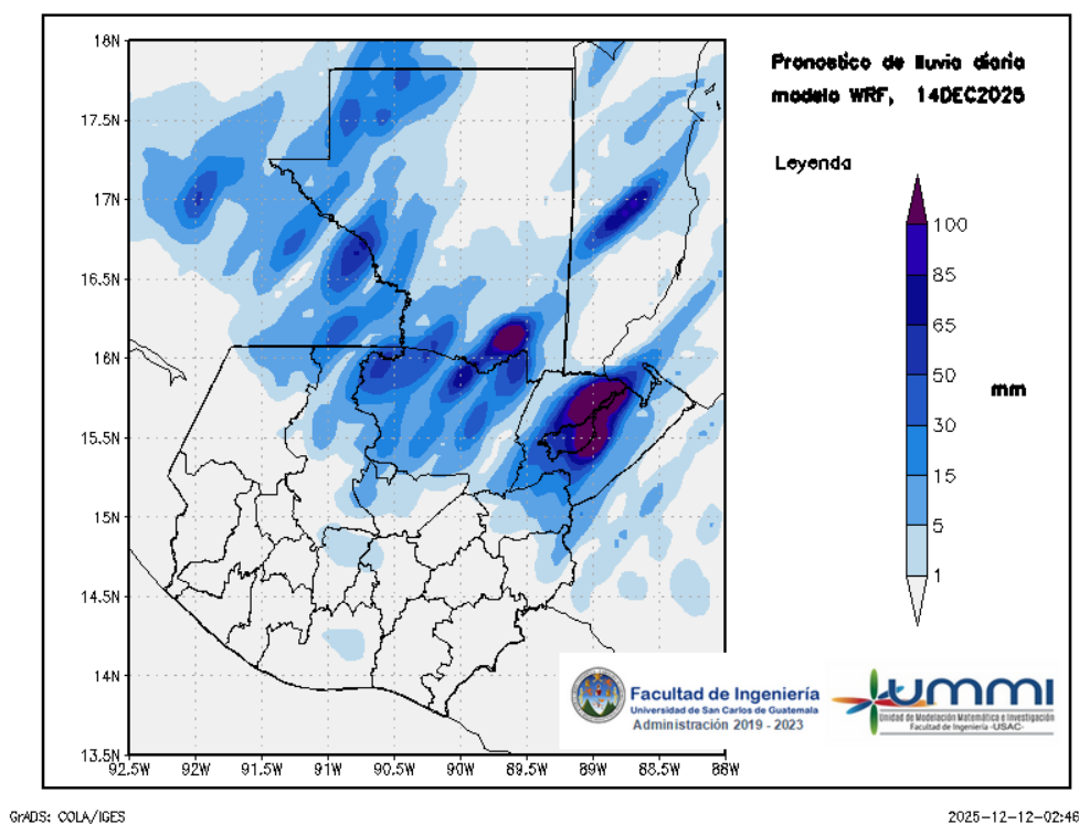
Figura 3: Pronóstico de lluvia diaria del 14 de December
