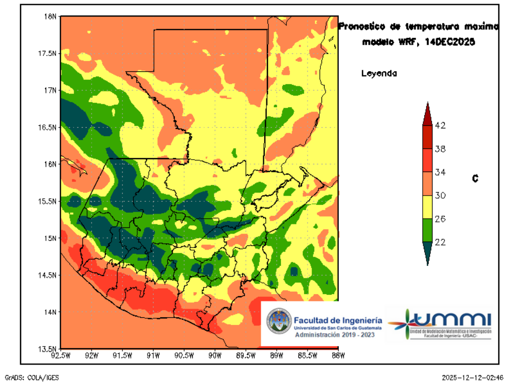
Figura 6: Pronóstico de temperatura máxima diaria del 14 de December
