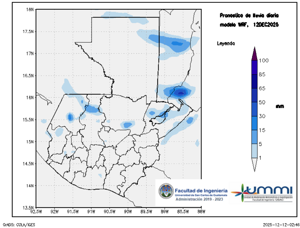
Figura 1: Pronóstico de lluvia diaria del 12 de December
