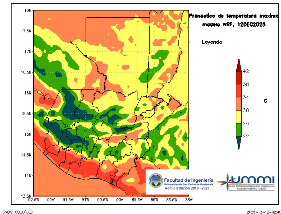
Figura 4: Pronóstico de temperatura máxima diaria del 12 de December
