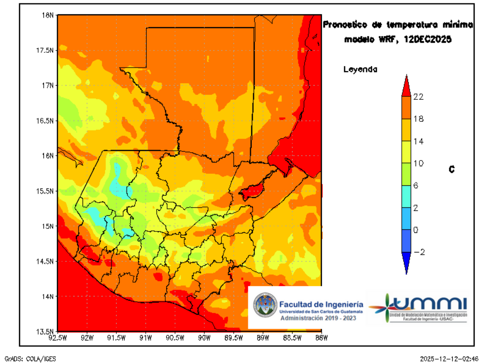
Figura 7: Pronóstico de temperatura mínima diaria del 13 de December
