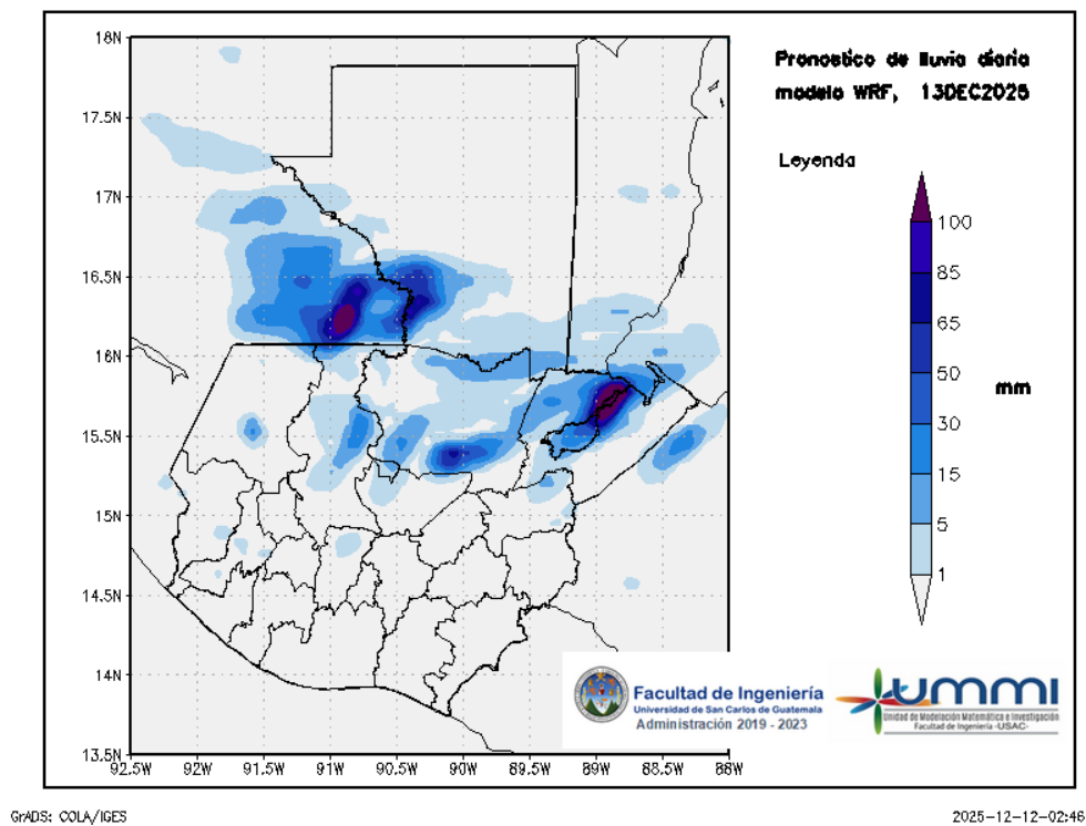
Figura 2: Pronóstico de lluvia diaria del 13 de December
