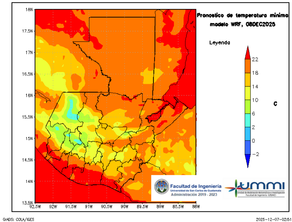
Figura 8: Pronóstico de temperatura mínima diaria del 09 de December
