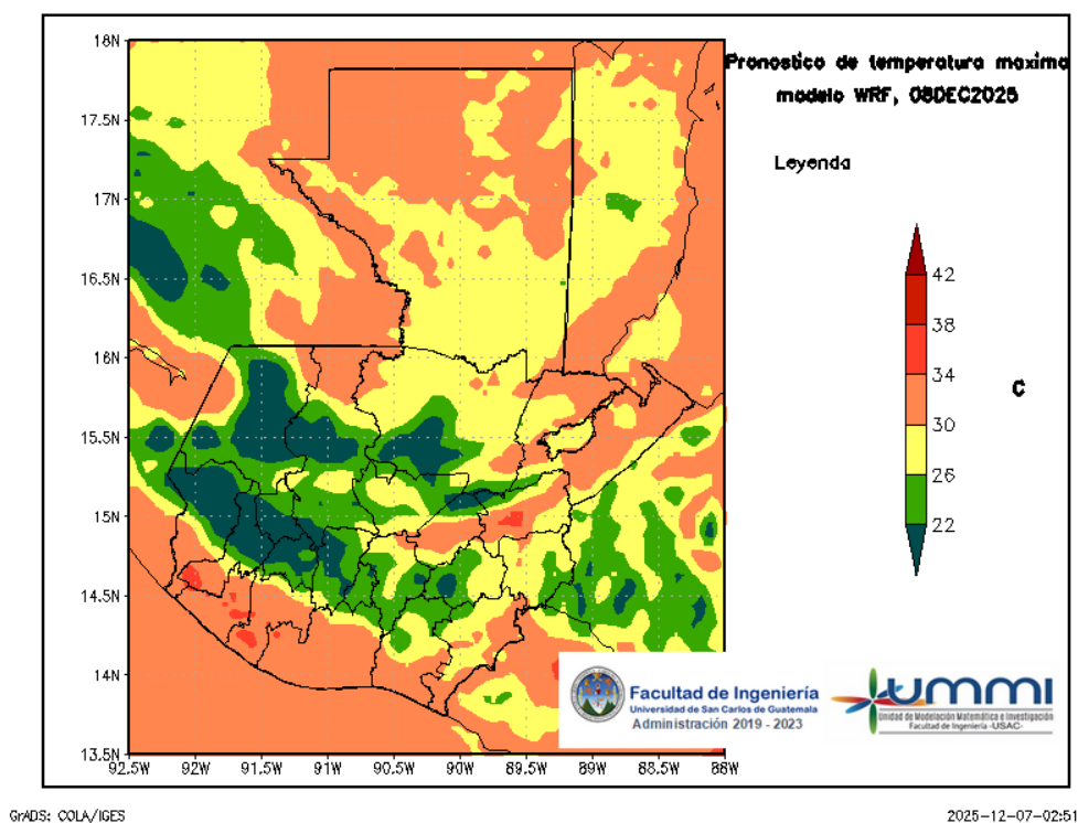
Figura 5: Pronóstico de temperatura máxima diaria del 08 de December
