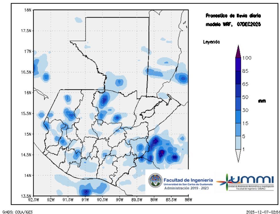
Figura 1: Pronóstico de lluvia diaria del 07 de December
