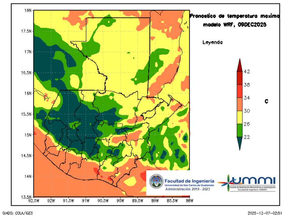
Figura 6: Pronóstico de temperatura máxima diaria del 09 de December
