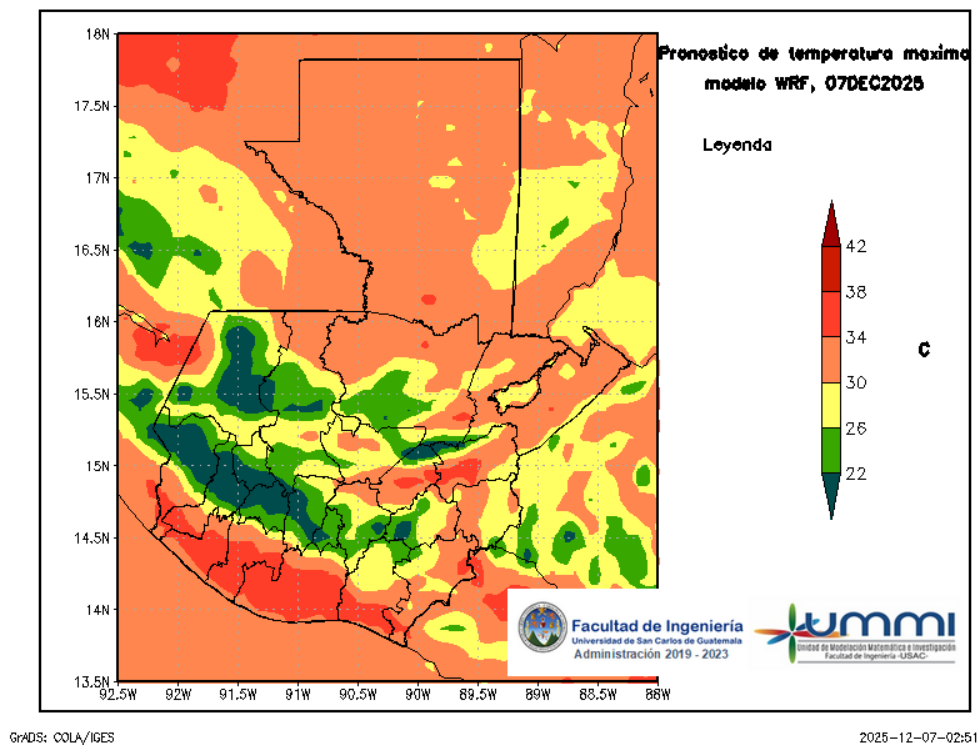
Figura 4: Pronóstico de temperatura máxima diaria del 07 de December
