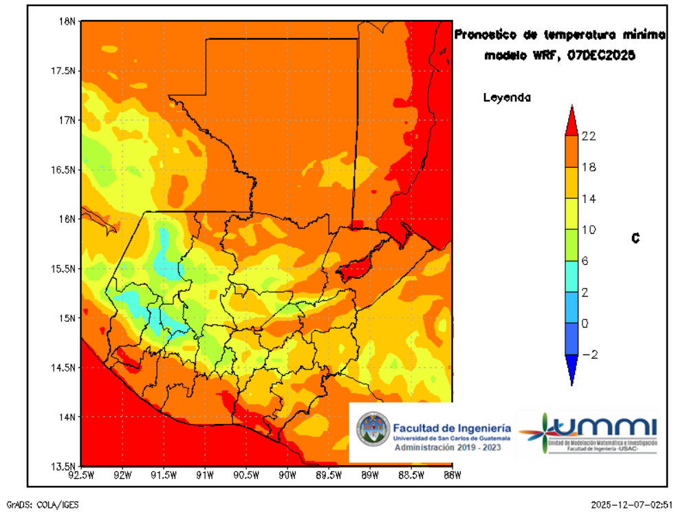
Figura 7: Pronóstico de temperatura mínima diaria del 08 de December
