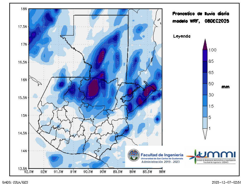
Figura 2: Pronóstico de lluvia diaria del 08 de December
