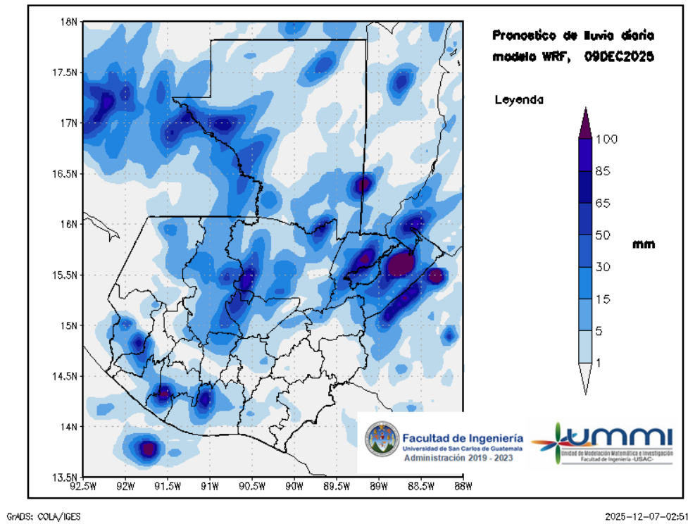
Figura 3: Pronóstico de lluvia diaria del 09 de December
