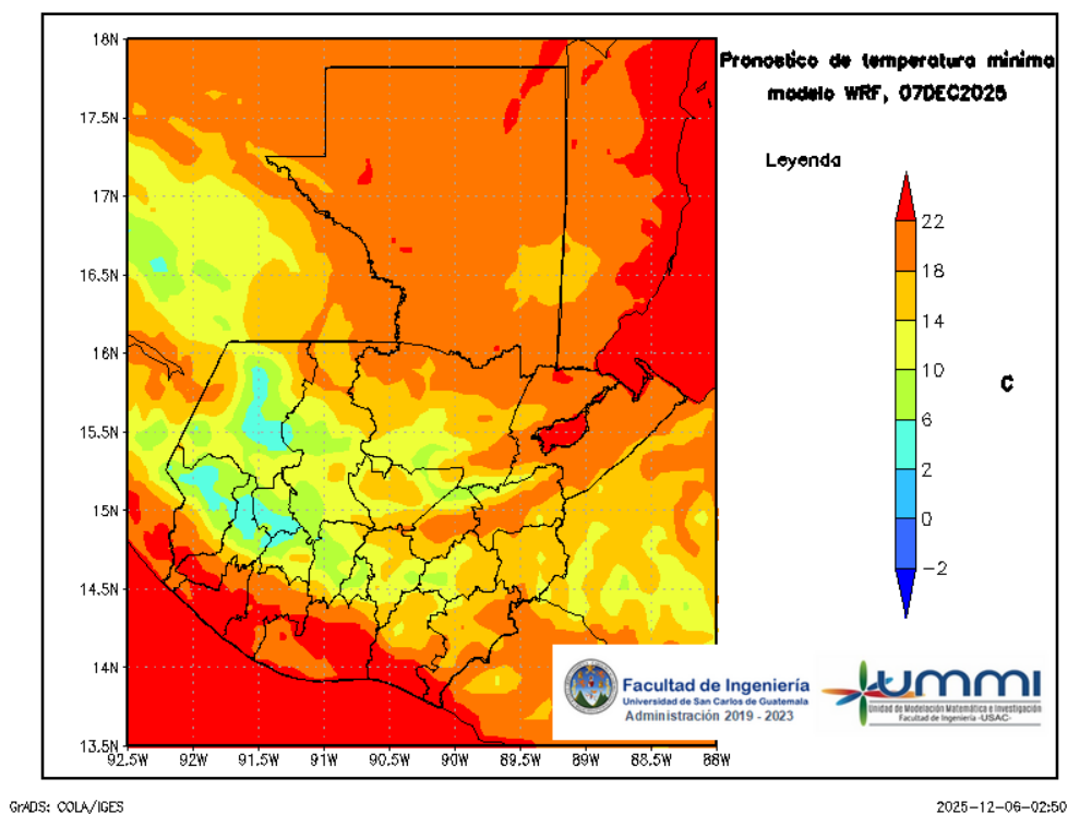
Figura 8: Pronóstico de temperatura mínima diaria del 08 de December
