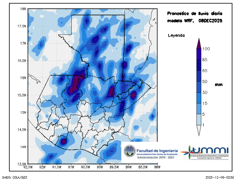
Figura 3: Pronóstico de lluvia diaria del 08 de December
