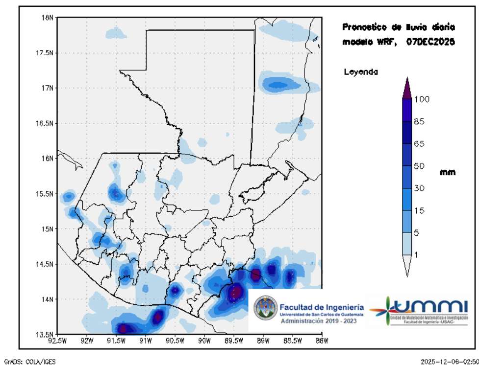
Figura 2: Pronóstico de lluvia diaria del 07 de December
