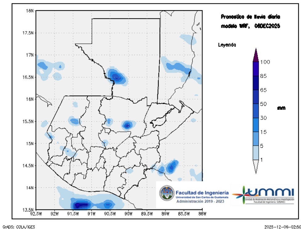
Figura 1: Pronóstico de lluvia diaria del 06 de December
