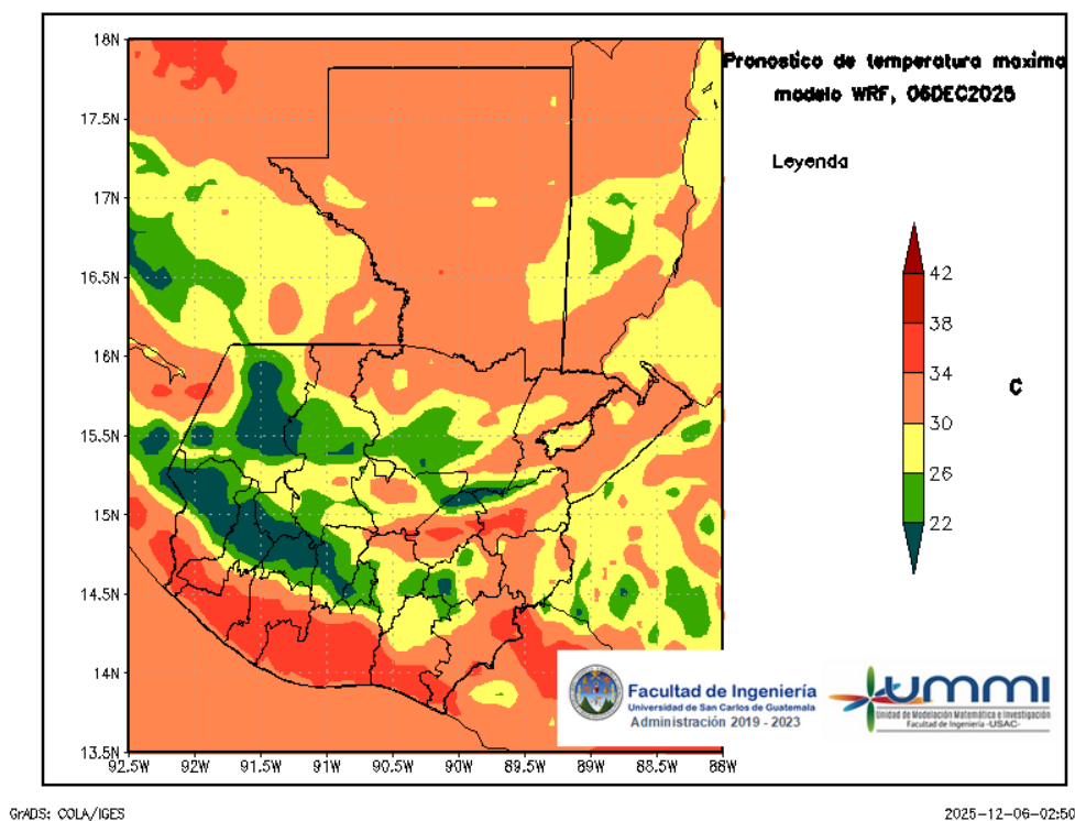
Figura 4: Pronóstico de temperatura máxima diaria del 06 de December
