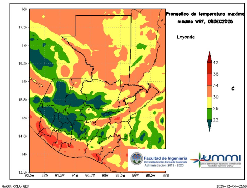
Figura 6: Pronóstico de temperatura máxima diaria del 08 de December
