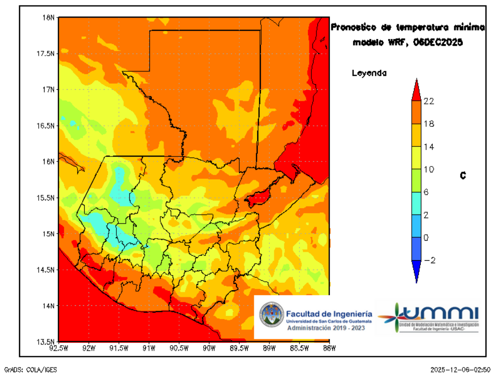
Figura 7: Pronóstico de temperatura mínima diaria del 07 de December
