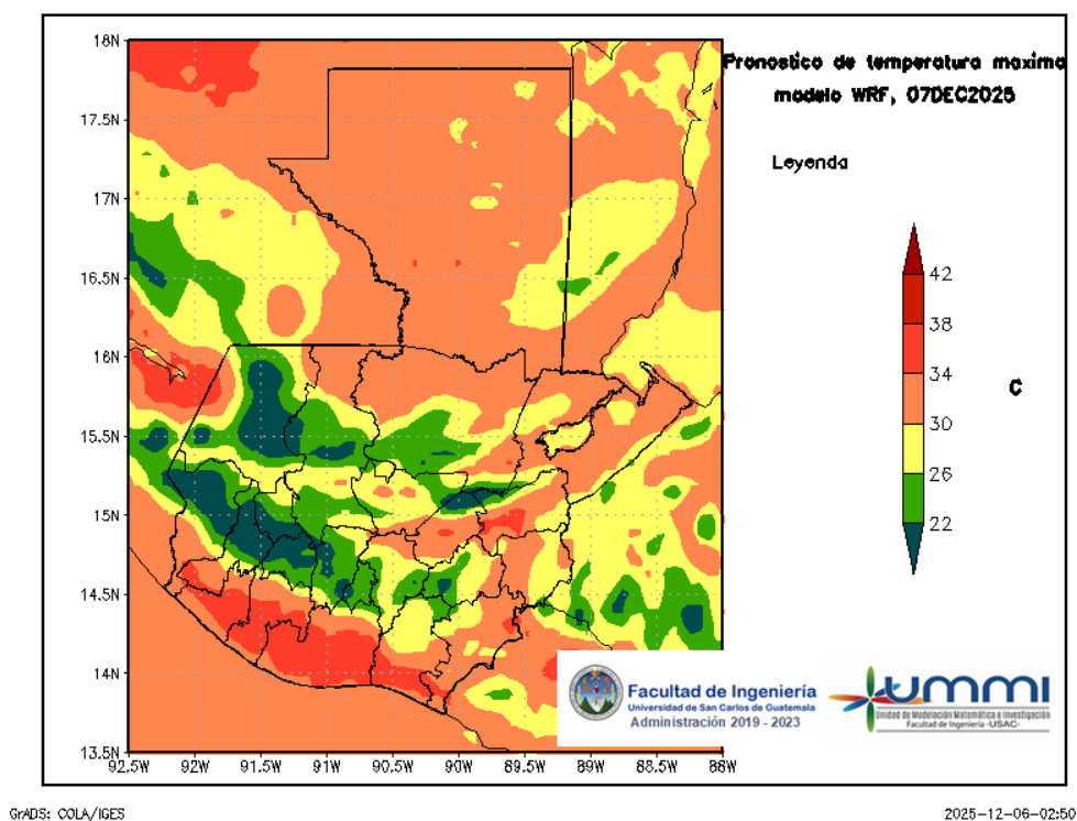
Figura 5: Pronóstico de temperatura máxima diaria del 07 de December
