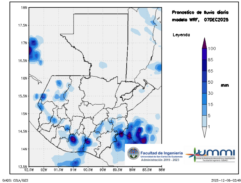
Figura 3: Pronóstico de lluvia diaria del 07 de December
