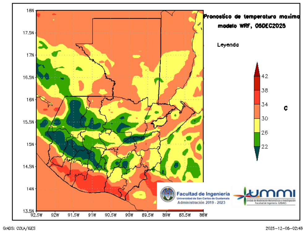
Figura 4: Pronóstico de temperatura máxima diaria del 05 de December
