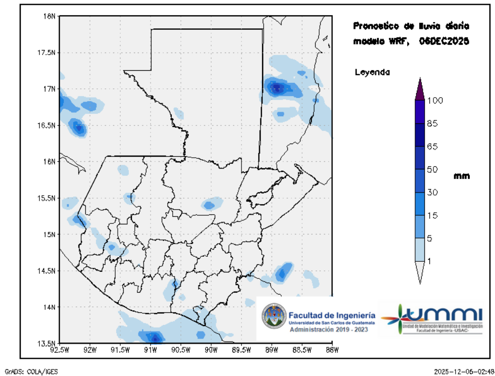
Figura 2: Pronóstico de lluvia diaria del 06 de December
