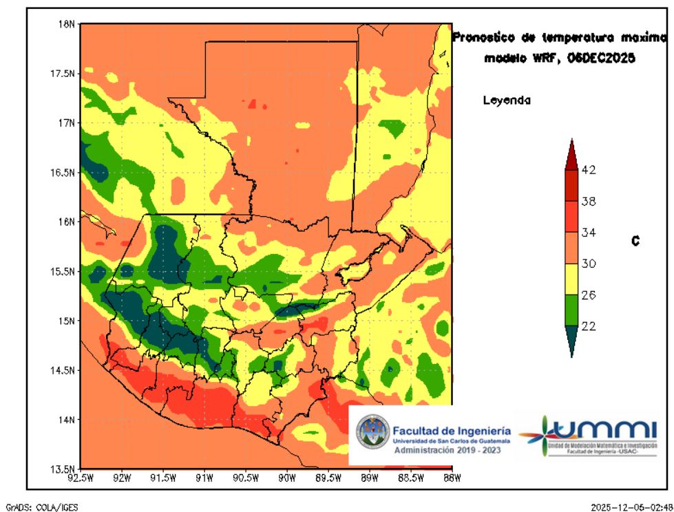
Figura 5: Pronóstico de temperatura máxima diaria del 06 de December
