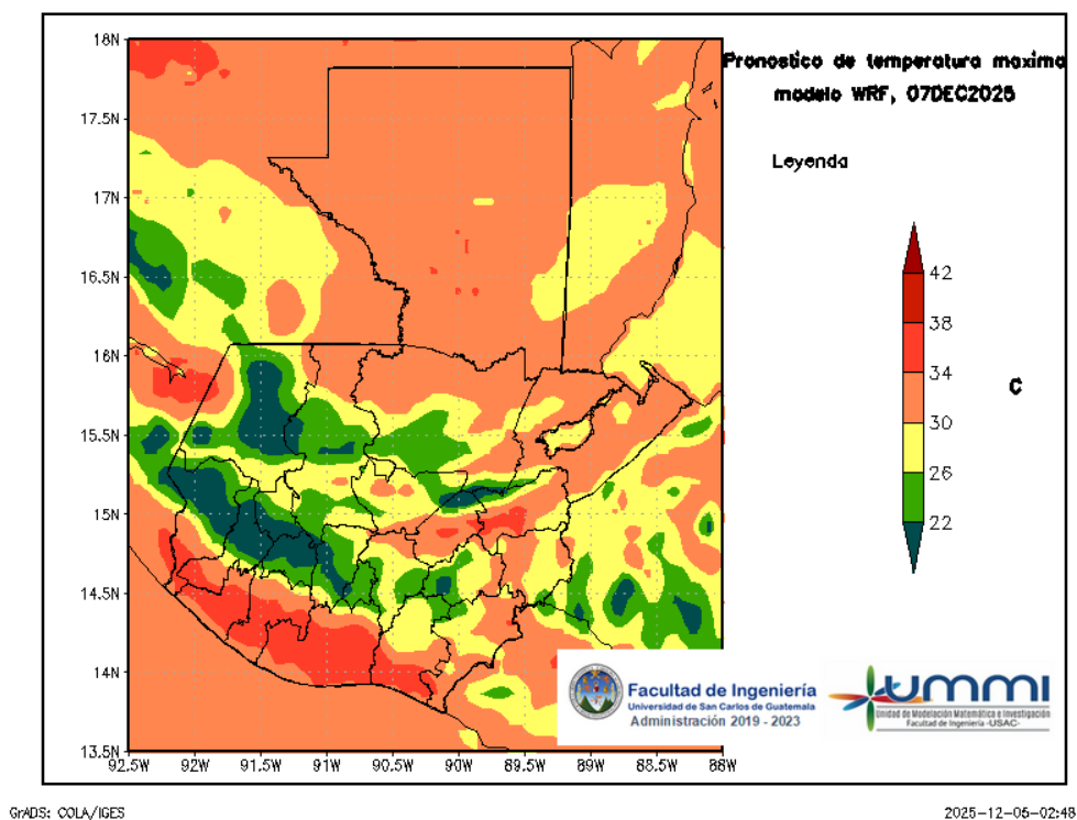
Figura 6: Pronóstico de temperatura máxima diaria del 07 de December
