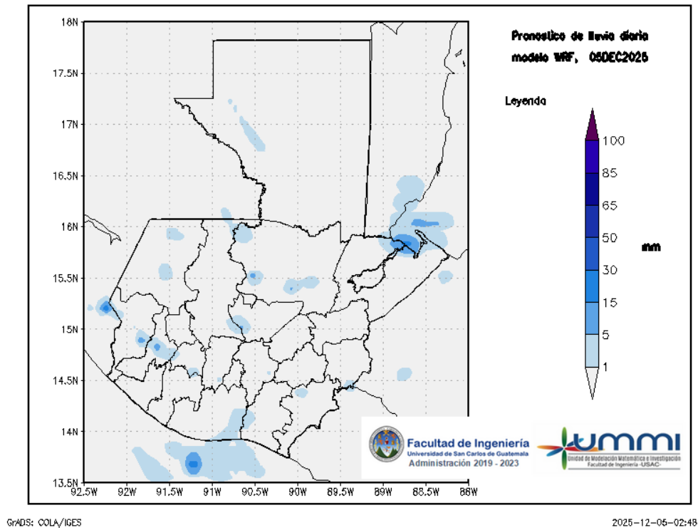
Figura 1: Pronóstico de lluvia diaria del 05 de December
