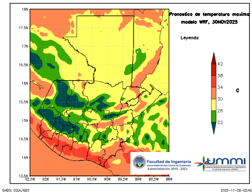
Figura 6: Pronóstico de temperatura máxima diaria del 30 de November
