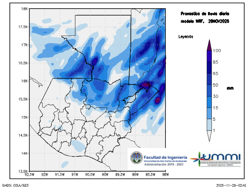
Figura 1: Pronóstico de lluvia diaria del 28 de November
