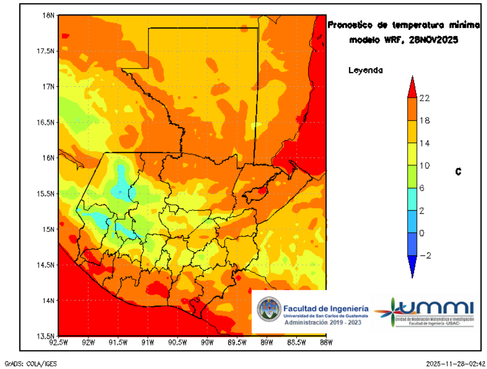
Figura 7: Pronóstico de temperatura mínima diaria del 29 de November
