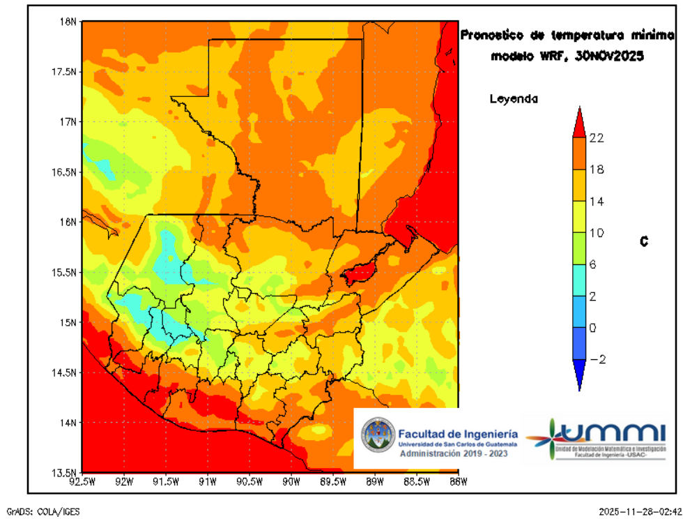
Figura 9: Pronóstico de temperatura mínima diaria del 01 de December
