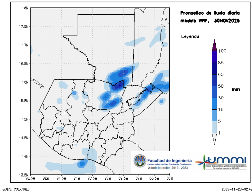
Figura 3: Pronóstico de lluvia diaria del 30 de November
