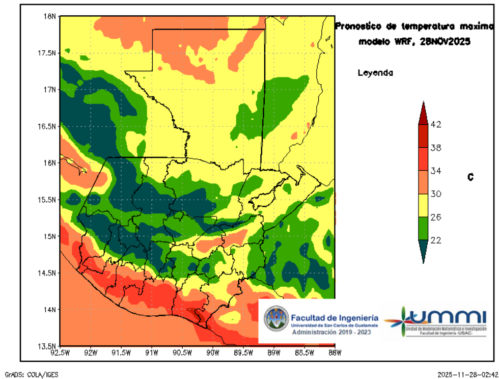
Figura 4: Pronóstico de temperatura máxima diaria del 28 de November
