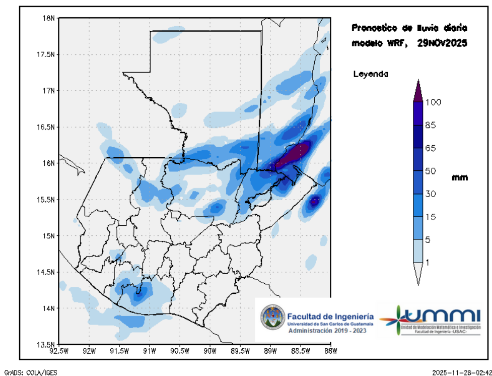
Figura 2: Pronóstico de lluvia diaria del 29 de November
