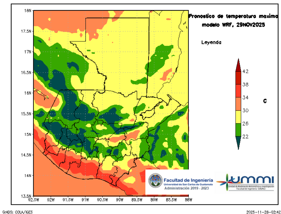
Figura 5: Pronóstico de temperatura máxima diaria del 29 de November
