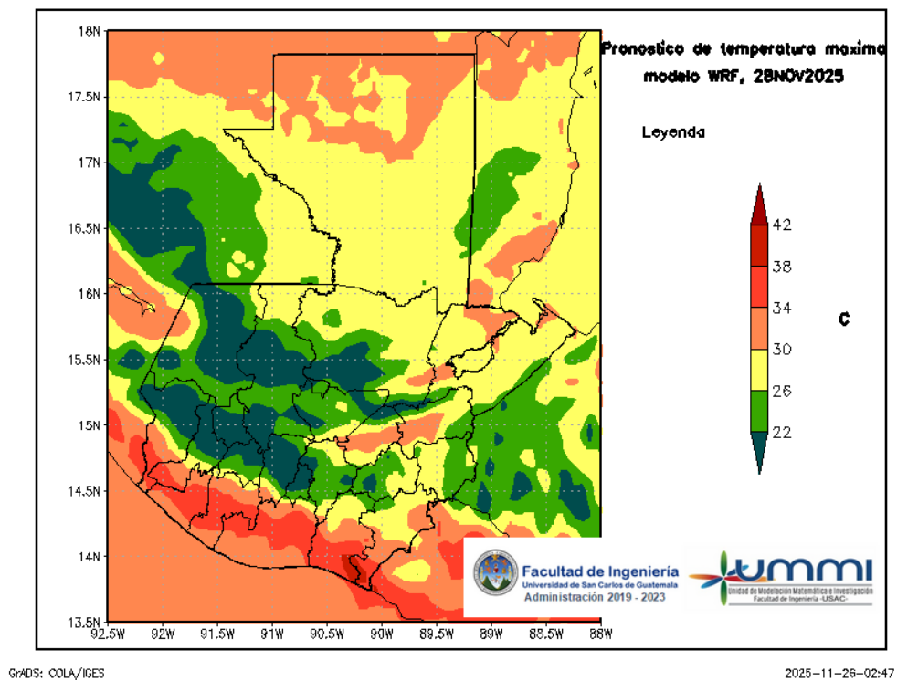
Figura 6: Pronóstico de temperatura máxima diaria del 28 de November
