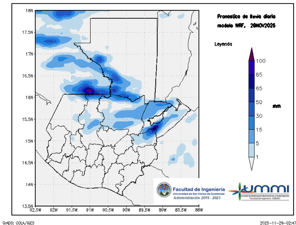
Figura 1: Pronóstico de lluvia diaria del 26 de November
