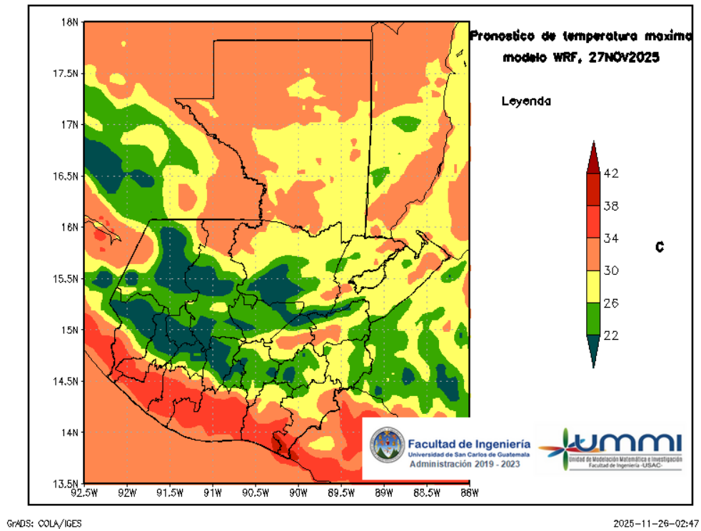
Figura 5: Pronóstico de temperatura máxima diaria del 27 de November
