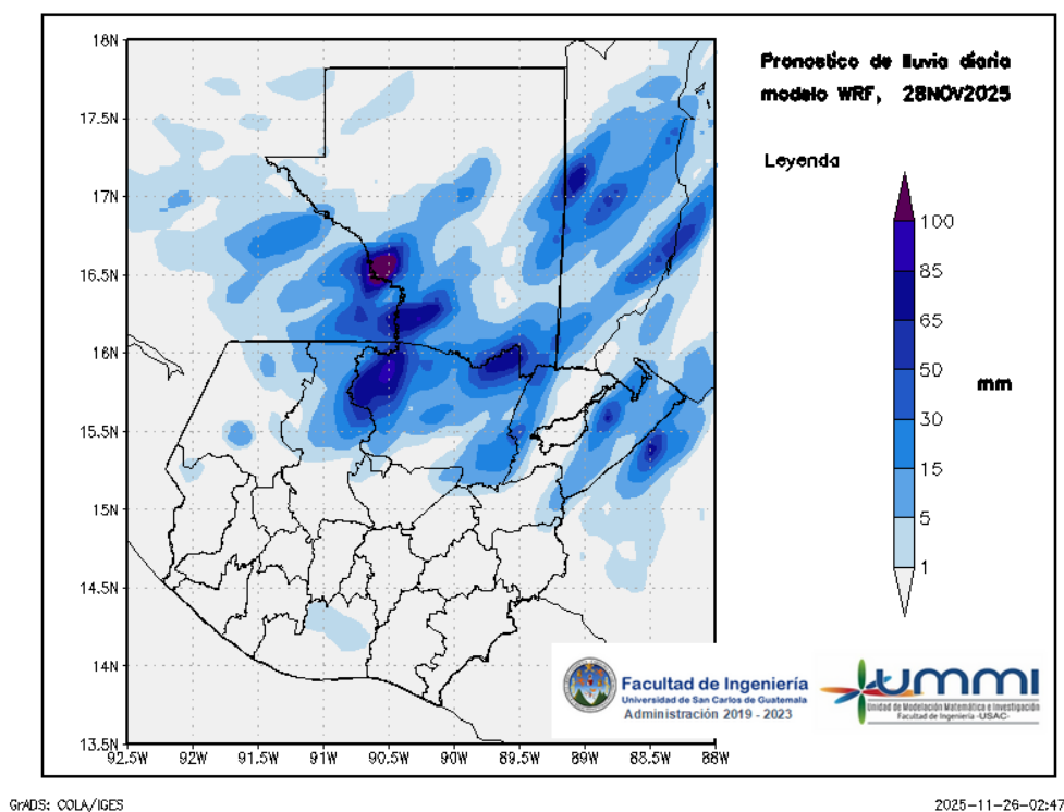
Figura 3: Pronóstico de lluvia diaria del 28 de November
