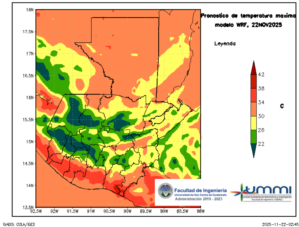
Figura 4: Pronóstico de temperatura máxima diaria del 22 de November
