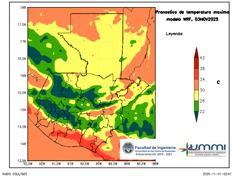
Figura 6: Pronóstico de temperatura máxima diaria del 03 de November
