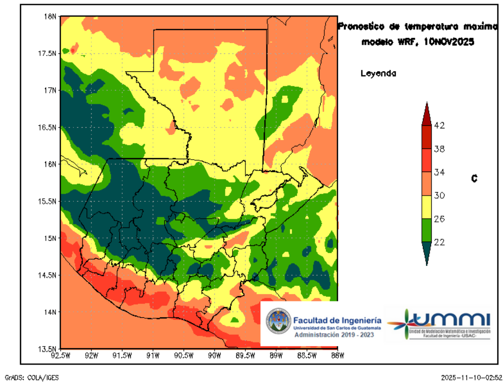
Figura 4: Pronóstico de temperatura máxima diaria del 10 de November
