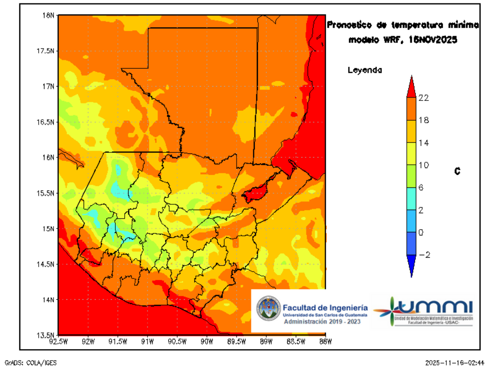
Figura 7: Pronóstico de temperatura mínima diaria del 17 de November
