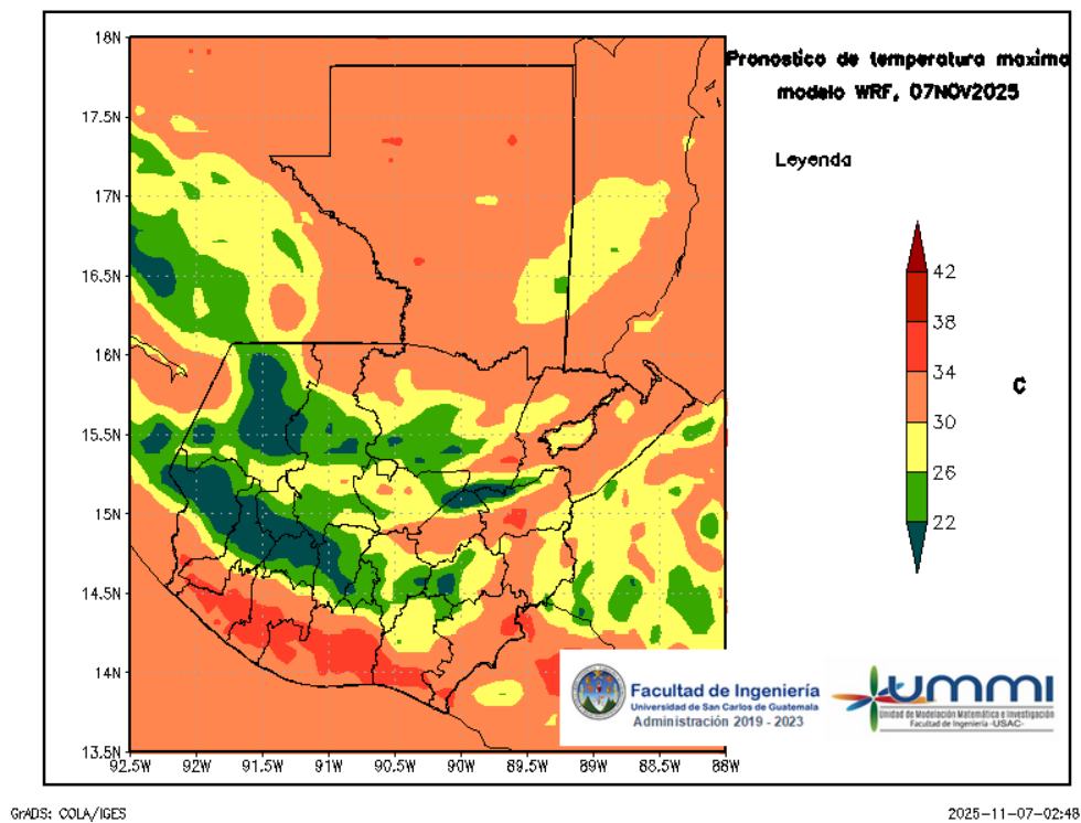
Figura 4: Pronóstico de temperatura máxima diaria del 07 de November
