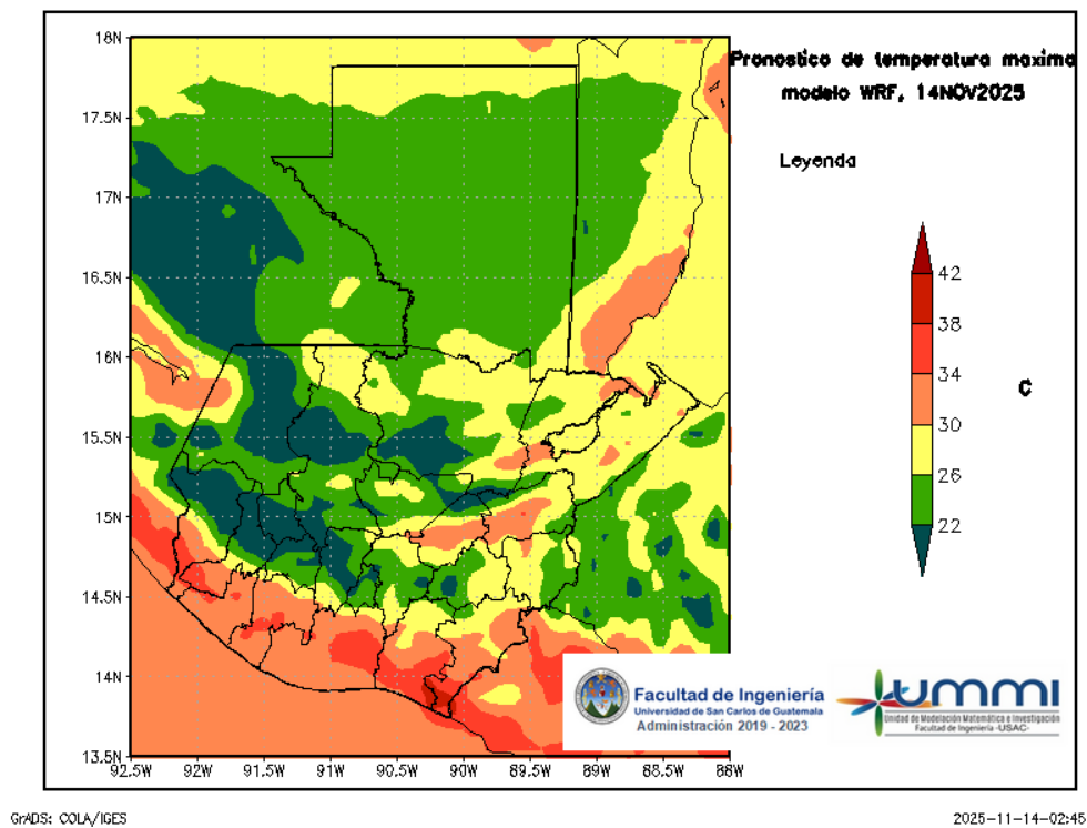
Figura 4: Pronóstico de temperatura máxima diaria del 14 de November
