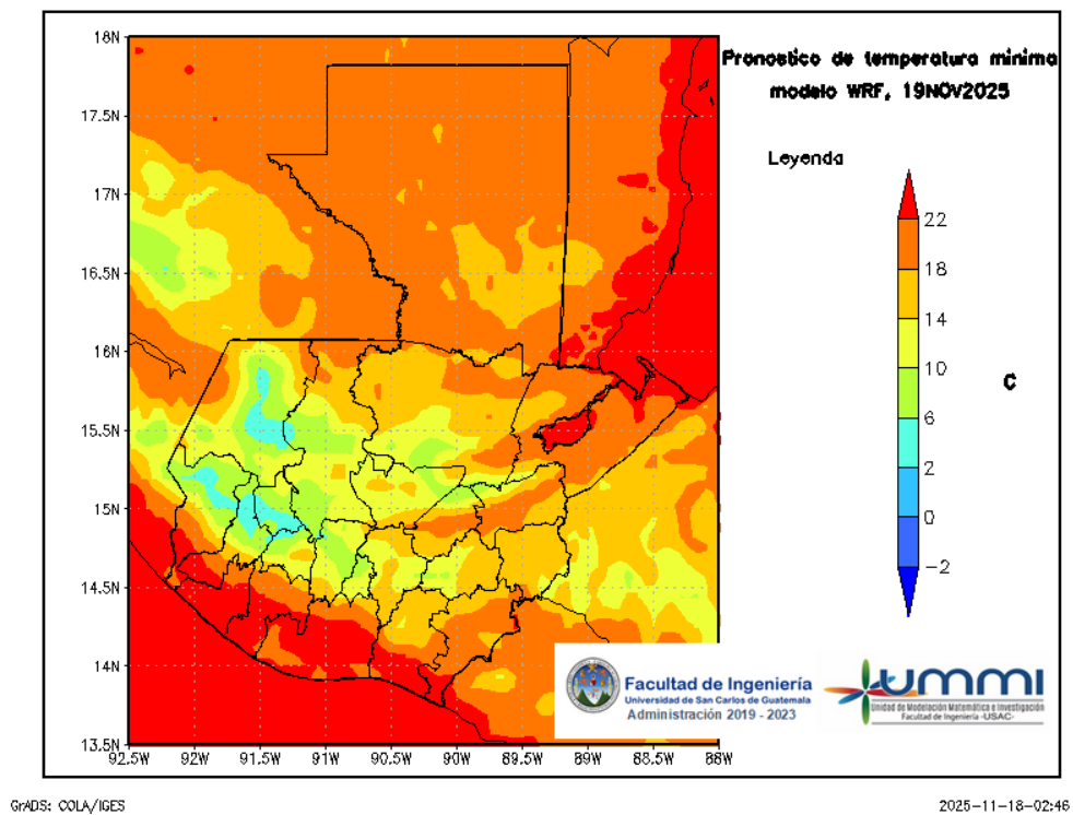
Figura 8: Pronóstico de temperatura mínima diaria del 20 de November
