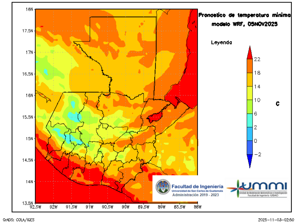
Figura 9: Pronóstico de temperatura mínima diaria del 06 de November
