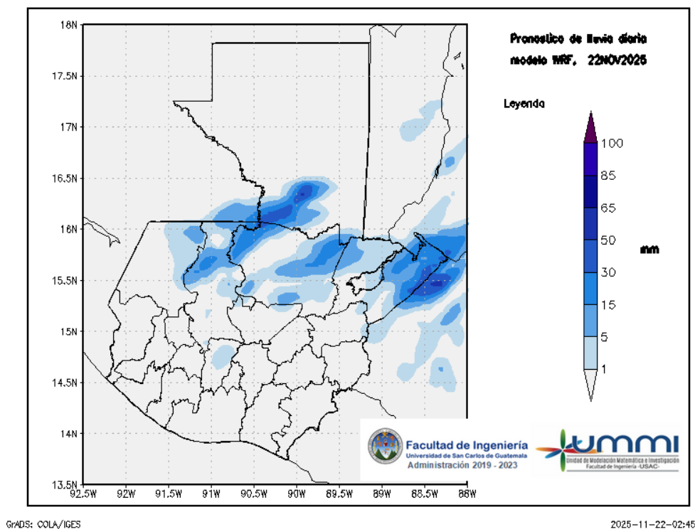
Figura 1: Pronóstico de lluvia diaria del 22 de November
