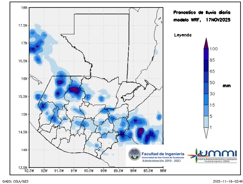
Figura 3: Pronóstico de lluvia diaria del 17 de November
