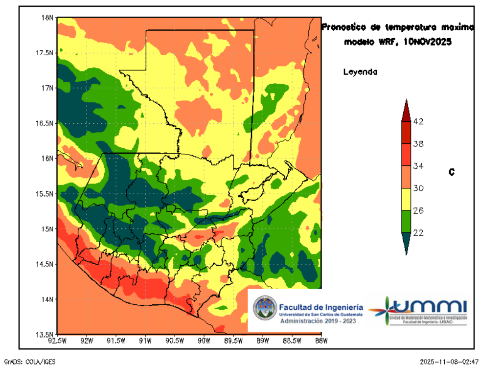
Figura 6: Pronóstico de temperatura máxima diaria del 10 de November
