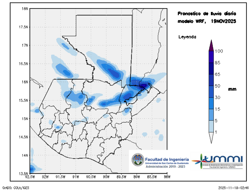
Figura 2: Pronóstico de lluvia diaria del 19 de November
