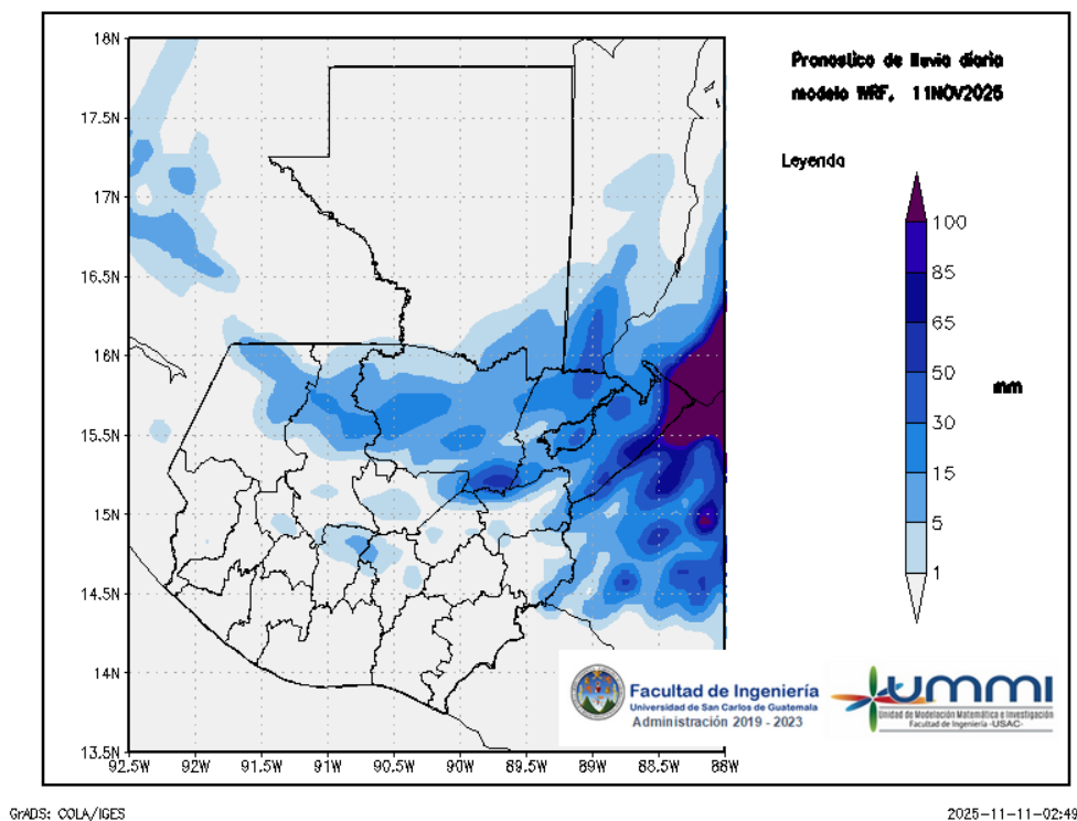
Figura 1: Pronóstico de lluvia diaria del 11 de November
