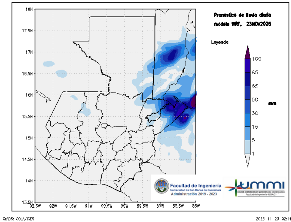
Figura 1: Pronóstico de lluvia diaria del 23 de November
