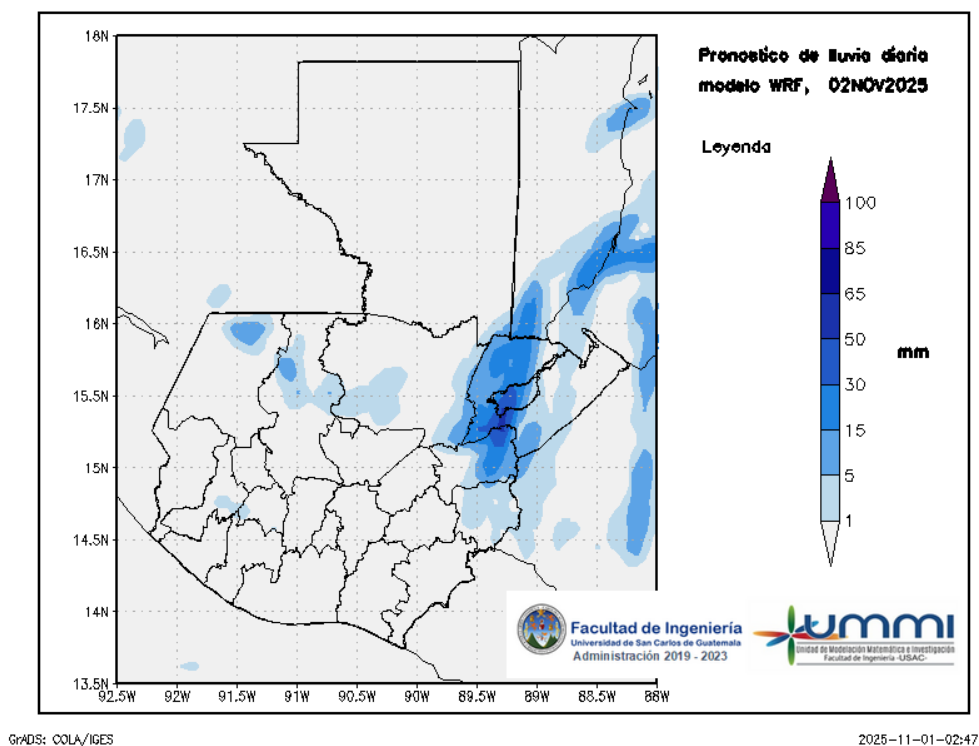
Figura 2: Pronóstico de lluvia diaria del 02 de November
