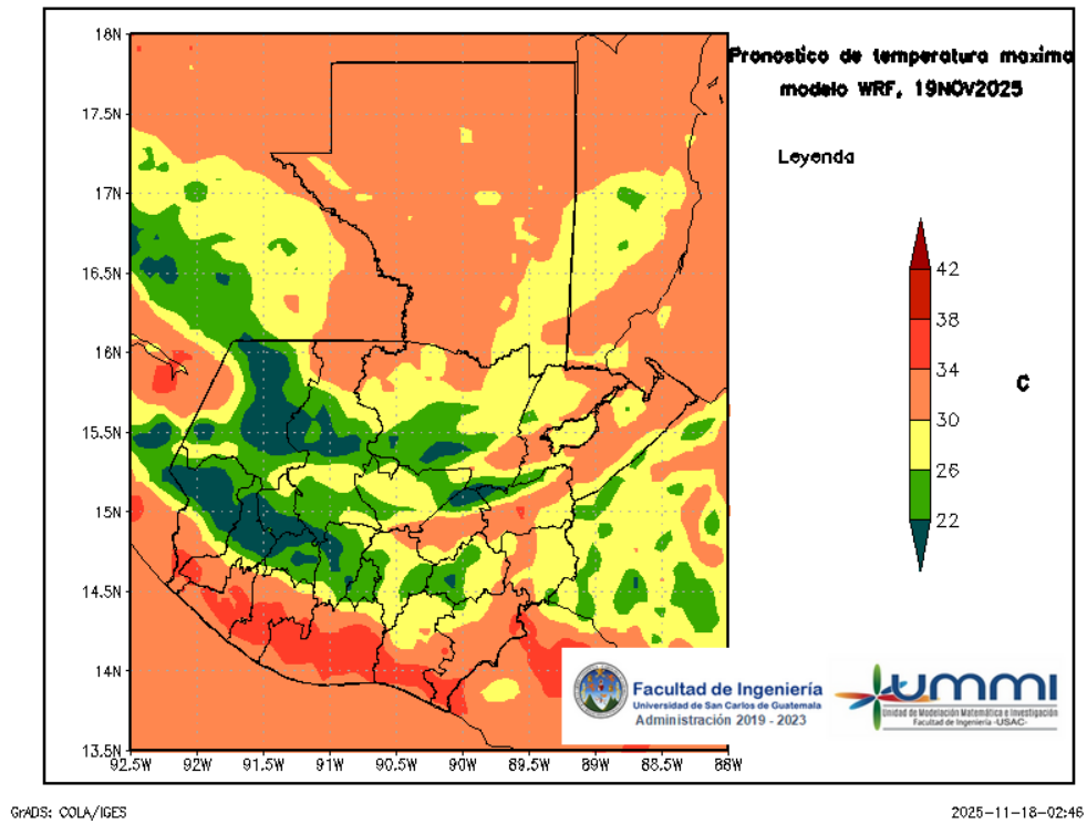
Figura 5: Pronóstico de temperatura máxima diaria del 19 de November
