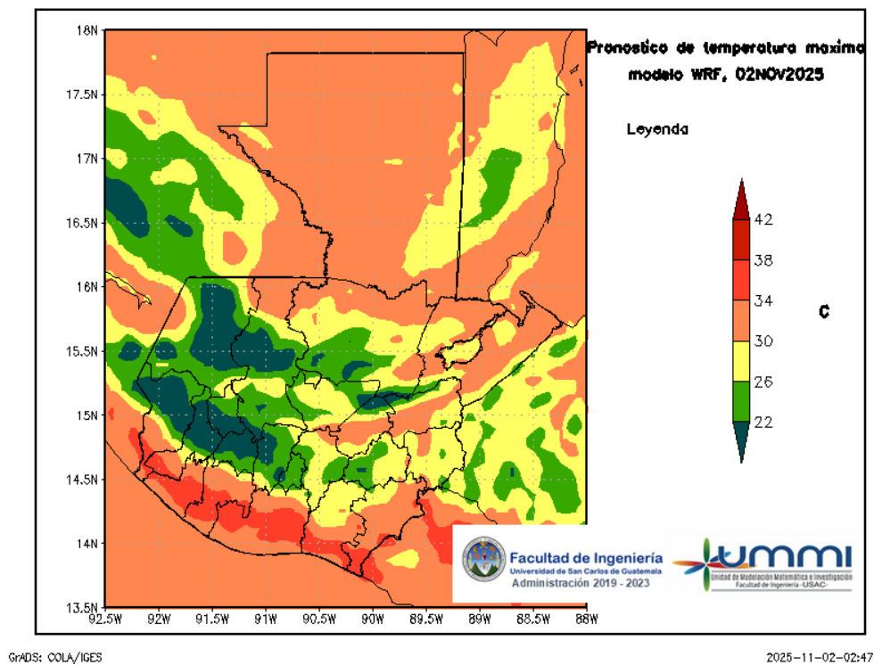
Figura 4: Pronóstico de temperatura máxima diaria del 02 de November
