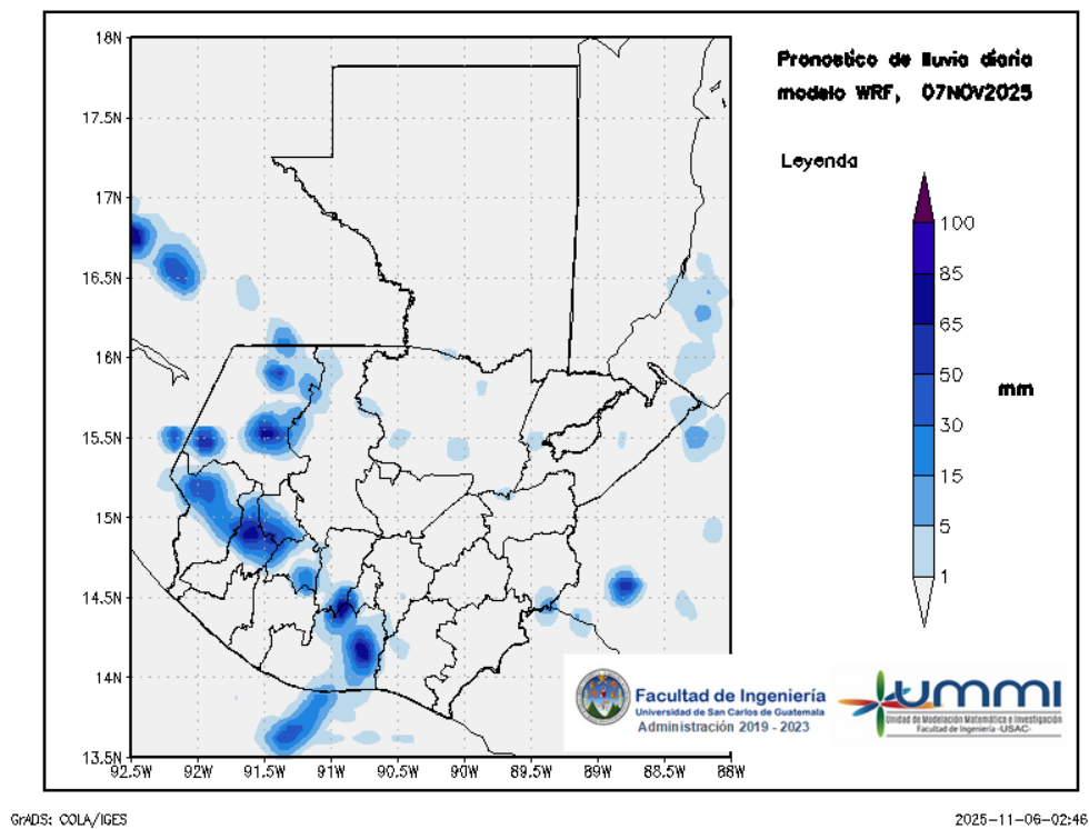
Figura 2: Pronóstico de lluvia diaria del 07 de November
