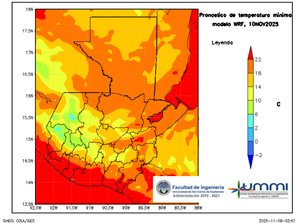
Figura 9: Pronóstico de temperatura mínima diaria del 11 de November
