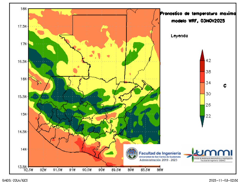
Figura 4: Pronóstico de temperatura máxima diaria del 03 de November
