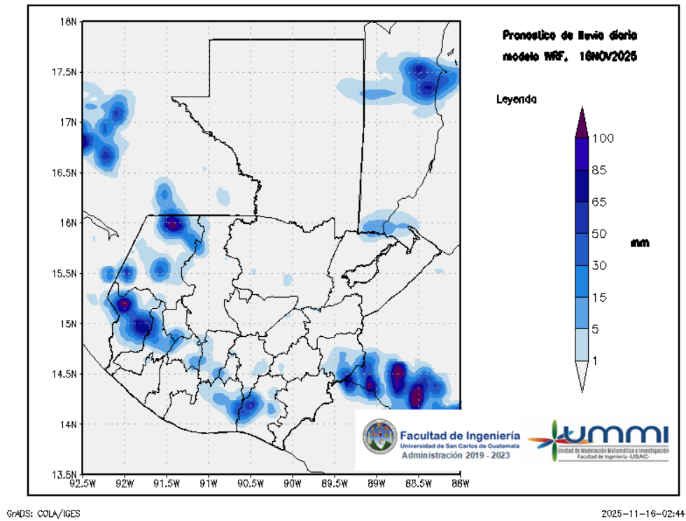
Figura 1: Pronóstico de lluvia diaria del 16 de November
