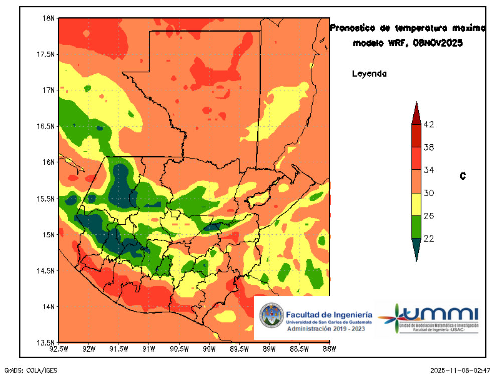
Figura 4: Pronóstico de temperatura máxima diaria del 08 de November
