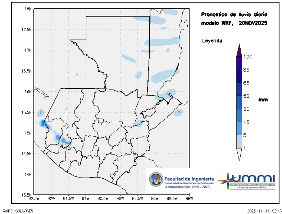
Figura 3: Pronóstico de lluvia diaria del 20 de November
