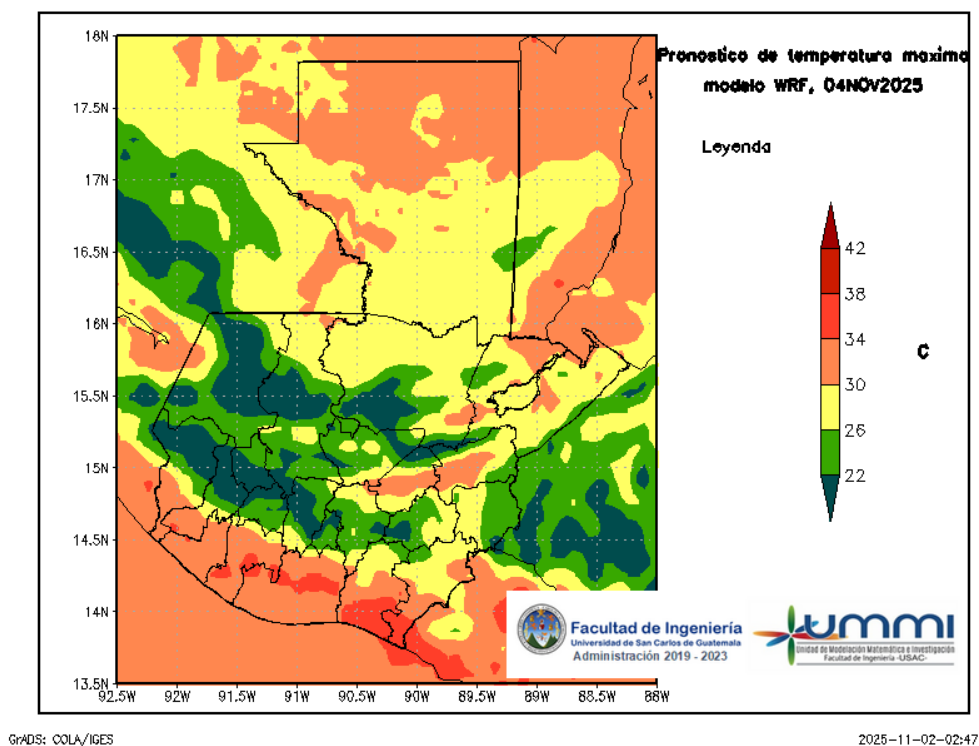
Figura 6: Pronóstico de temperatura máxima diaria del 04 de November
