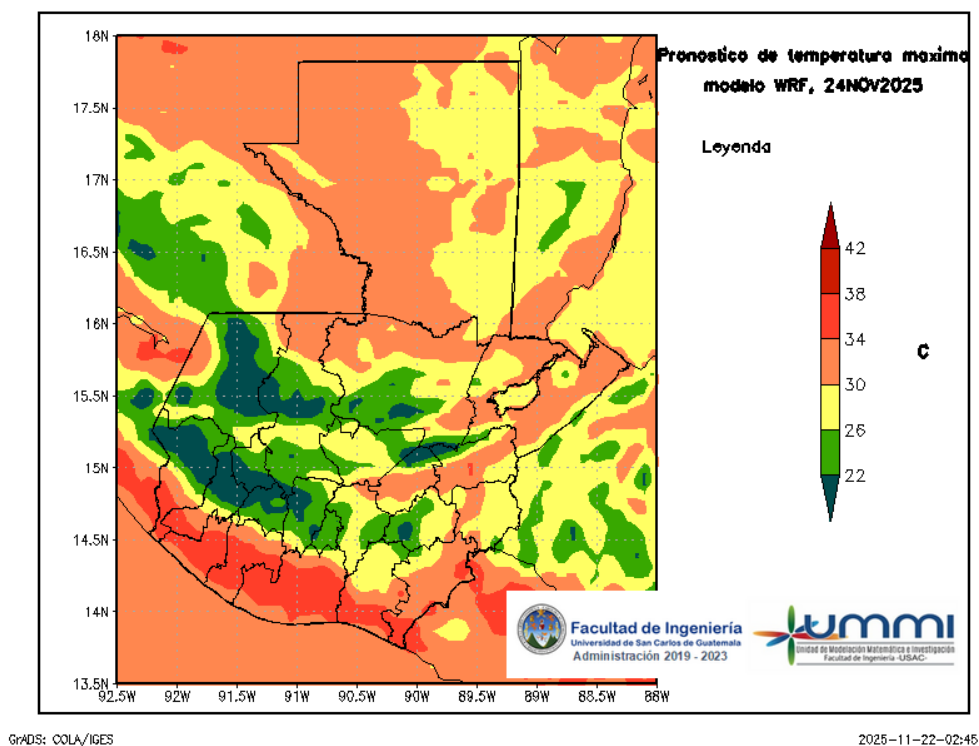
Figura 6: Pronóstico de temperatura máxima diaria del 24 de November
