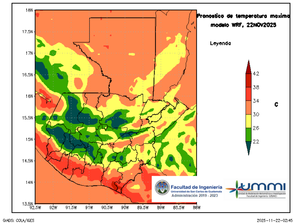
Figura 4: Pronóstico de temperatura máxima diaria del 22 de November
