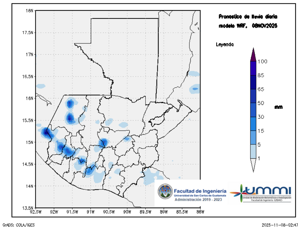
Figura 1: Pronóstico de lluvia diaria del 08 de November
