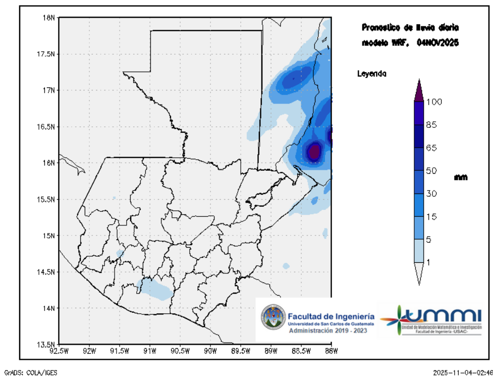
Figura 1: Pronóstico de lluvia diaria del 04 de November
