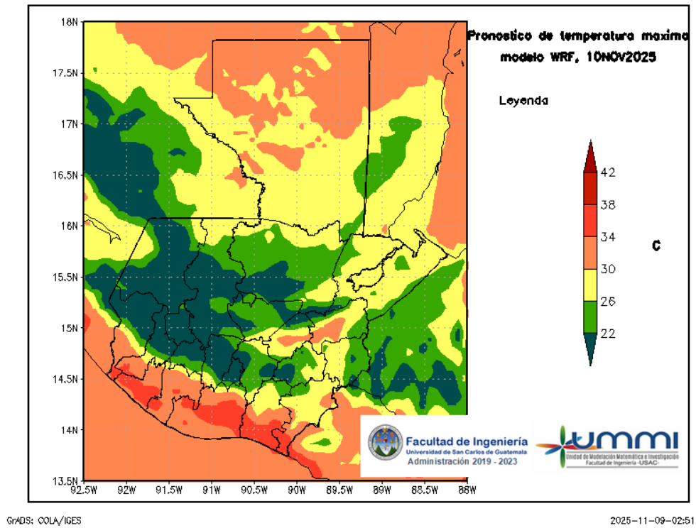
Figura 5: Pronóstico de temperatura máxima diaria del 10 de November
