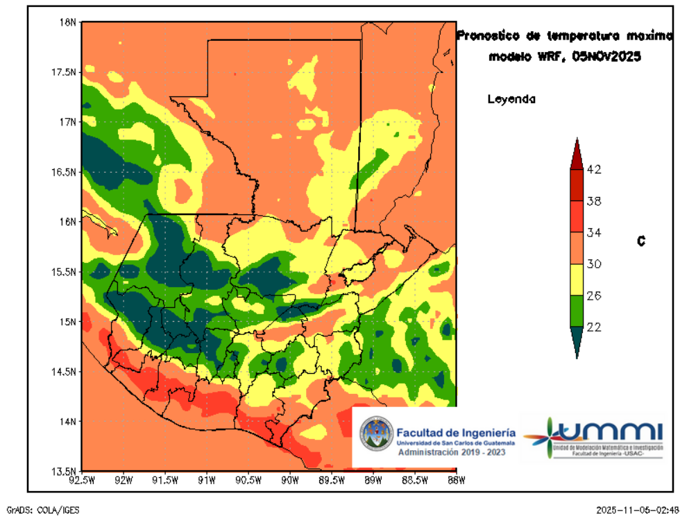
Figura 4: Pronóstico de temperatura máxima diaria del 05 de November
