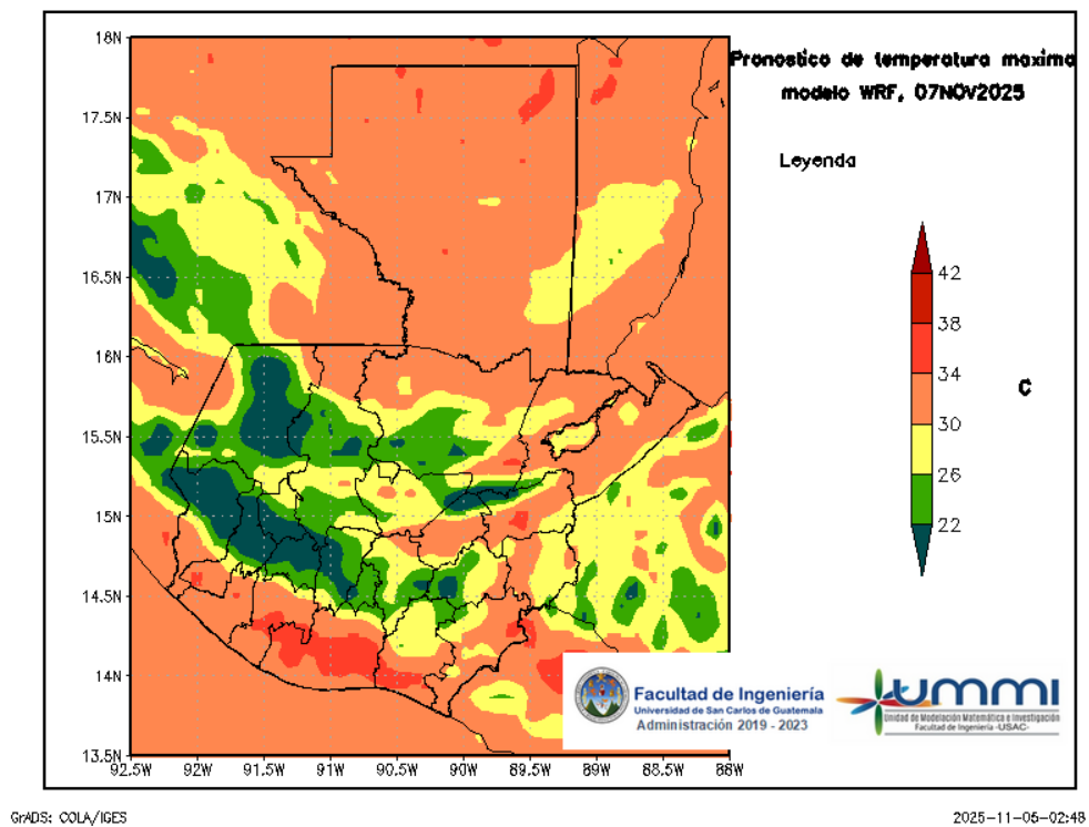
Figura 6: Pronóstico de temperatura máxima diaria del 07 de November
