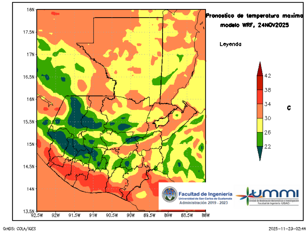
Figura 5: Pronóstico de temperatura máxima diaria del 24 de November
