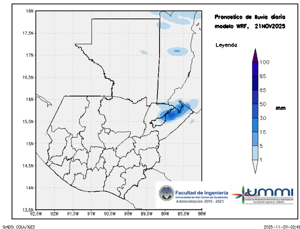
Figura 2: Pronóstico de lluvia diaria del 21 de November
