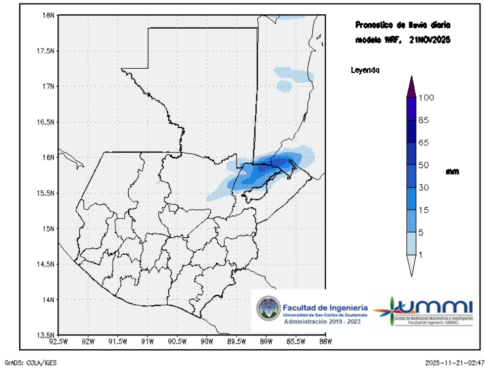
Figura 1: Pronóstico de lluvia diaria del 21 de November
