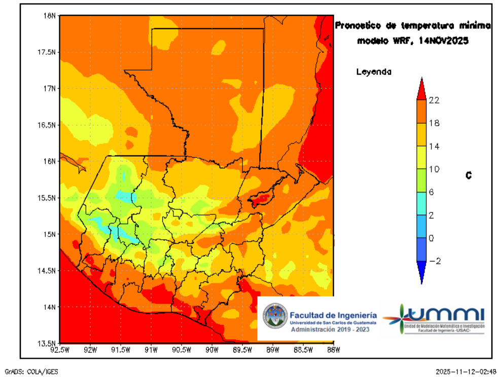
Figura 9: Pronóstico de temperatura mínima diaria del 15 de November
