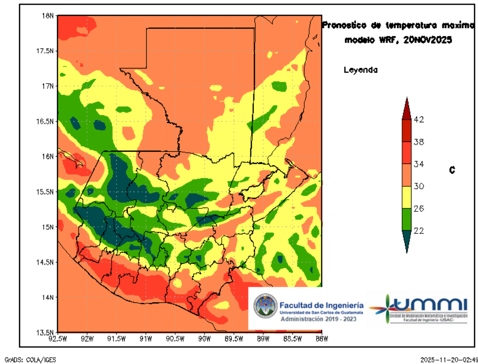
Figura 4: Pronóstico de temperatura máxima diaria del 20 de November
