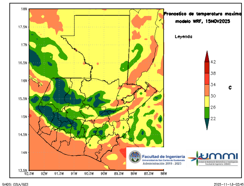
Figura 6: Pronóstico de temperatura máxima diaria del 15 de November
