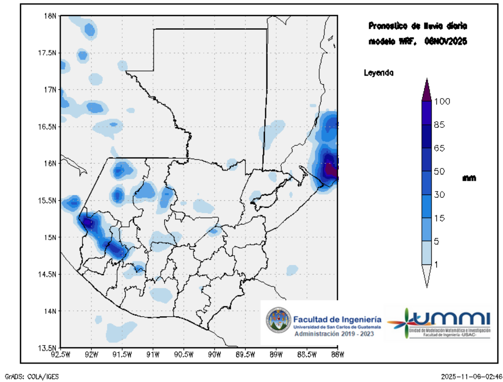
Figura 1: Pronóstico de lluvia diaria del 06 de November
