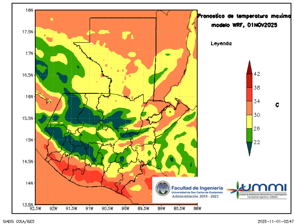
Figura 4: Pronóstico de temperatura máxima diaria del 01 de November
