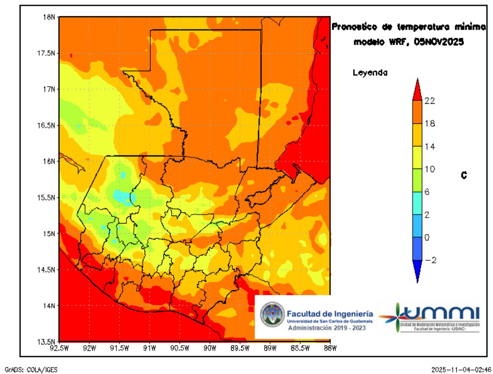
Figura 8: Pronóstico de temperatura mínima diaria del 06 de November
