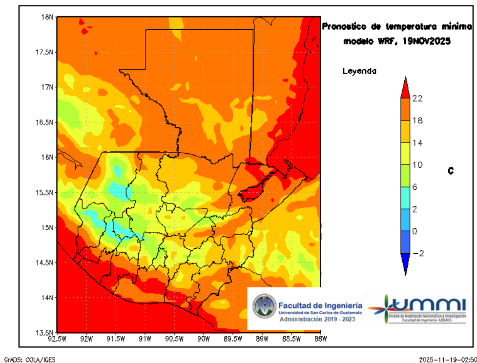
Figura 7: Pronóstico de temperatura mínima diaria del 20 de November
