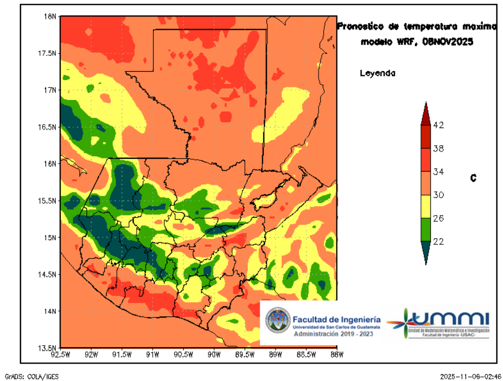
Figura 6: Pronóstico de temperatura máxima diaria del 08 de November
