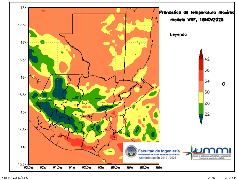
Figura 4: Pronóstico de temperatura máxima diaria del 16 de November
