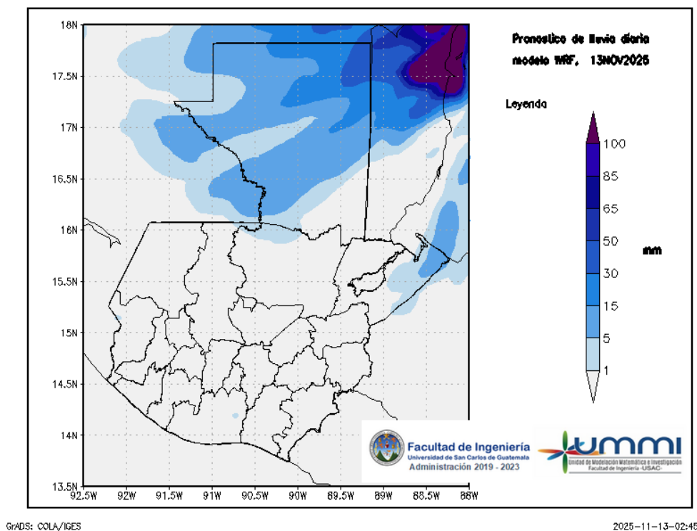
Figura 1: Pronóstico de lluvia diaria del 13 de November
