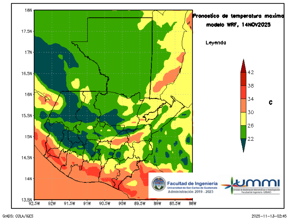
Figura 5: Pronóstico de temperatura máxima diaria del 14 de November
