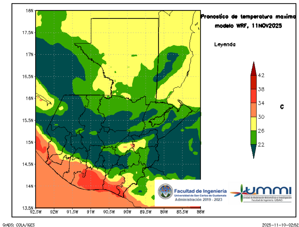
Figura 5: Pronóstico de temperatura máxima diaria del 11 de November
