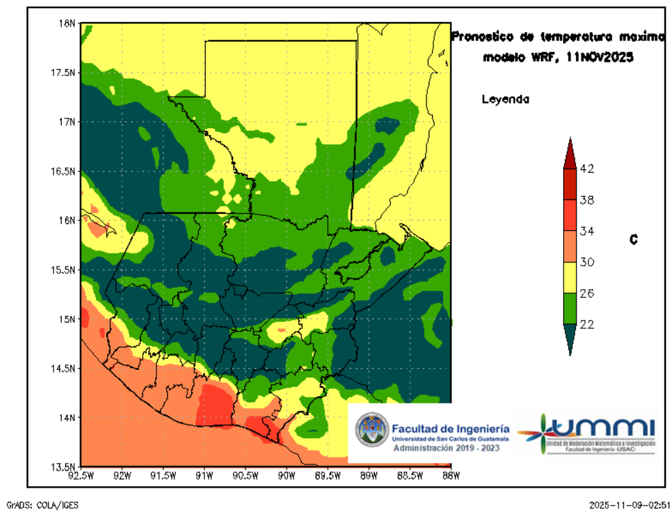
Figura 6: Pronóstico de temperatura máxima diaria del 11 de November
