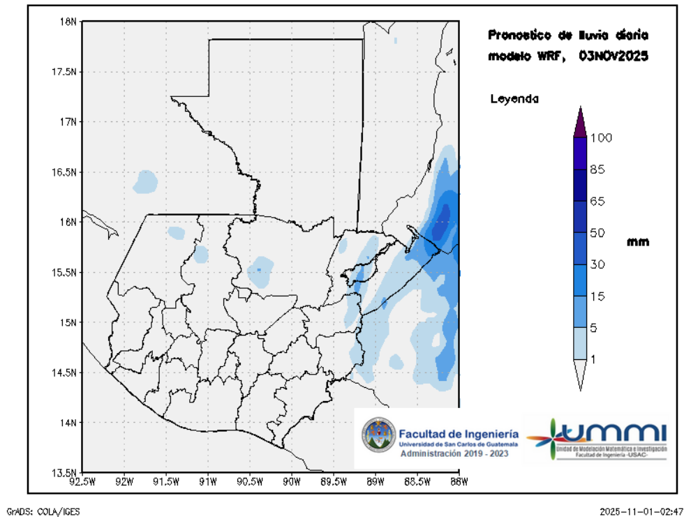
Figura 3: Pronóstico de lluvia diaria del 03 de November
