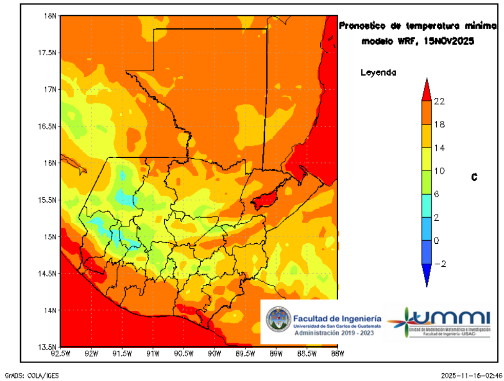
Figura 7: Pronóstico de temperatura mínima diaria del 16 de November
