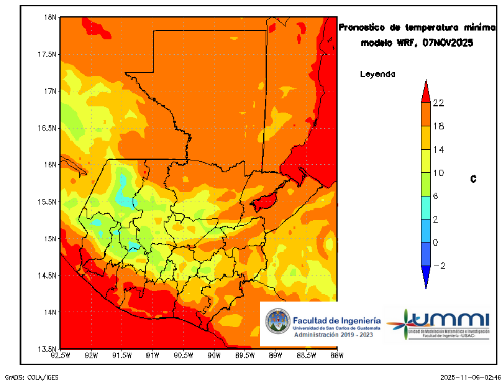
Figura 8: Pronóstico de temperatura mínima diaria del 08 de November
