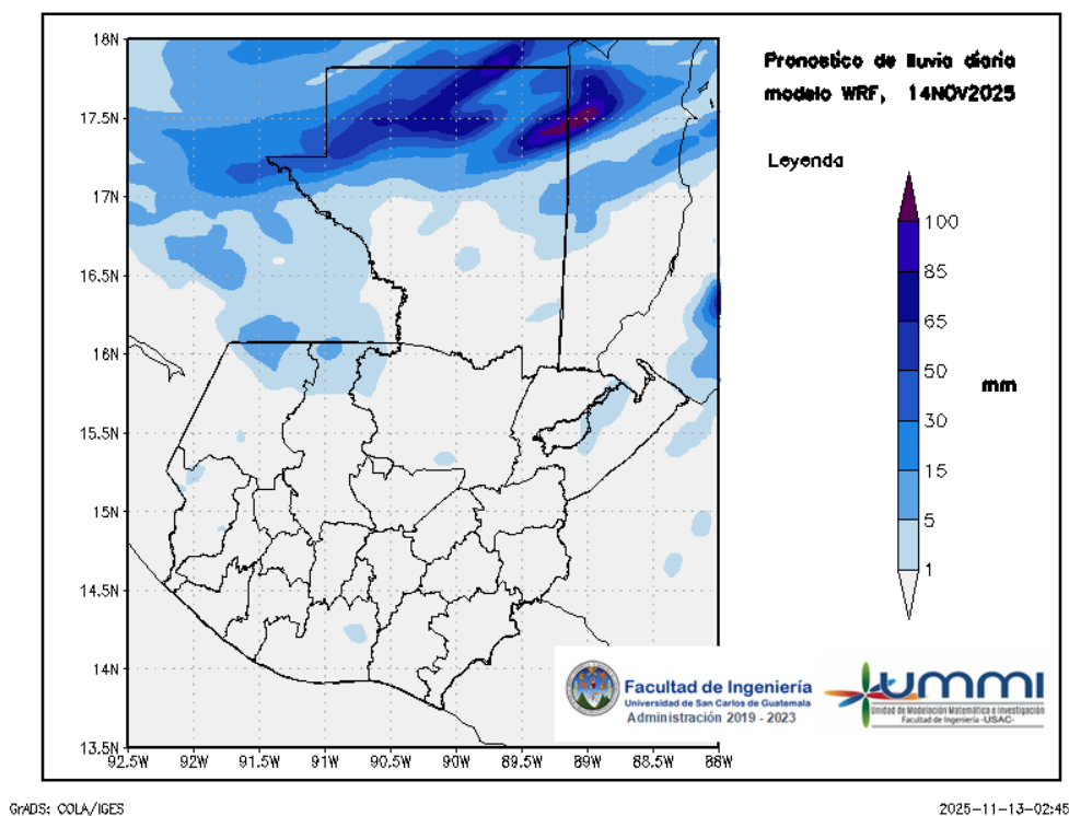
Figura 2: Pronóstico de lluvia diaria del 14 de November
