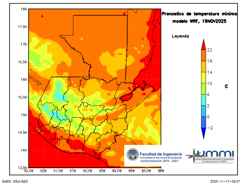
Figura 9: Pronóstico de temperatura mínima diaria del 20 de November
