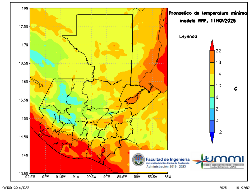
Figura 8: Pronóstico de temperatura mínima diaria del 12 de November
