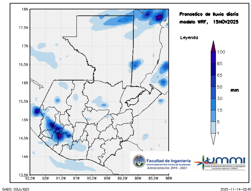
Figura 2: Pronóstico de lluvia diaria del 15 de November
