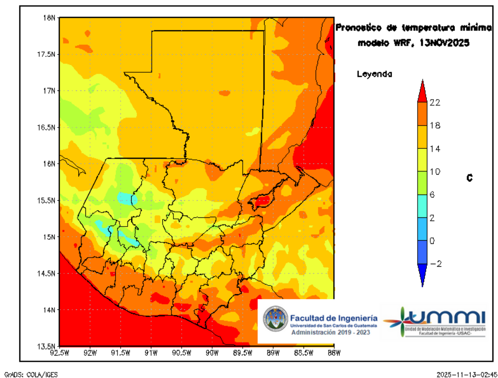
Figura 7: Pronóstico de temperatura mínima diaria del 14 de November
