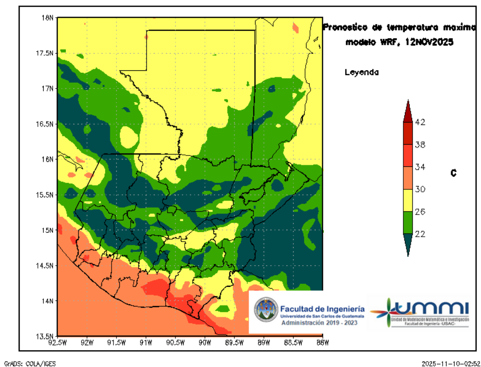
Figura 6: Pronóstico de temperatura máxima diaria del 12 de November
