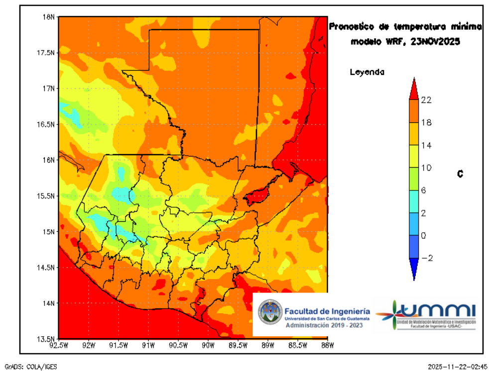
Figura 8: Pronóstico de temperatura mínima diaria del 24 de November
