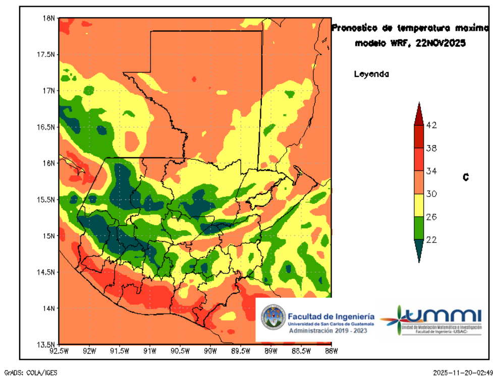
Figura 6: Pronóstico de temperatura máxima diaria del 22 de November
