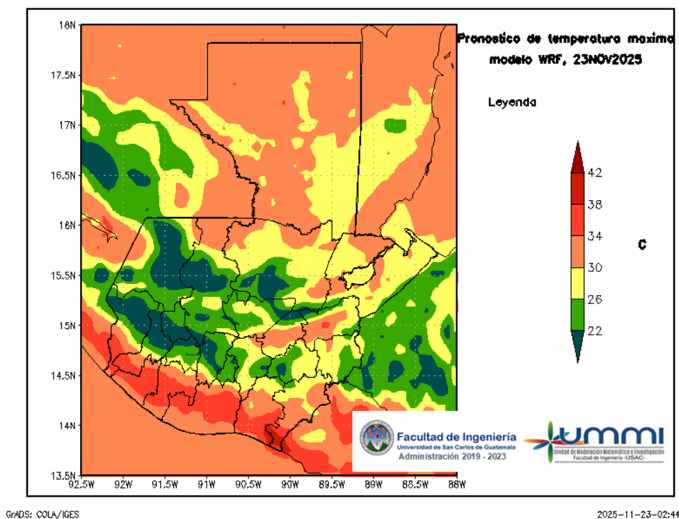
Figura 4: Pronóstico de temperatura máxima diaria del 23 de November
