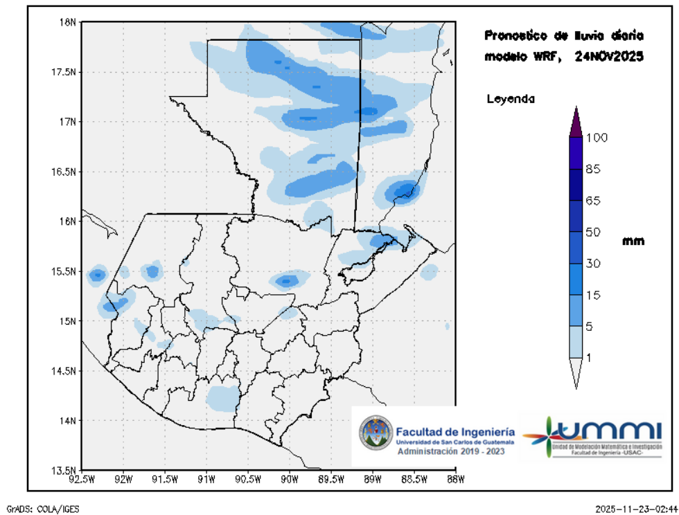
Figura 2: Pronóstico de lluvia diaria del 24 de November
