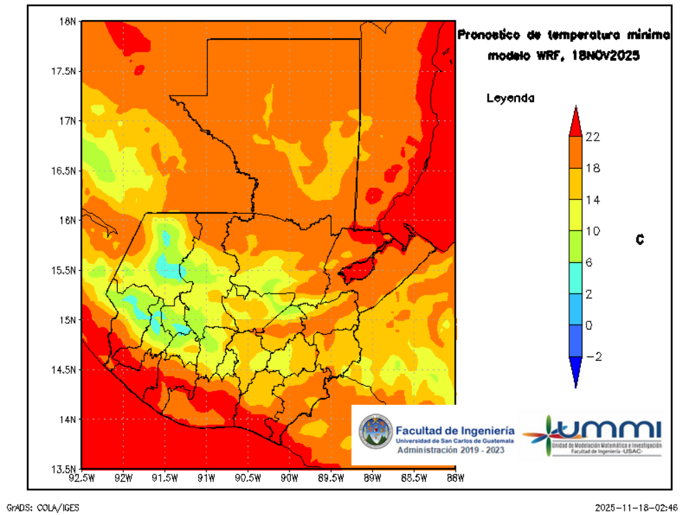
Figura 7: Pronóstico de temperatura mínima diaria del 19 de November
