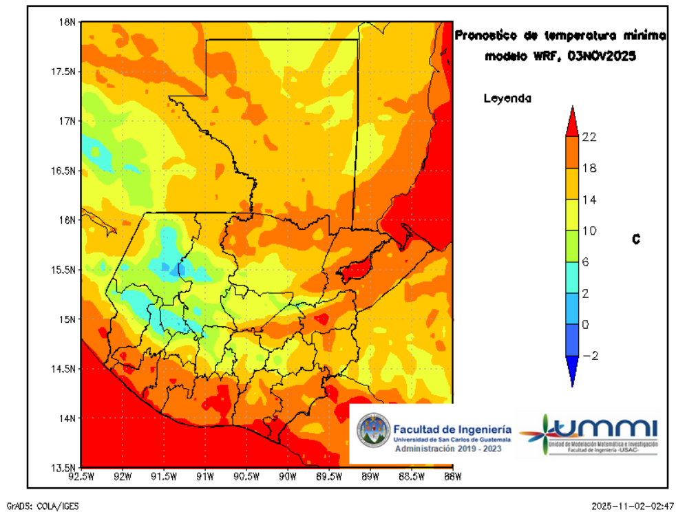
Figura 8: Pronóstico de temperatura mínima diaria del 04 de November
