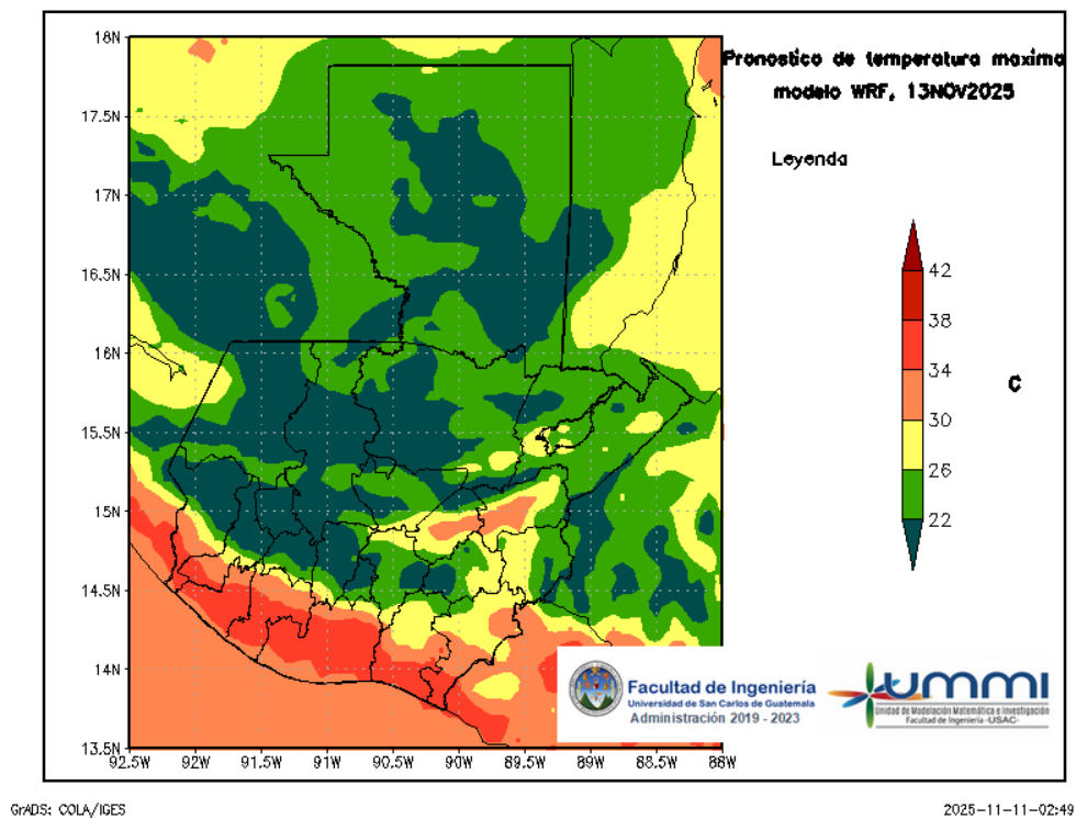
Figura 6: Pronóstico de temperatura máxima diaria del 13 de November
