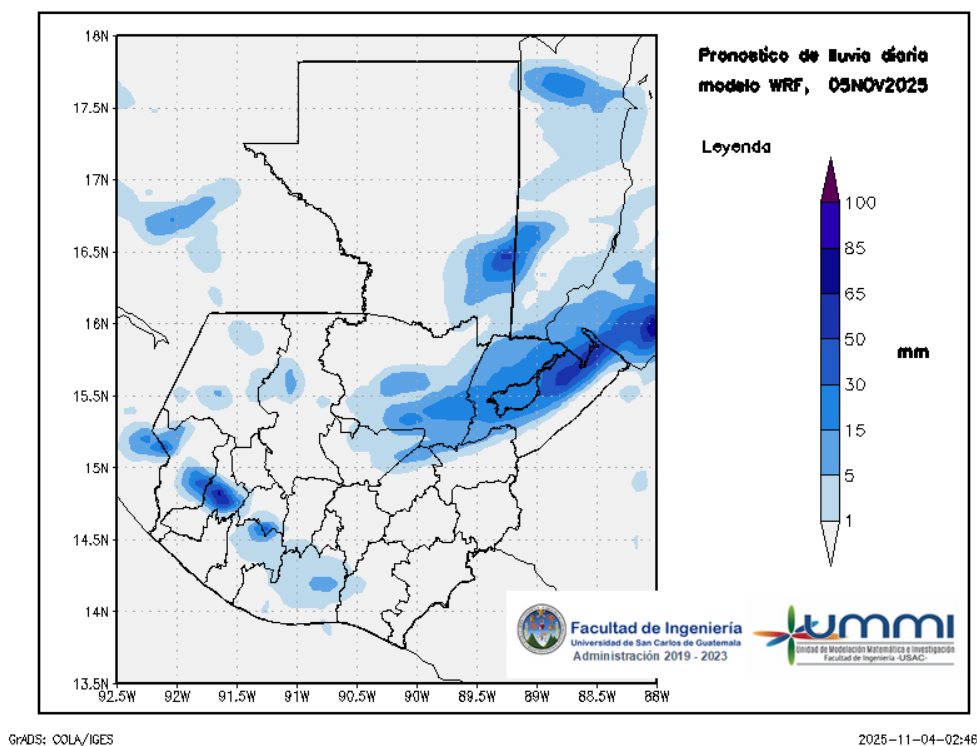
Figura 2: Pronóstico de lluvia diaria del 05 de November
