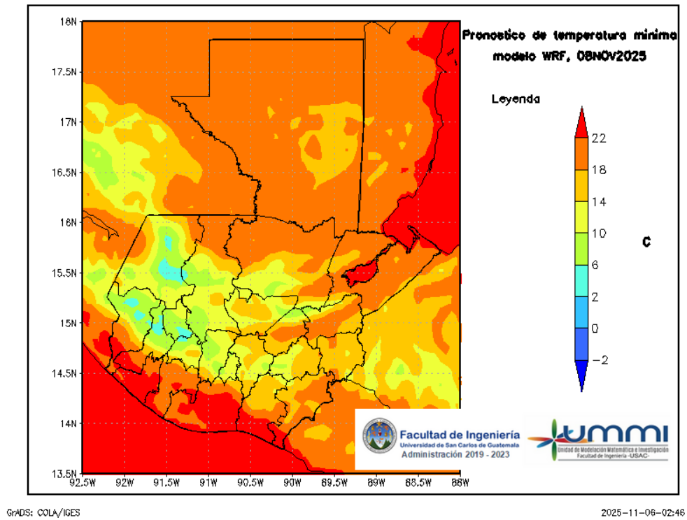
Figura 9: Pronóstico de temperatura mínima diaria del 09 de November
