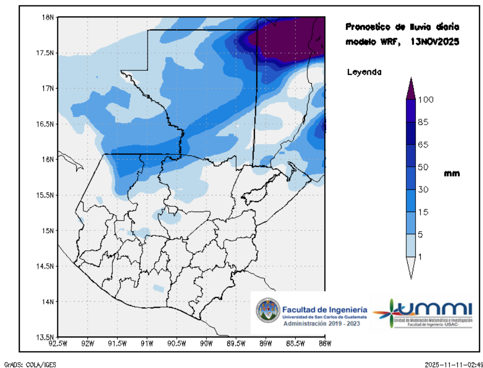
Figura 3: Pronóstico de lluvia diaria del 13 de November
