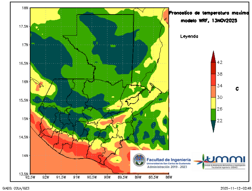
Figura 5: Pronóstico de temperatura máxima diaria del 13 de November
