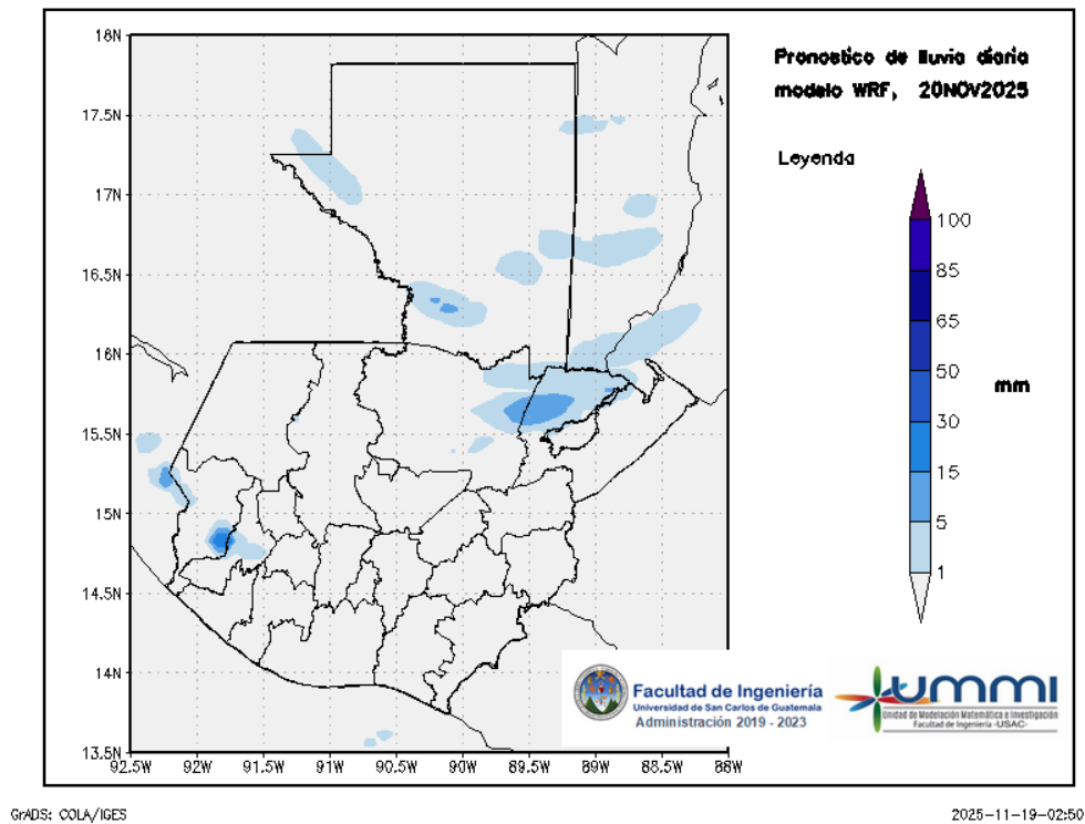
Figura 2: Pronóstico de lluvia diaria del 20 de November
