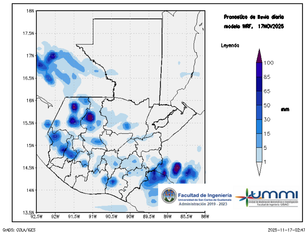
Figura 1: Pronóstico de lluvia diaria del 17 de November
