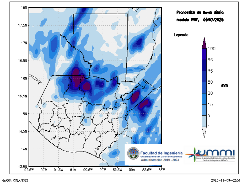
Figura 1: Pronóstico de lluvia diaria del 09 de November
