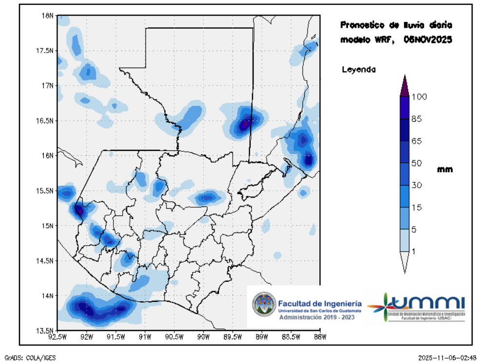
Figura 2: Pronóstico de lluvia diaria del 06 de November
