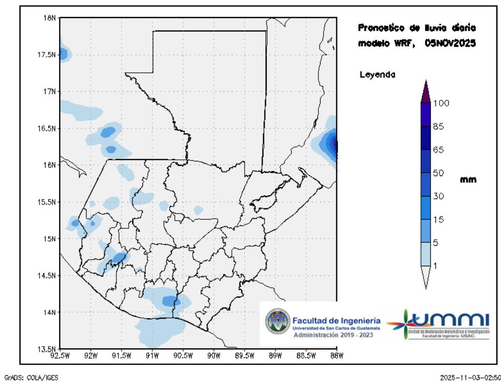
Figura 3: Pronóstico de lluvia diaria del 05 de November
