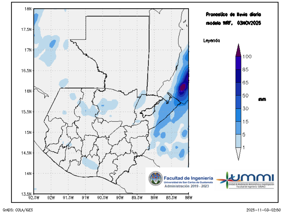
Figura 1: Pronóstico de lluvia diaria del 03 de November
