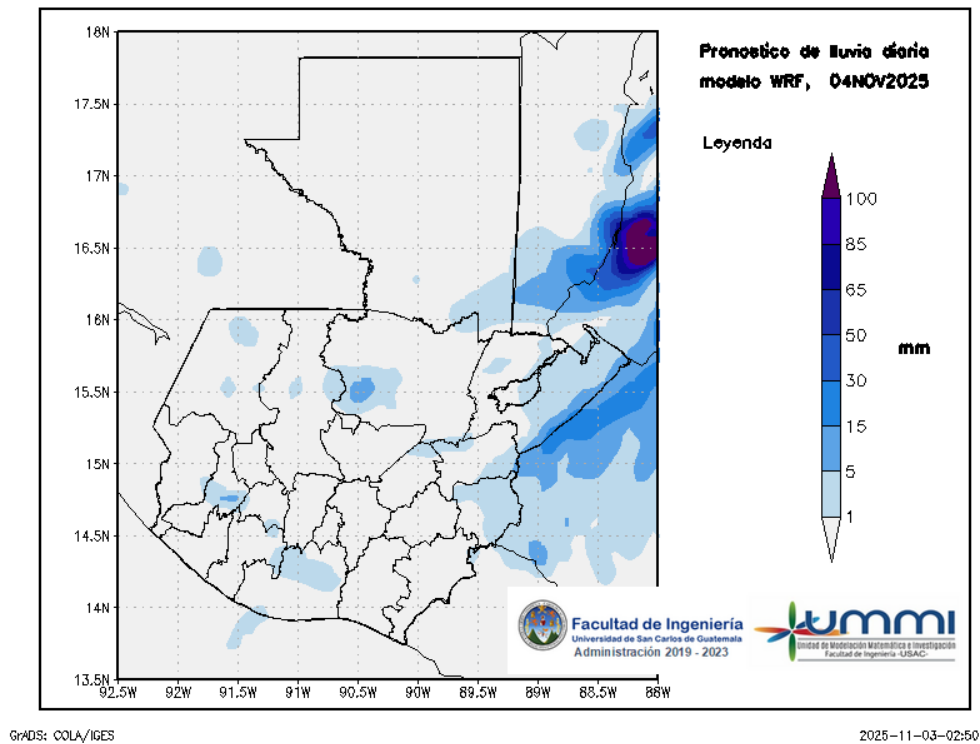
Figura 2: Pronóstico de lluvia diaria del 04 de November
