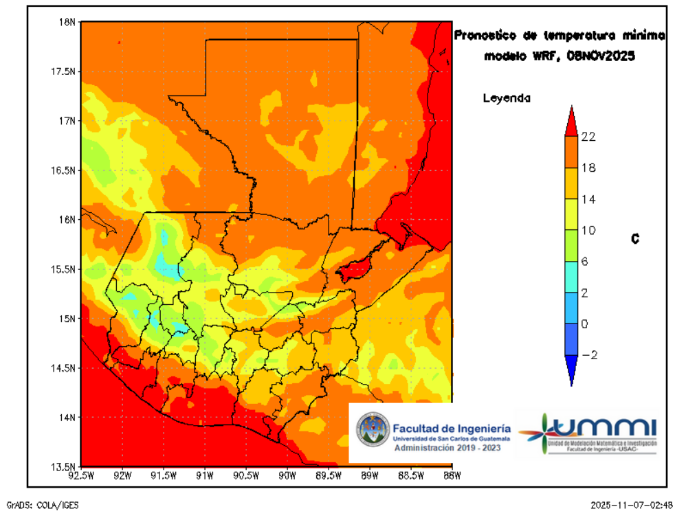
Figura 8: Pronóstico de temperatura mínima diaria del 09 de November
