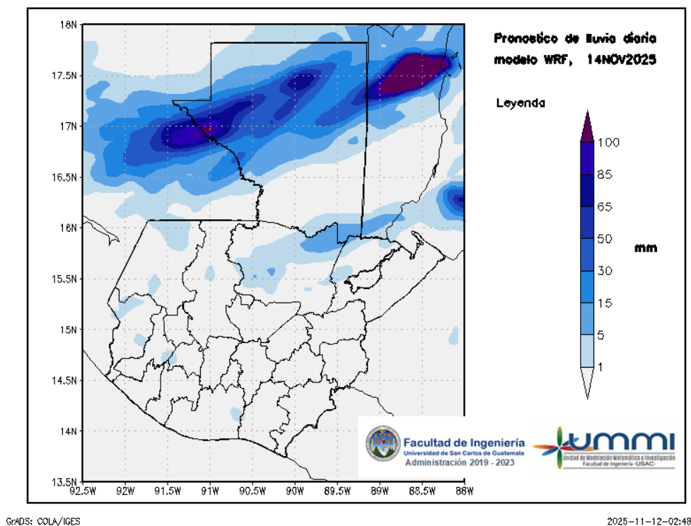
Figura 3: Pronóstico de lluvia diaria del 14 de November
