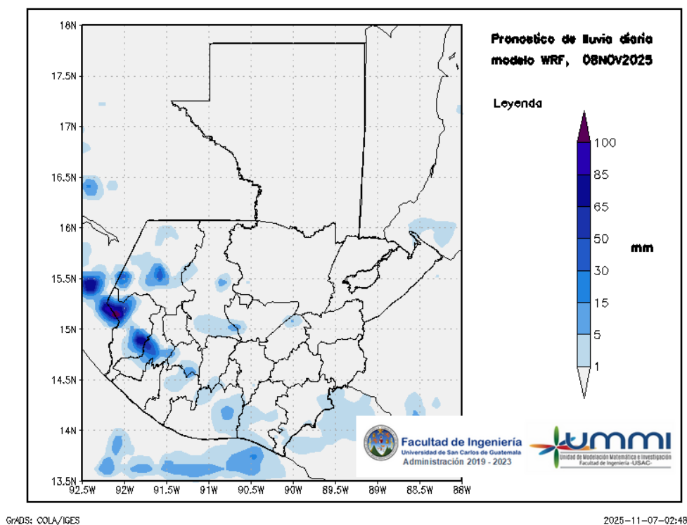
Figura 2: Pronóstico de lluvia diaria del 08 de November
