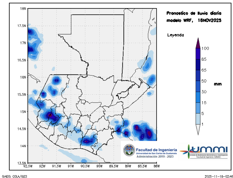
Figura 2: Pronóstico de lluvia diaria del 16 de November
