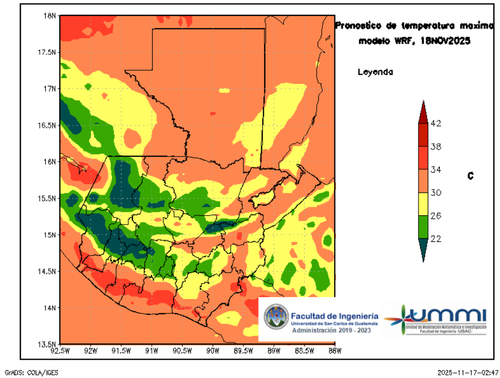
Figura 5: Pronóstico de temperatura máxima diaria del 18 de November
