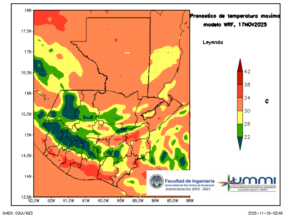
Figura 6: Pronóstico de temperatura máxima diaria del 17 de November
