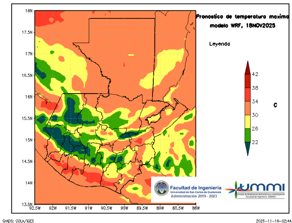
Figura 6: Pronóstico de temperatura máxima diaria del 18 de November
