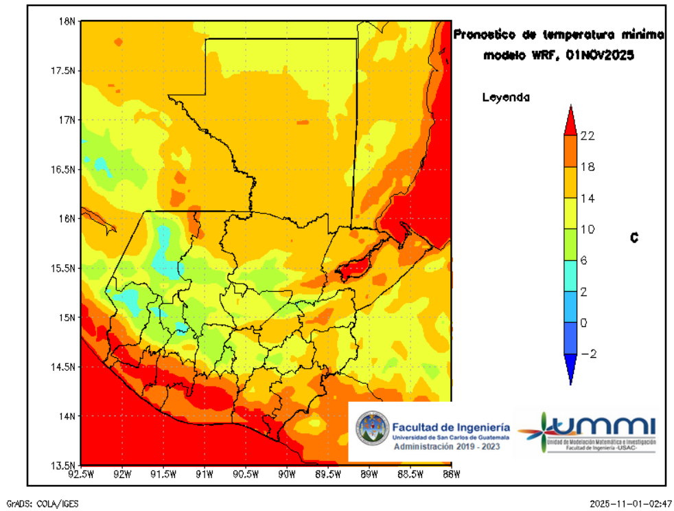
Figura 7: Pronóstico de temperatura mínima diaria del 02 de November
