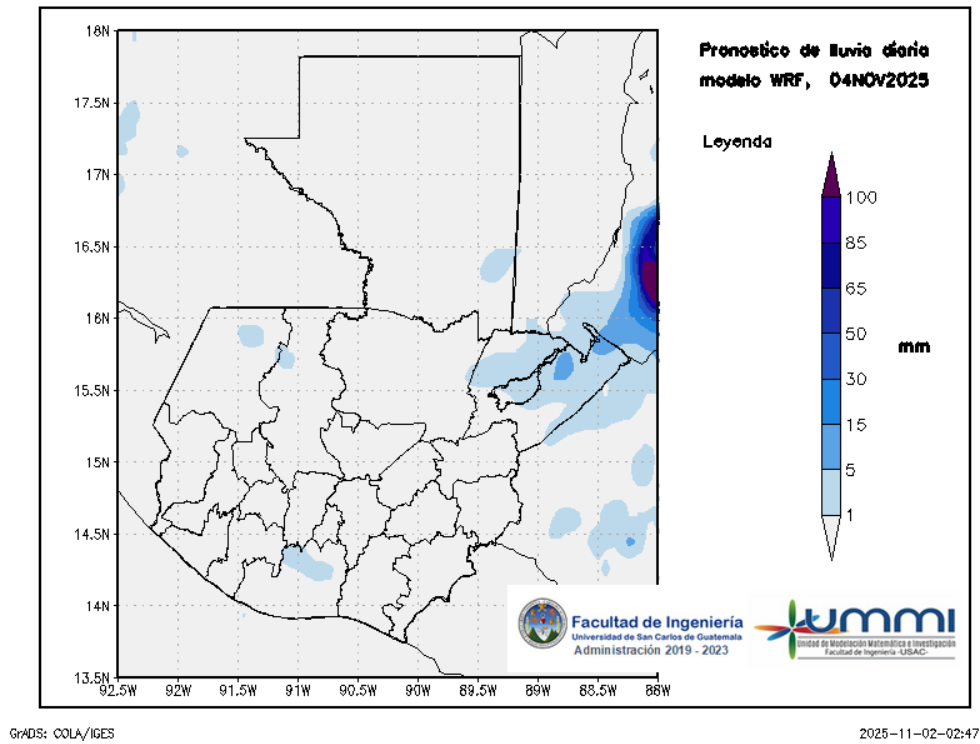
Figura 3: Pronóstico de lluvia diaria del 04 de November
