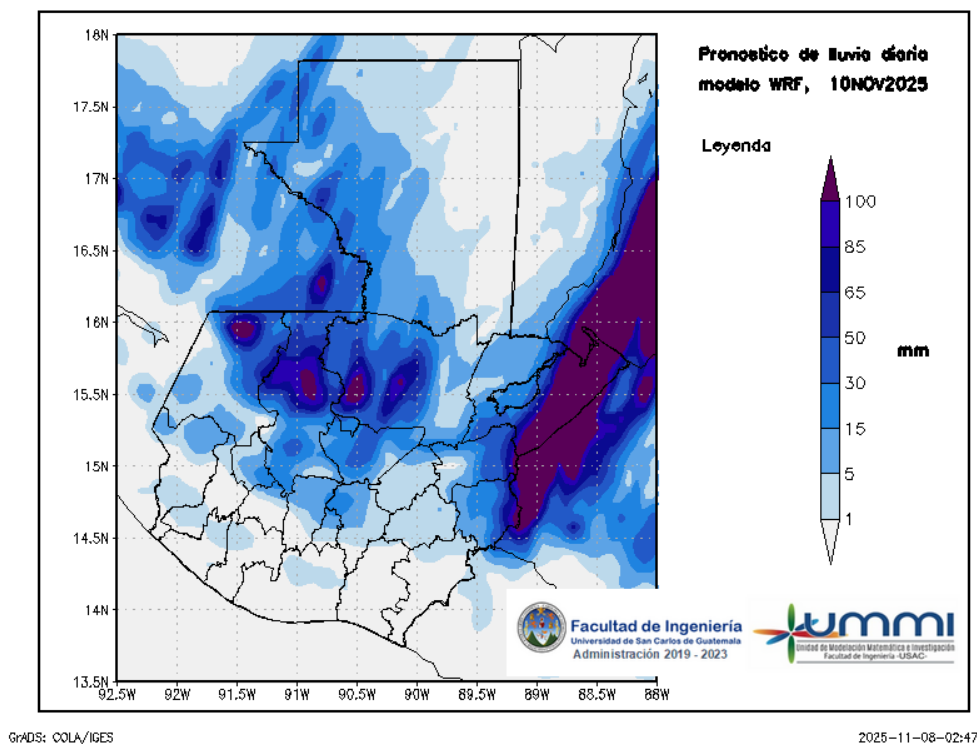
Figura 3: Pronóstico de lluvia diaria del 10 de November
