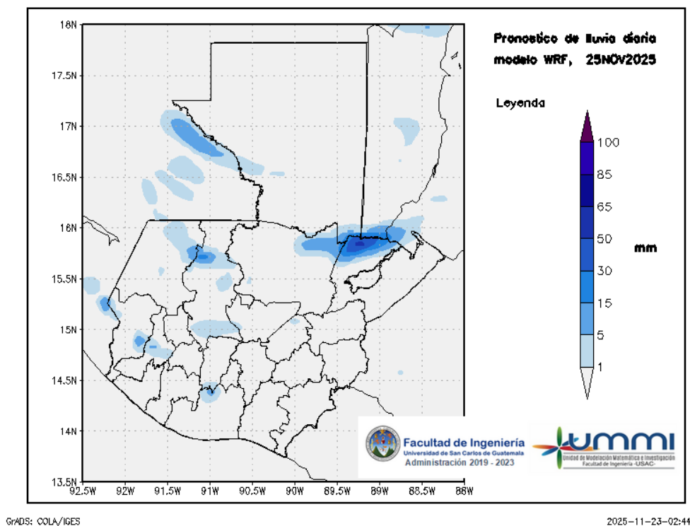
Figura 3: Pronóstico de lluvia diaria del 25 de November
