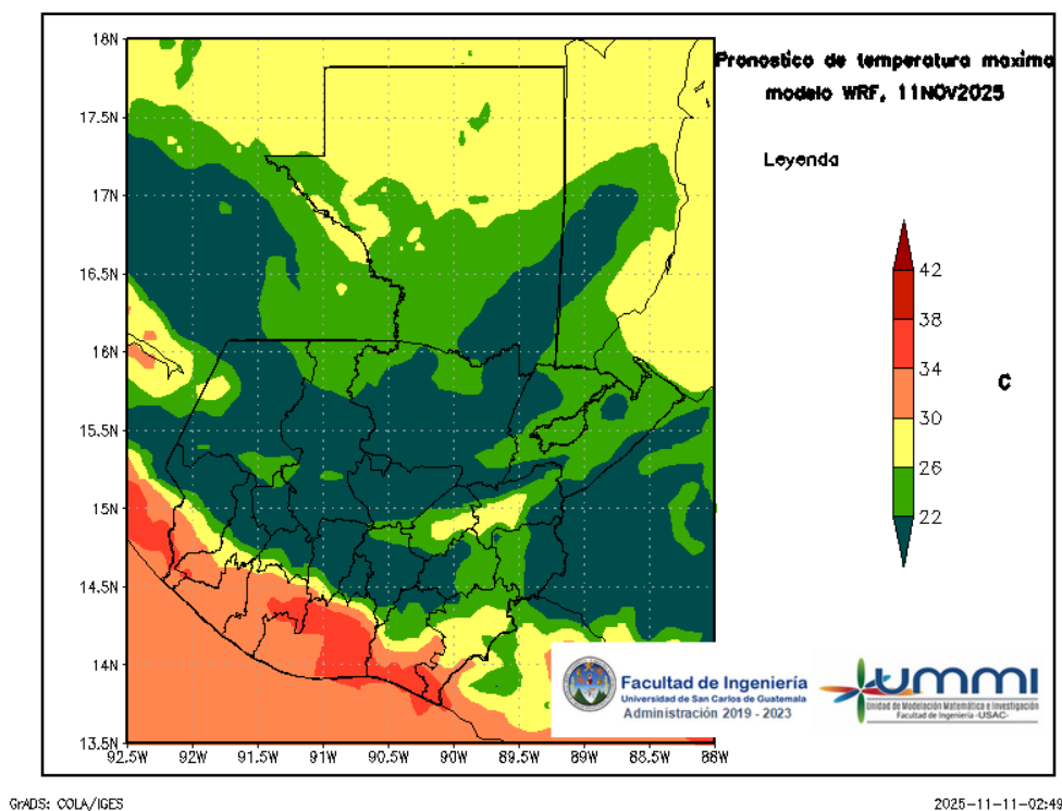
Figura 4: Pronóstico de temperatura máxima diaria del 11 de November
