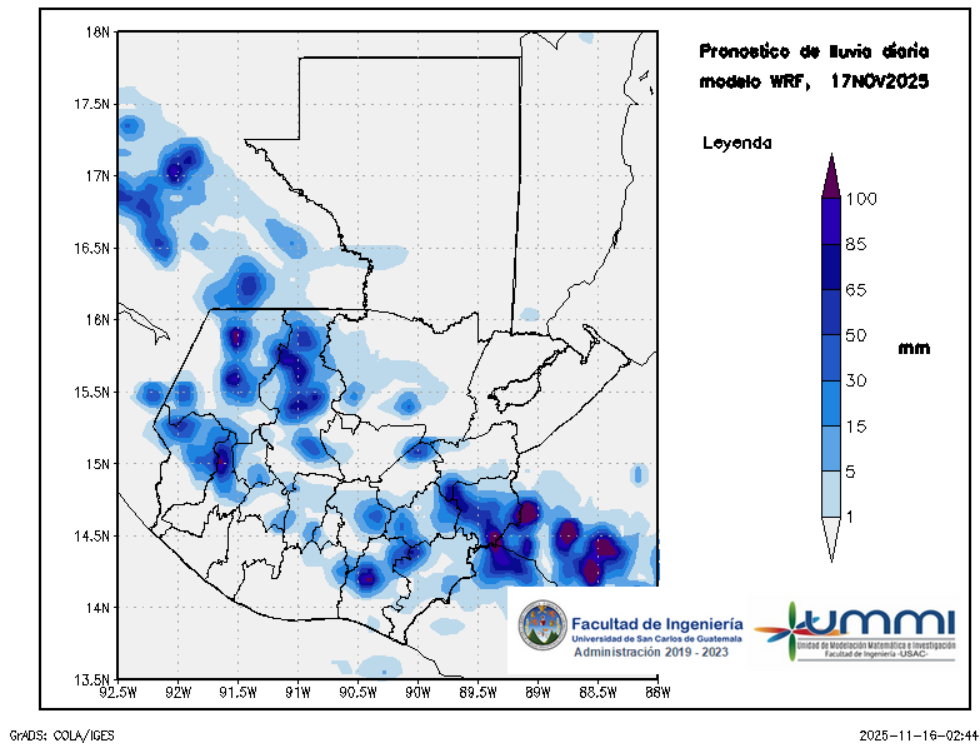
Figura 2: Pronóstico de lluvia diaria del 17 de November
