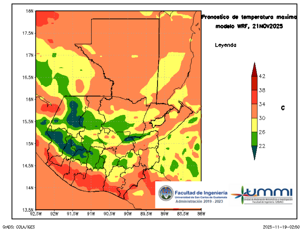
Figura 6: Pronóstico de temperatura máxima diaria del 21 de November
