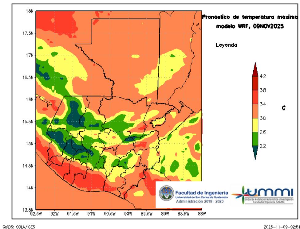
Figura 4: Pronóstico de temperatura máxima diaria del 09 de November
