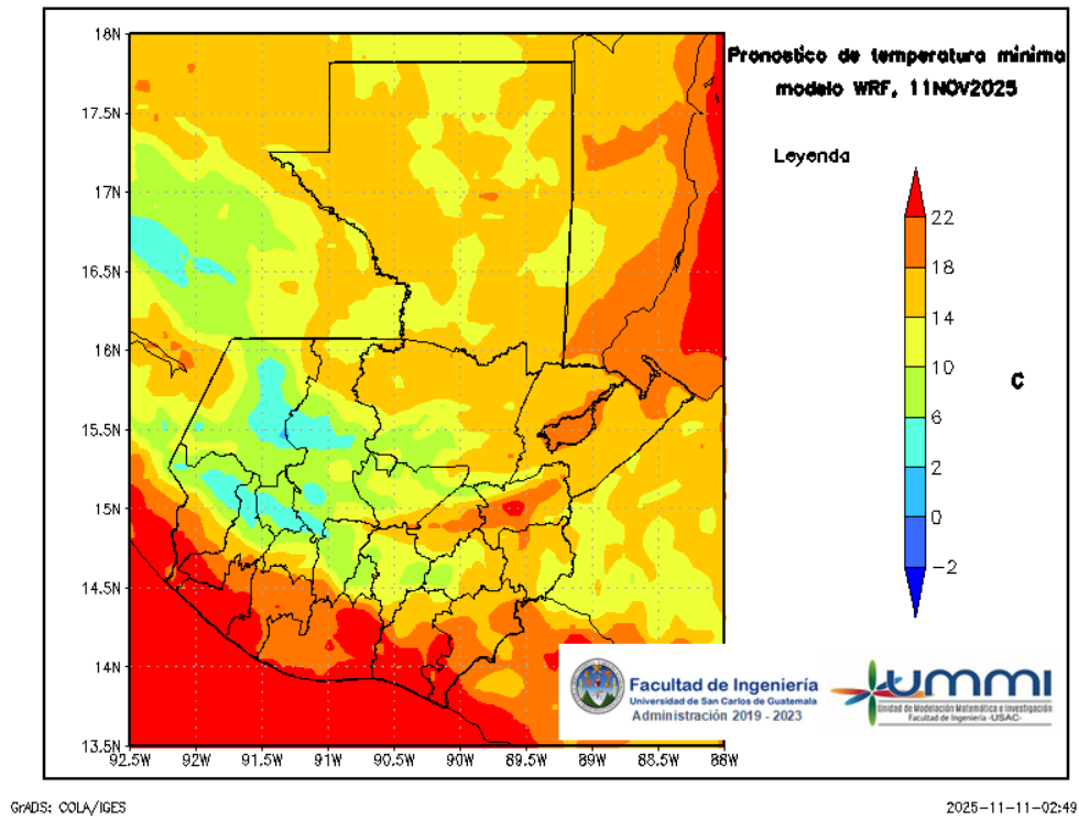
Figura 7: Pronóstico de temperatura mínima diaria del 12 de November
