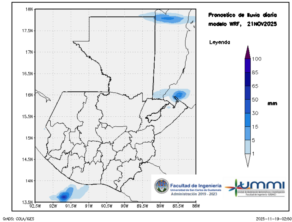
Figura 3: Pronóstico de lluvia diaria del 21 de November
