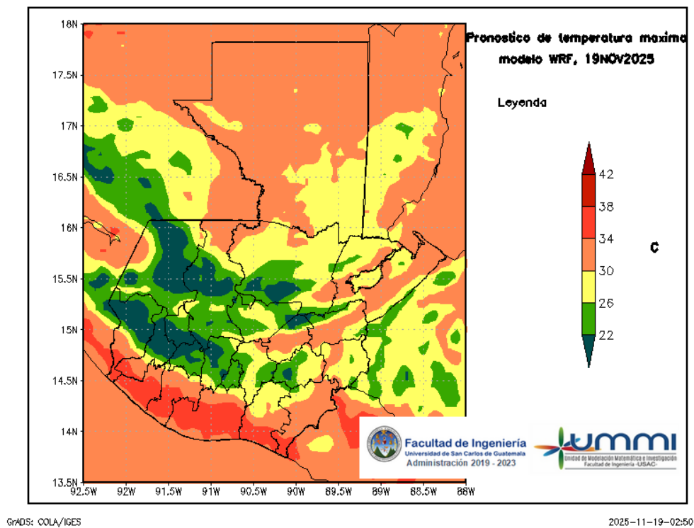
Figura 4: Pronóstico de temperatura máxima diaria del 19 de November
