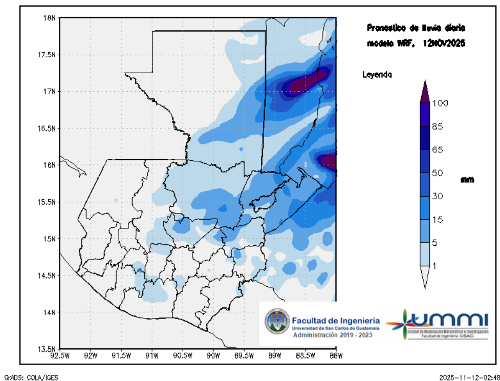
Figura 1: Pronóstico de lluvia diaria del 12 de November
