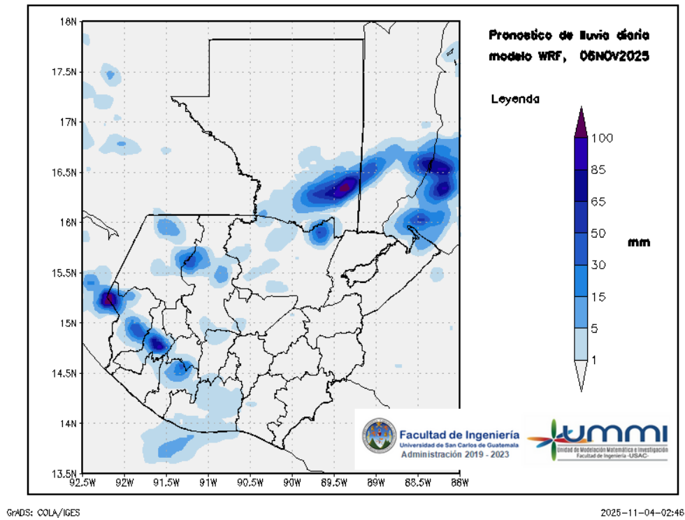
Figura 3: Pronóstico de lluvia diaria del 06 de November
