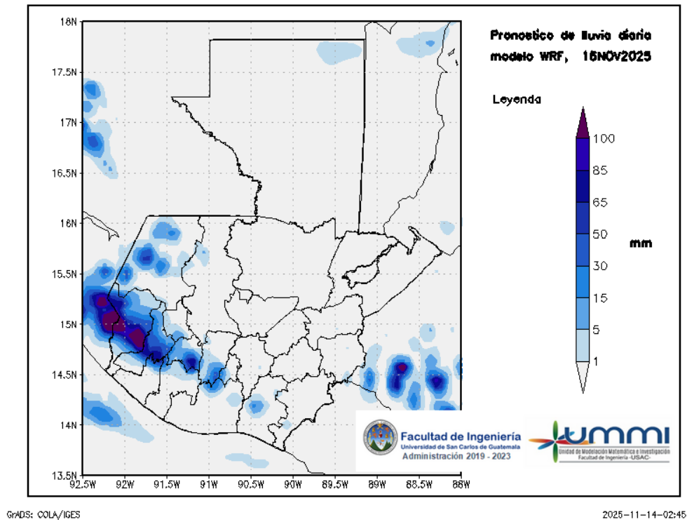
Figura 3: Pronóstico de lluvia diaria del 16 de November
