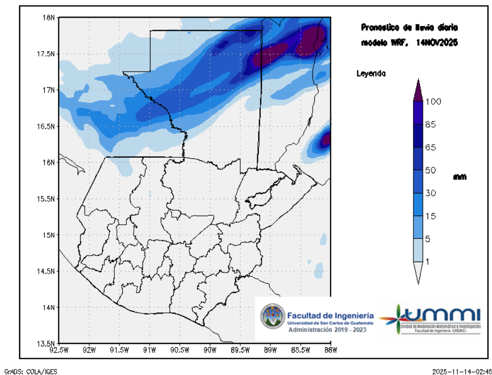
Figura 1: Pronóstico de lluvia diaria del 14 de November
