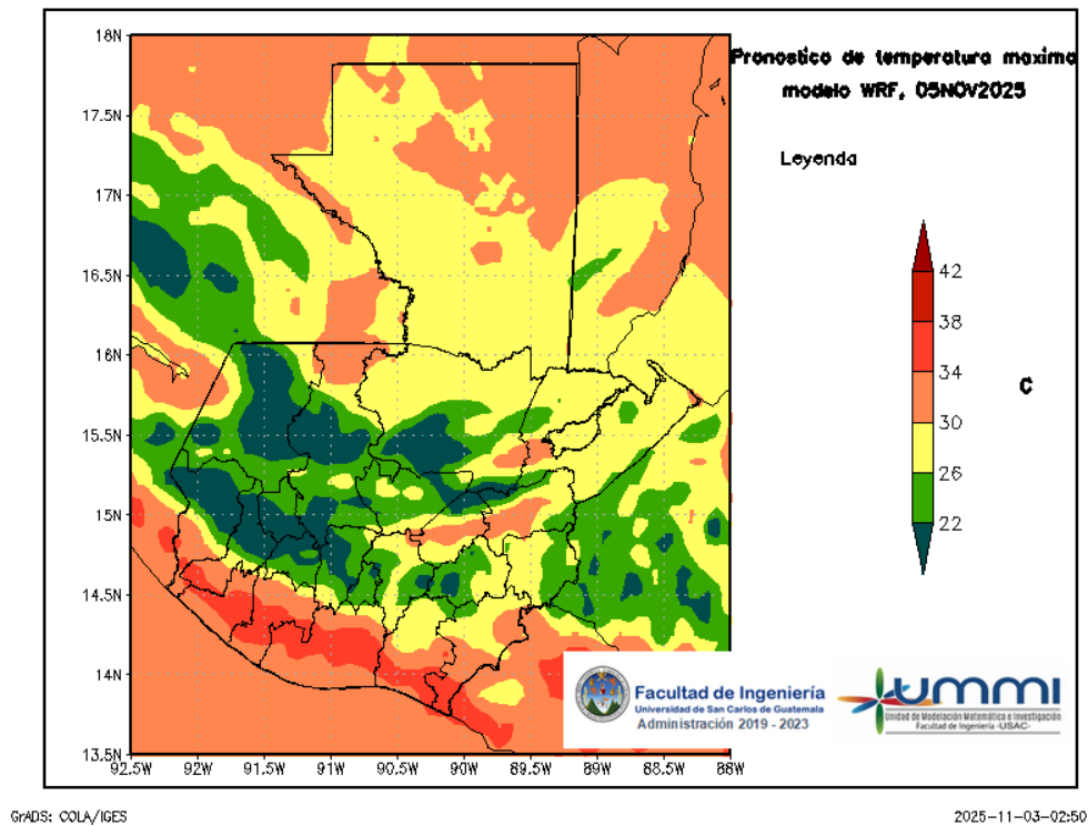
Figura 6: Pronóstico de temperatura máxima diaria del 05 de November
