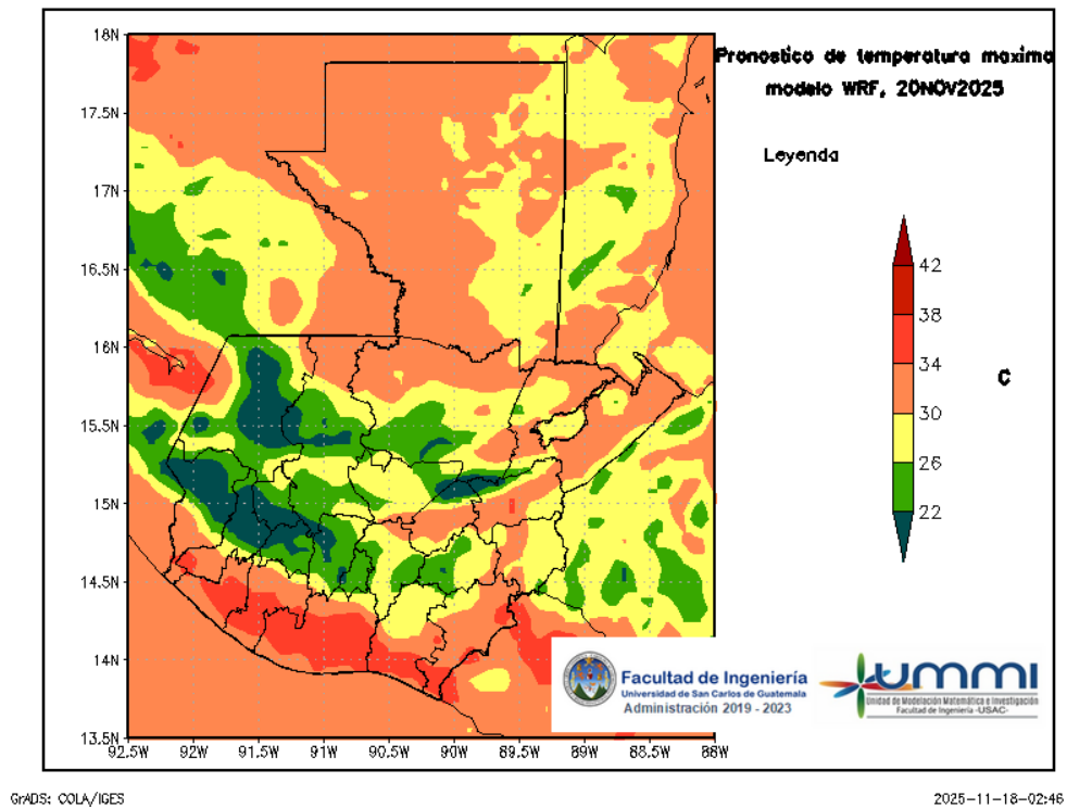
Figura 6: Pronóstico de temperatura máxima diaria del 20 de November
