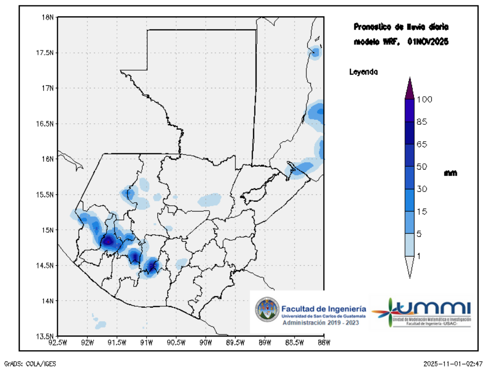
Figura 1: Pronóstico de lluvia diaria del 01 de November
