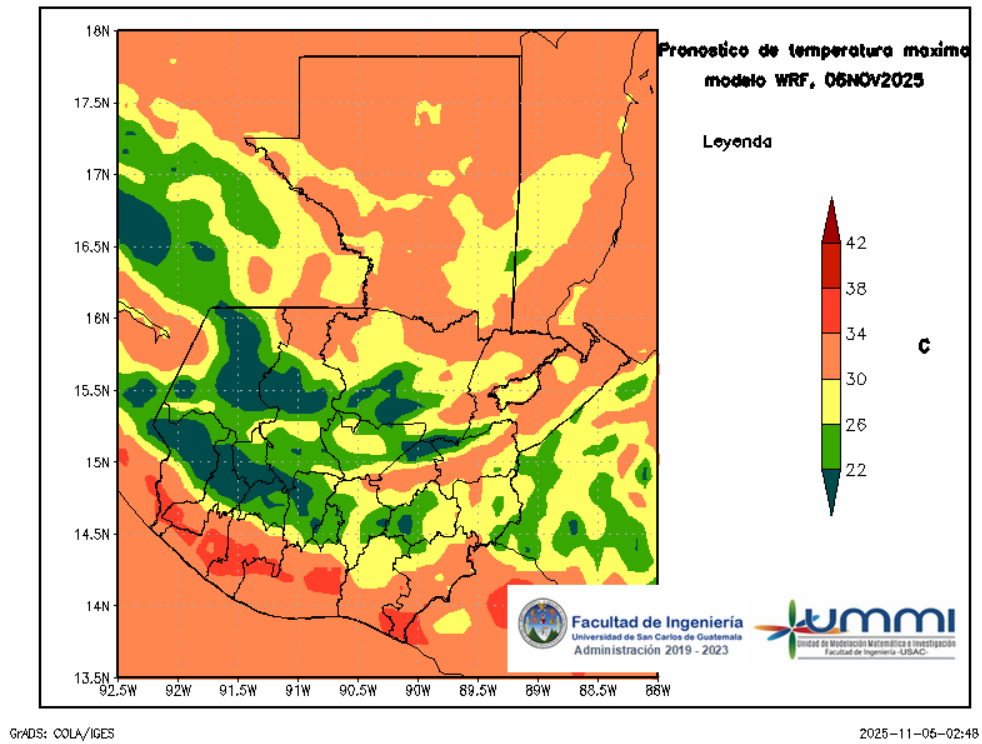
Figura 5: Pronóstico de temperatura máxima diaria del 06 de November
