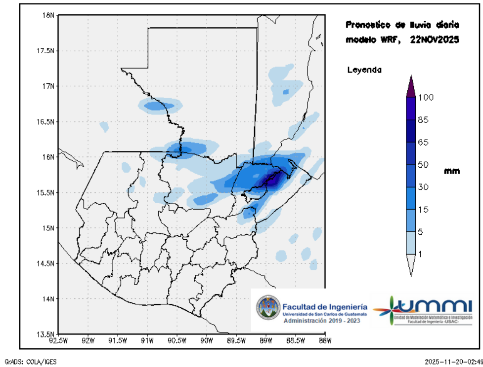
Figura 3: Pronóstico de lluvia diaria del 22 de November
