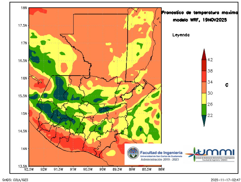
Figura 6: Pronóstico de temperatura máxima diaria del 19 de November
