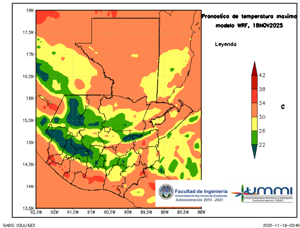
Figura 4: Pronóstico de temperatura máxima diaria del 18 de November
