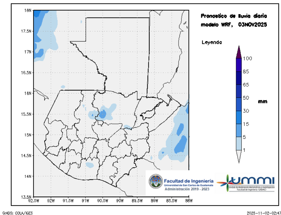
Figura 2: Pronóstico de lluvia diaria del 03 de November
