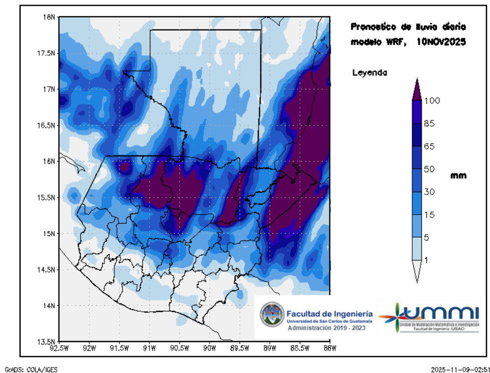
Figura 2: Pronóstico de lluvia diaria del 10 de November
