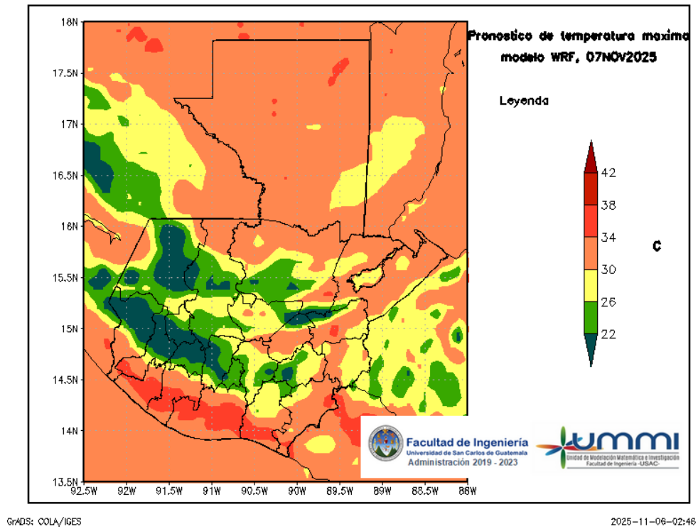
Figura 5: Pronóstico de temperatura máxima diaria del 07 de November
