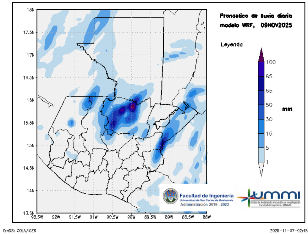
Figura 3: Pronóstico de lluvia diaria del 09 de November
