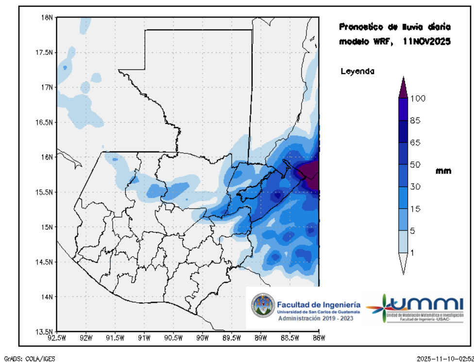
Figura 2: Pronóstico de lluvia diaria del 11 de November
