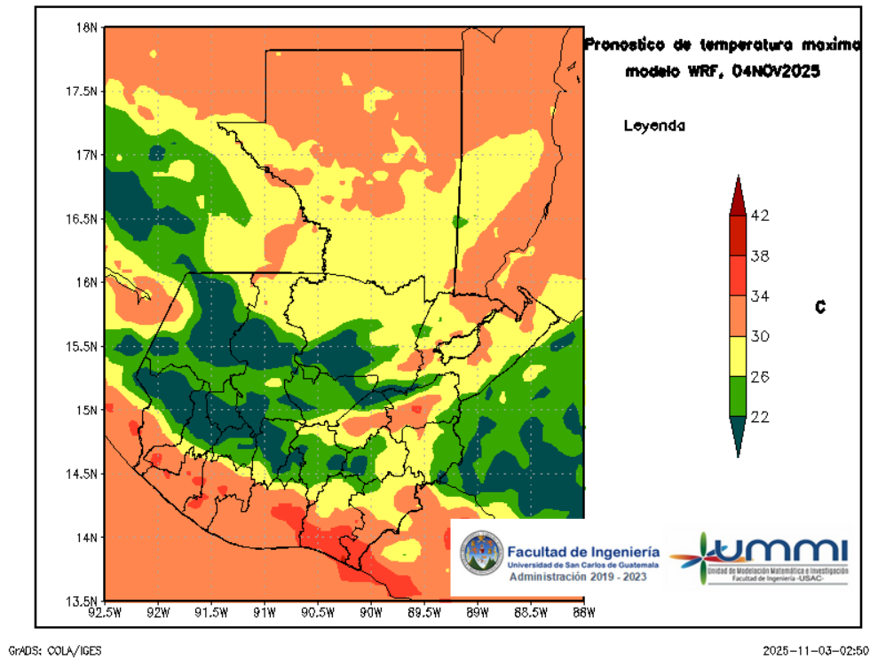
Figura 5: Pronóstico de temperatura máxima diaria del 04 de November
