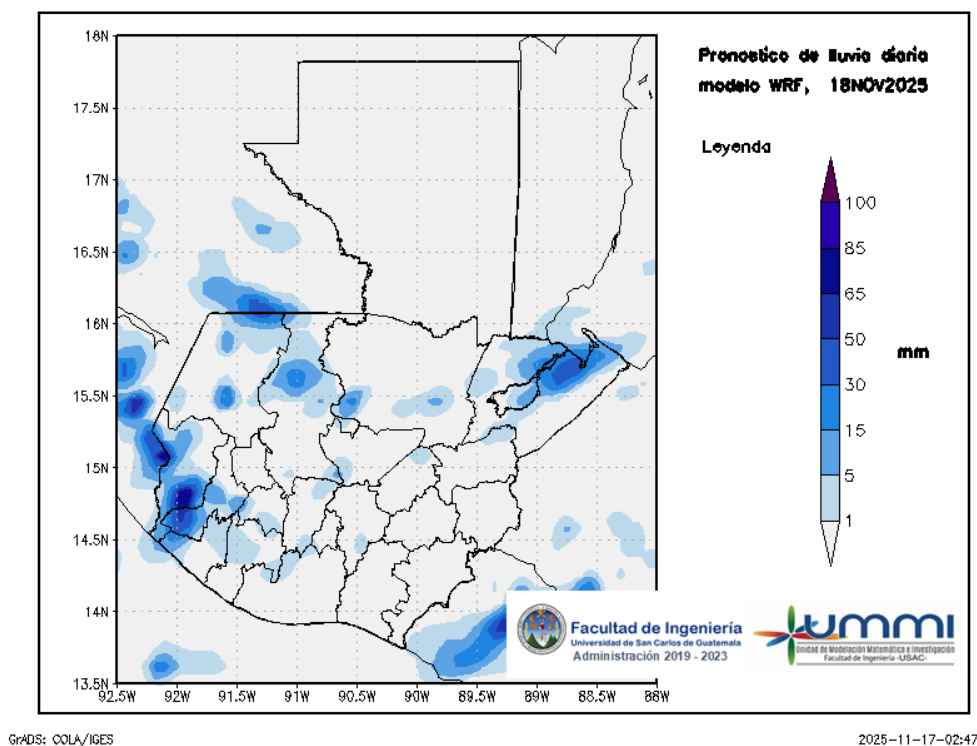
Figura 2: Pronóstico de lluvia diaria del 18 de November
