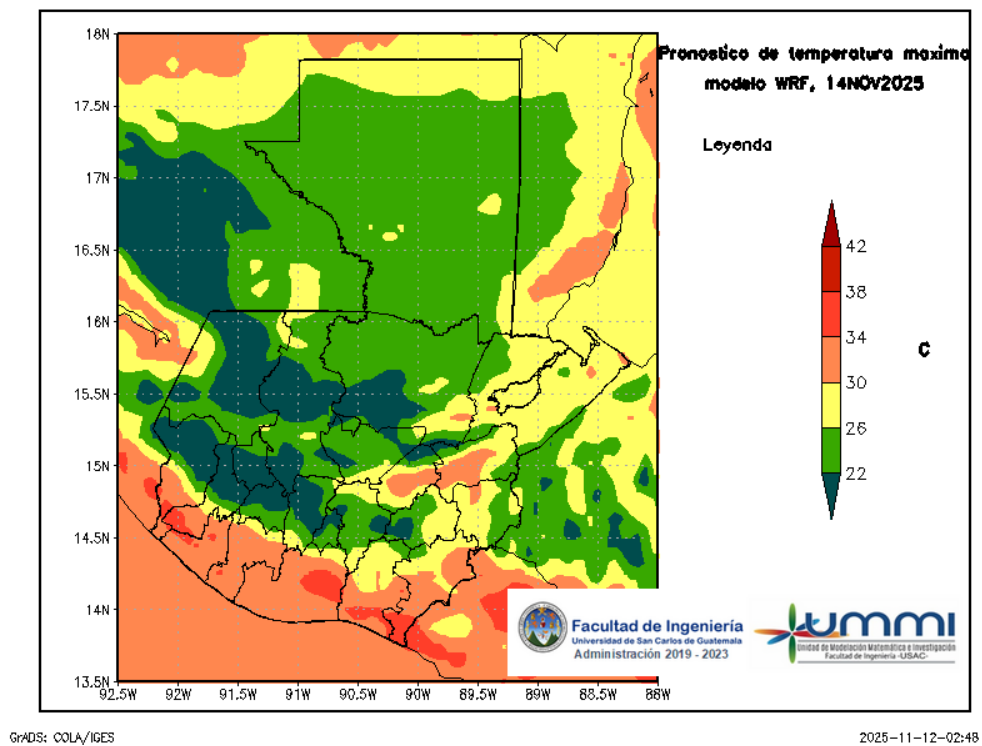
Figura 6: Pronóstico de temperatura máxima diaria del 14 de November
