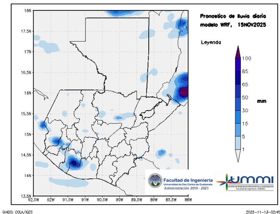
Figura 3: Pronóstico de lluvia diaria del 15 de November
