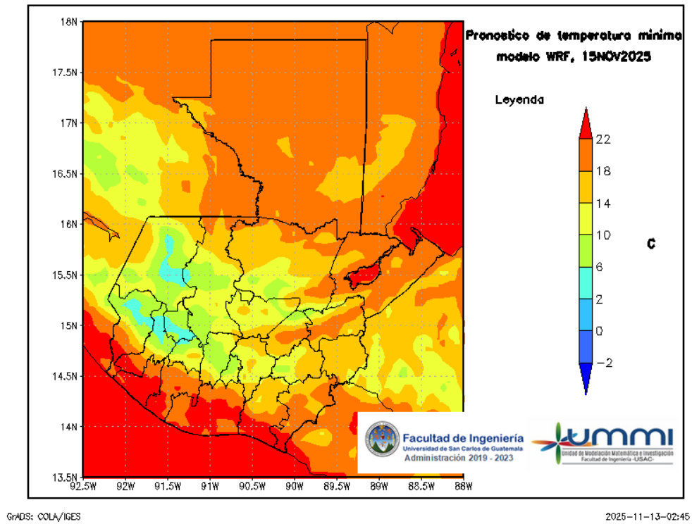
Figura 9: Pronóstico de temperatura mínima diaria del 16 de November
