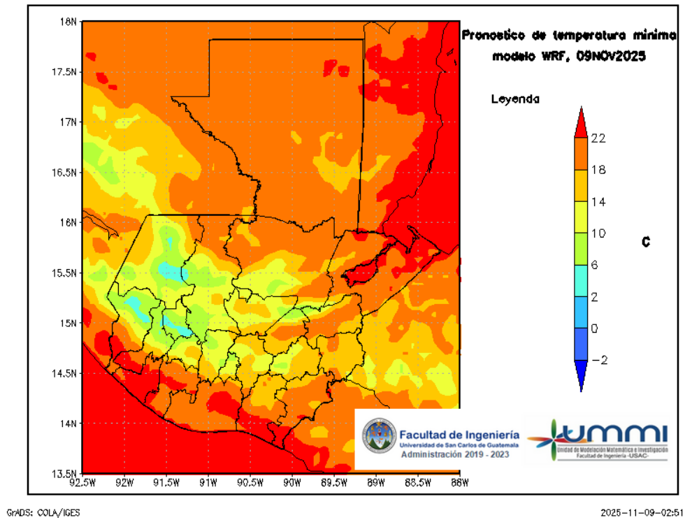
Figura 7: Pronóstico de temperatura mínima diaria del 10 de November
