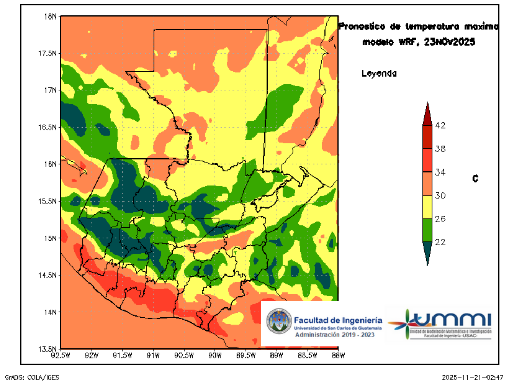
Figura 6: Pronóstico de temperatura máxima diaria del 23 de November
