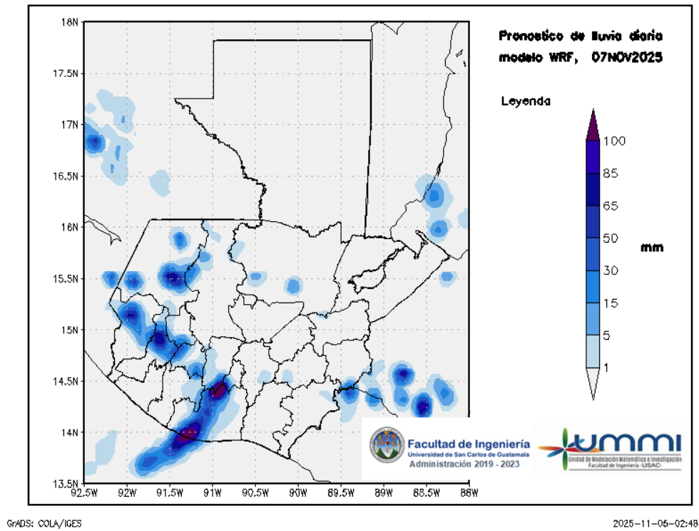
Figura 3: Pronóstico de lluvia diaria del 07 de November
