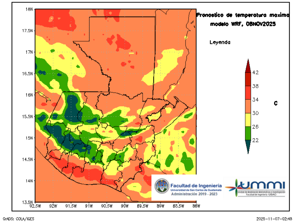
Figura 5: Pronóstico de temperatura máxima diaria del 08 de November
