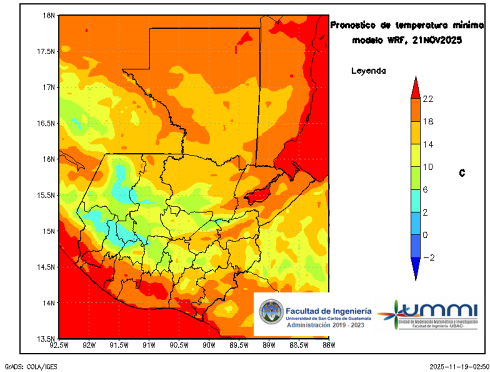
Figura 9: Pronóstico de temperatura mínima diaria del 22 de November
