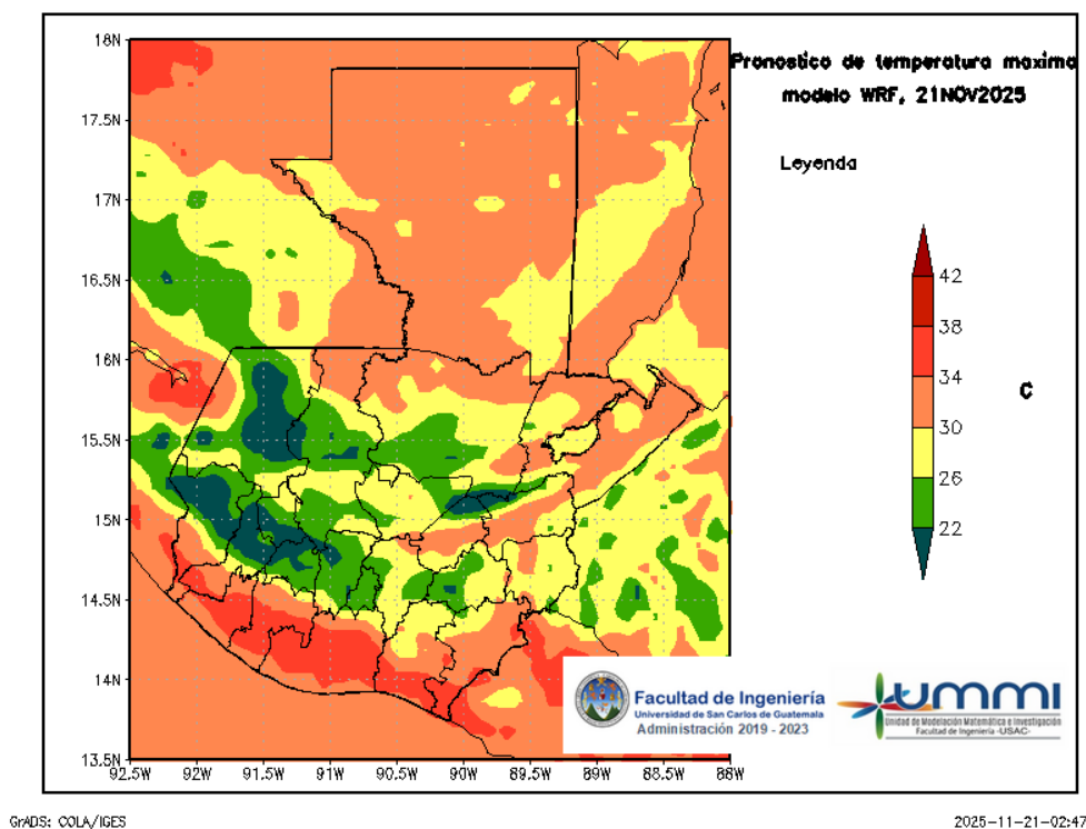
Figura 4: Pronóstico de temperatura máxima diaria del 21 de November
