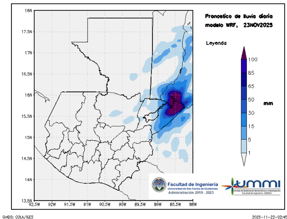
Figura 2: Pronóstico de lluvia diaria del 23 de November
