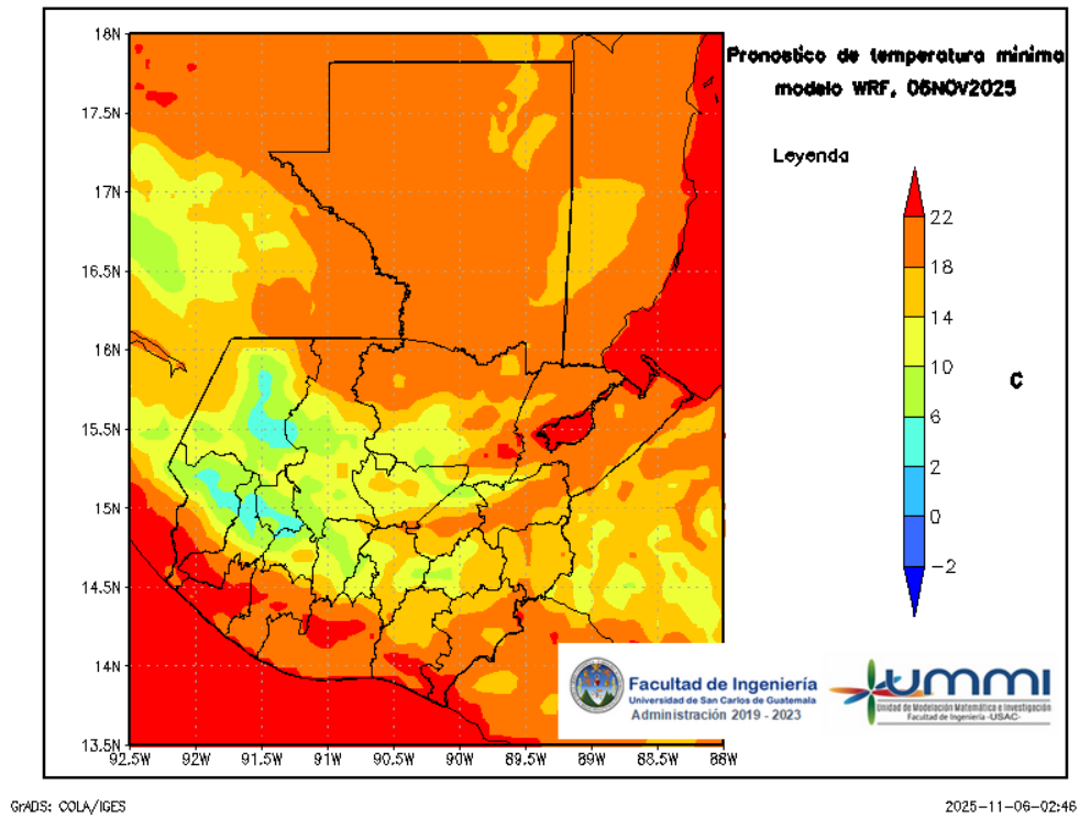
Figura 7: Pronóstico de temperatura mínima diaria del 07 de November
