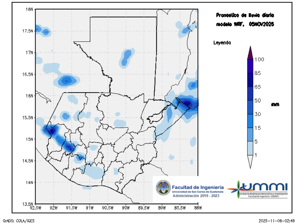
Figura 1: Pronóstico de lluvia diaria del 05 de November
