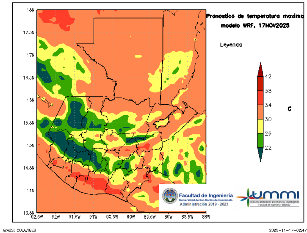
Figura 4: Pronóstico de temperatura máxima diaria del 17 de November
