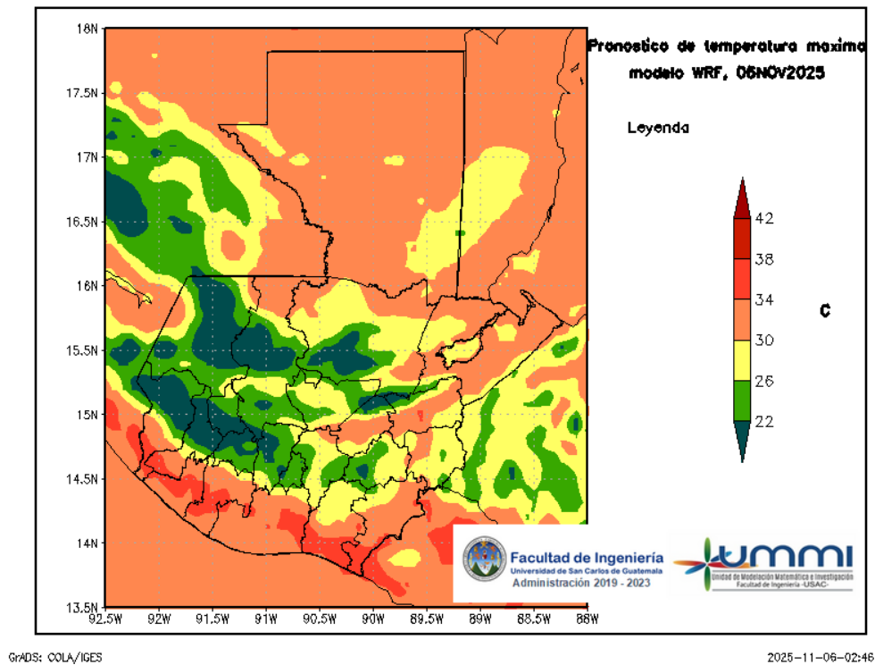
Figura 4: Pronóstico de temperatura máxima diaria del 06 de November
