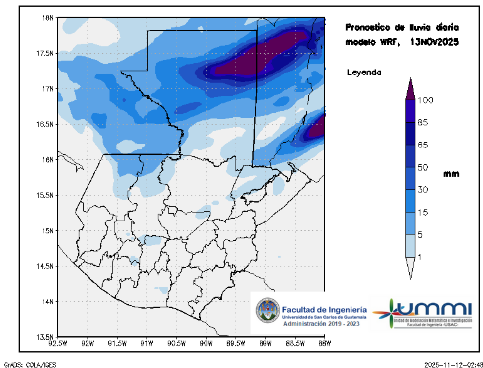
Figura 2: Pronóstico de lluvia diaria del 13 de November
