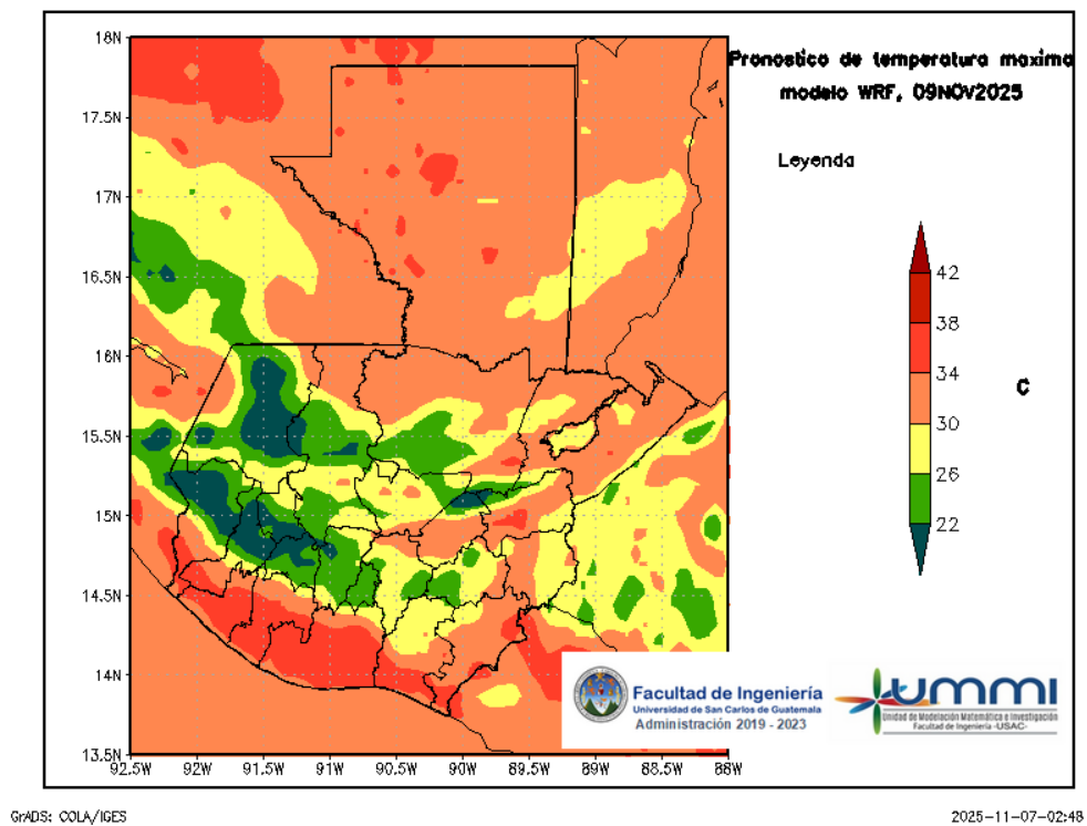
Figura 6: Pronóstico de temperatura máxima diaria del 09 de November
