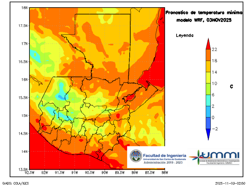
Figura 7: Pronóstico de temperatura mínima diaria del 04 de November
