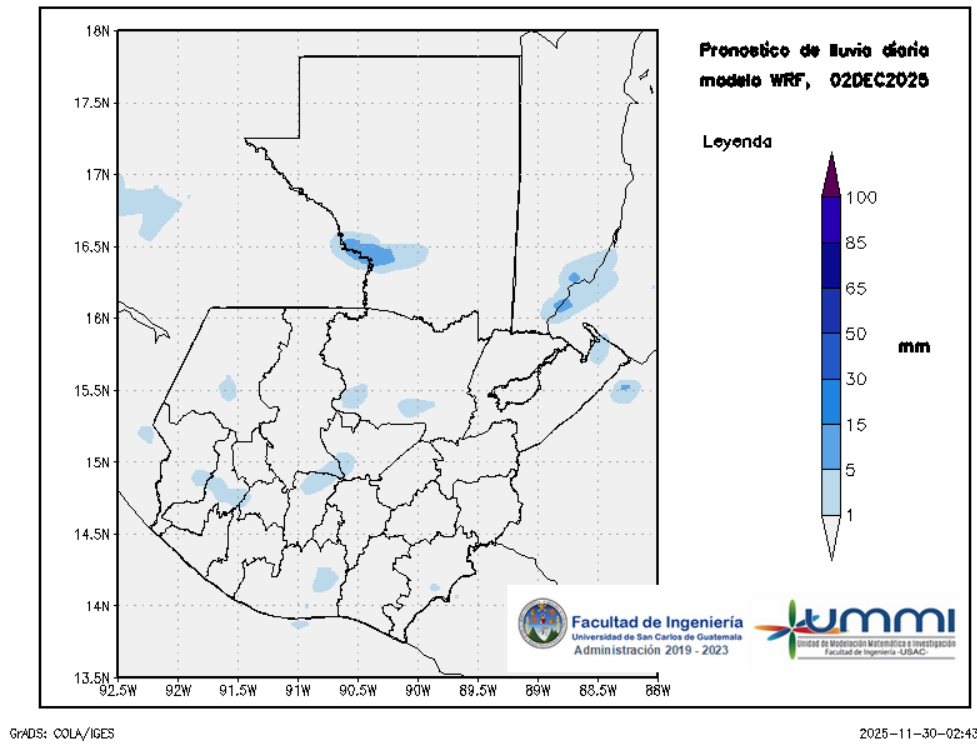
Figura 3: Pronóstico de lluvia diaria del 02 de December
