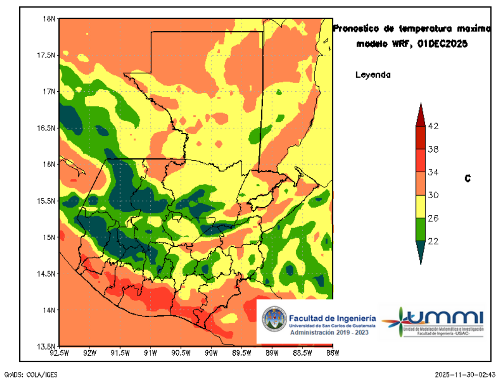
Figura 5: Pronóstico de temperatura máxima diaria del 01 de December
