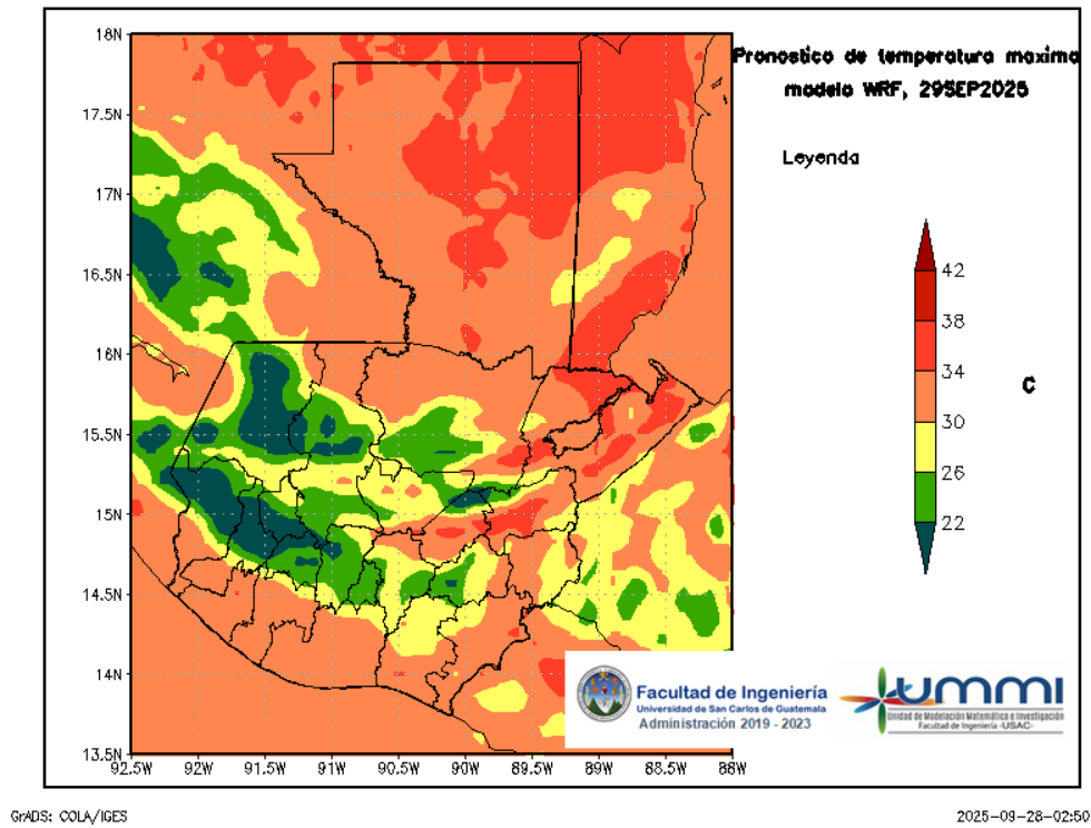
Figura 5: Pronóstico de temperatura máxima diaria del 29 de September
