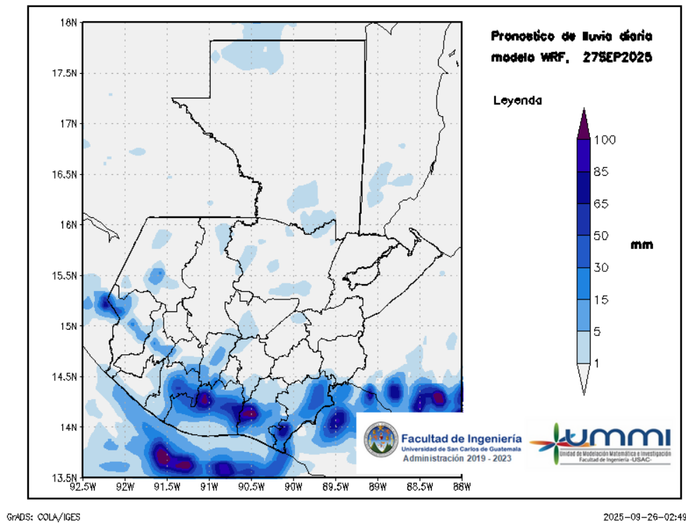
Figura 2: Pronóstico de lluvia diaria del 27 de September
