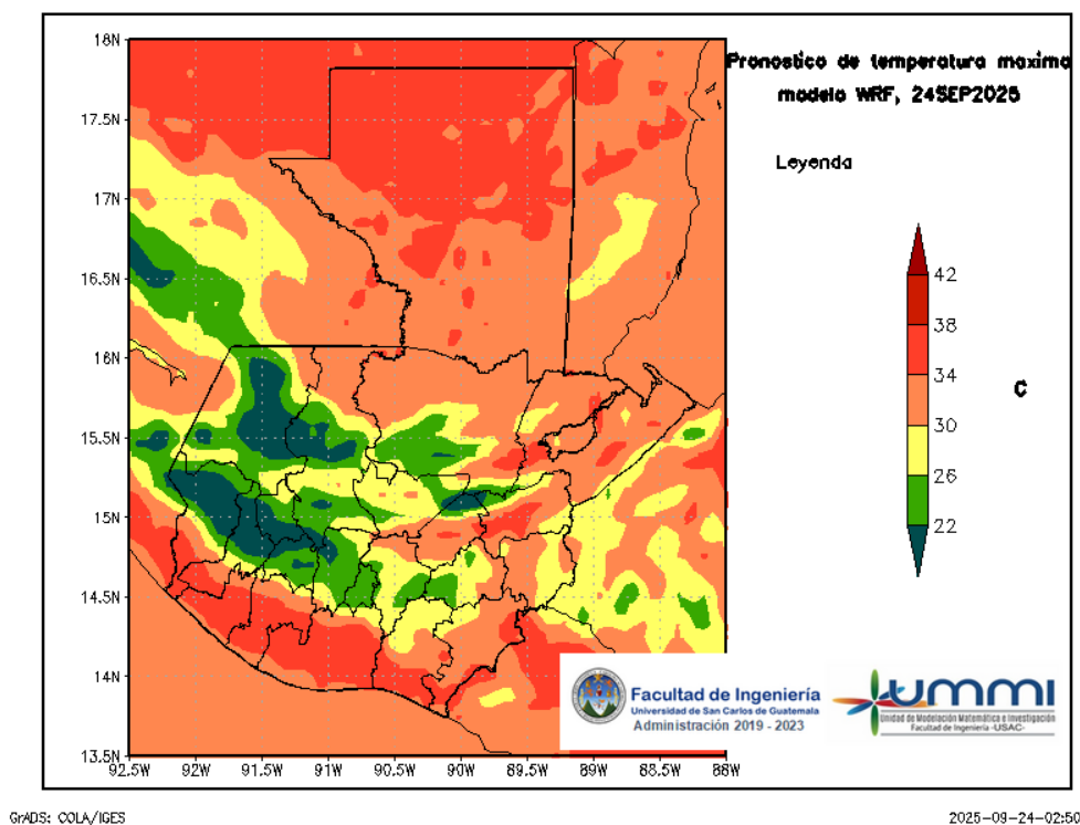
Figura 4: Pronóstico de temperatura máxima diaria del 24 de September
