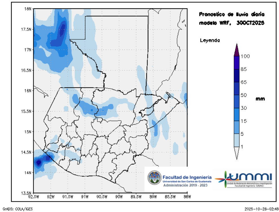
Figura 3: Pronóstico de lluvia diaria del 30 de October
