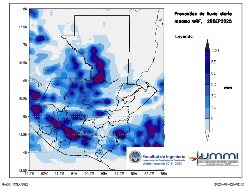
Figura 2: Pronóstico de lluvia diaria del 29 de September
