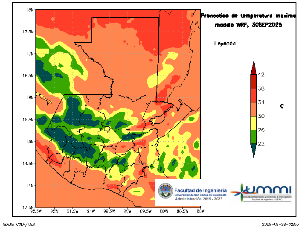
Figura 6: Pronóstico de temperatura máxima diaria del 30 de September
