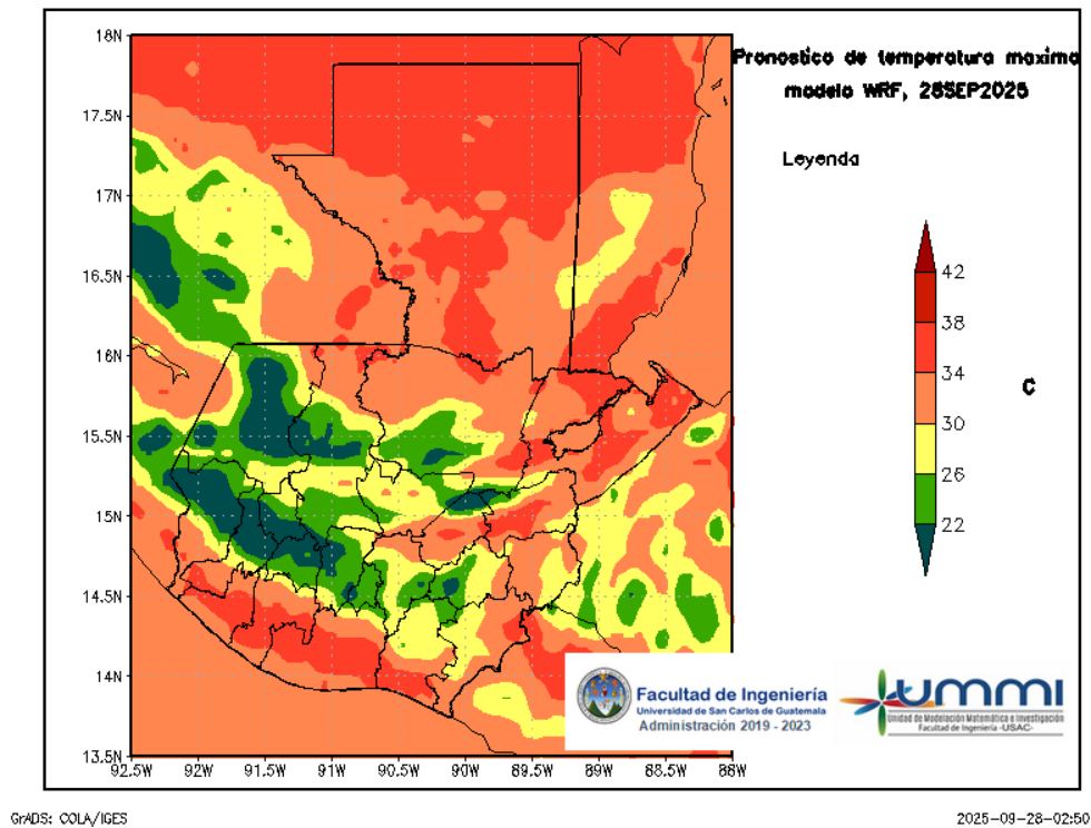
Figura 4: Pronóstico de temperatura máxima diaria del 28 de September
