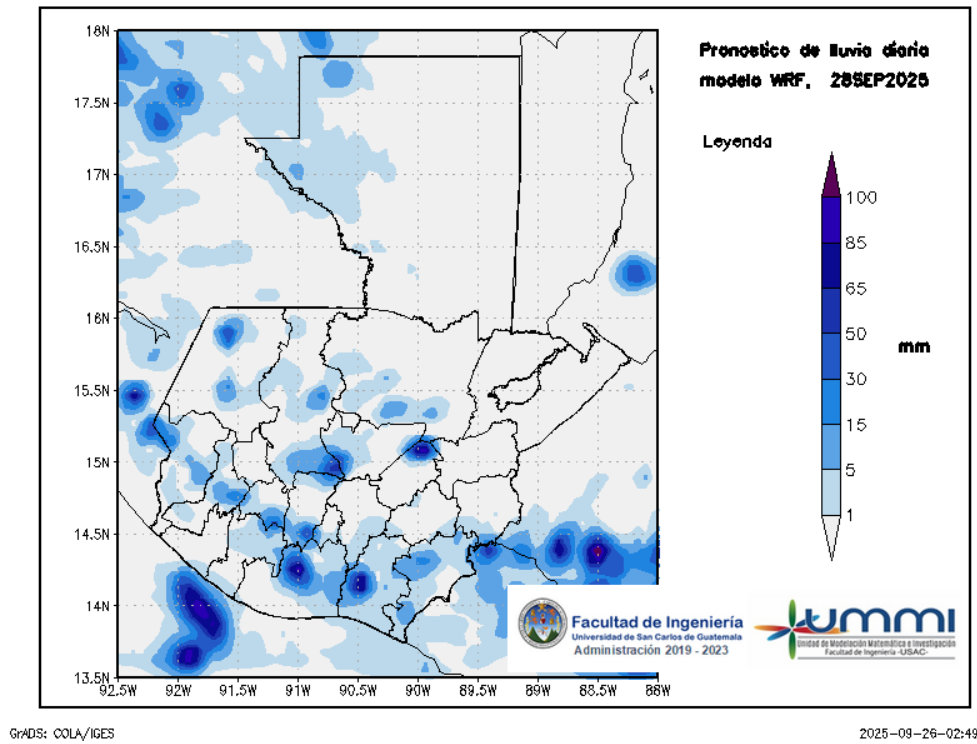
Figura 3: Pronóstico de lluvia diaria del 28 de September
