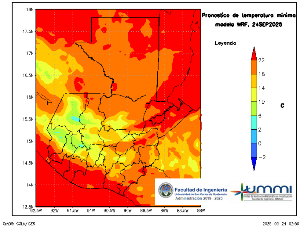
Figura 7: Pronóstico de temperatura mínima diaria del 25 de September
