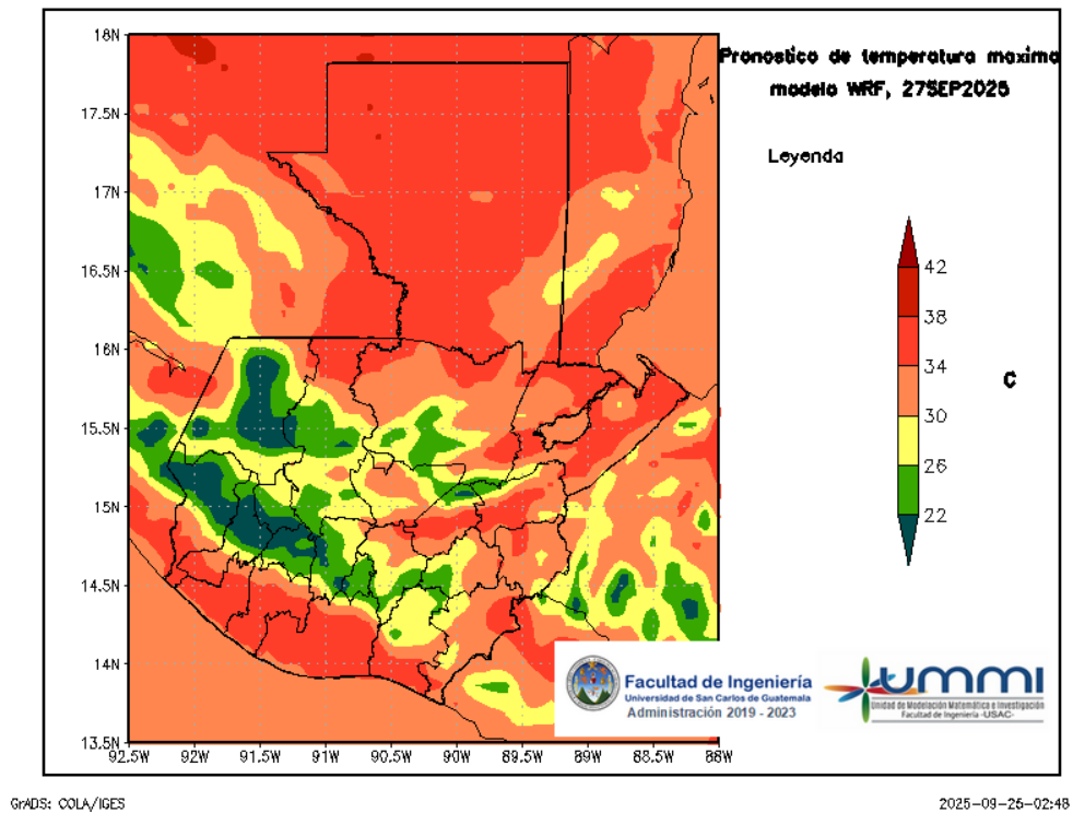
Figura 6: Pronóstico de temperatura máxima diaria del 27 de September
