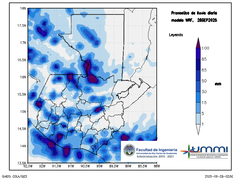
Figura 1: Pronóstico de lluvia diaria del 28 de September
