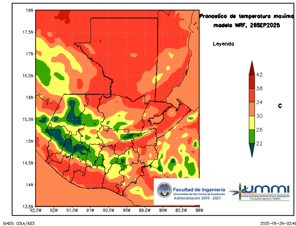
Figura 4: Pronóstico de temperatura máxima diaria del 26 de September
