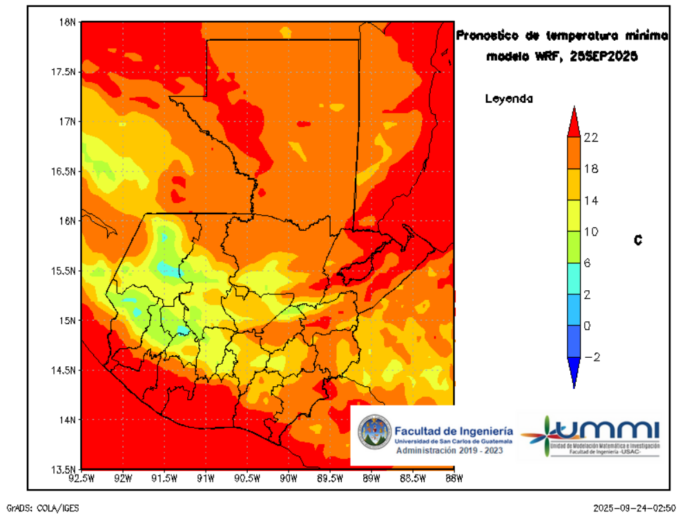
Figura 8: Pronóstico de temperatura mínima diaria del 26 de September
