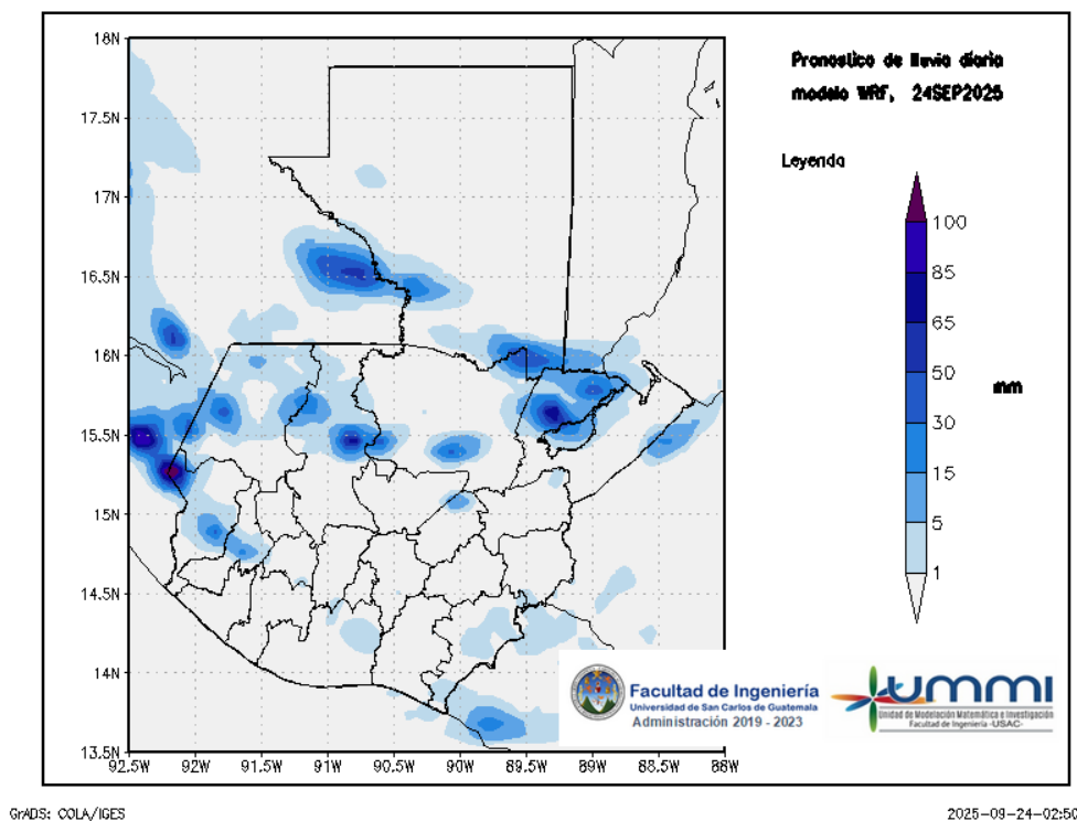
Figura 1: Pronóstico de lluvia diaria del 24 de September
