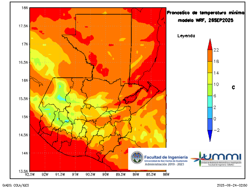
Figura 9: Pronóstico de temperatura mínima diaria del 27 de September
