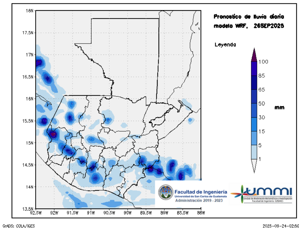
Figura 3: Pronóstico de lluvia diaria del 26 de September
