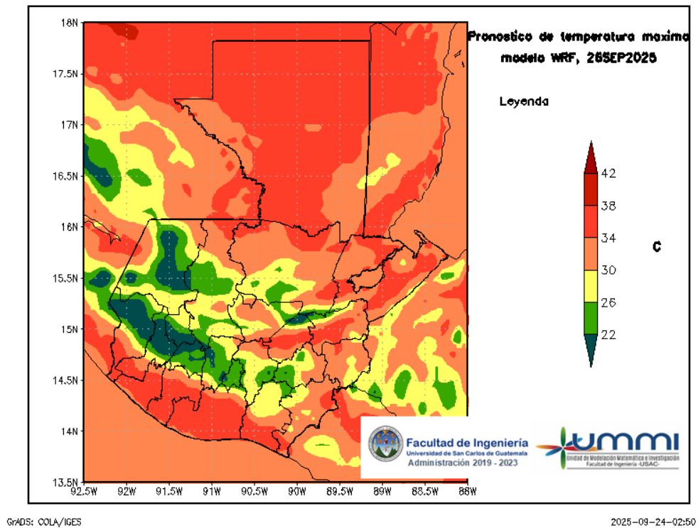
Figura 6: Pronóstico de temperatura máxima diaria del 26 de September
