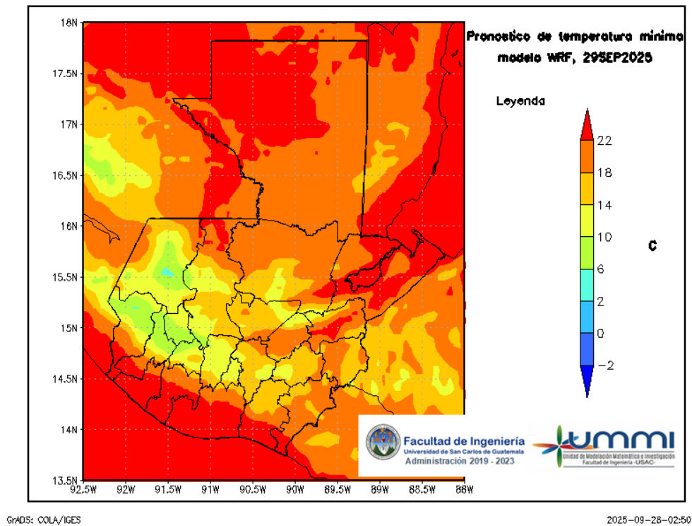
Figura 8: Pronóstico de temperatura mínima diaria del 30 de September
