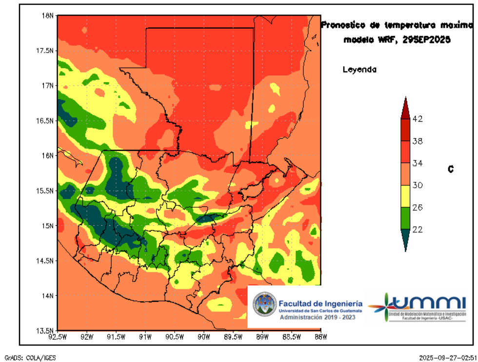
Figura 6: Pronóstico de temperatura máxima diaria del 29 de September
