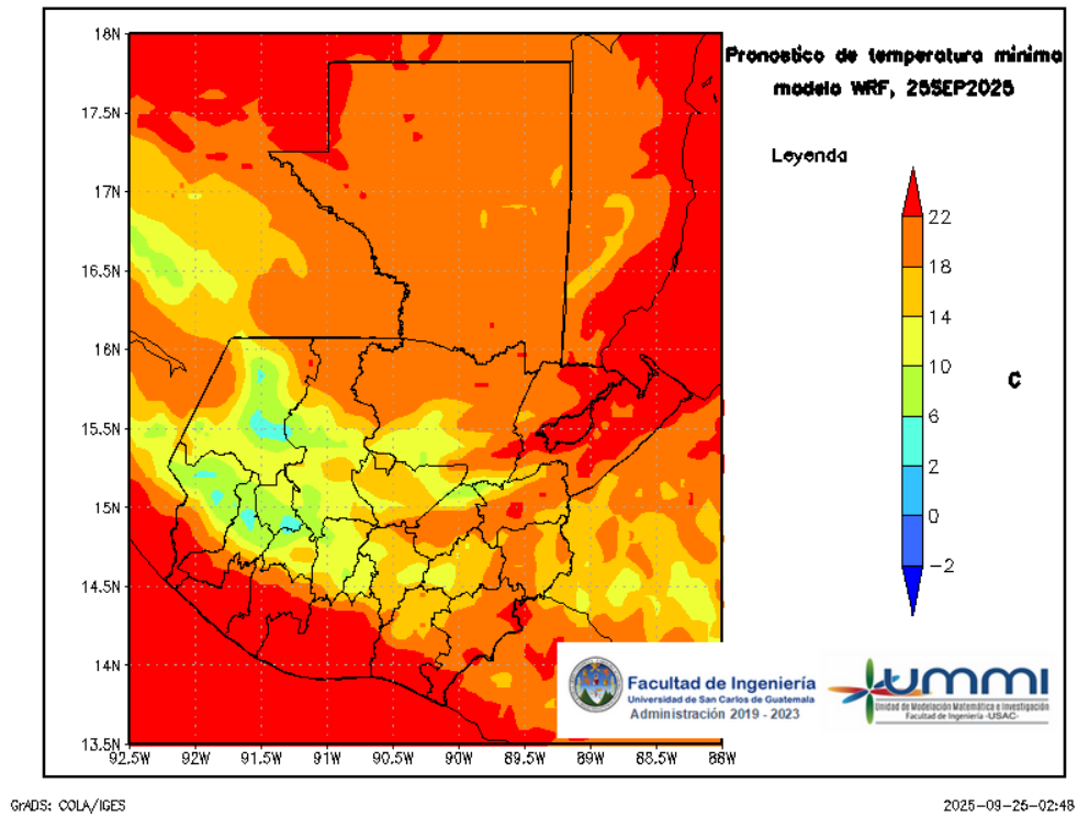
Figura 7: Pronóstico de temperatura mínima diaria del 26 de September
