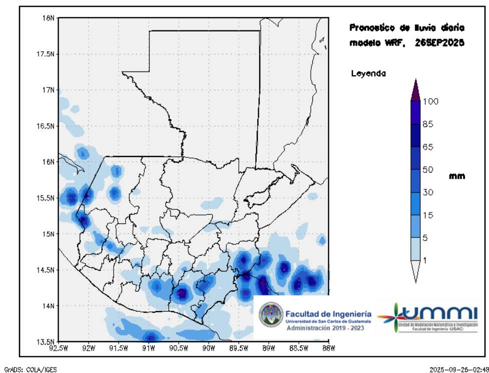
Figura 2: Pronóstico de lluvia diaria del 26 de September
