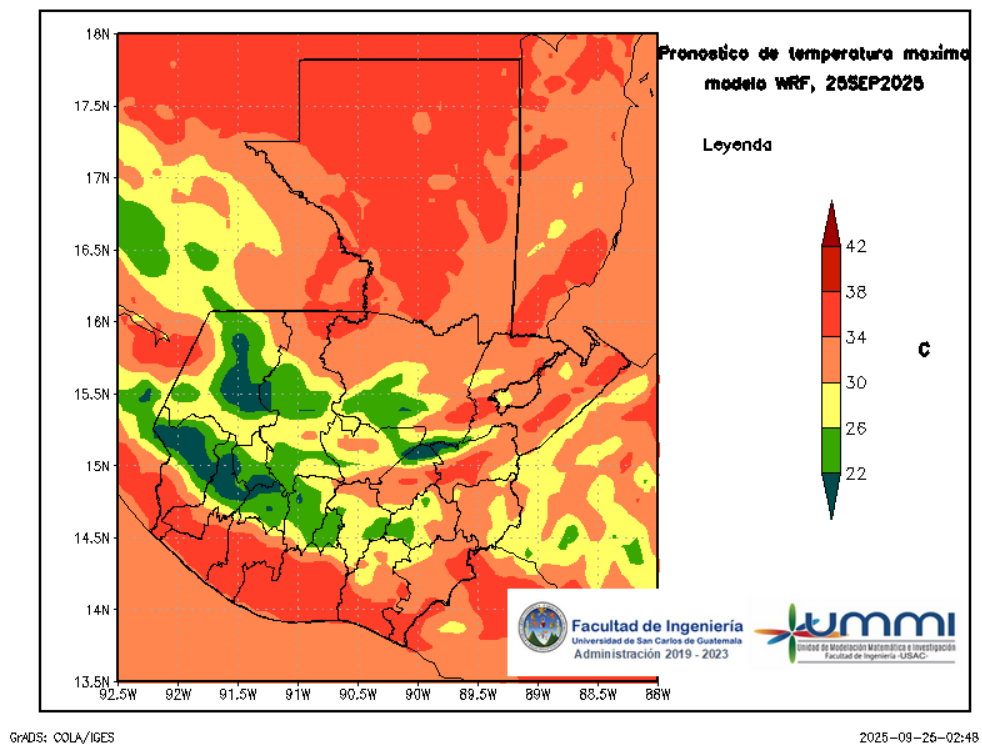
Figura 4: Pronóstico de temperatura máxima diaria del 25 de September
