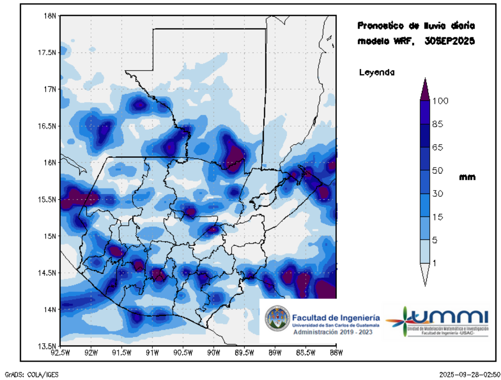
Figura 3: Pronóstico de lluvia diaria del 30 de September
