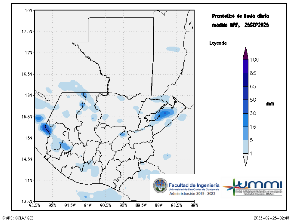
Figura 1: Pronóstico de lluvia diaria del 25 de September
