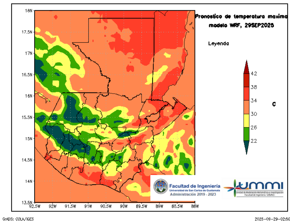
Figura 4: Pronóstico de temperatura máxima diaria del 29 de September
