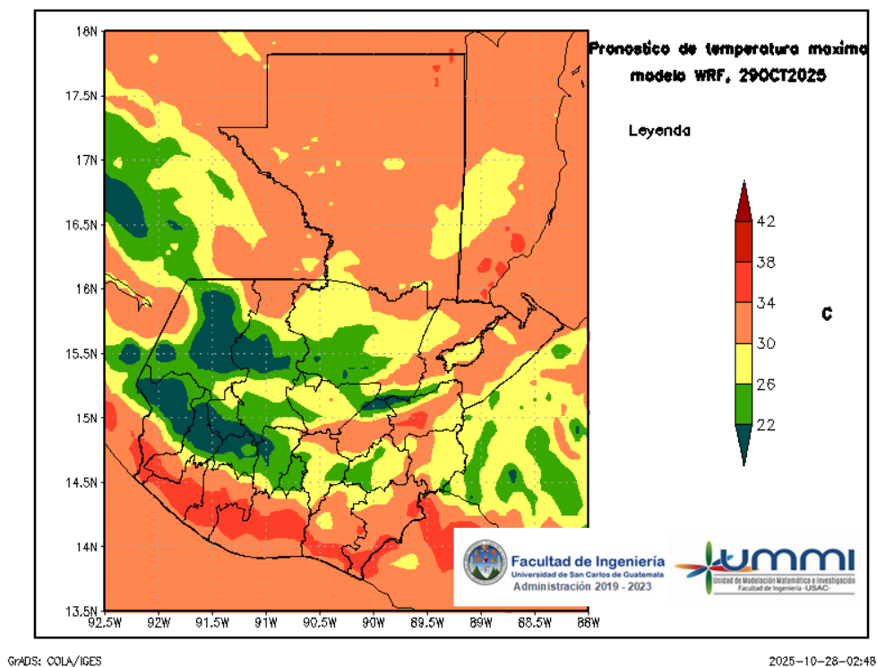
Figura 5: Pronóstico de temperatura máxima diaria del 29 de October
