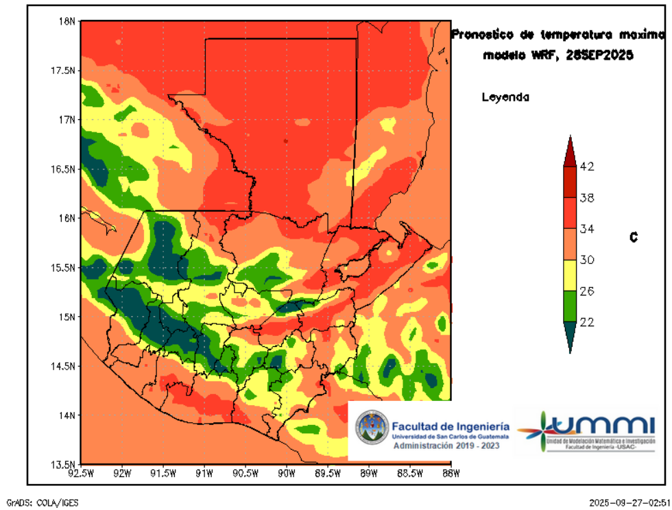
Figura 5: Pronóstico de temperatura máxima diaria del 28 de September
