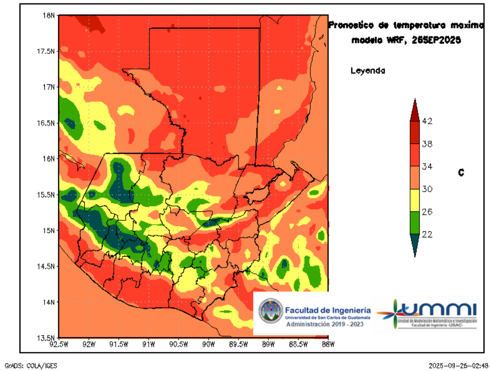
Figura 5: Pronóstico de temperatura máxima diaria del 26 de September
