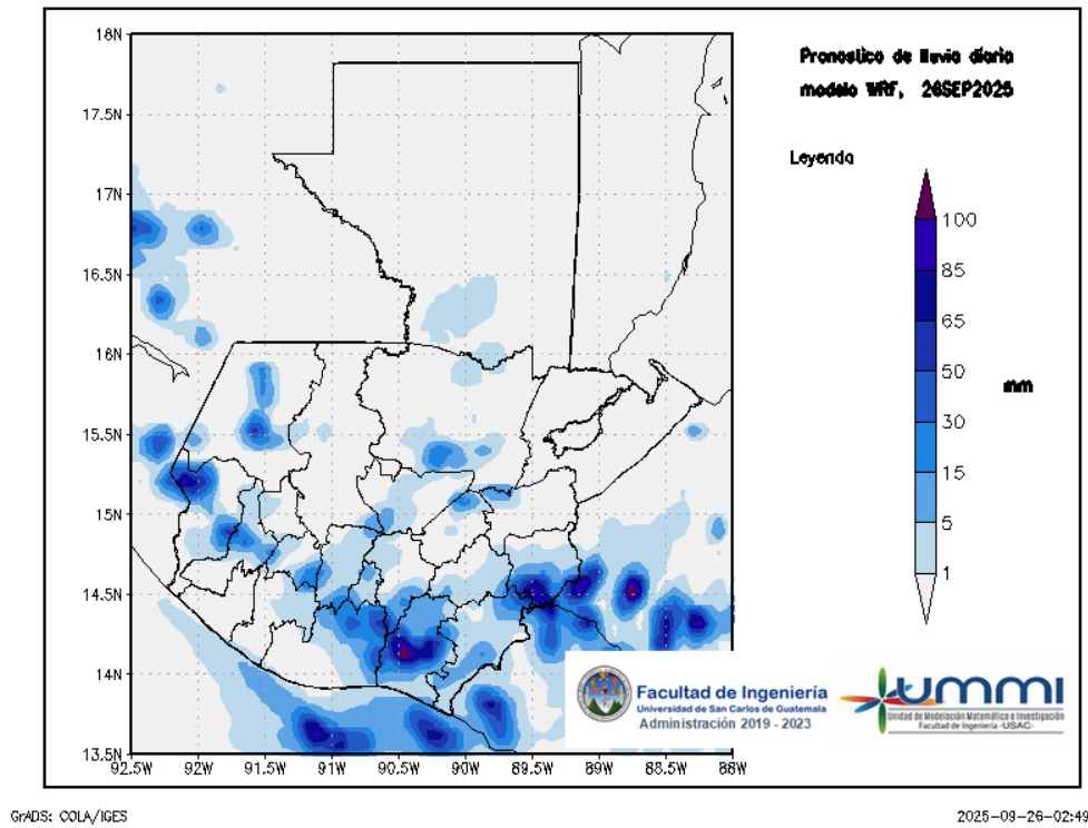
Figura 1: Pronóstico de lluvia diaria del 26 de September
