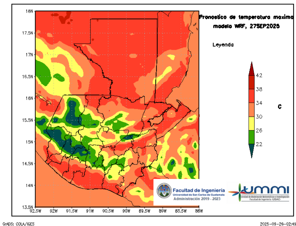
Figura 5: Pronóstico de temperatura máxima diaria del 27 de September
