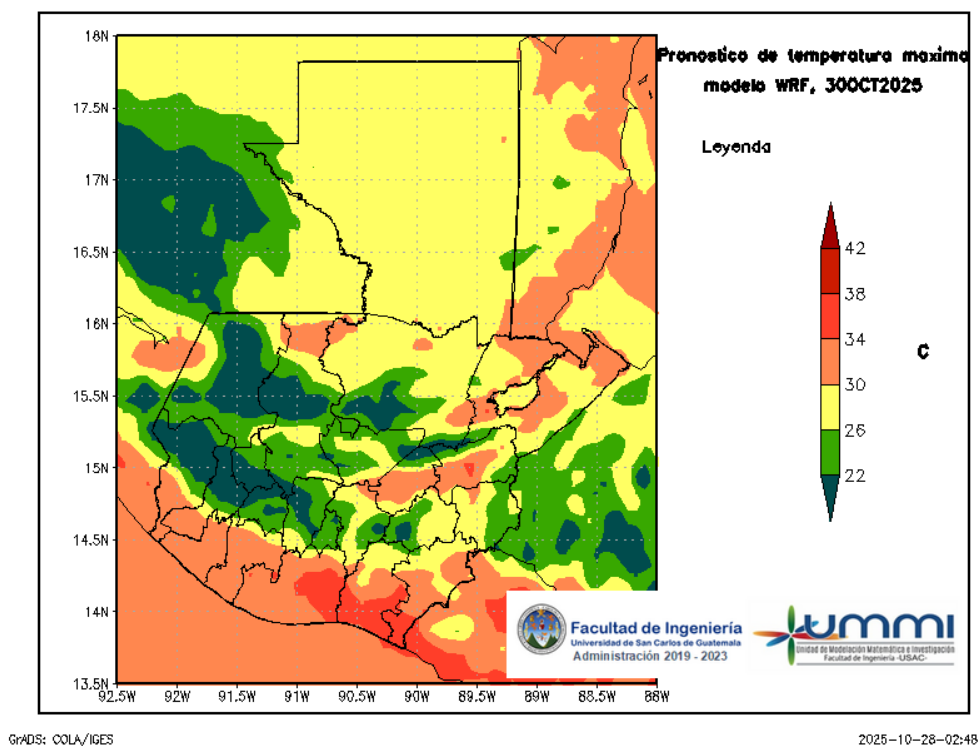
Figura 6: Pronóstico de temperatura máxima diaria del 30 de October
