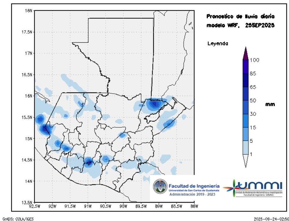
Figura 2: Pronóstico de lluvia diaria del 25 de September
