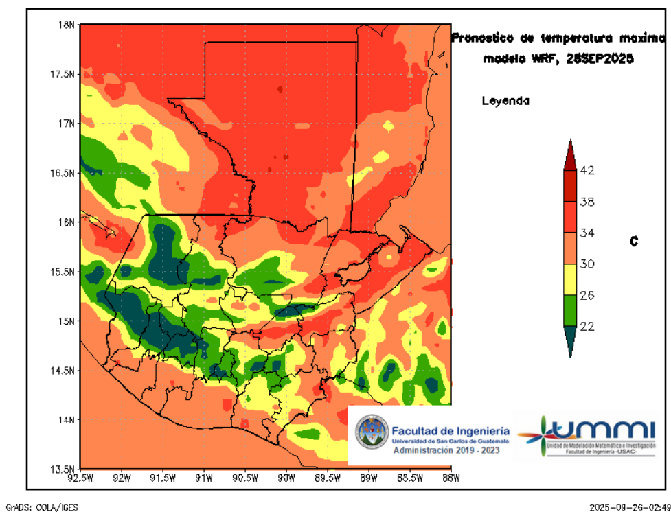
Figura 6: Pronóstico de temperatura máxima diaria del 28 de September
