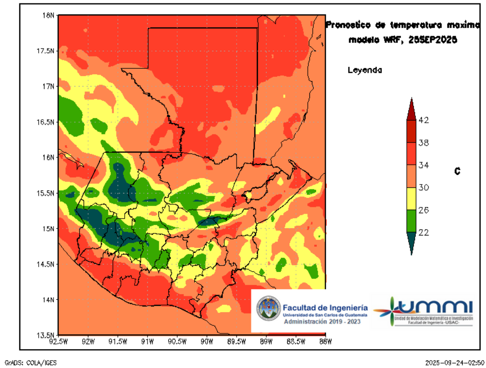
Figura 5: Pronóstico de temperatura máxima diaria del 25 de September
