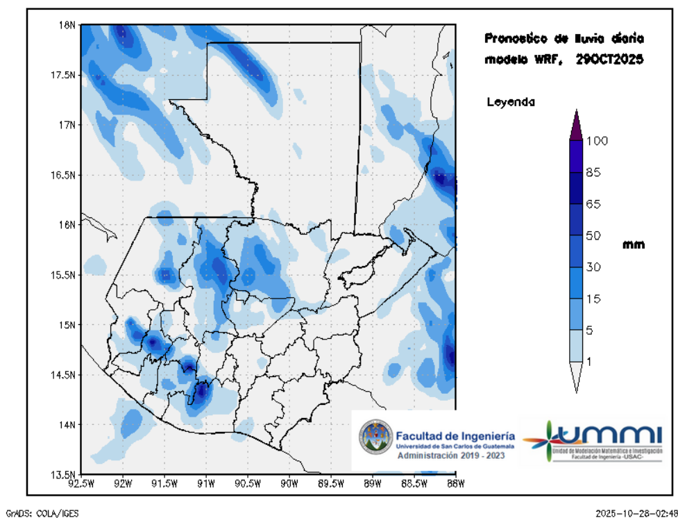
Figura 2: Pronóstico de lluvia diaria del 29 de October
