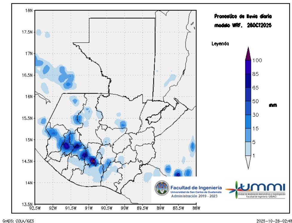
Figura 1: Pronóstico de lluvia diaria del 28 de October
