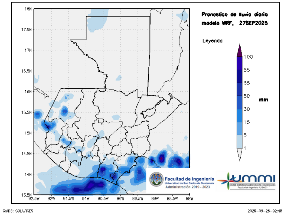
Figura 3: Pronóstico de lluvia diaria del 27 de September
