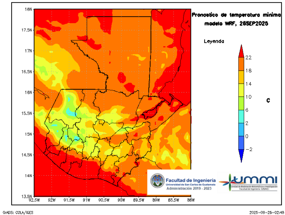
Figura 8: Pronóstico de temperatura mínima diaria del 27 de September
