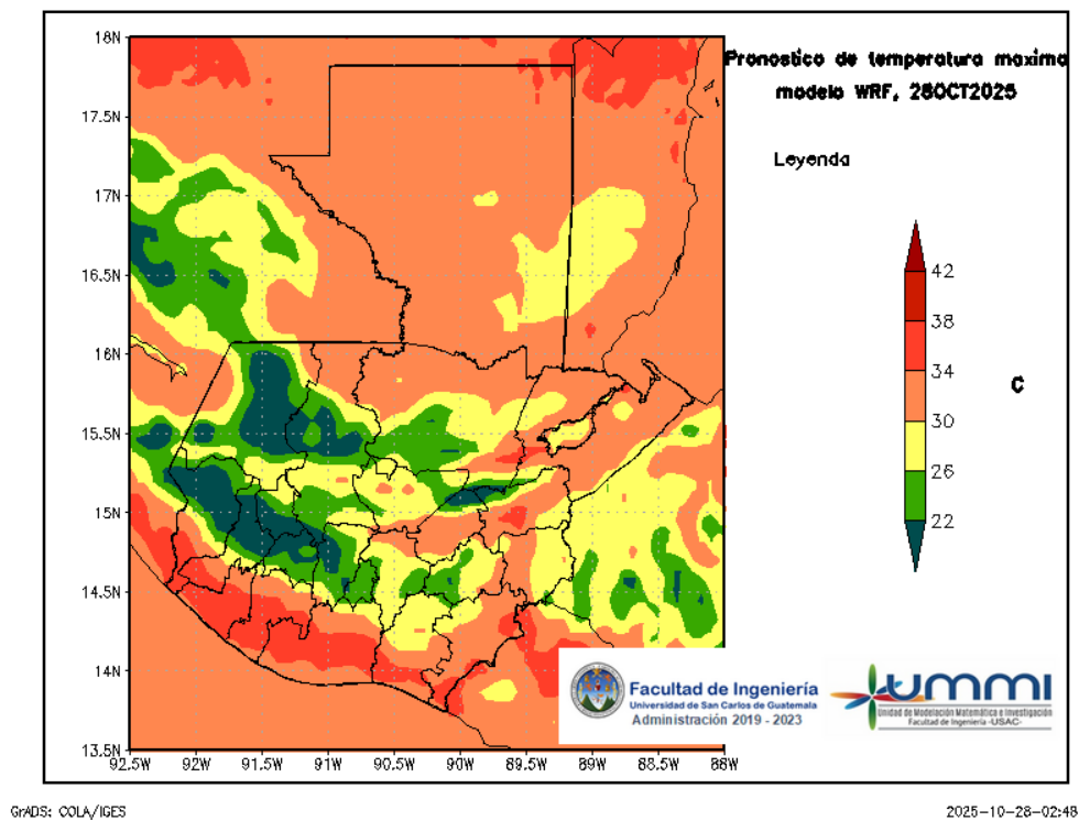
Figura 4: Pronóstico de temperatura máxima diaria del 28 de October
