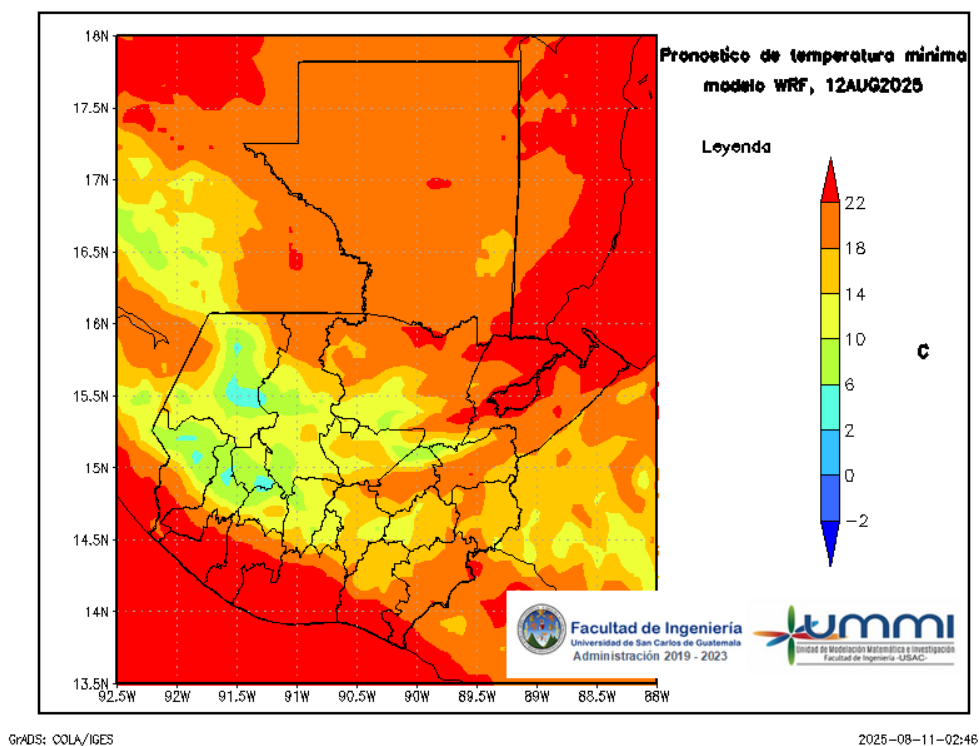
Figura 8: Pronóstico de temperatura mínima diaria del 13 de August
