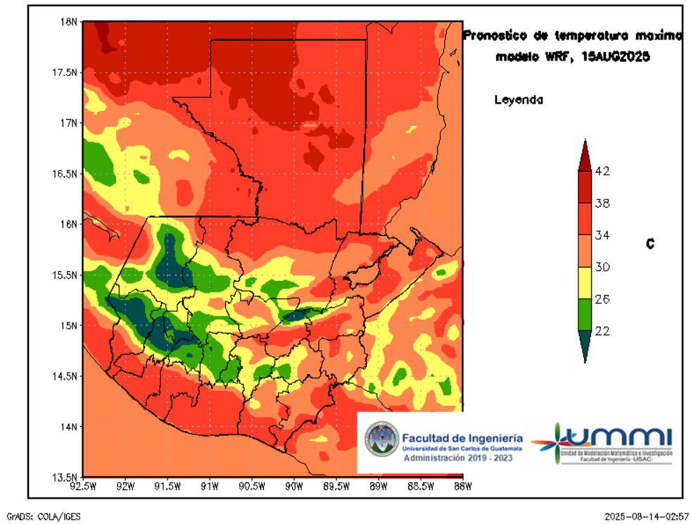
Figura 5: Pronóstico de temperatura máxima diaria del 15 de August
