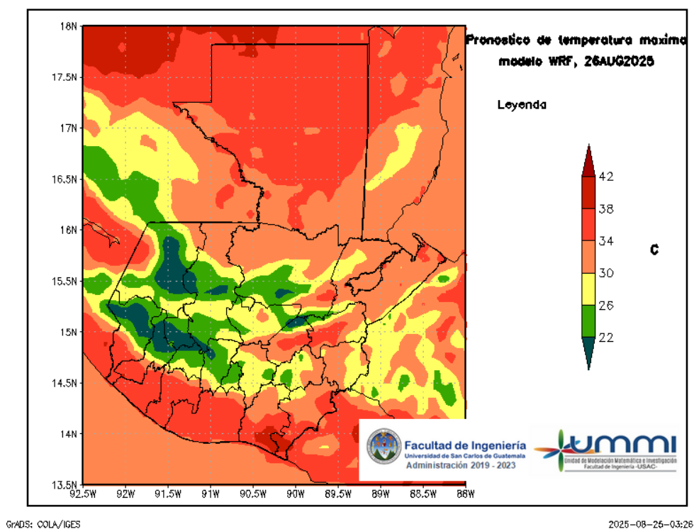
Figura 5: Pronóstico de temperatura máxima diaria del 26 de August
