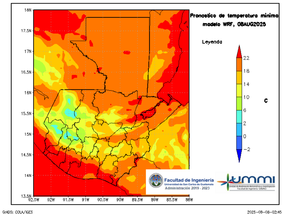
Figura 7: Pronóstico de temperatura mínima diaria del 09 de August
