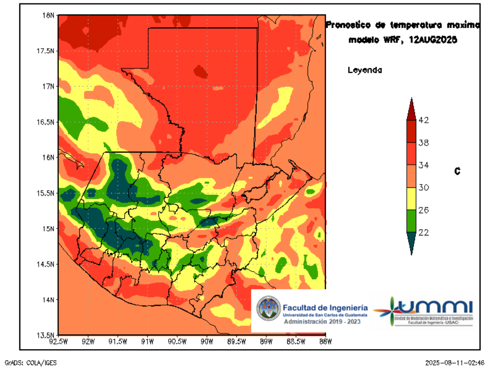
Figura 5: Pronóstico de temperatura máxima diaria del 12 de August
