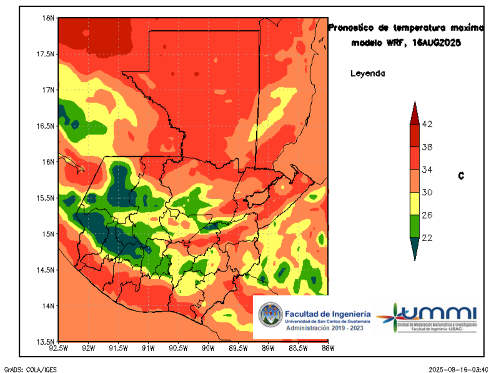
Figura 4: Pronóstico de temperatura máxima diaria del 16 de August
