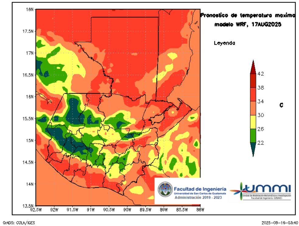
Figura 5: Pronóstico de temperatura máxima diaria del 17 de August
