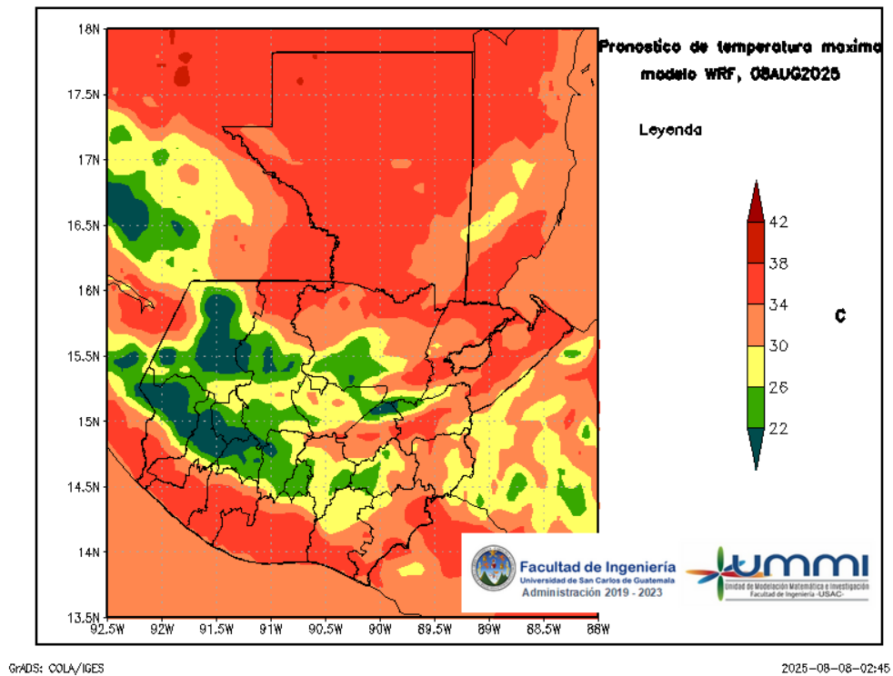
Figura 4: Pronóstico de temperatura máxima diaria del 08 de August
