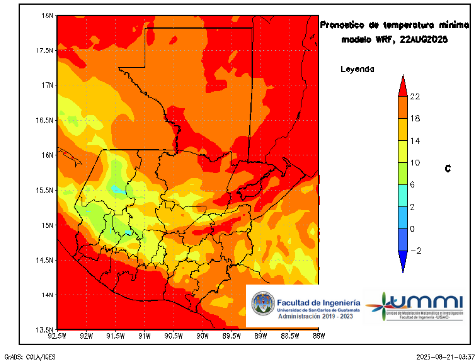
Figura 8: Pronóstico de temperatura mínima diaria del 23 de August
