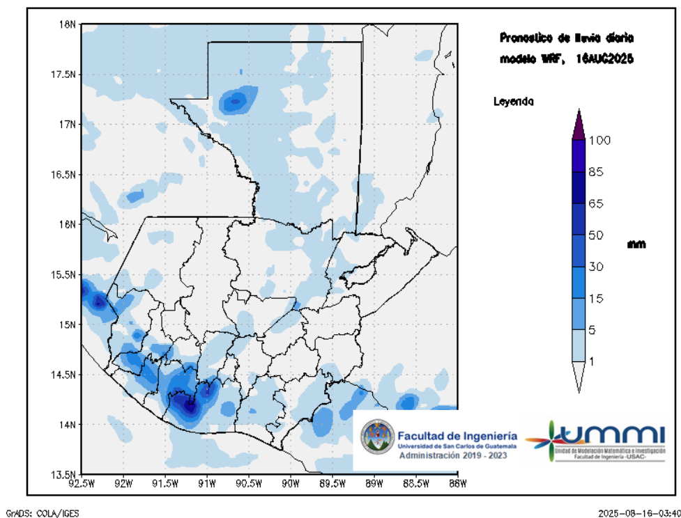
Figura 1: Pronóstico de lluvia diaria del 16 de August
