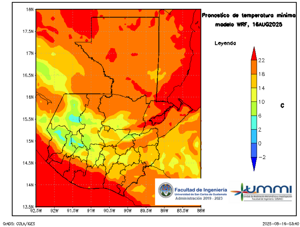
Figura 7: Pronóstico de temperatura mínima diaria del 17 de August
