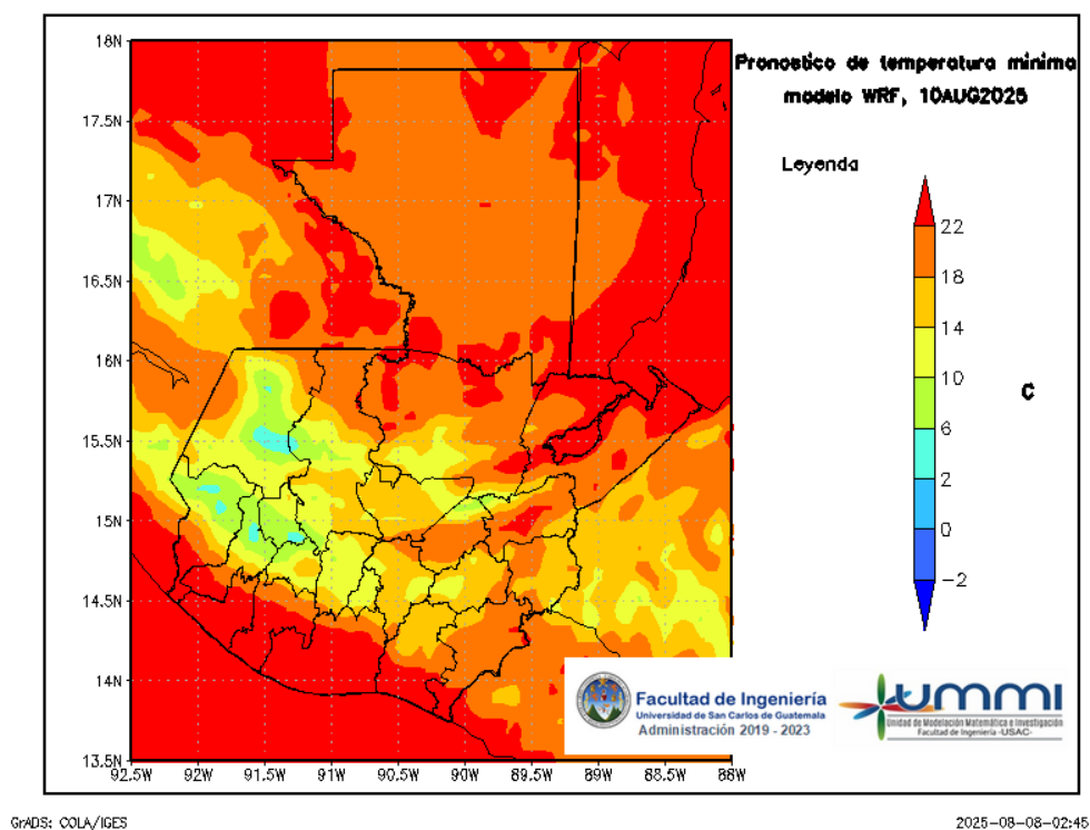
Figura 9: Pronóstico de temperatura mínima diaria del 11 de August
