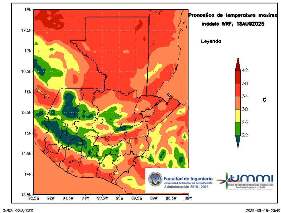
Figura 6: Pronóstico de temperatura máxima diaria del 18 de August
