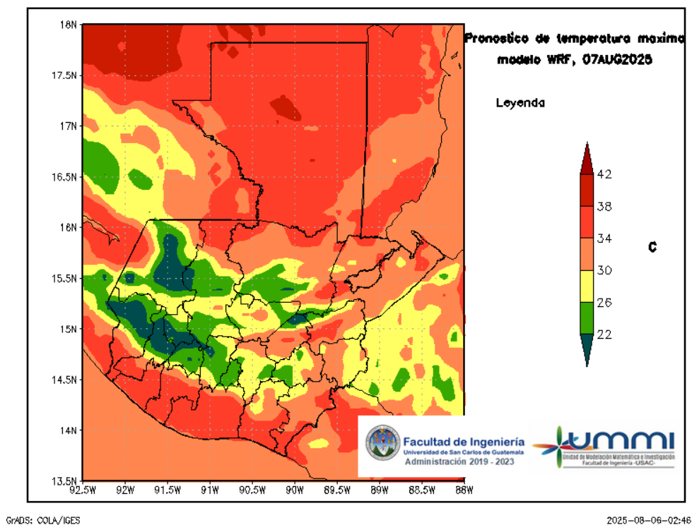
Figura 5: Pronóstico de temperatura máxima diaria del 07 de August
