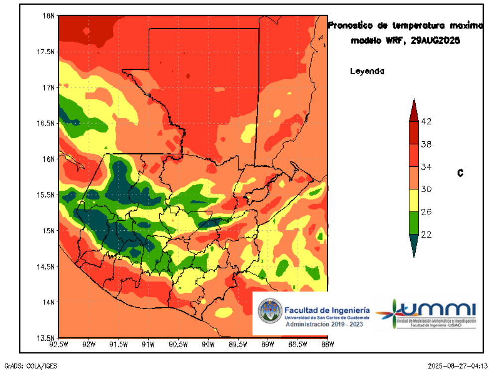
Figura 6: Pronóstico de temperatura máxima diaria del 29 de August
