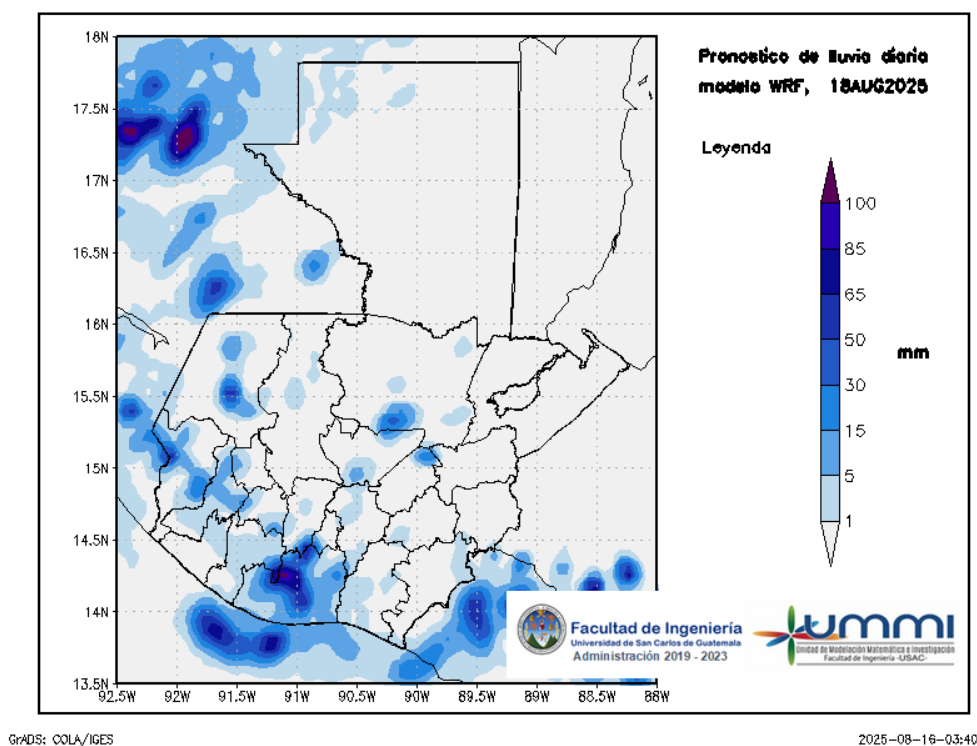
Figura 3: Pronóstico de lluvia diaria del 18 de August
