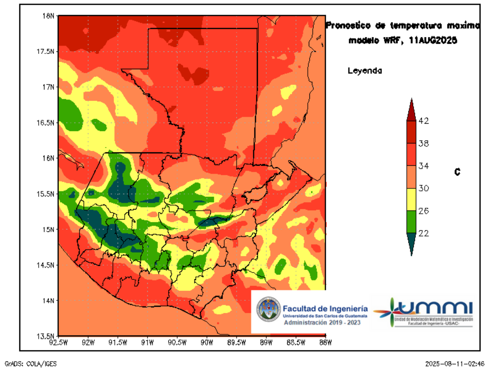
Figura 4: Pronóstico de temperatura máxima diaria del 11 de August
