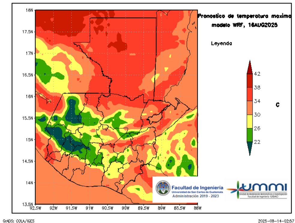
Figura 6: Pronóstico de temperatura máxima diaria del 16 de August
