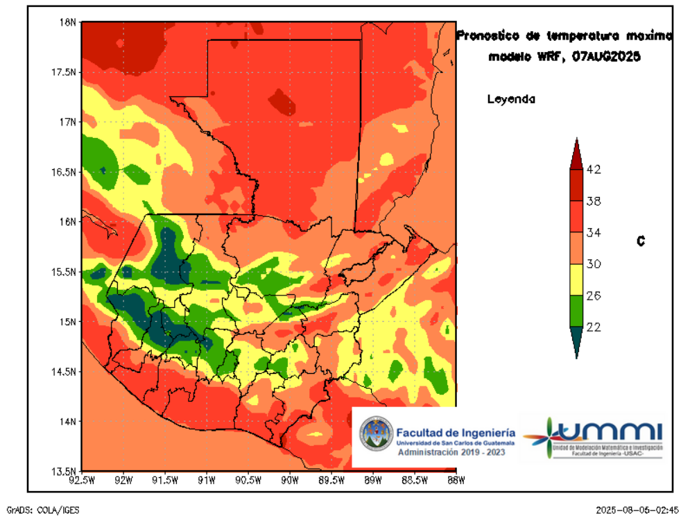
Figura 6: Pronóstico de temperatura máxima diaria del 07 de August
