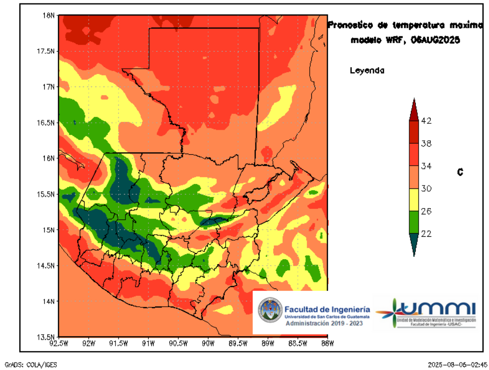
Figura 5: Pronóstico de temperatura máxima diaria del 06 de August
