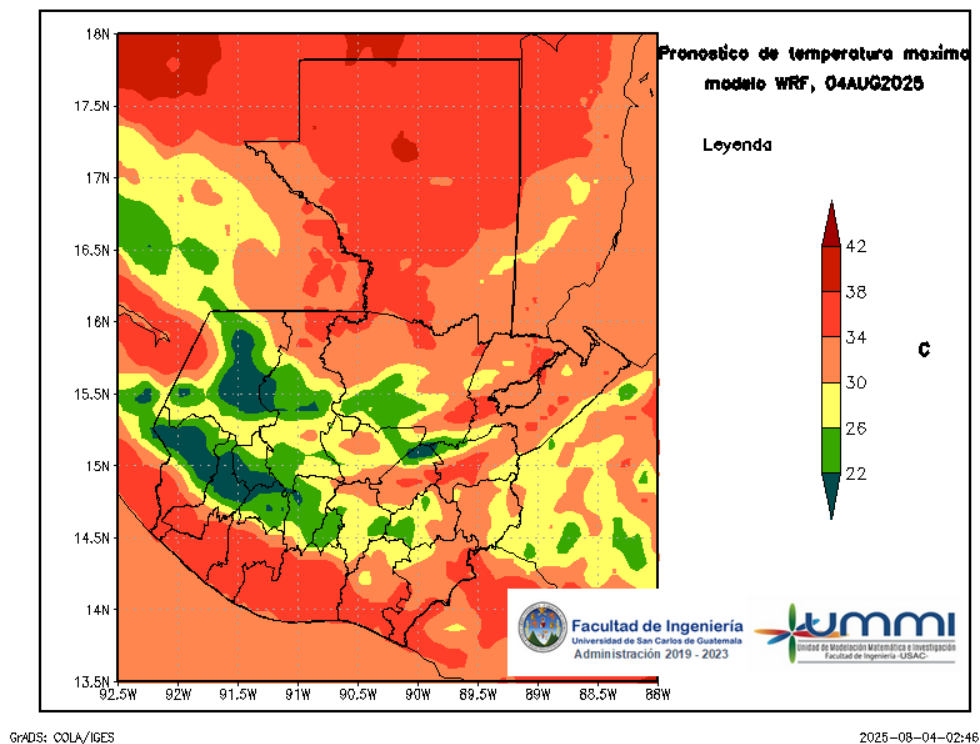
Figura 4: Pronóstico de temperatura máxima diaria del 04 de August
