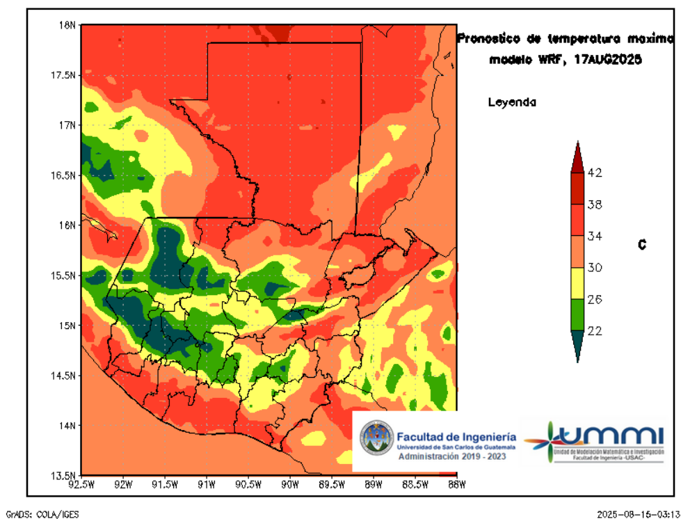
Figura 6: Pronóstico de temperatura máxima diaria del 17 de August
