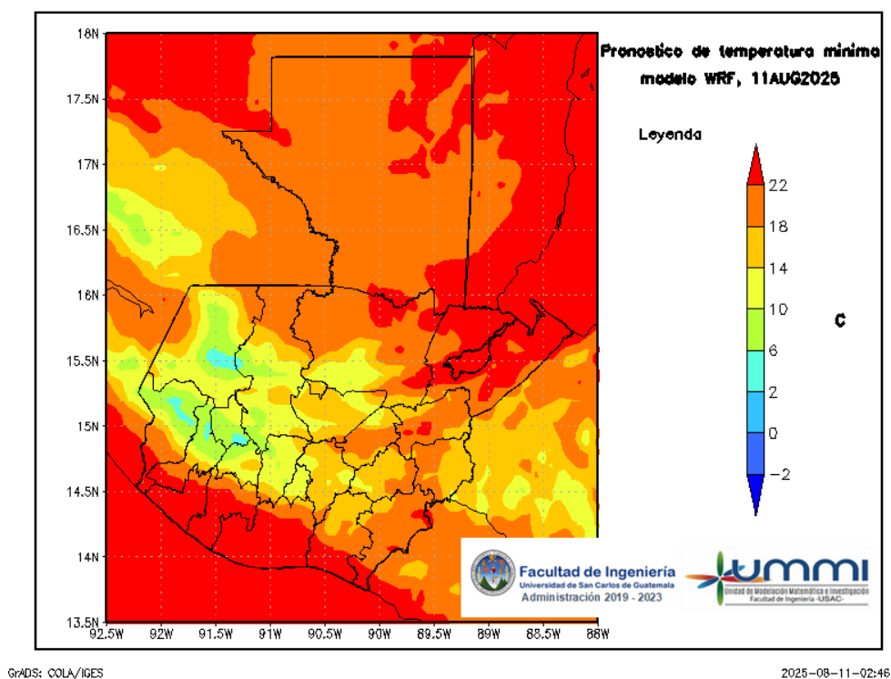
Figura 7: Pronóstico de temperatura mínima diaria del 12 de August
