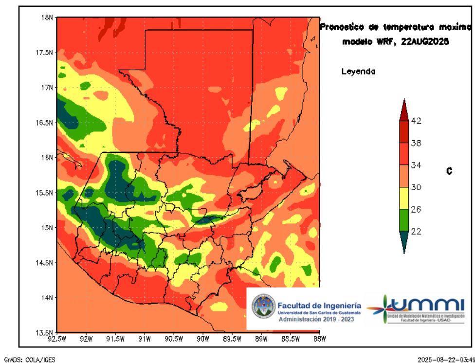
Figura 4: Pronóstico de temperatura máxima diaria del 22 de August
