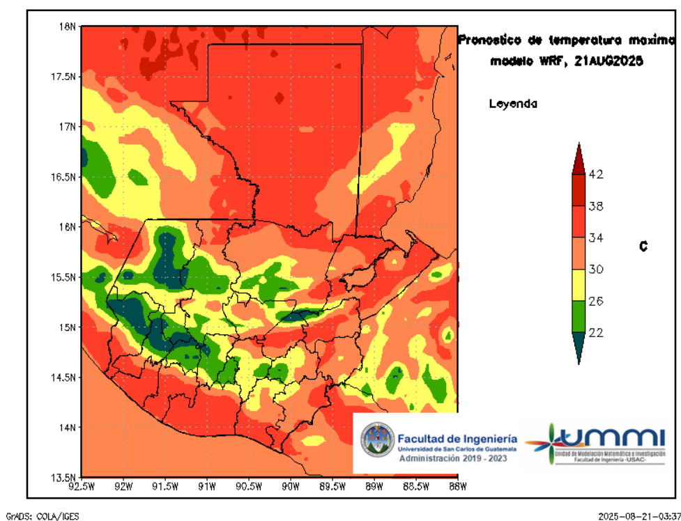
Figura 4: Pronóstico de temperatura máxima diaria del 21 de August
