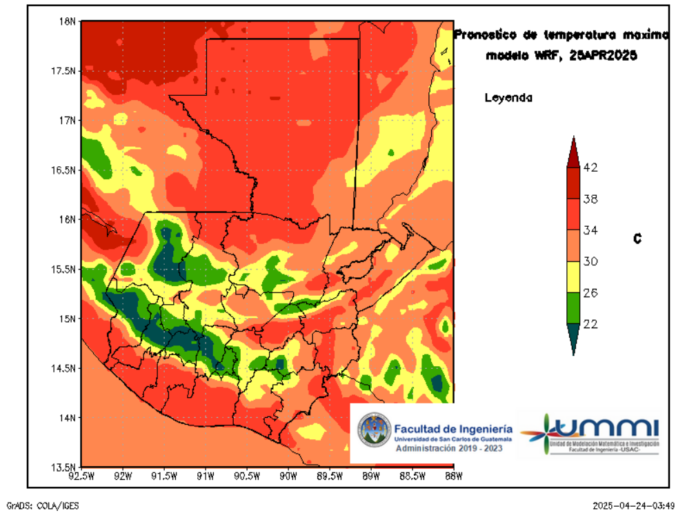
Figura 5: Pronóstico de temperatura máxima diaria del 25 de April
