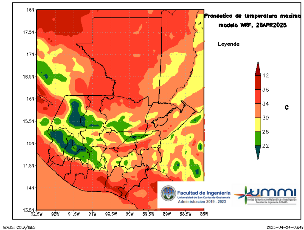
Figura 6: Pronóstico de temperatura máxima diaria del 26 de April
