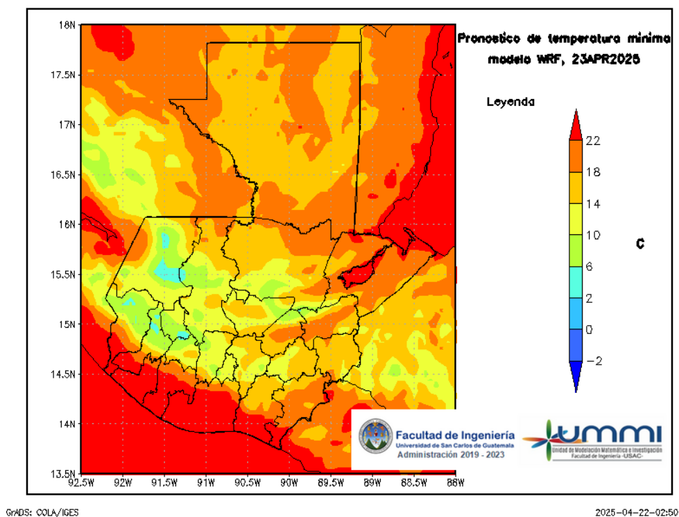
Figura 8: Pronóstico de temperatura mínima diaria del 24 de April
