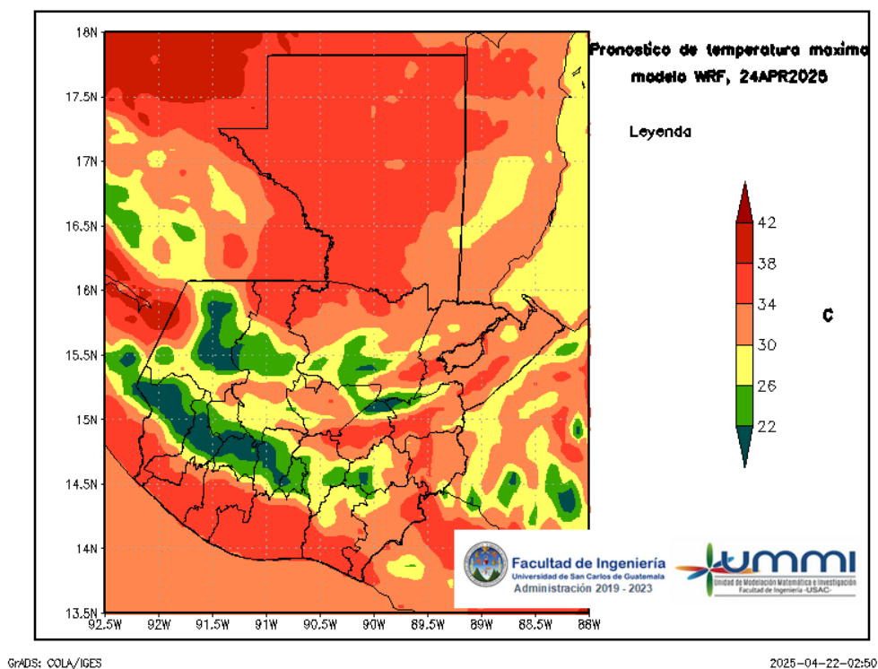
Figura 6: Pronóstico de temperatura máxima diaria del 24 de April
