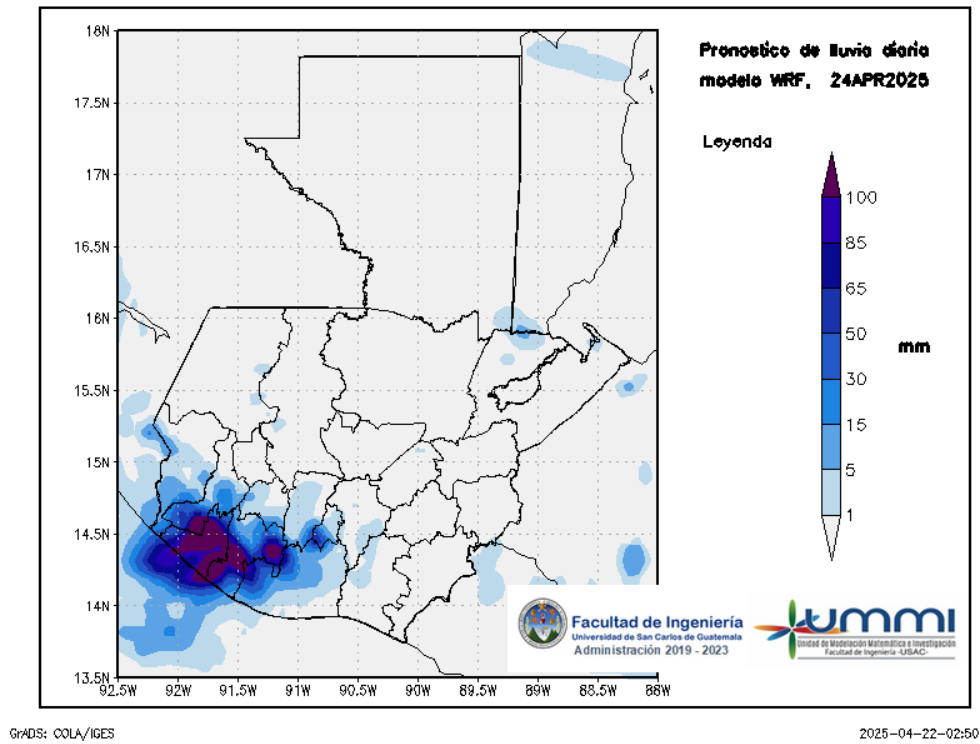
Figura 3: Pronóstico de lluvia diaria del 24 de April
