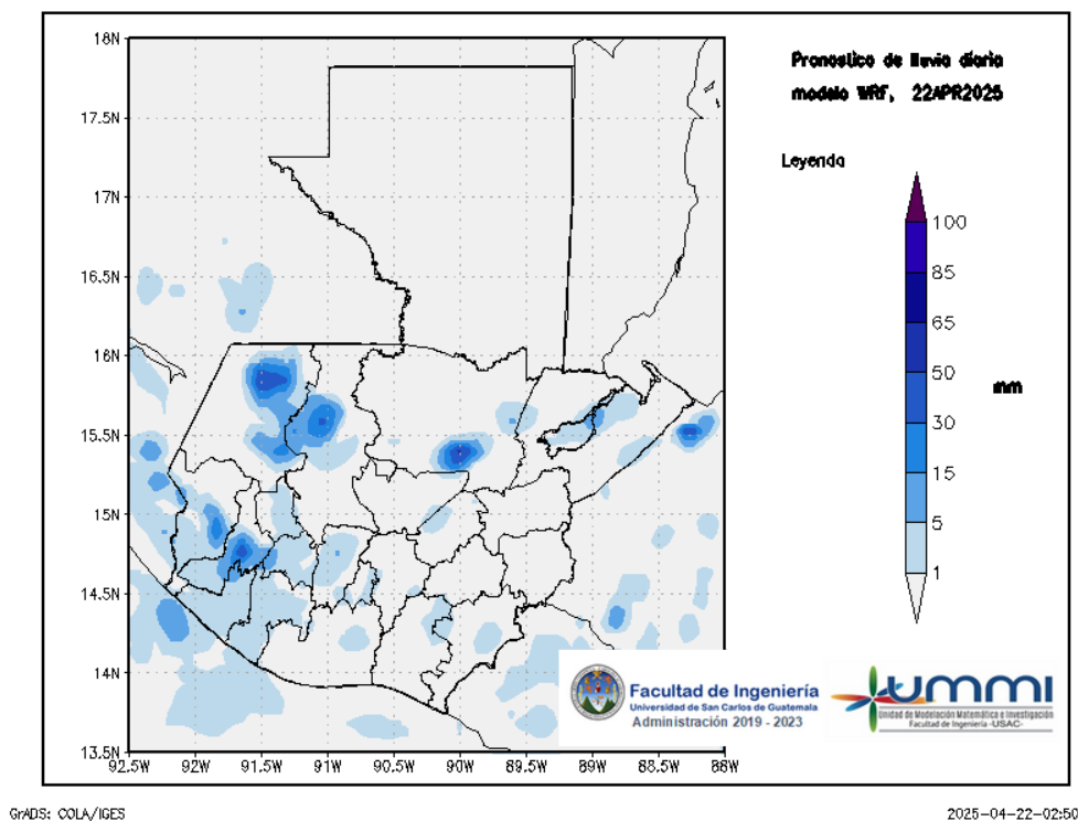
Figura 1: Pronóstico de lluvia diaria del 22 de April
