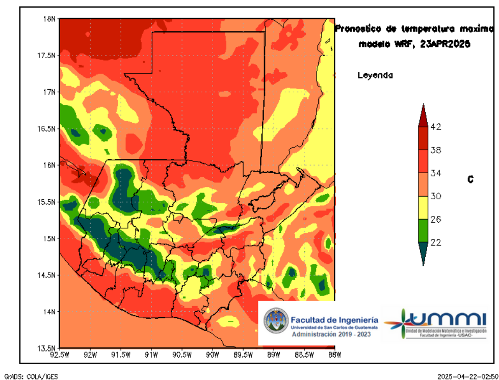
Figura 5: Pronóstico de temperatura máxima diaria del 23 de April
