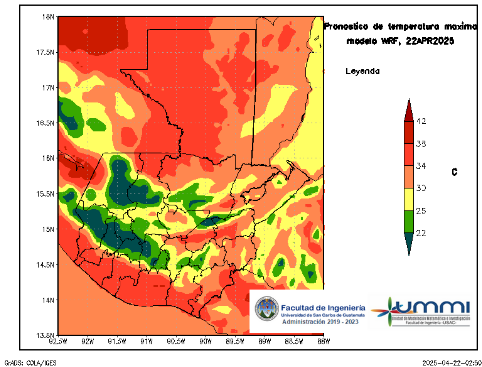
Figura 4: Pronóstico de temperatura máxima diaria del 22 de April
