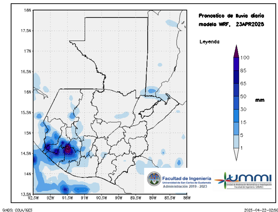
Figura 2: Pronóstico de lluvia diaria del 23 de April
