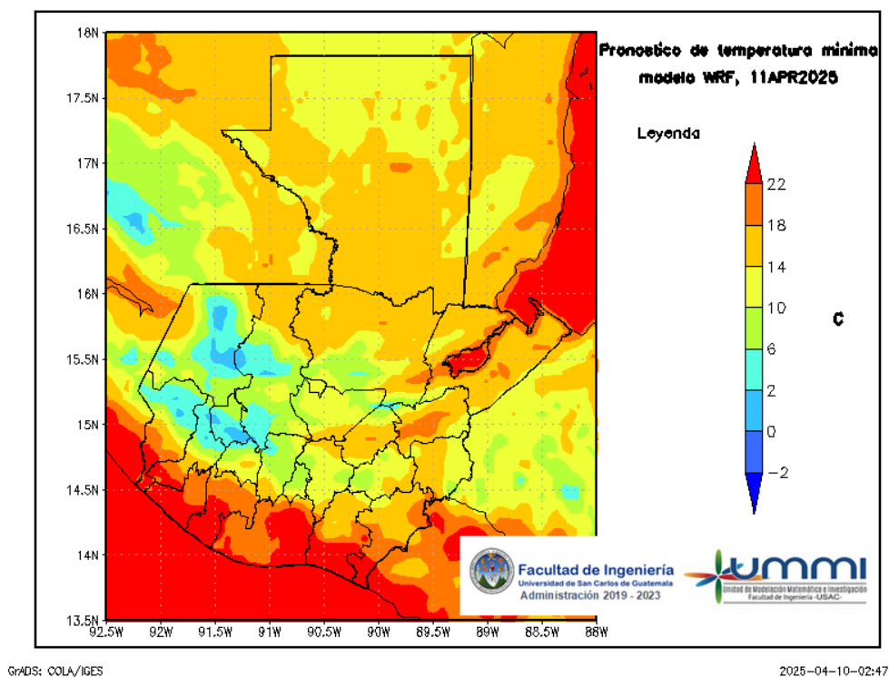
Figura 8: Pronóstico de temperatura mínima diaria del 12 de April
