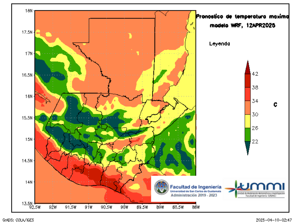
Figura 6: Pronóstico de temperatura máxima diaria del 12 de April
