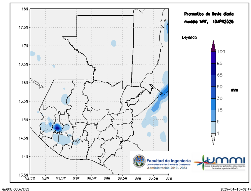
Figura 1: Pronóstico de lluvia diaria del 10 de April
