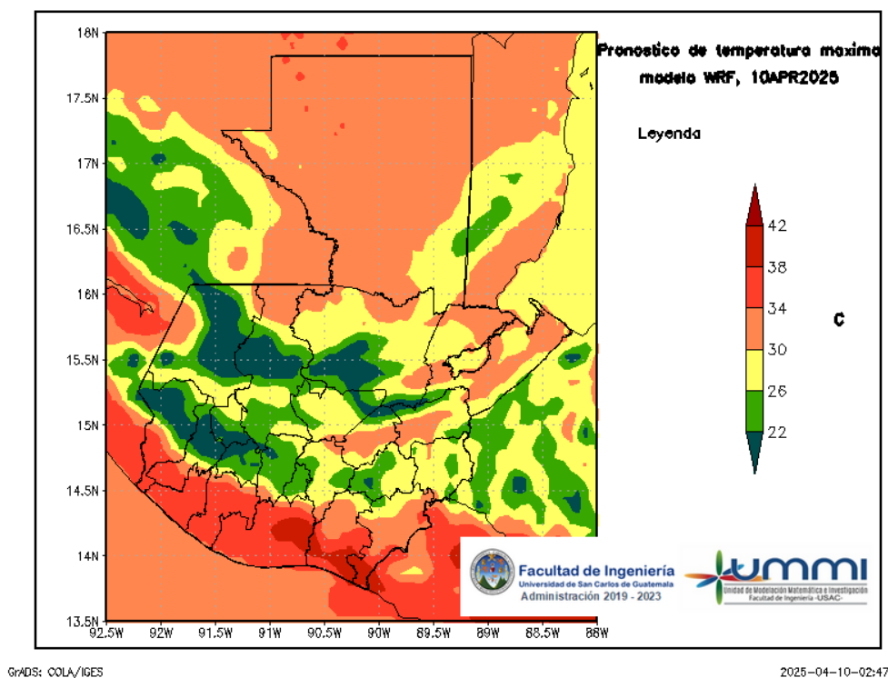
Figura 4: Pronóstico de temperatura máxima diaria del 10 de April
