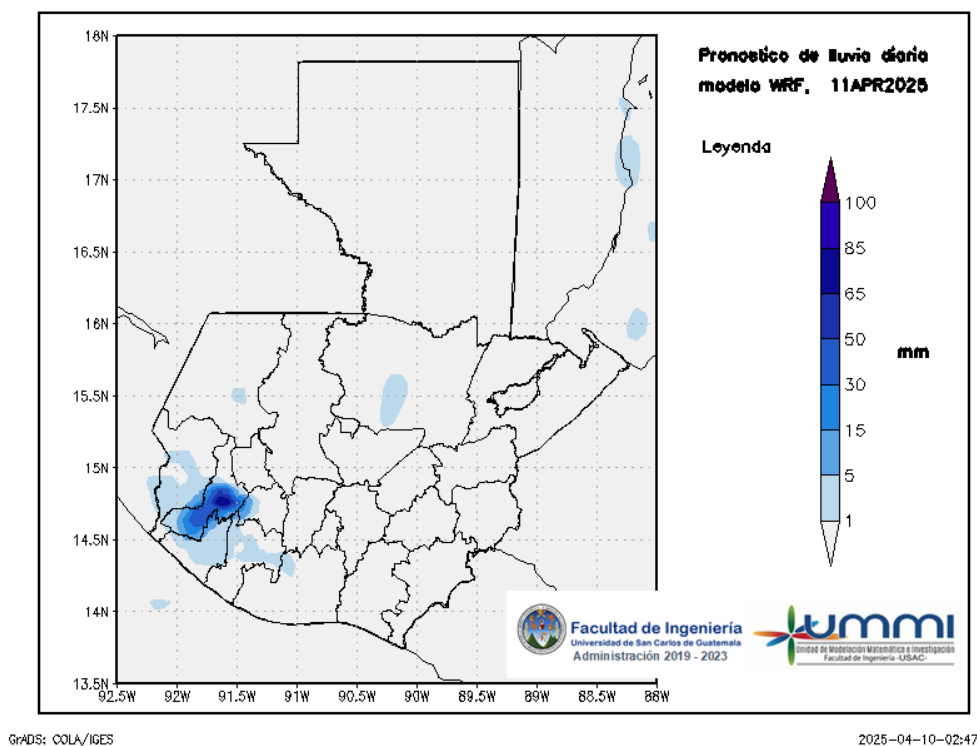
Figura 2: Pronóstico de lluvia diaria del 11 de April
