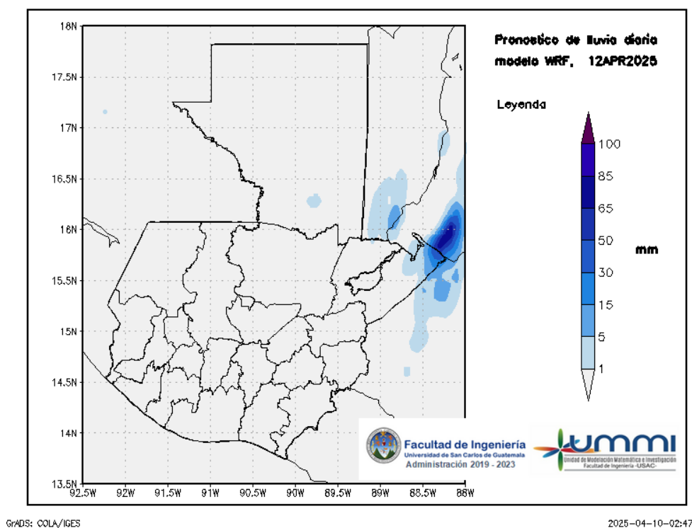
Figura 3: Pronóstico de lluvia diaria del 12 de April
