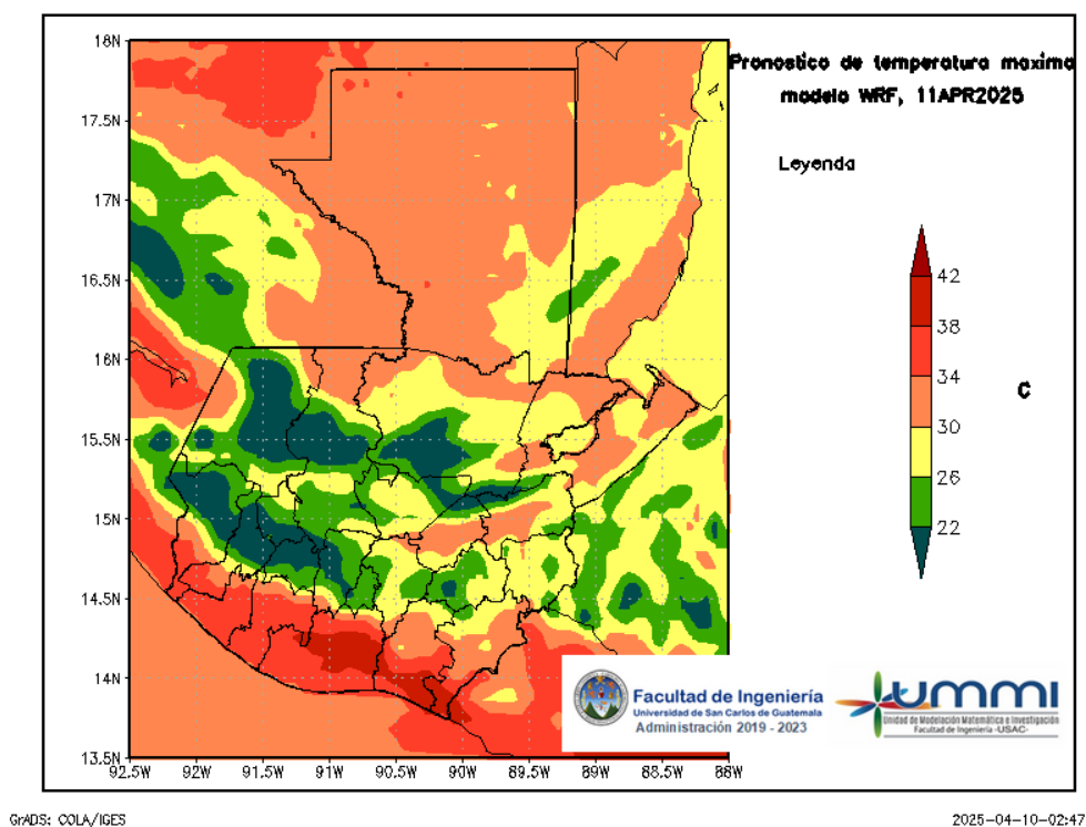
Figura 5: Pronóstico de temperatura máxima diaria del 11 de April
