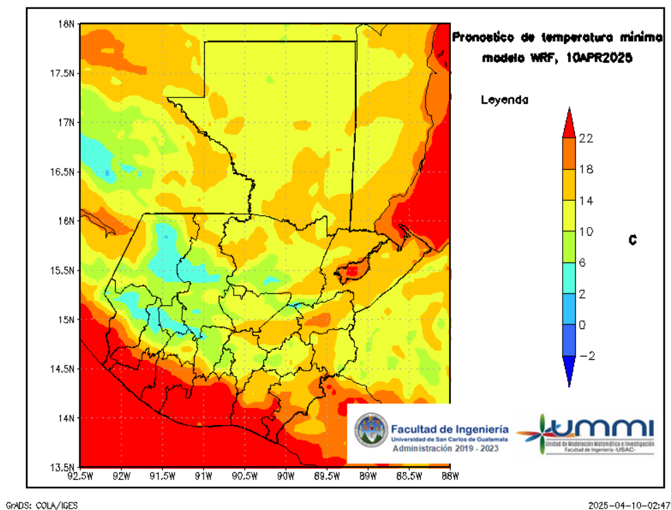
Figura 7: Pronóstico de temperatura mínima diaria del 11 de April
