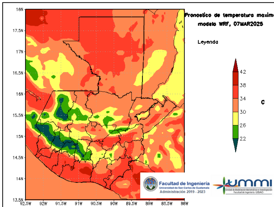
Figura 4: Pronóstico de temperatura máxima diaria del 07 de March
