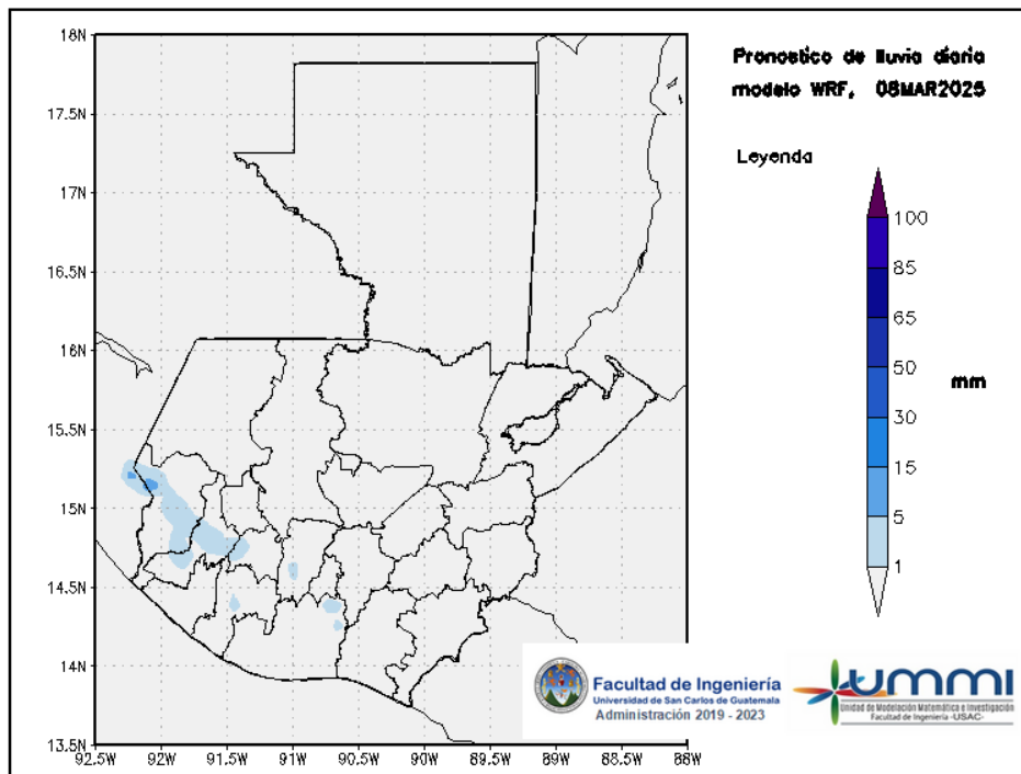
Figura 2: Pronóstico de lluvia diaria del 08 de March
