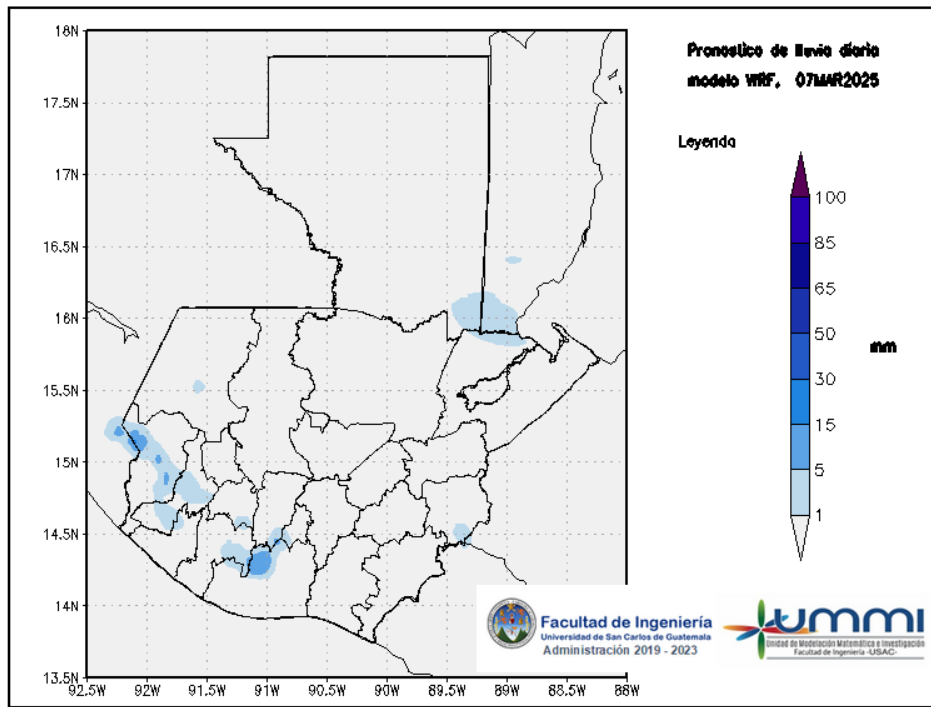
Figura 1: Pronóstico de lluvia diaria del 07 de March
