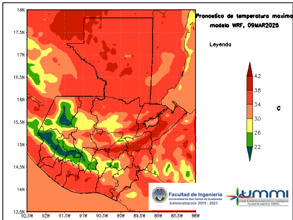
Figura 6: Pronóstico de temperatura máxima diaria del 09 de March
