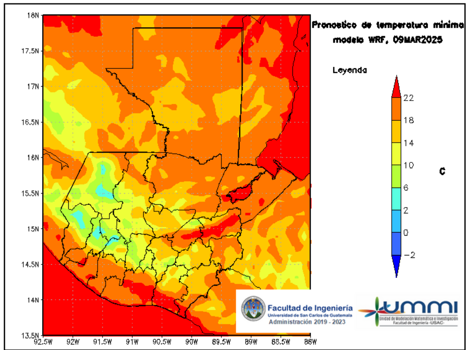
Figura 9: Pronóstico de temperatura mínima diaria del 10 de March
