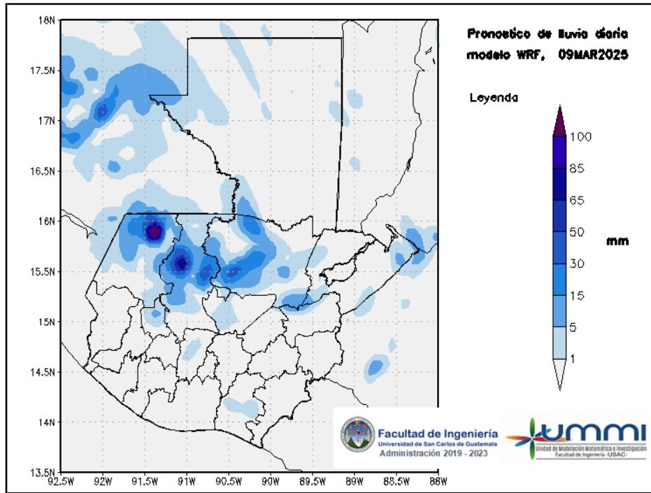
Figura 3: Pronóstico de lluvia diaria del 09 de March
