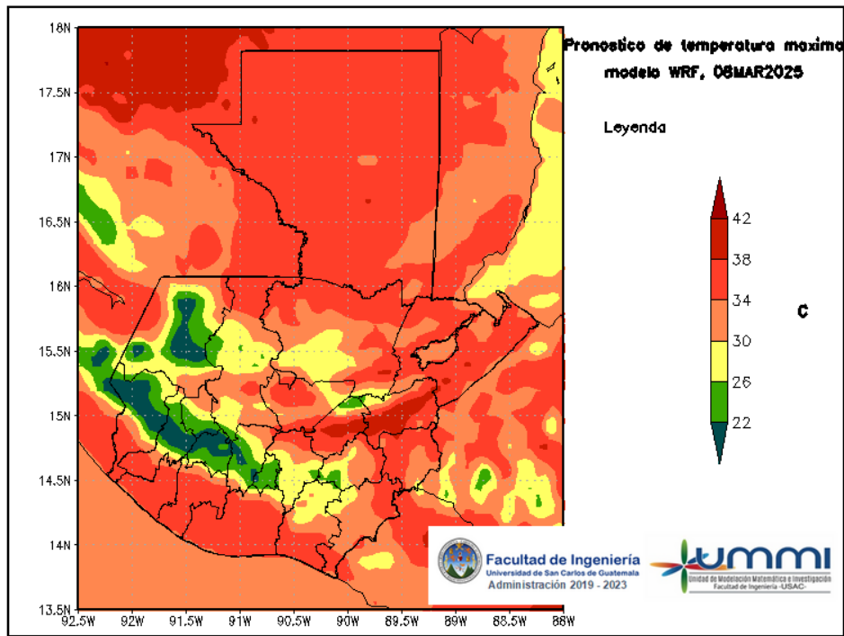
Figura 5: Pronóstico de temperatura máxima diaria del 08 de March
