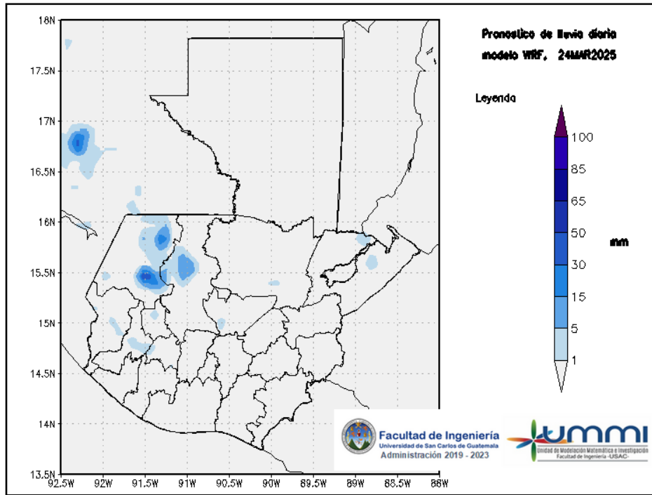
Figura 1: Pronóstico de lluvia diaria del 24 de March
