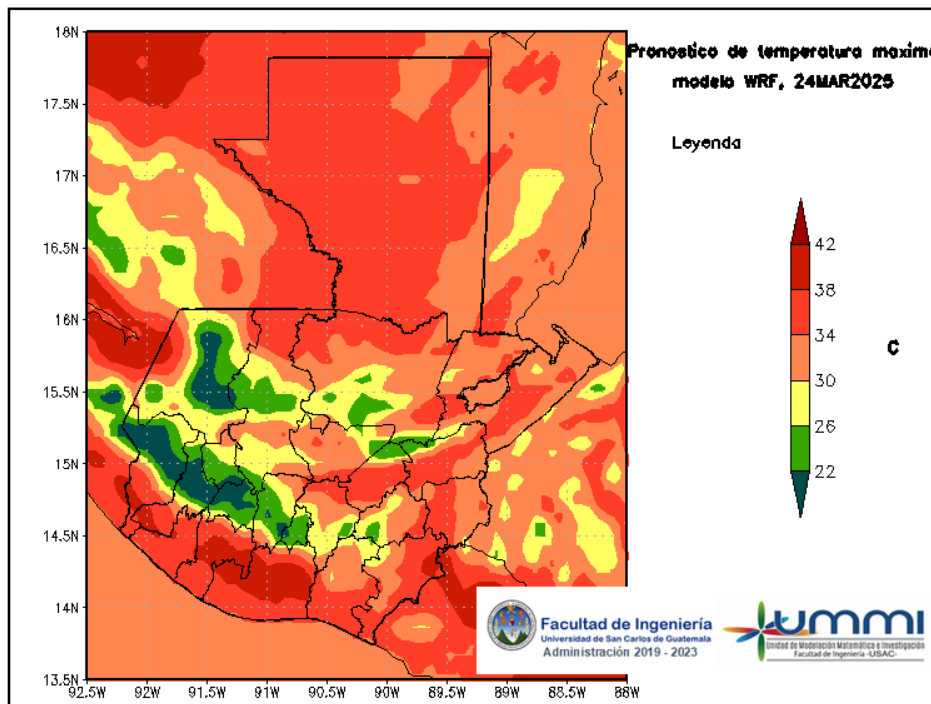
Figura 4: Pronóstico de temperatura máxima diaria del 24 de March
