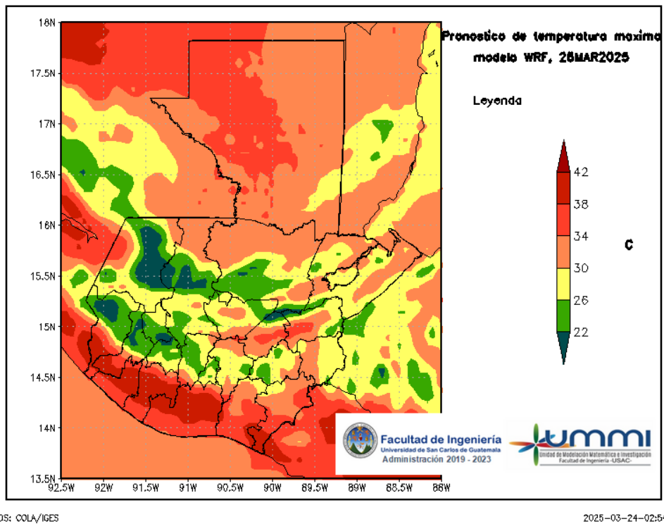
Figura 6: Pronóstico de temperatura máxima diaria del 26 de March
