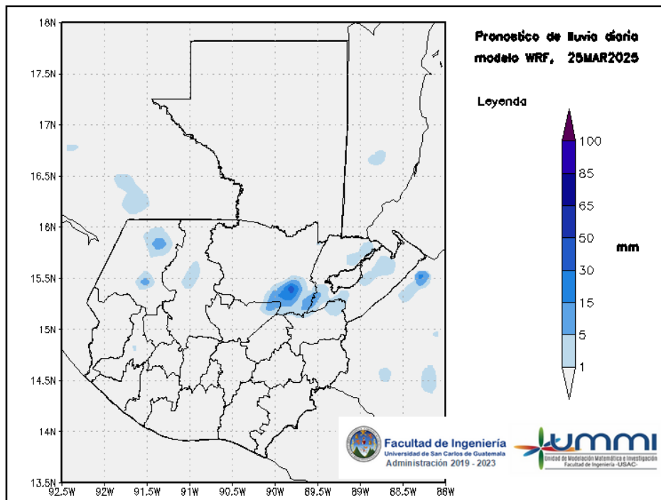
Figura 2: Pronóstico de lluvia diaria del 25 de March
