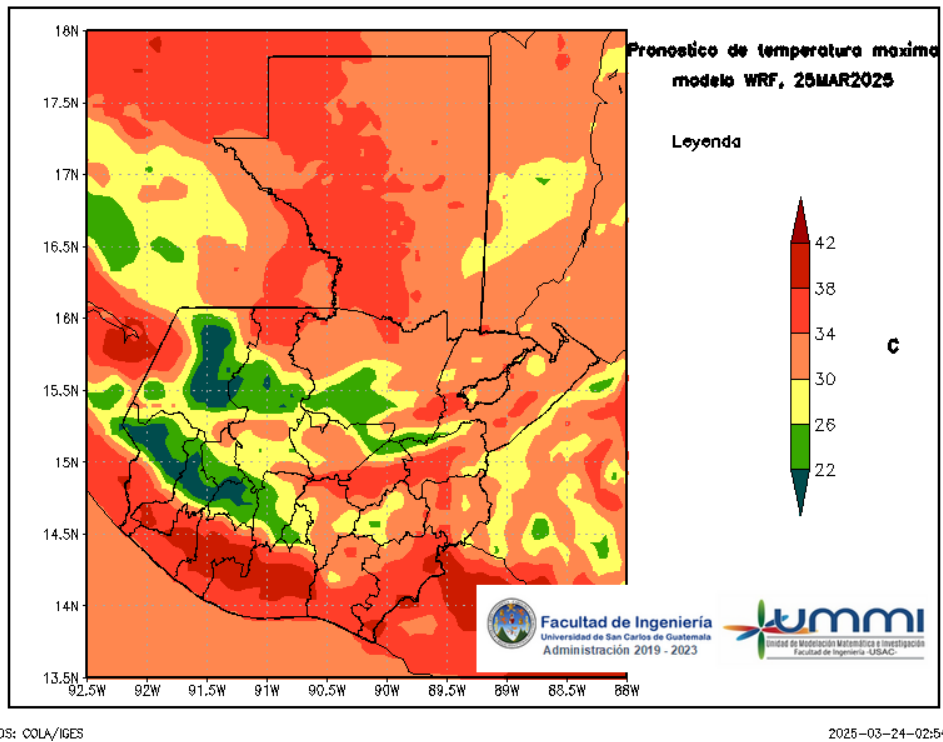
Figura 5: Pronóstico de temperatura máxima diaria del 25 de March
