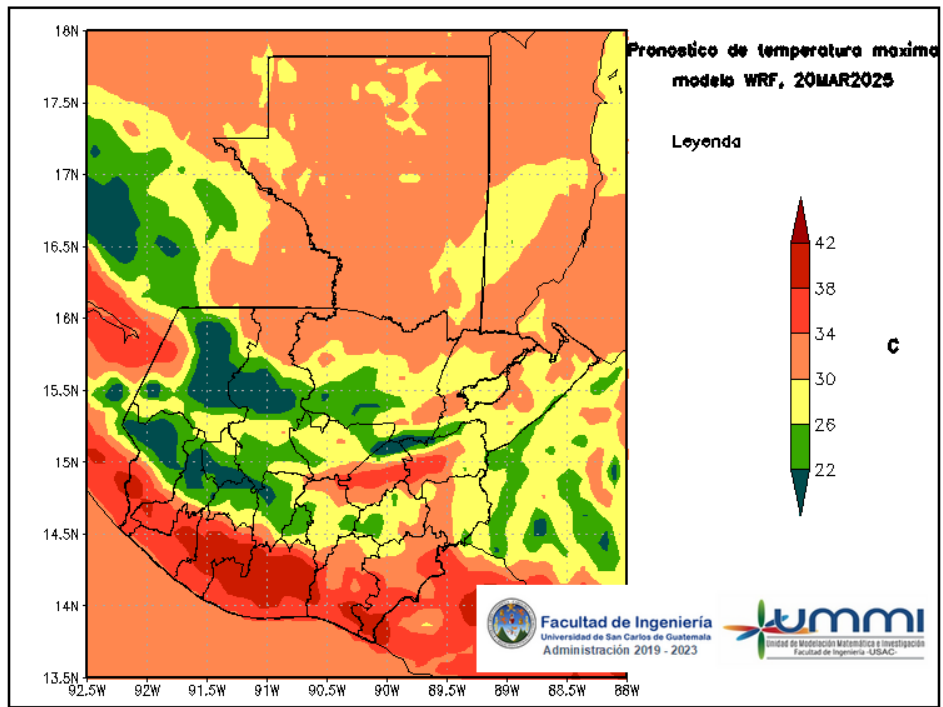
Figura 5: Pronóstico de temperatura máxima diaria del 20 de March
