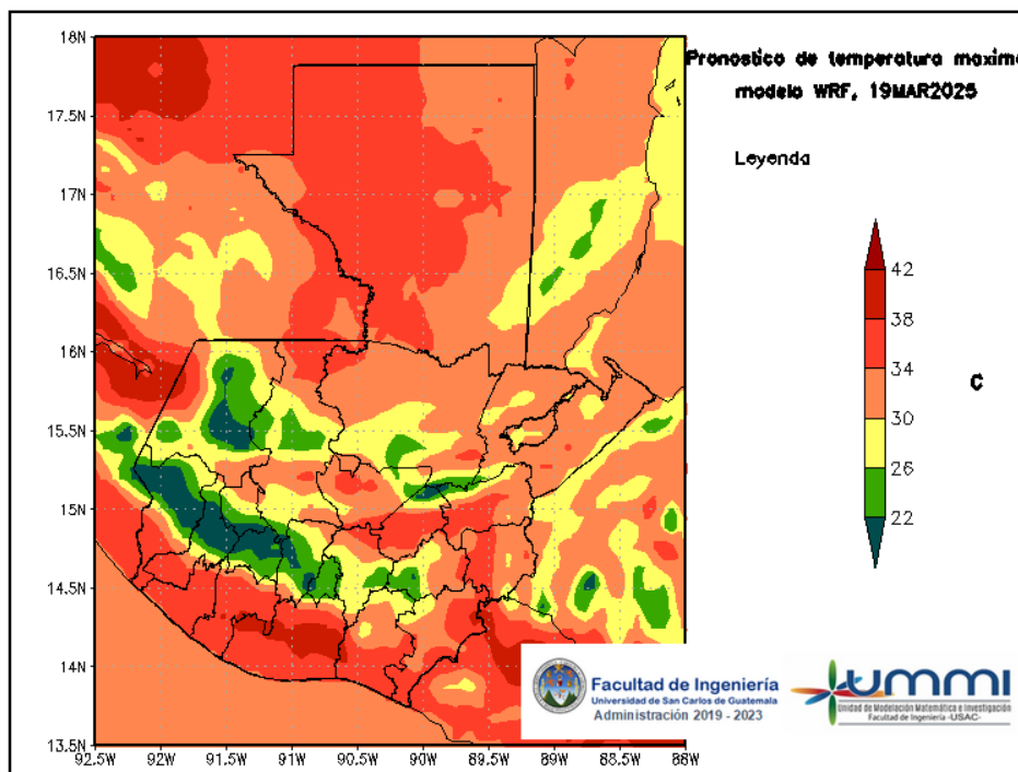
Figura 4: Pronóstico de temperatura máxima diaria del 19 de March
