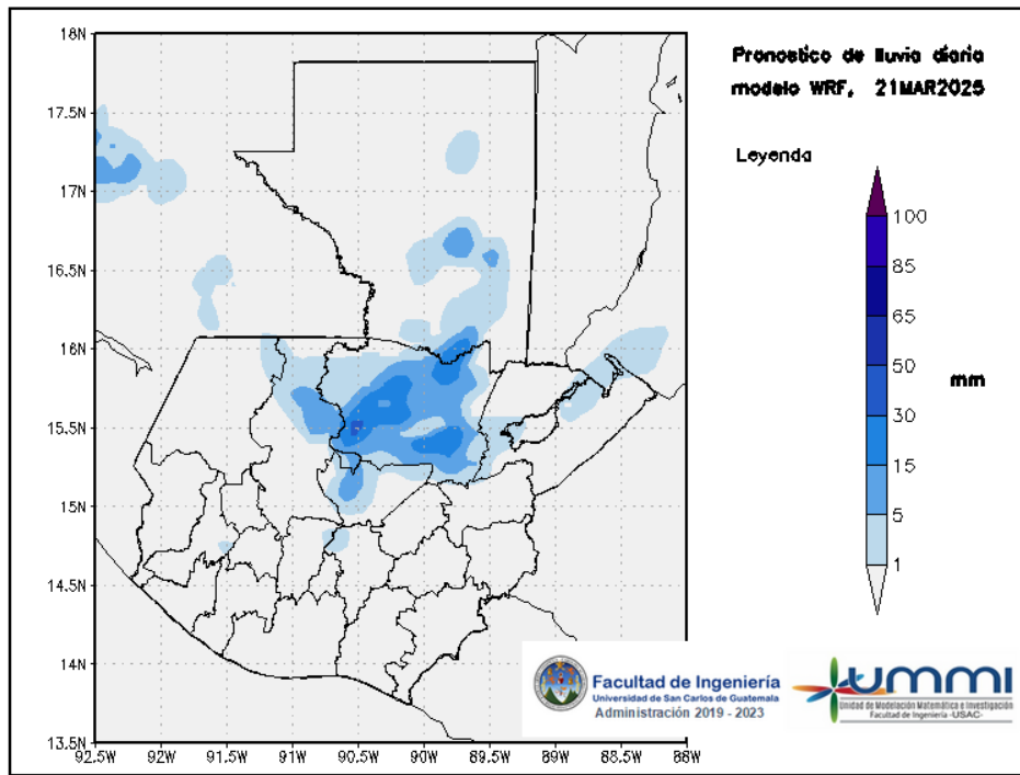
Figura 3: Pronóstico de lluvia diaria del 21 de March
