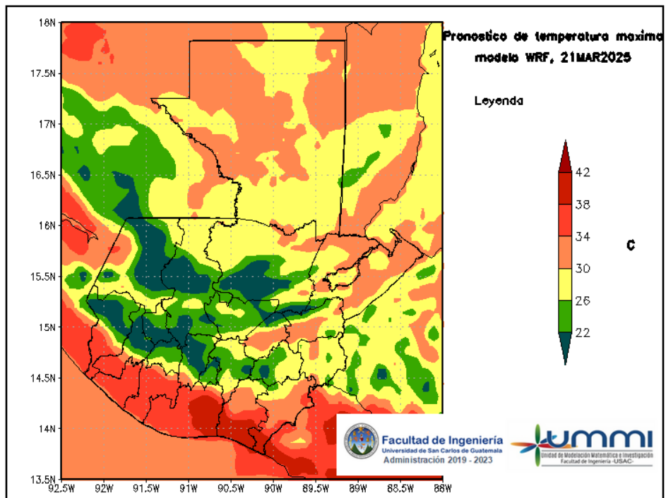
Figura 6: Pronóstico de temperatura máxima diaria del 21 de March
