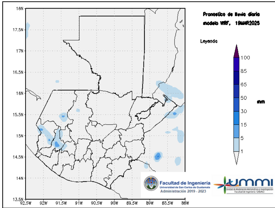
Figura 1: Pronóstico de lluvia diaria del 19 de March
