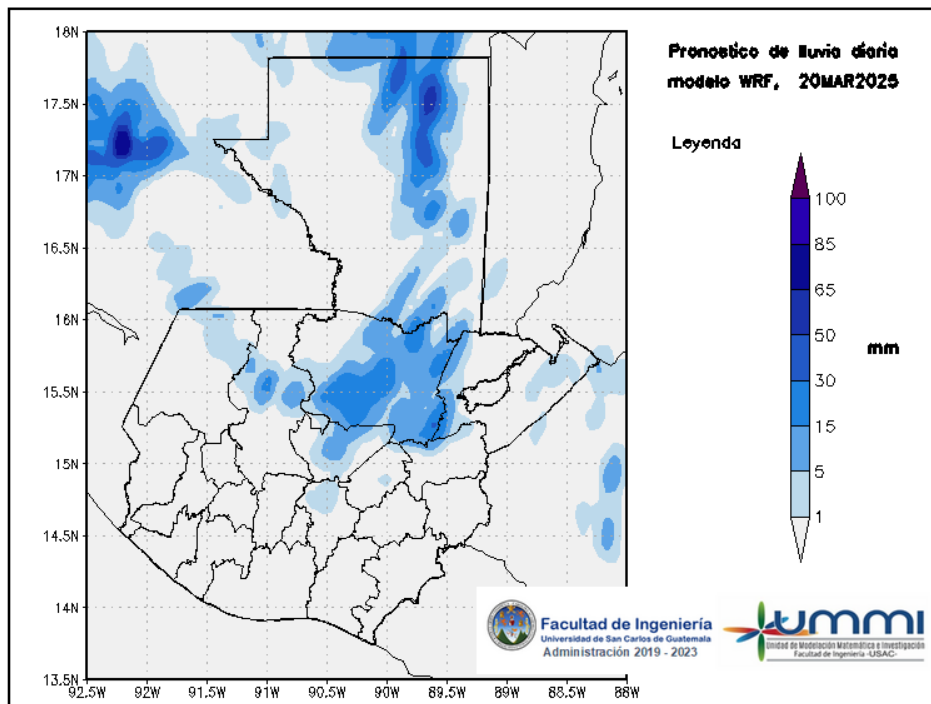
Figura 2: Pronóstico de lluvia diaria del 20 de March
