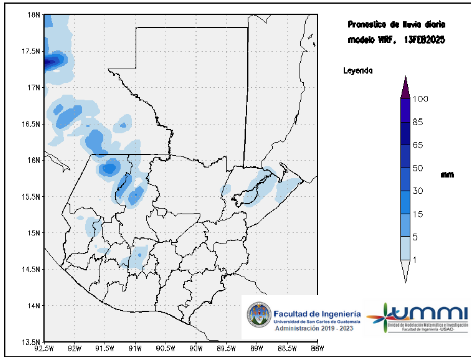
Figura 1: Pronóstico de lluvia diaria del 13 de February
