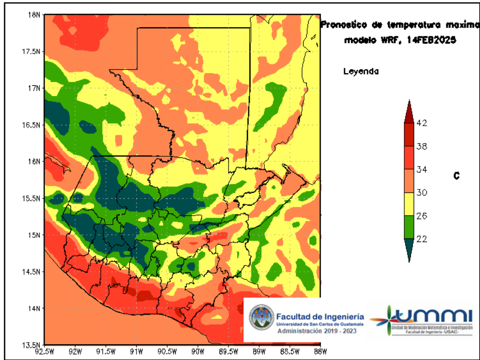
Figura 5: Pronóstico de temperatura máxima diaria del 14 de February
