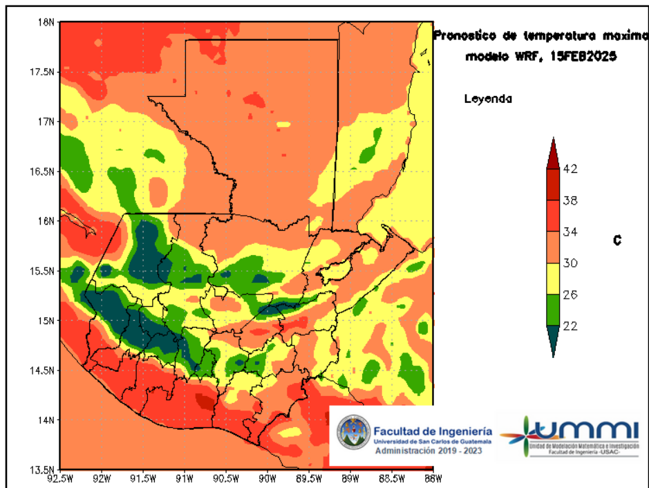
Figura 6: Pronóstico de temperatura máxima diaria del 15 de February
