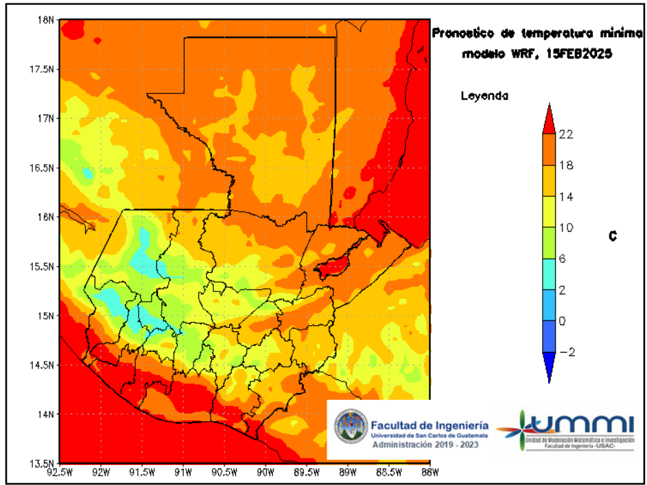
Figura 9: Pronóstico de temperatura mínima diaria del 16 de February
