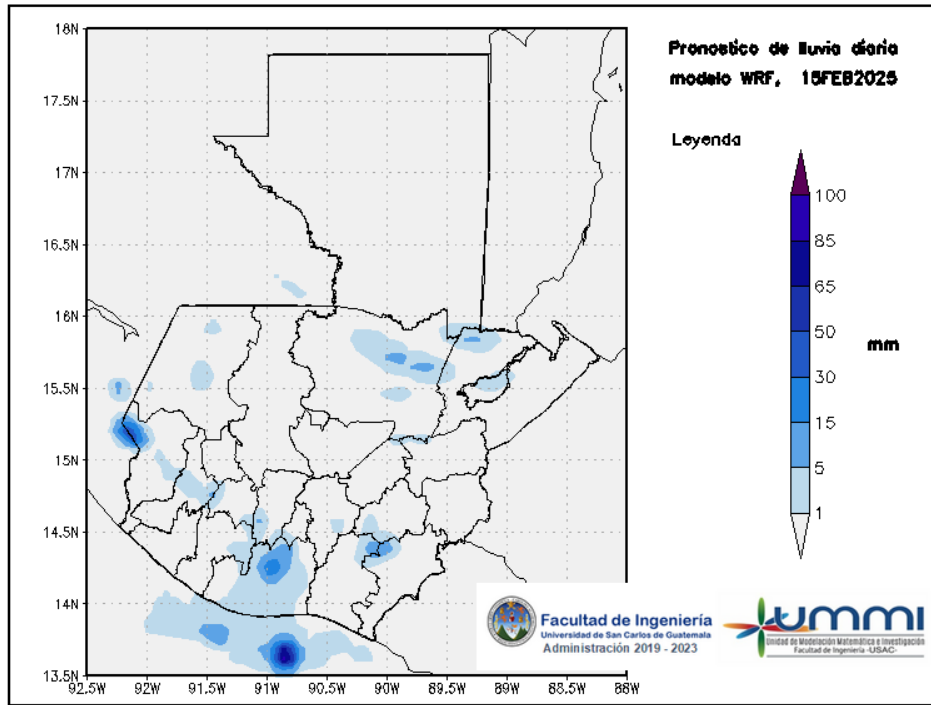
Figura 3: Pronóstico de lluvia diaria del 15 de February
