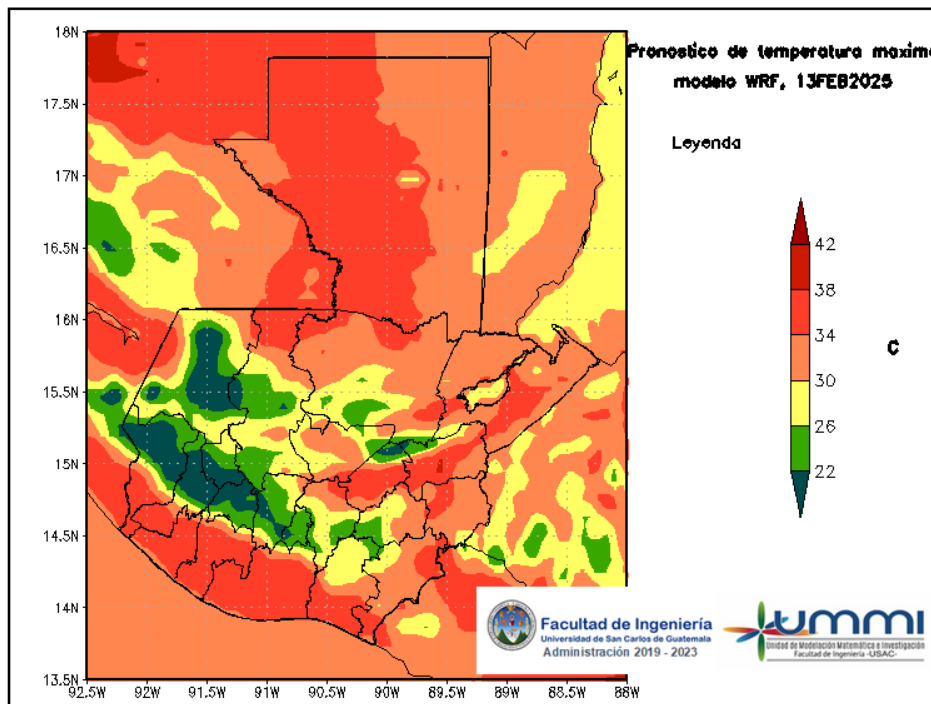
Figura 4: Pronóstico de temperatura máxima diaria del 13 de February
