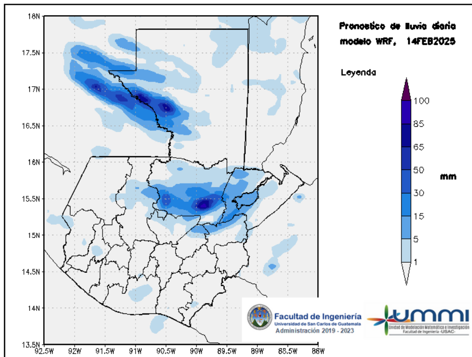
Figura 2: Pronóstico de lluvia diaria del 14 de February
