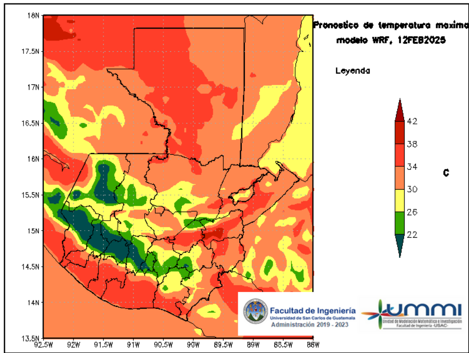
Figura 5: Pronóstico de temperatura máxima diaria del 12 de February
