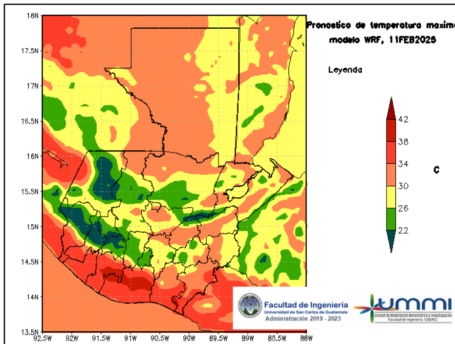
Figura 4: Pronóstico de temperatura máxima diaria del 11 de February
