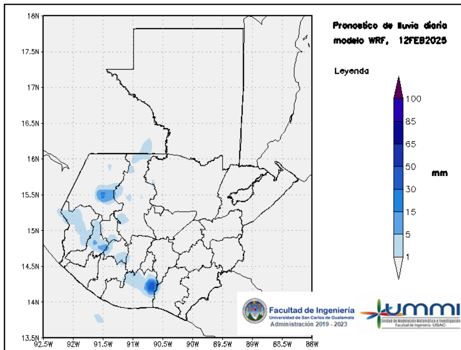
Figura 2: Pronóstico de lluvia diaria del 12 de February
