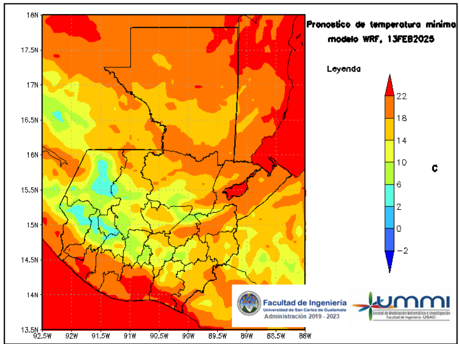
Figura 9: Pronóstico de temperatura mínima diaria del 14 de February
