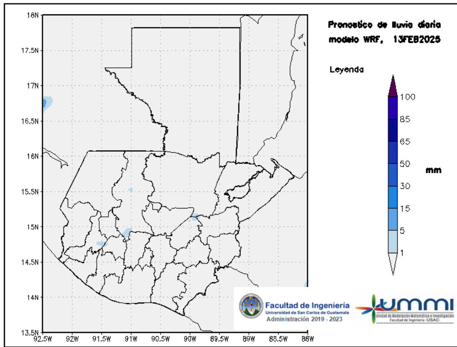
Figura 3: Pronóstico de lluvia diaria del 13 de February
