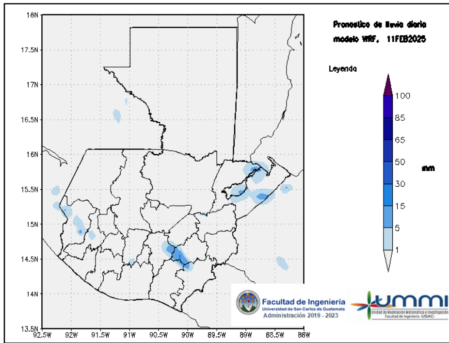
Figura 1: Pronóstico de lluvia diaria del 11 de February
