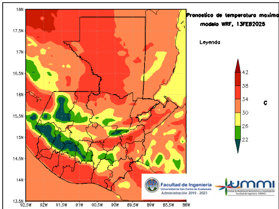
Figura 6: Pronóstico de temperatura máxima diaria del 13 de February
