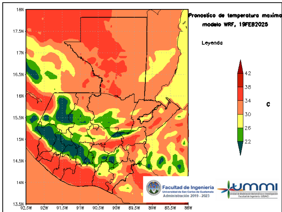
Figura 6: Pronóstico de temperatura máxima diaria del 19 de February
