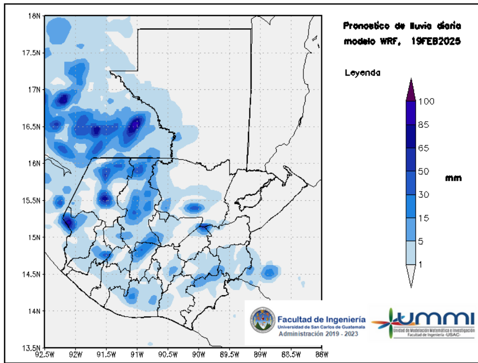
Figura 3: Pronóstico de lluvia diaria del 19 de February
