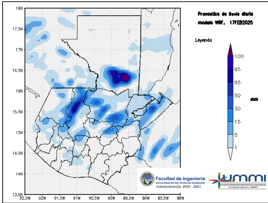
Figura 1: Pronóstico de lluvia diaria del 17 de February
