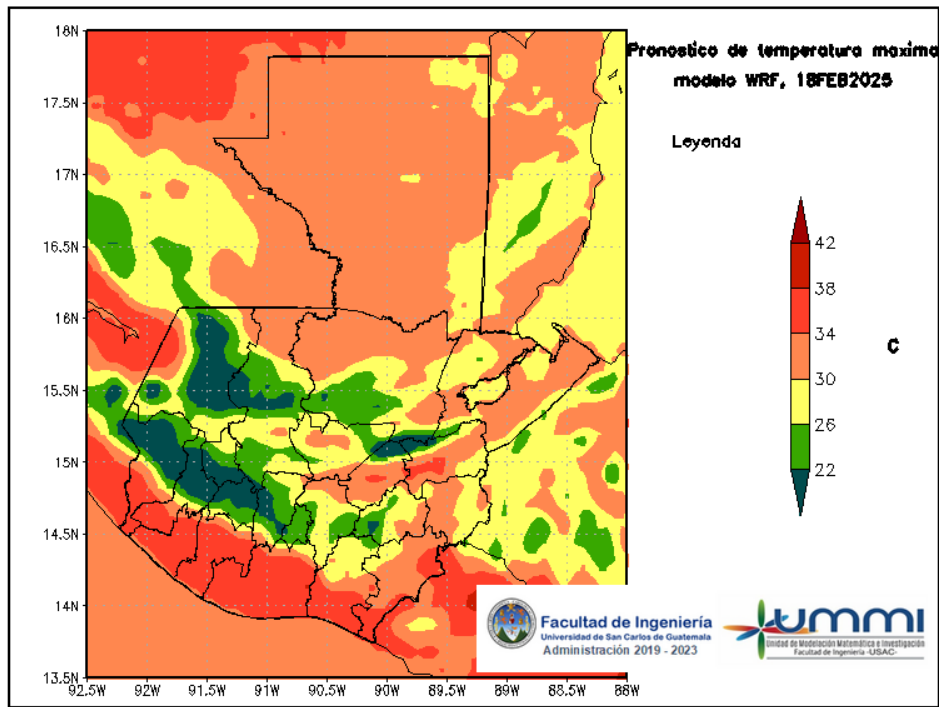
Figura 5: Pronóstico de temperatura máxima diaria del 18 de February
