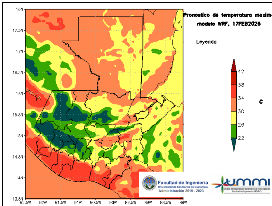
Figura 4: Pronóstico de temperatura máxima diaria del 17 de February
