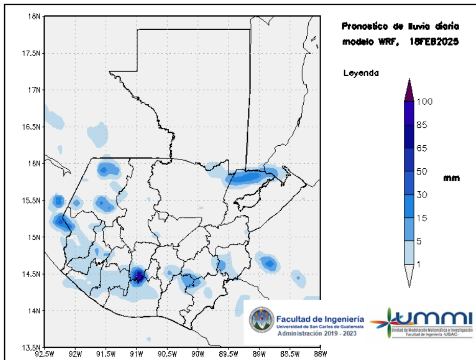
Figura 2: Pronóstico de lluvia diaria del 18 de February
