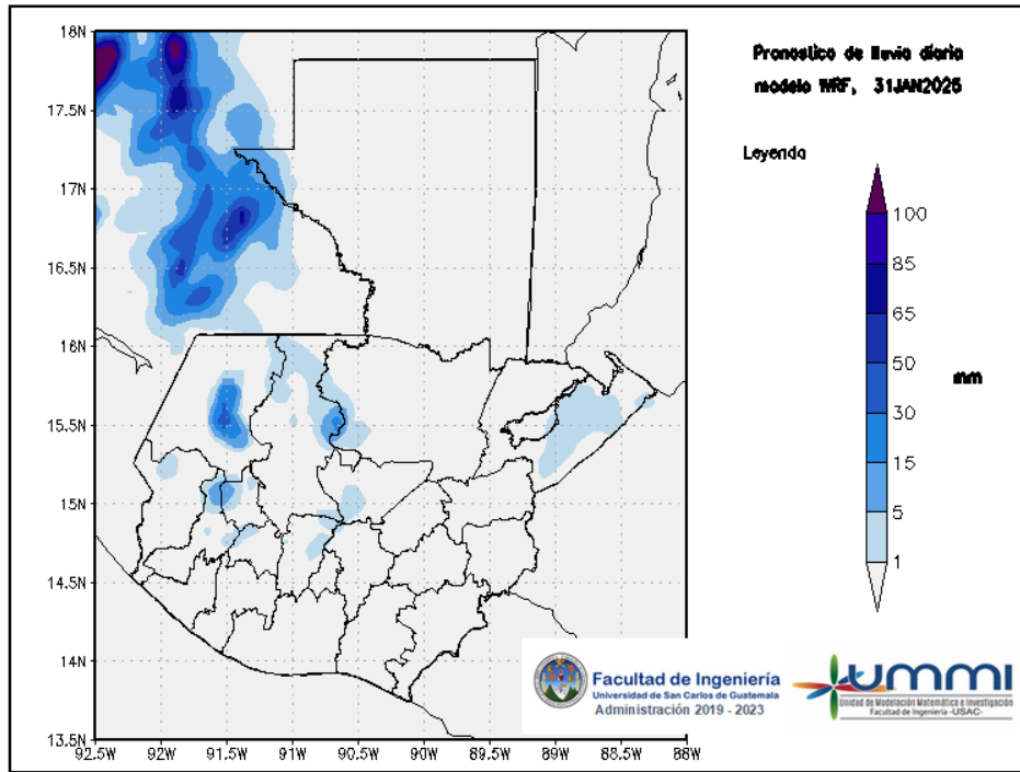
Figura 1: Pronóstico de lluvia diaria del 31 de January
