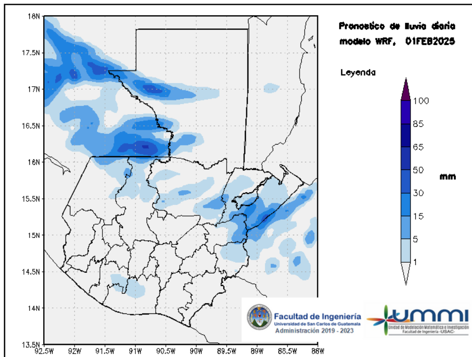
Figura 2: Pronóstico de lluvia diaria del 01 de February
