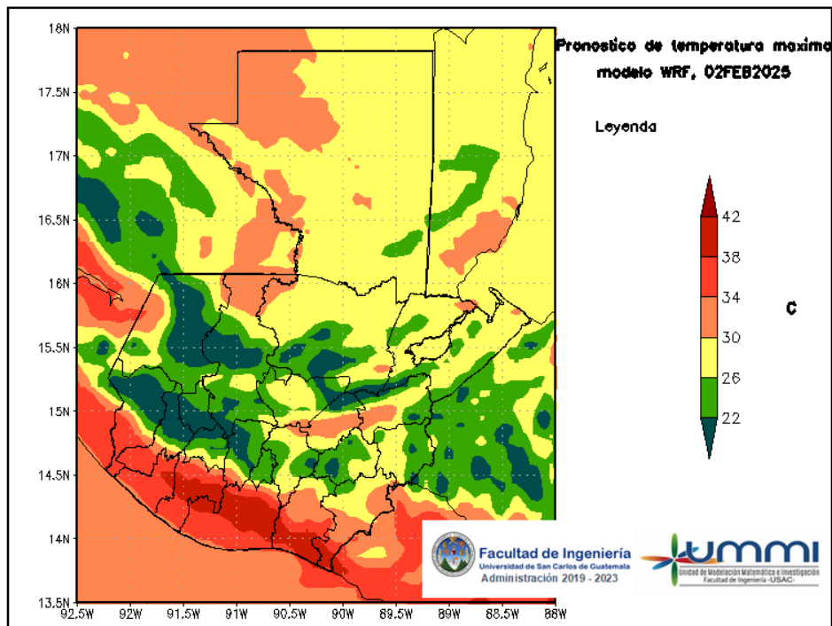
Figura 6: Pronóstico de temperatura máxima diaria del 02 de February
