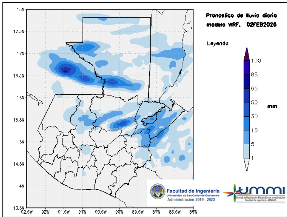
Figura 3: Pronóstico de lluvia diaria del 02 de February
