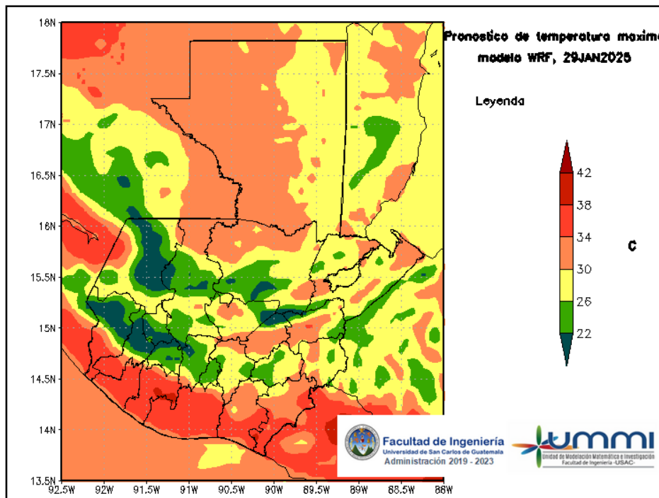
Figura 4: Pronóstico de temperatura máxima diaria del 29 de January
