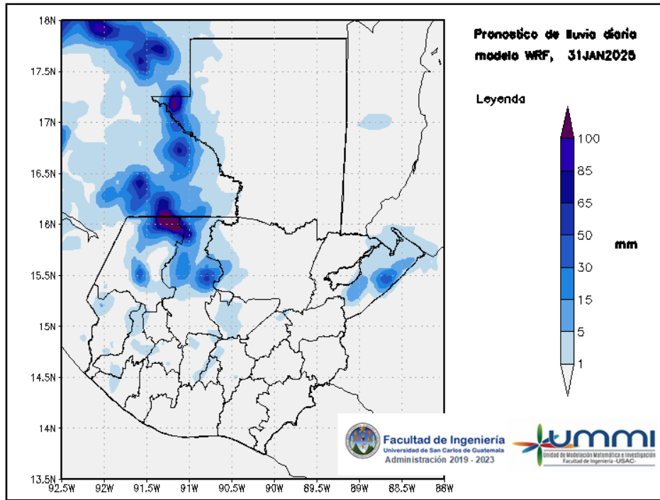
Figura 3: Pronóstico de lluvia diaria del 31 de January
