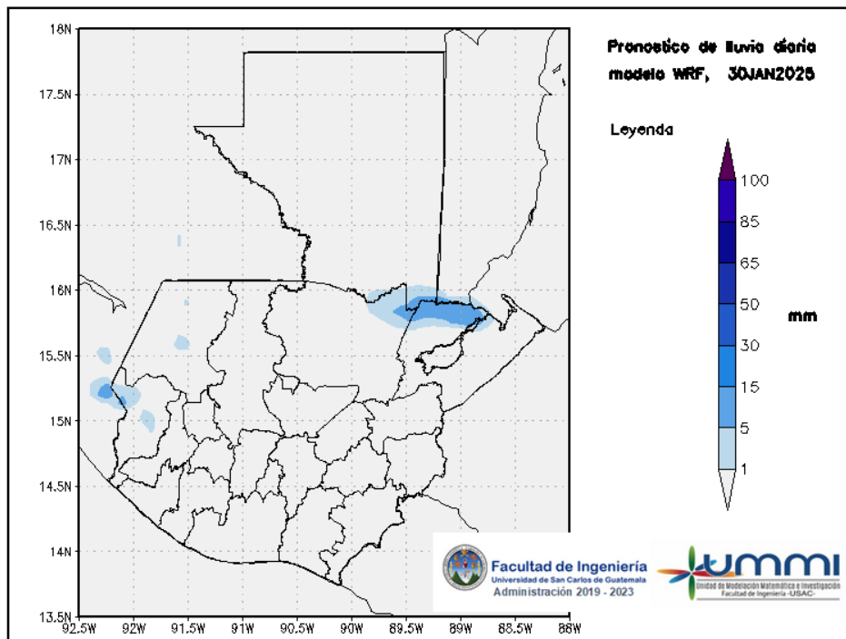
Figura 2: Pronóstico de lluvia diaria del 30 de January
