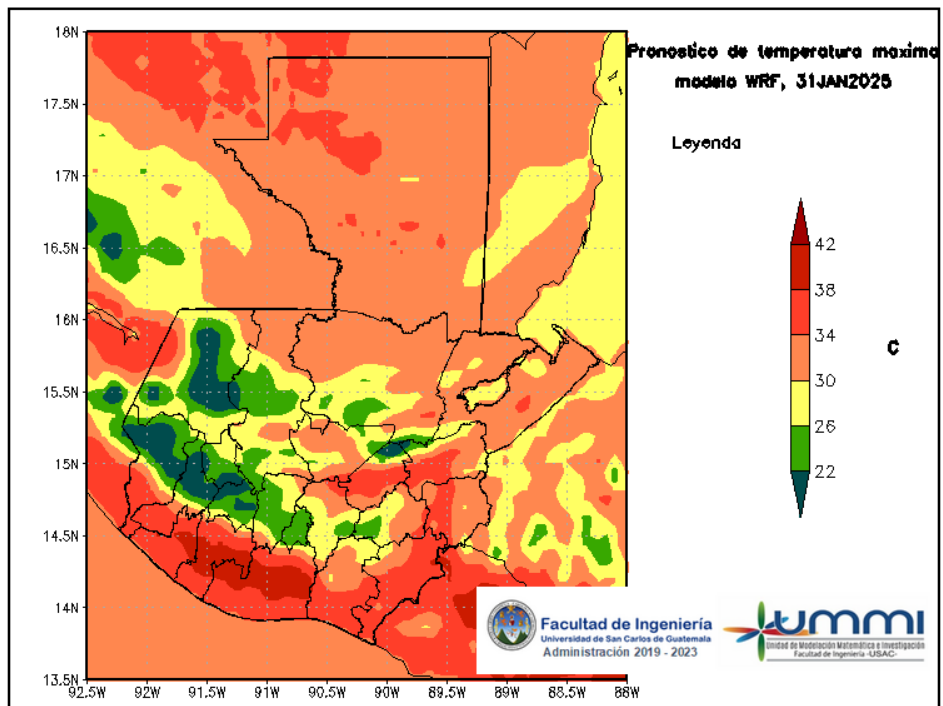
Figura 6: Pronóstico de temperatura máxima diaria del 31 de January
