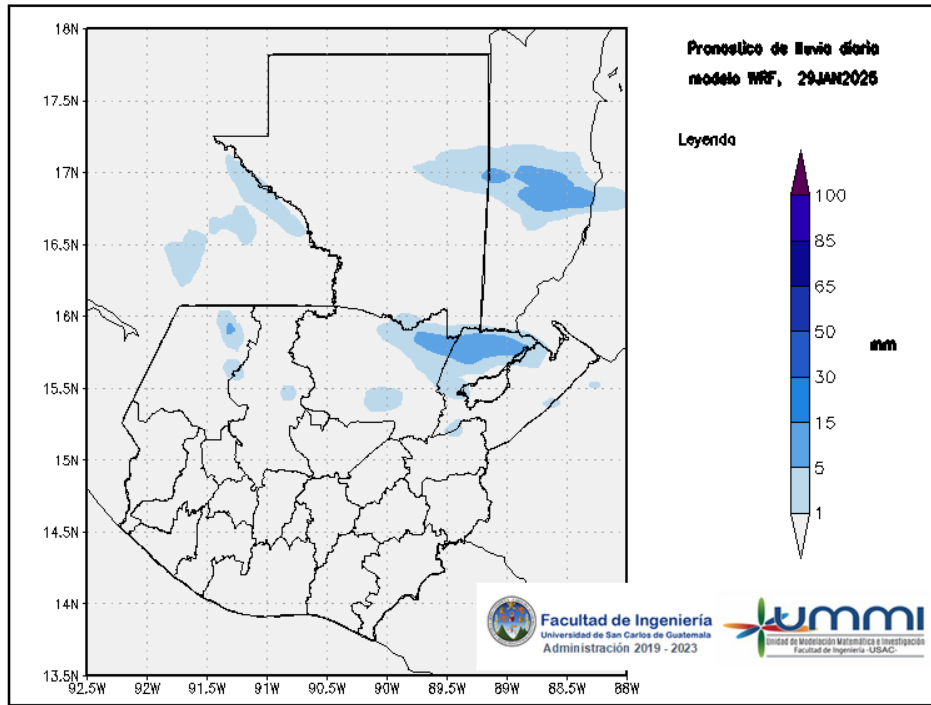
Figura 1: Pronóstico de lluvia diaria del 29 de January
