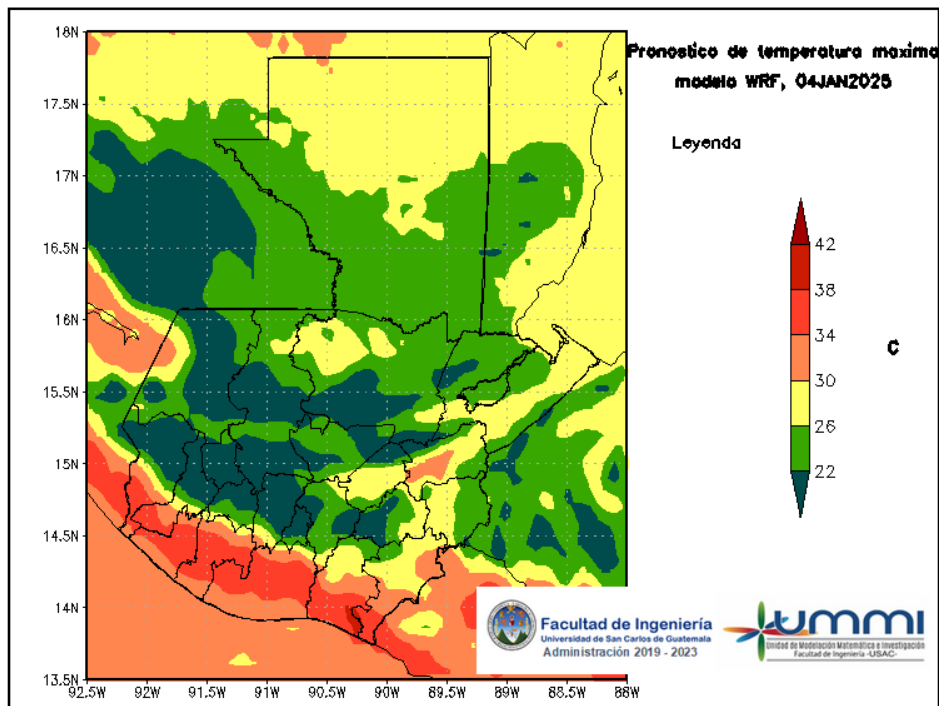
Figura 6: Pronóstico de temperatura máxima diaria del 04 de January
