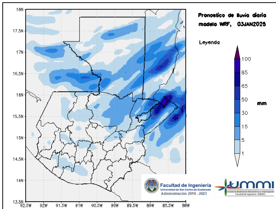
Figura 2: Pronóstico de lluvia diaria del 03 de January
