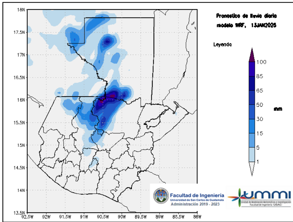
Figura 1: Pronóstico de lluvia diaria del 13 de January
