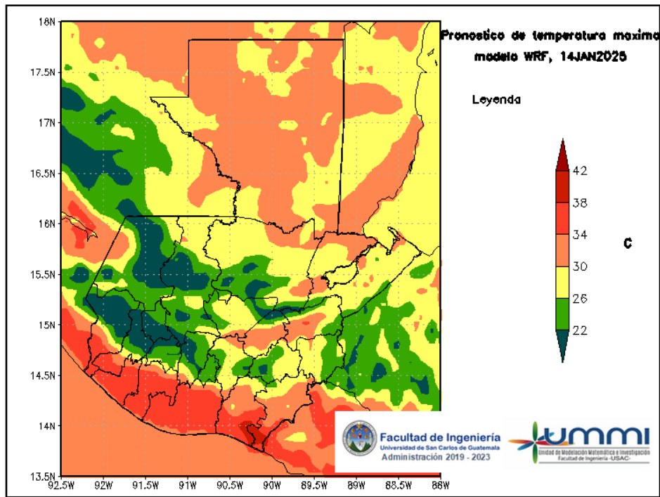
Figura 5: Pronóstico de temperatura máxima diaria del 14 de January
