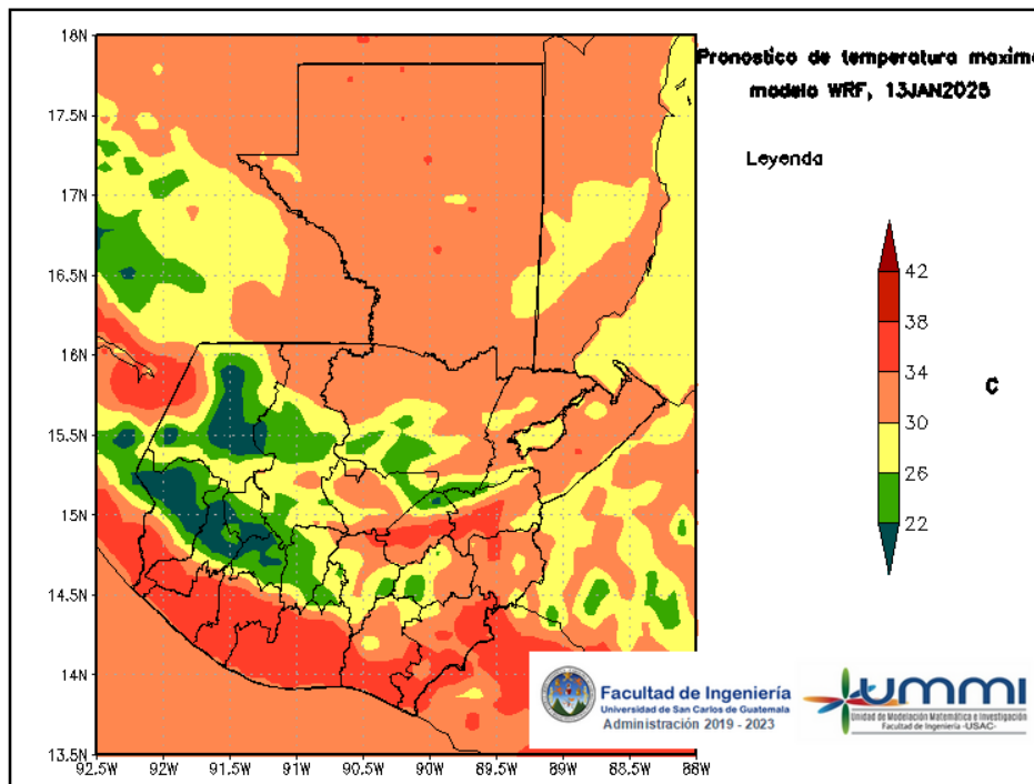
Figura 4: Pronóstico de temperatura máxima diaria del 13 de January
