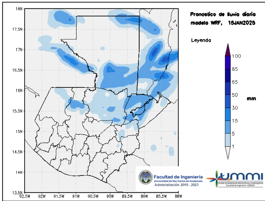
Figura 3: Pronóstico de lluvia diaria del 15 de January
