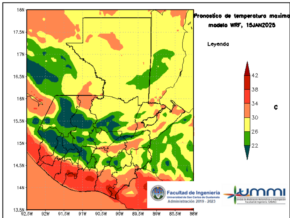
Figura 6: Pronóstico de temperatura máxima diaria del 15 de January
