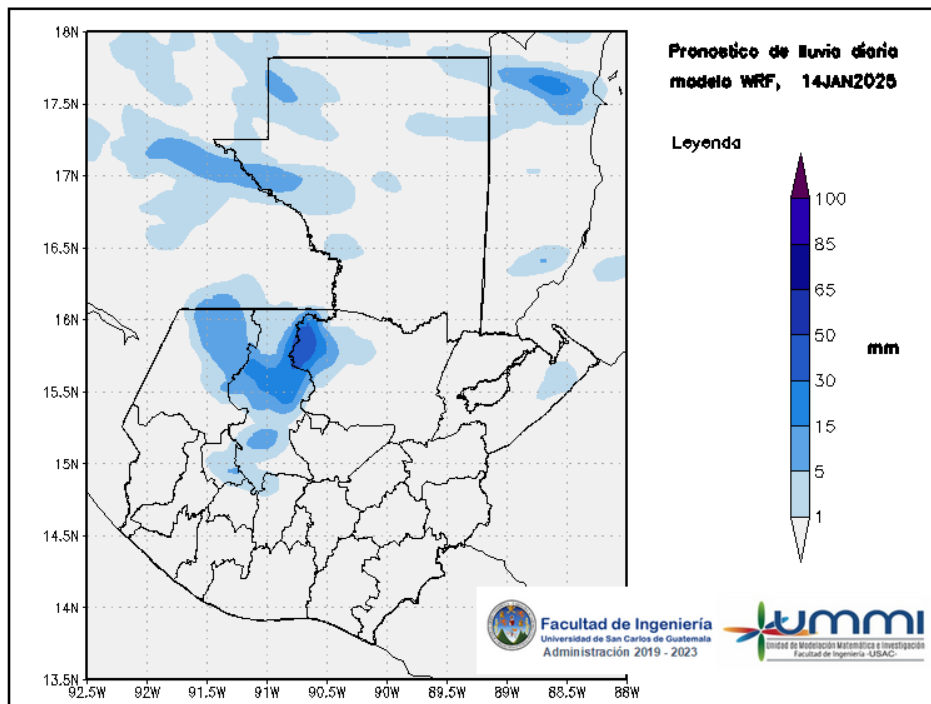
Figura 2: Pronóstico de lluvia diaria del 14 de January
