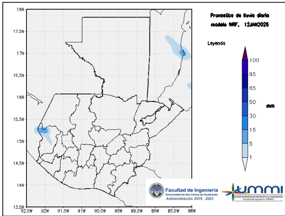
Figura 1: Pronóstico de lluvia diaria del 12 de January
