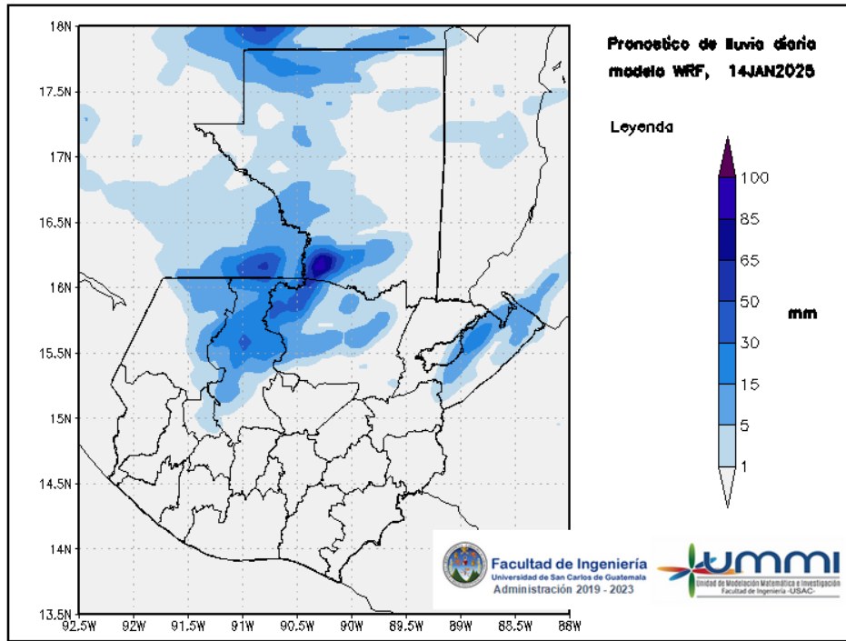
Figura 3: Pronóstico de lluvia diaria del 14 de January
