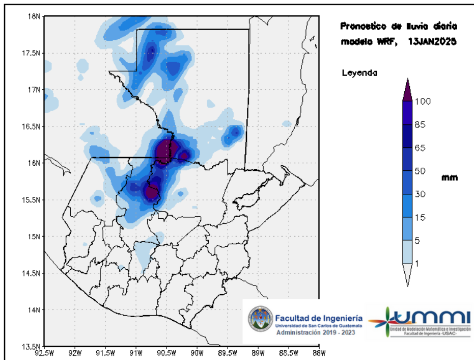
Figura 2: Pronóstico de lluvia diaria del 13 de January
