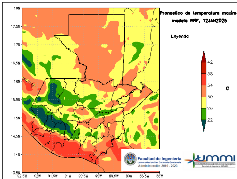
Figura 4: Pronóstico de temperatura máxima diaria del 12 de January
