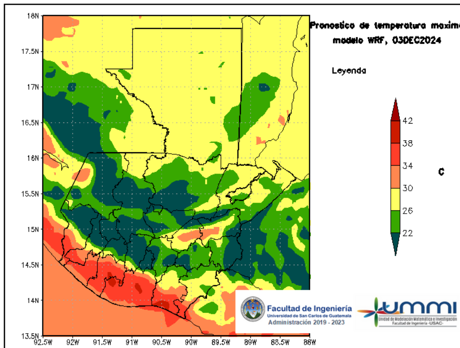
Figura 4: Pronóstico de temperatura máxima diaria del 03 de December
