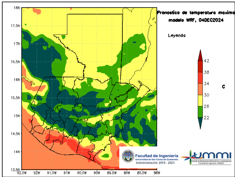
Figura 5: Pronóstico de temperatura máxima diaria del 04 de December
