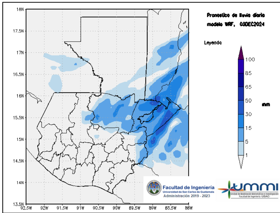
Figura 1: Pronóstico de lluvia diaria del 03 de December
