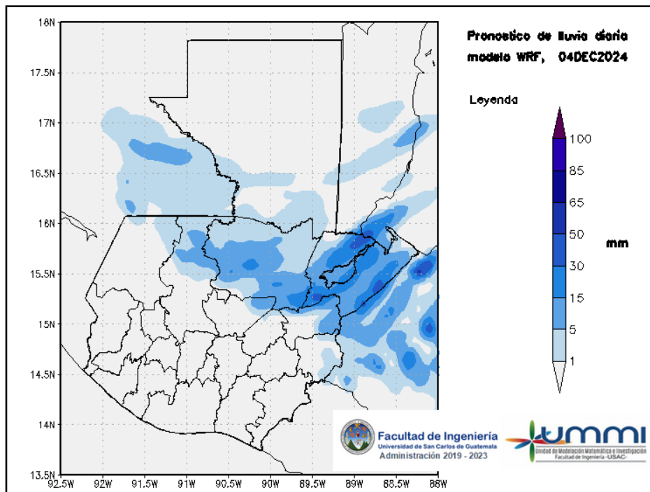
Figura 2: Pronóstico de lluvia diaria del 04 de December
