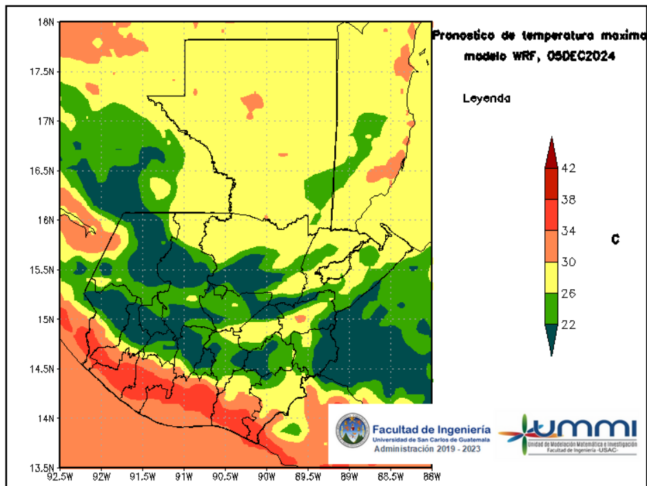
Figura 6: Pronóstico de temperatura máxima diaria del 05 de December
