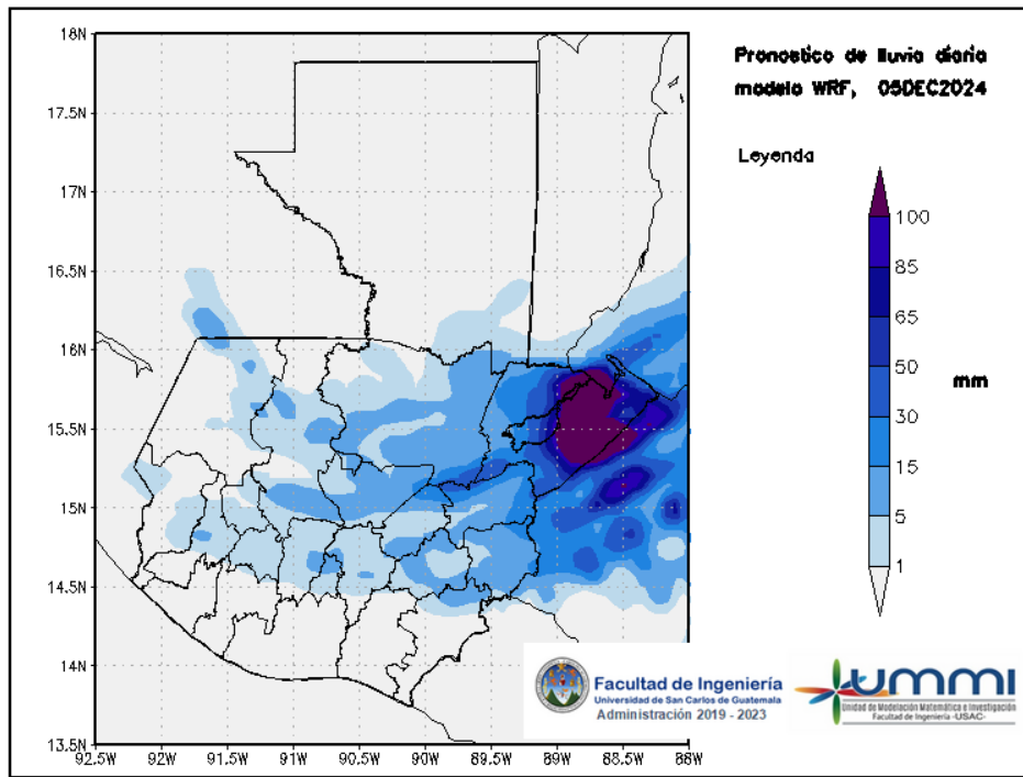
Figura 3: Pronóstico de lluvia diaria del 05 de December
