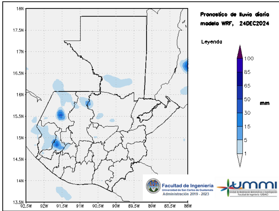
Figura 3: Pronóstico de lluvia diaria del 24 de December
