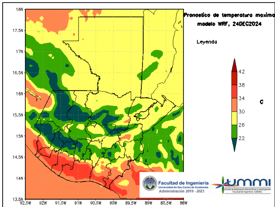
Figura 6: Pronóstico de temperatura máxima diaria del 24 de December
