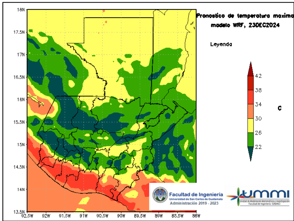
Figura 5: Pronóstico de temperatura máxima diaria del 23 de December
