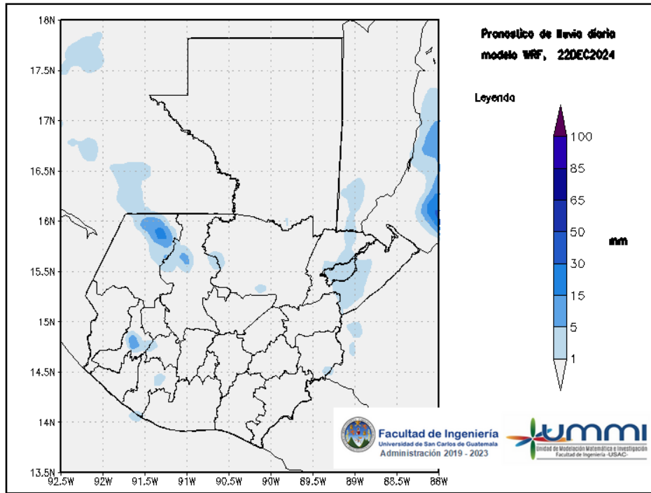
Figura 1: Pronóstico de lluvia diaria del 22 de December
