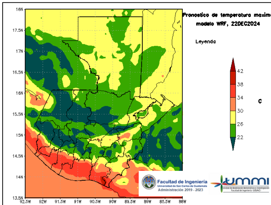
Figura 4: Pronóstico de temperatura máxima diaria del 22 de December
