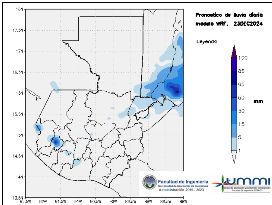
Figura 2: Pronóstico de lluvia diaria del 23 de December
