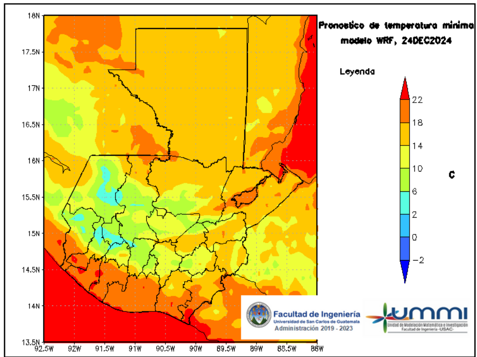
Figura 9: Pronóstico de temperatura mínima diaria del 25 de December
