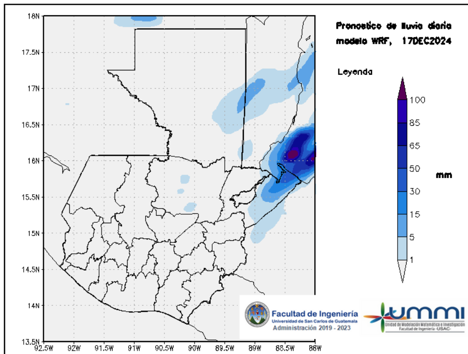
Figura 2: Pronóstico de lluvia diaria del 17 de December
