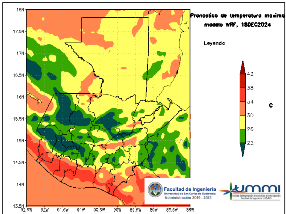
Figura 6: Pronóstico de temperatura máxima diaria del 18 de December
