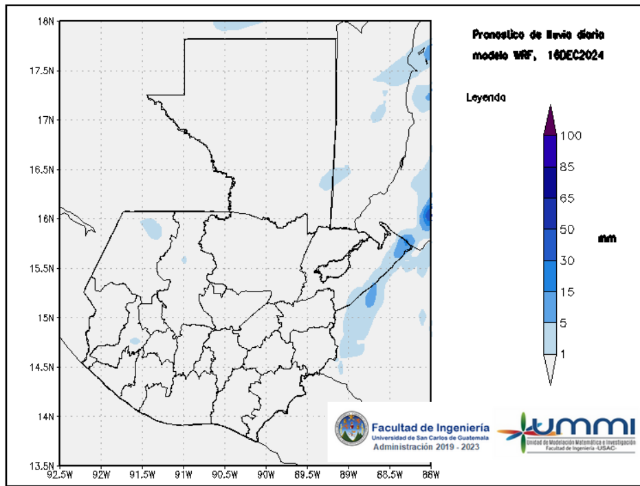
Figura 1: Pronóstico de lluvia diaria del 16 de December
