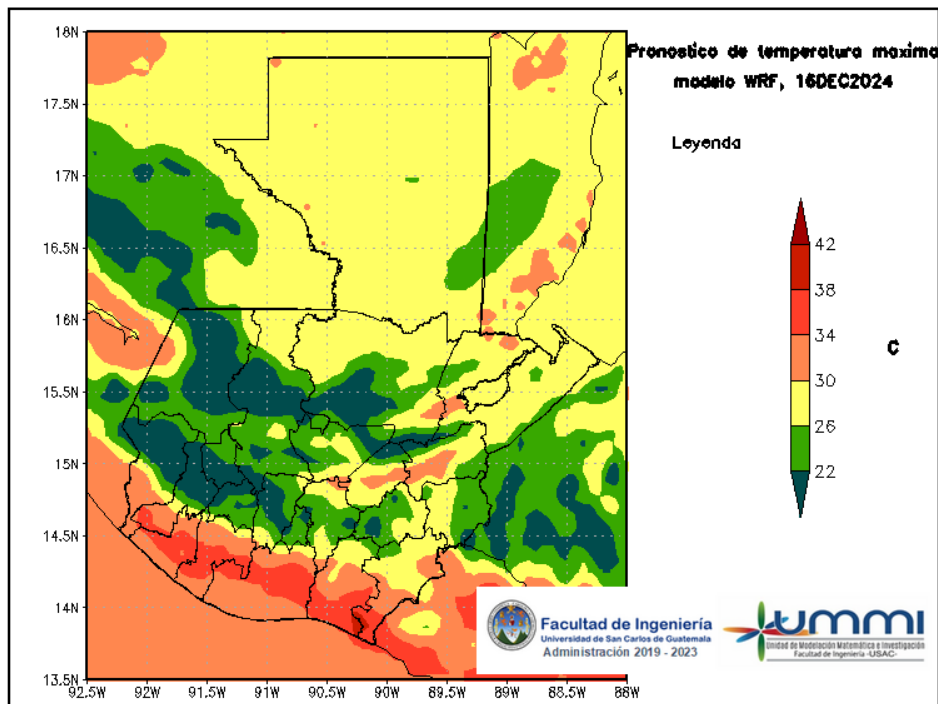
Figura 4: Pronóstico de temperatura máxima diaria del 16 de December
