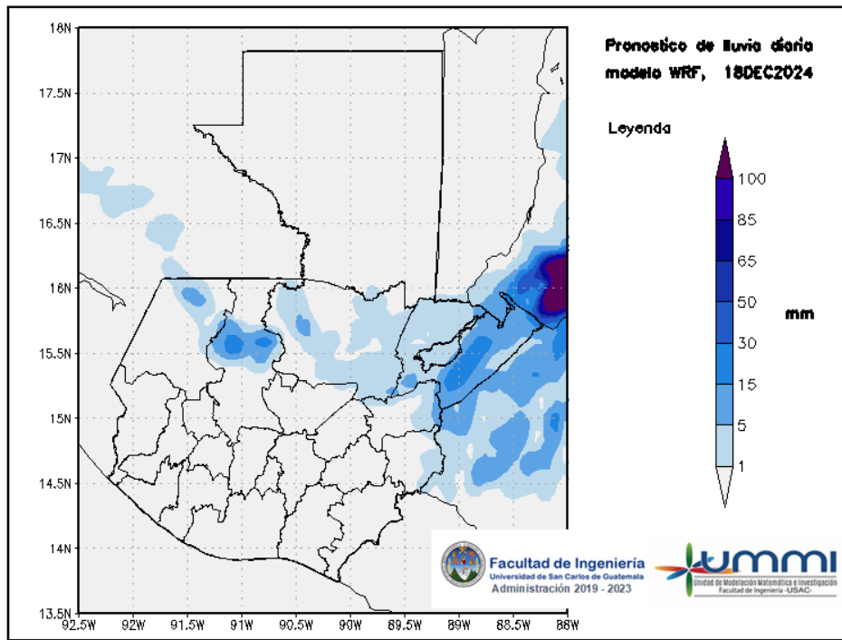
Figura 3: Pronóstico de lluvia diaria del 18 de December
