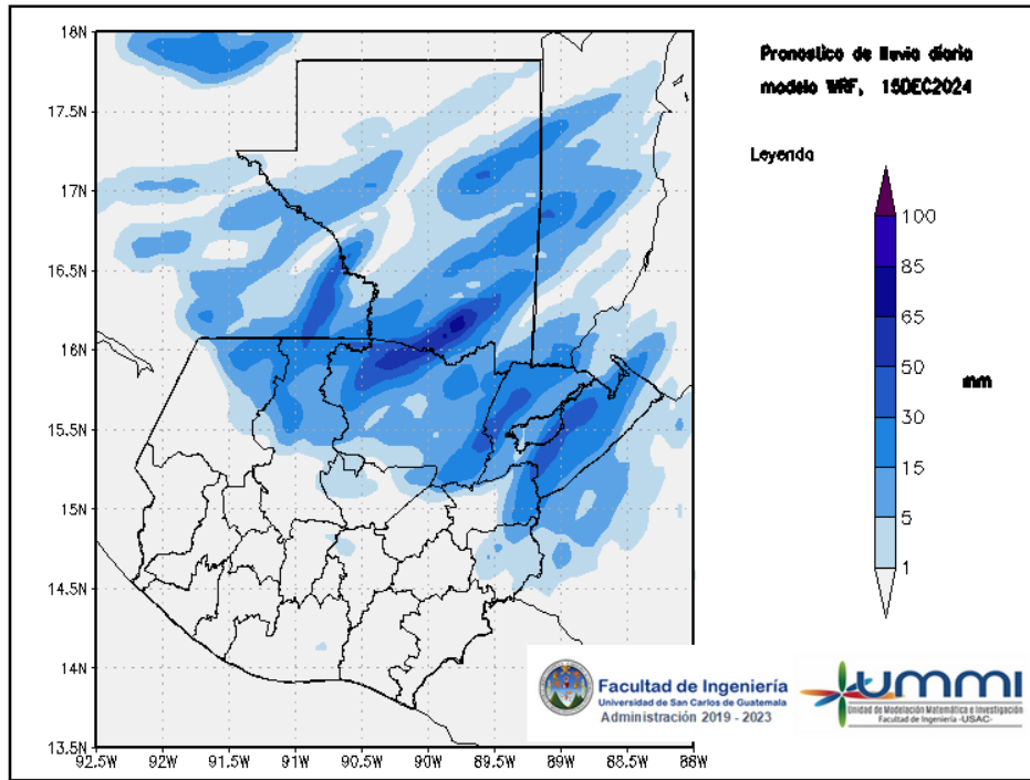
Figura 1: Pronóstico de lluvia diaria del 15 de December
