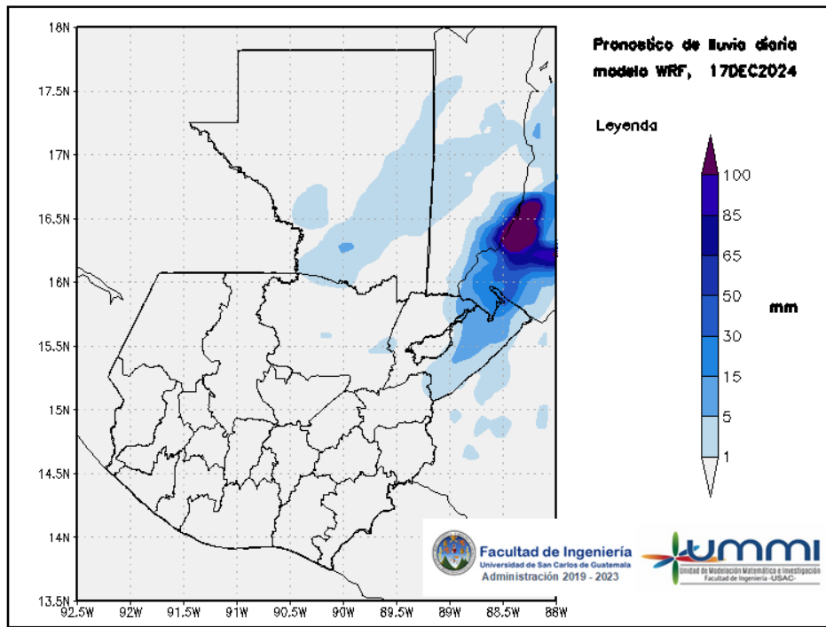
Figura 3: Pronóstico de lluvia diaria del 17 de December
