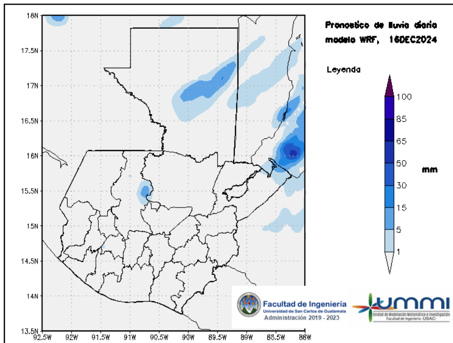
Figura 2: Pronóstico de lluvia diaria del 16 de December
