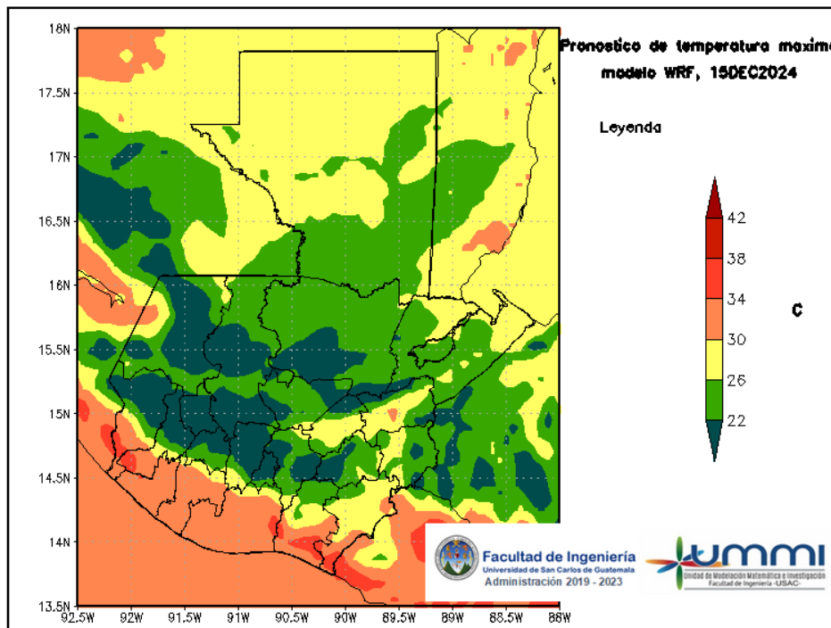
Figura 4: Pronóstico de temperatura máxima diaria del 15 de December
