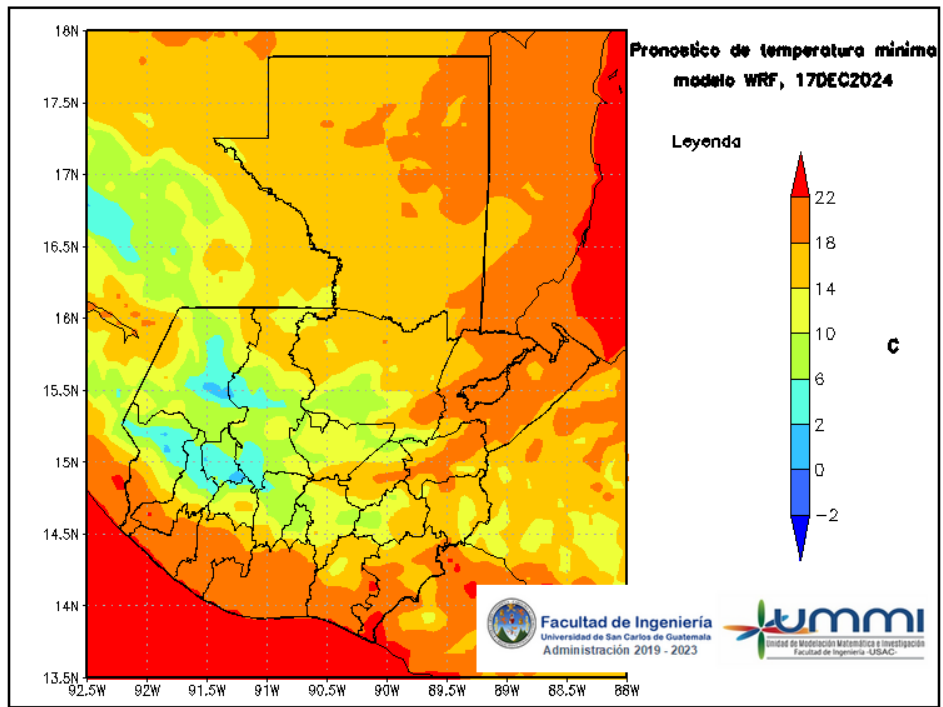
Figura 9: Pronóstico de temperatura mínima diaria del 18 de December
