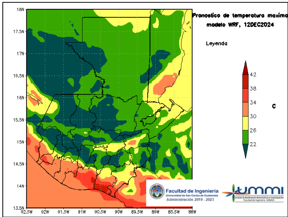
Figura 5: Pronóstico de temperatura máxima diaria del 12 de December
