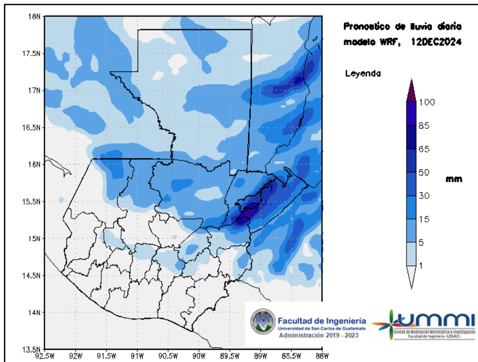
Figura 2: Pronóstico de lluvia diaria del 12 de December
