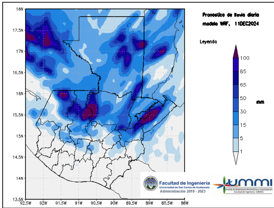
Figura 1: Pronóstico de lluvia diaria del 11 de December
