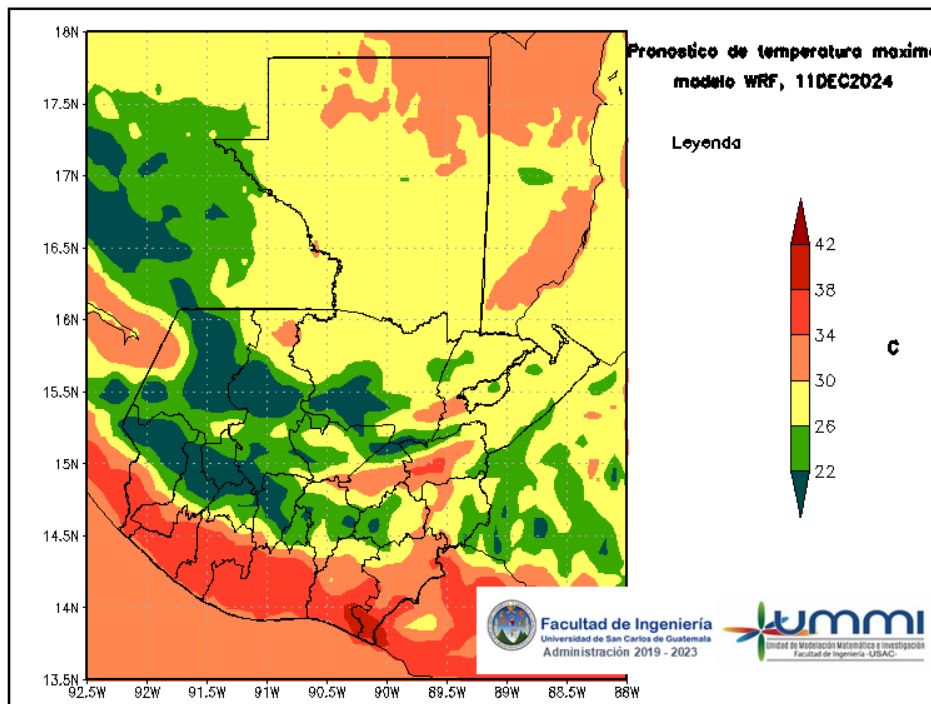
Figura 4: Pronóstico de temperatura máxima diaria del 11 de December
