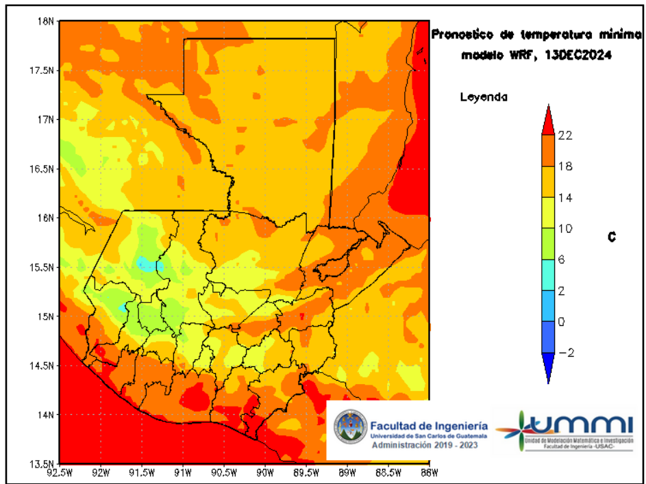
Figura 9: Pronóstico de temperatura mínima diaria del 14 de December
