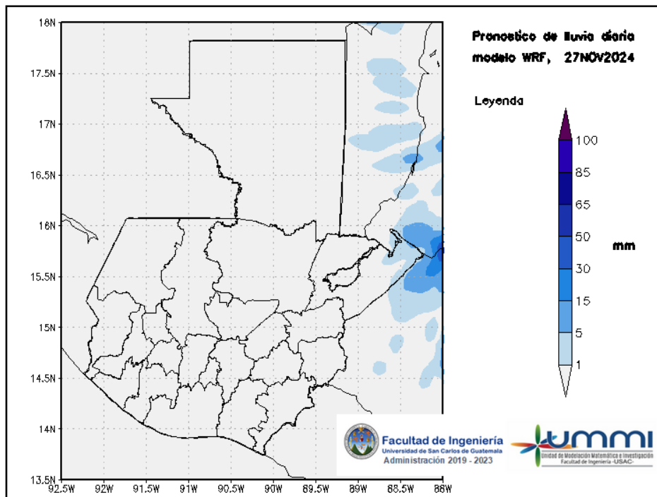
Figura 2: Pronóstico de lluvia diaria del 27 de November
