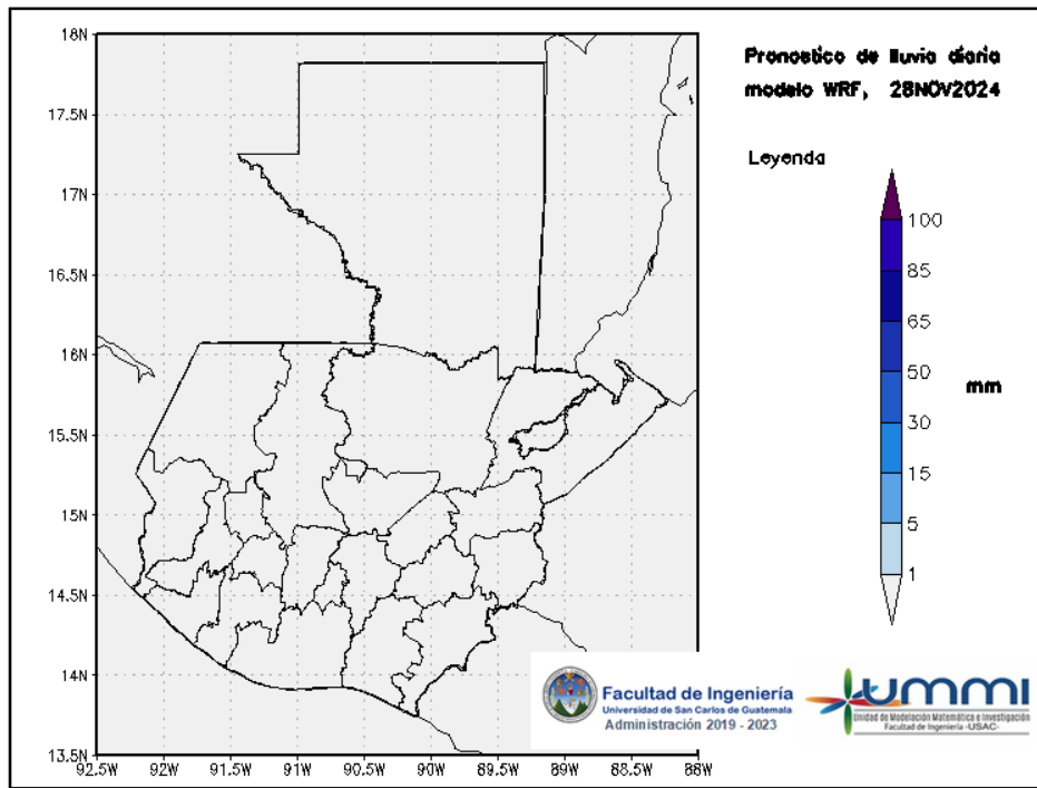
Figura 3: Pronóstico de lluvia diaria del 28 de November
