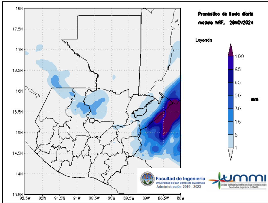
Figura 1: Pronóstico de lluvia diaria del 26 de November
