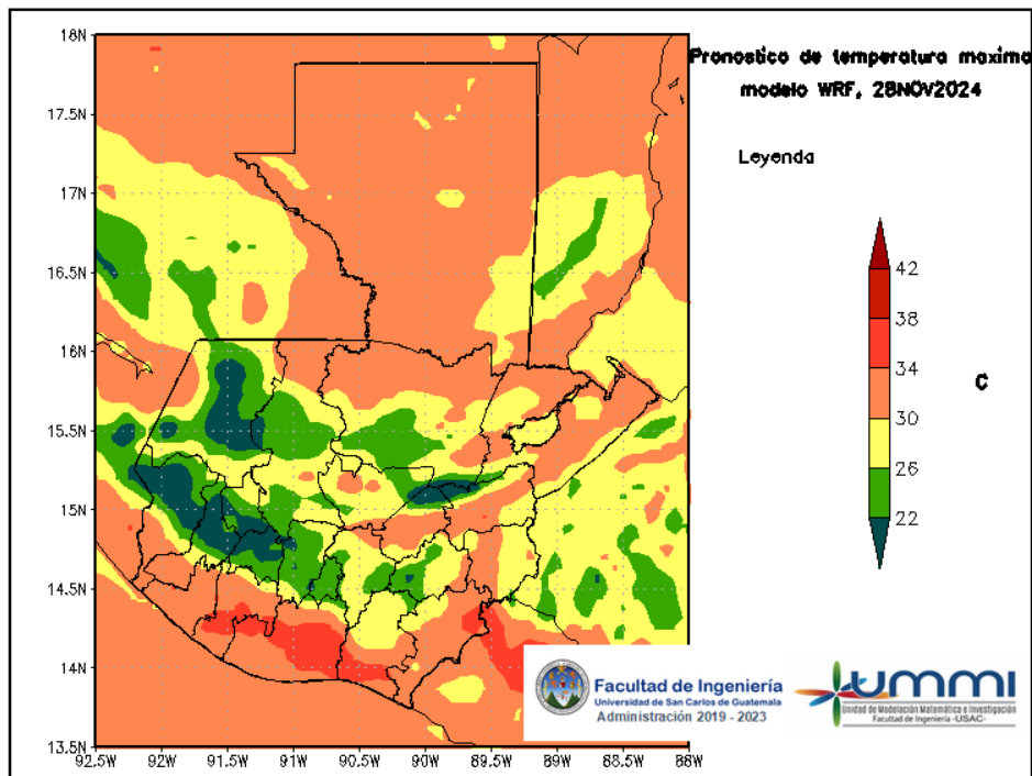
Figura 6: Pronóstico de temperatura máxima diaria del 28 de November
