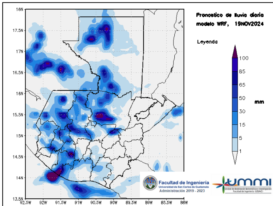
Figura 2: Pronóstico de lluvia diaria del 19 de November
