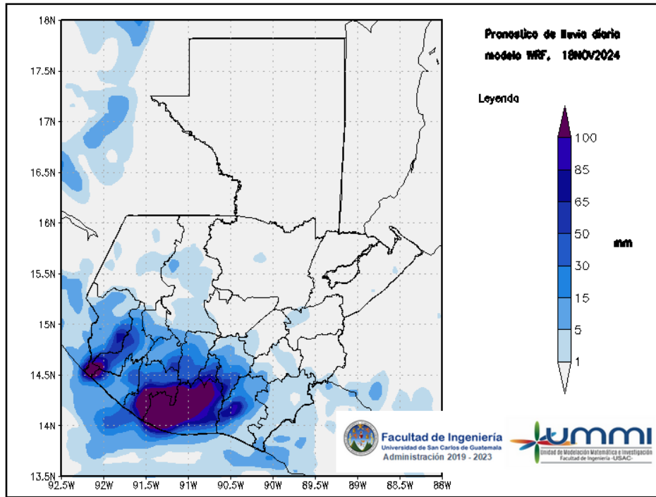
Figura 1: Pronóstico de lluvia diaria del 18 de November
