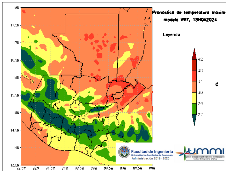
Figura 4: Pronóstico de temperatura máxima diaria del 18 de November
