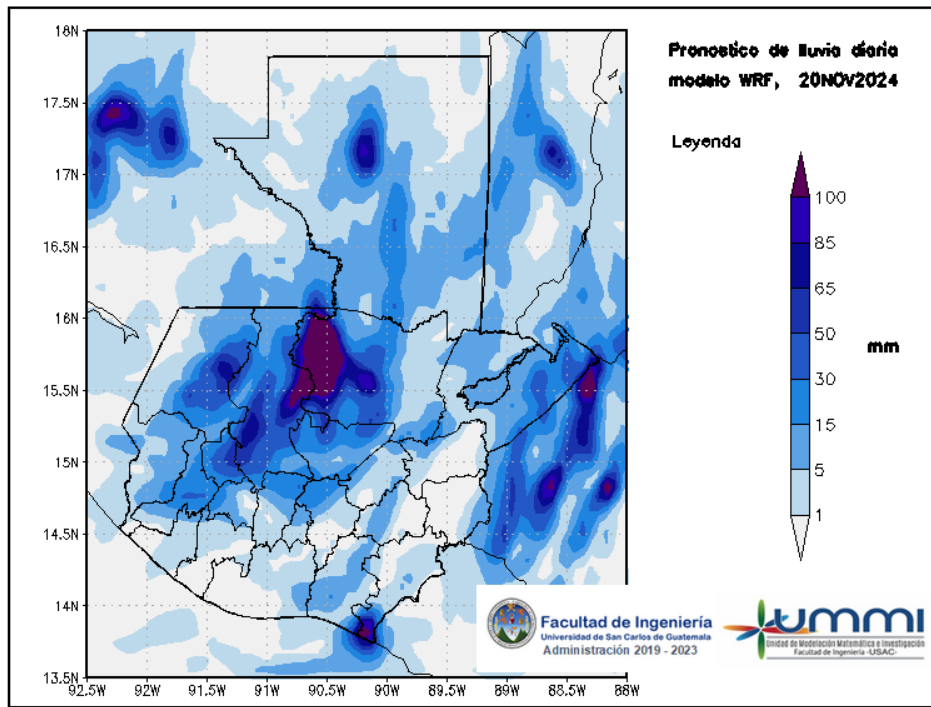
Figura 3: Pronóstico de lluvia diaria del 20 de November
