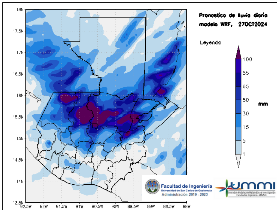
Figura 2: Pronóstico de lluvia diaria del 27 de October
