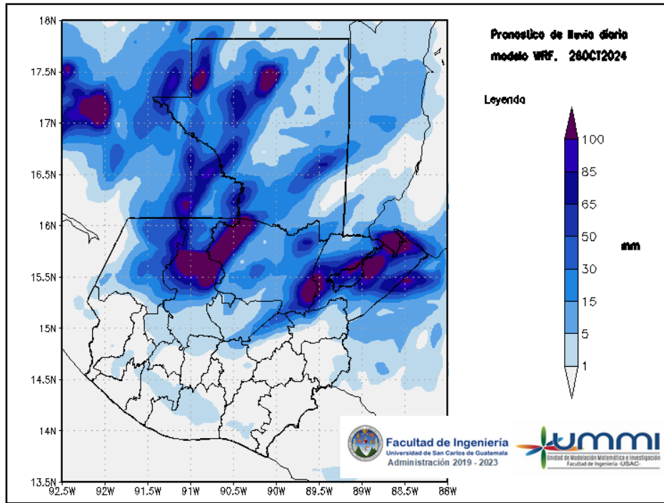
Figura 1: Pronóstico de lluvia diaria del 26 de October
