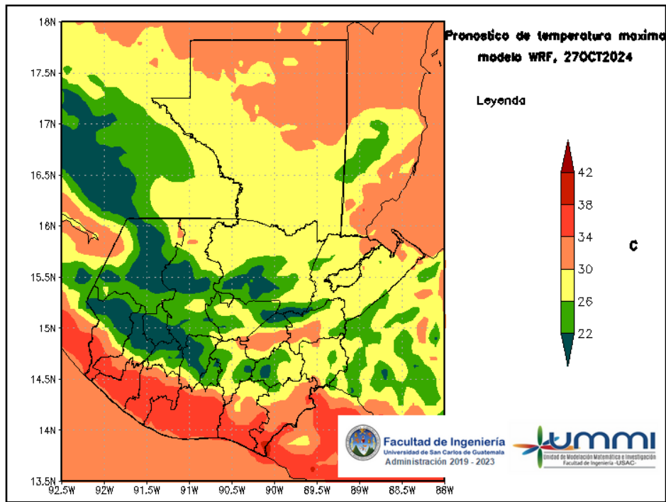
Figura 5: Pronóstico de temperatura máxima diaria del 27 de October
