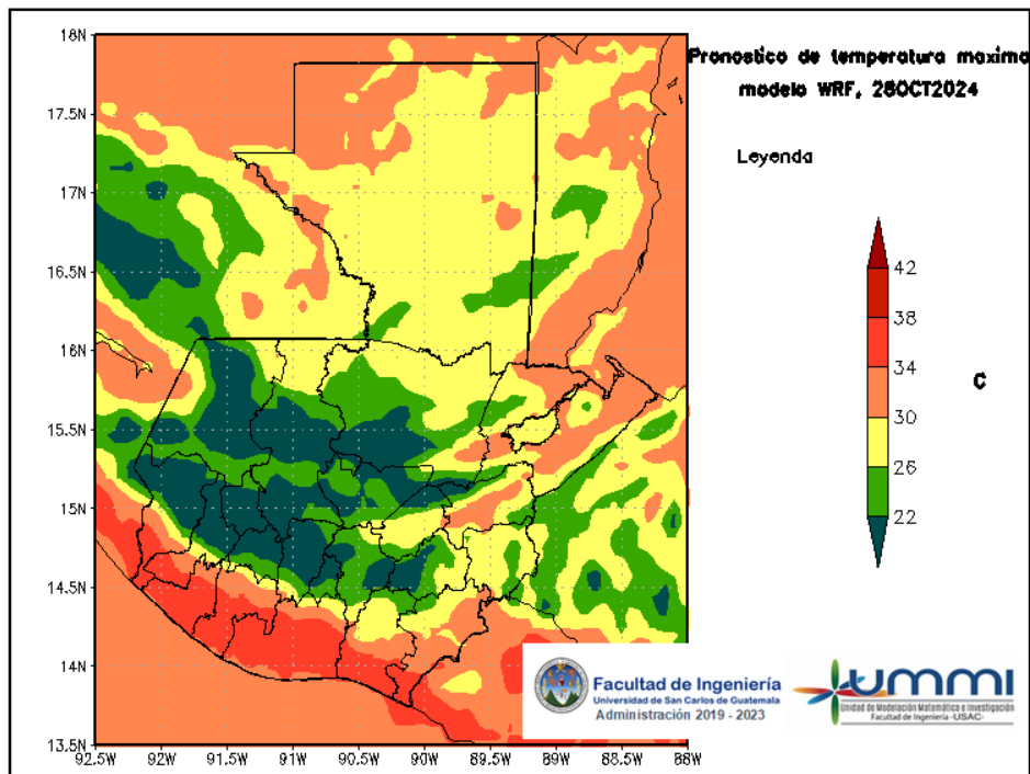
Figura 6: Pronóstico de temperatura máxima diaria del 28 de October
