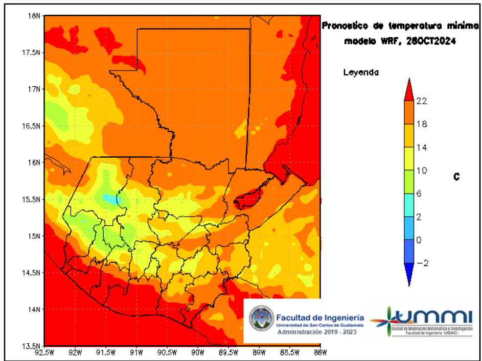
Figura 9: Pronóstico de temperatura mínima diaria del 29 de October
