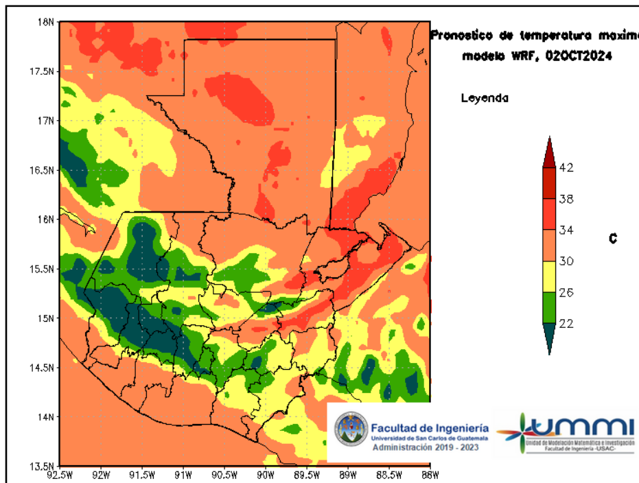
Figura 4: Pronóstico de temperatura máxima diaria del 02 de October
