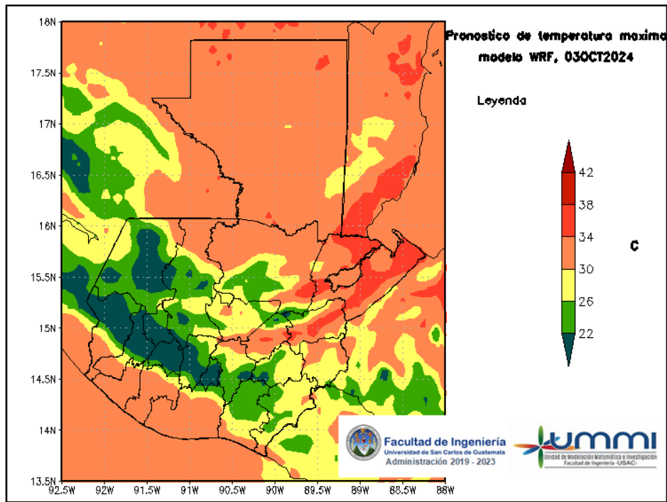
Figura 5: Pronóstico de temperatura máxima diaria del 03 de October
