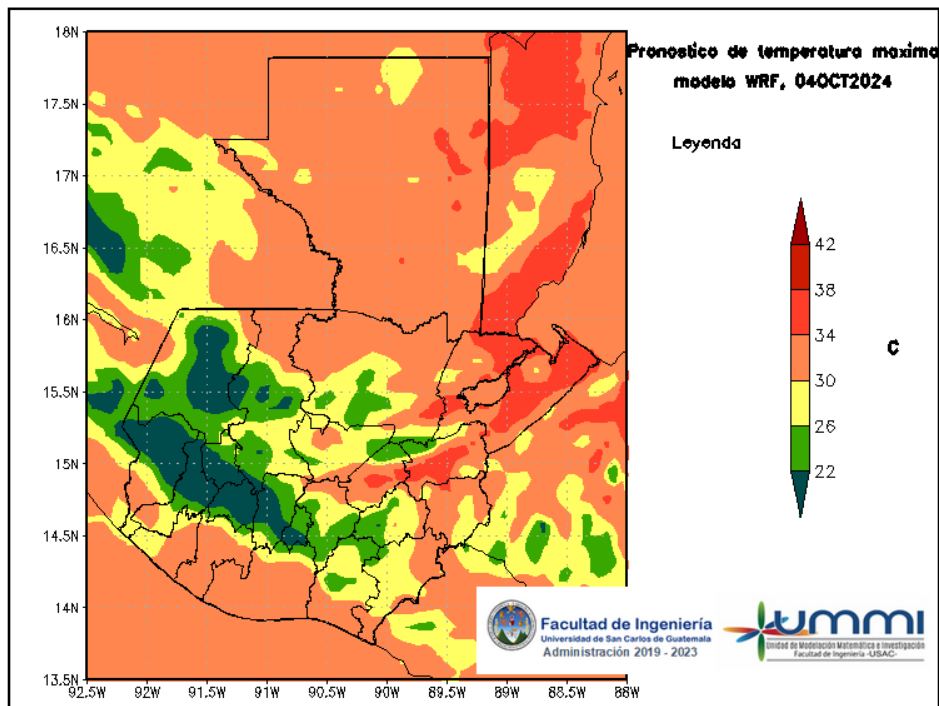
Figura 6: Pronóstico de temperatura máxima diaria del 04 de October
