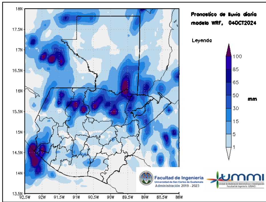
Figura 3: Pronóstico de lluvia diaria del 04 de October
