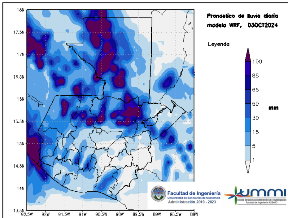
Figura 2: Pronóstico de lluvia diaria del 03 de October
