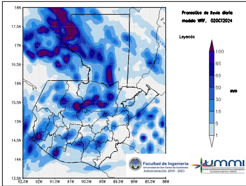
Figura 1: Pronóstico de lluvia diaria del 02 de October
