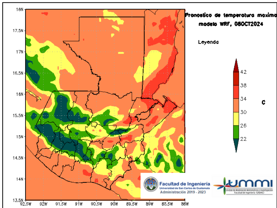
Figura 6: Pronóstico de temperatura máxima diaria del 08 de October
