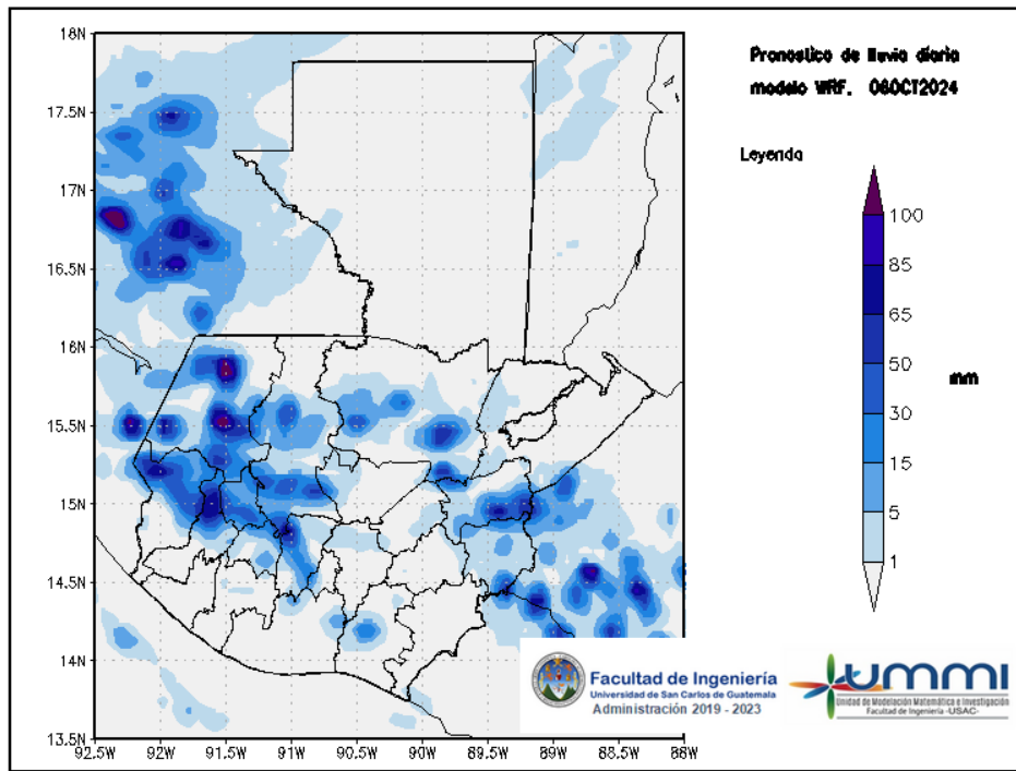
Figura 1: Pronóstico de lluvia diaria del 06 de October
