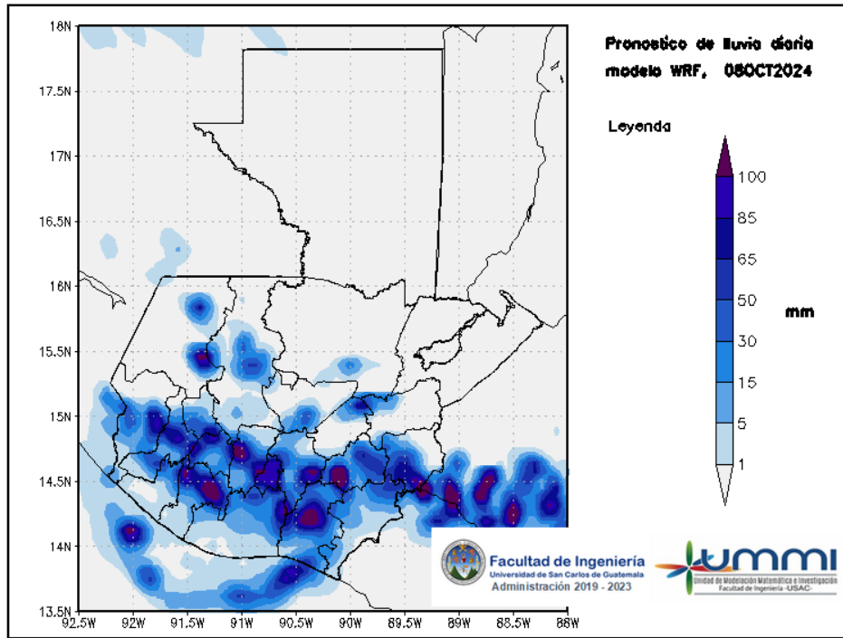
Figura 3: Pronóstico de lluvia diaria del 08 de October
