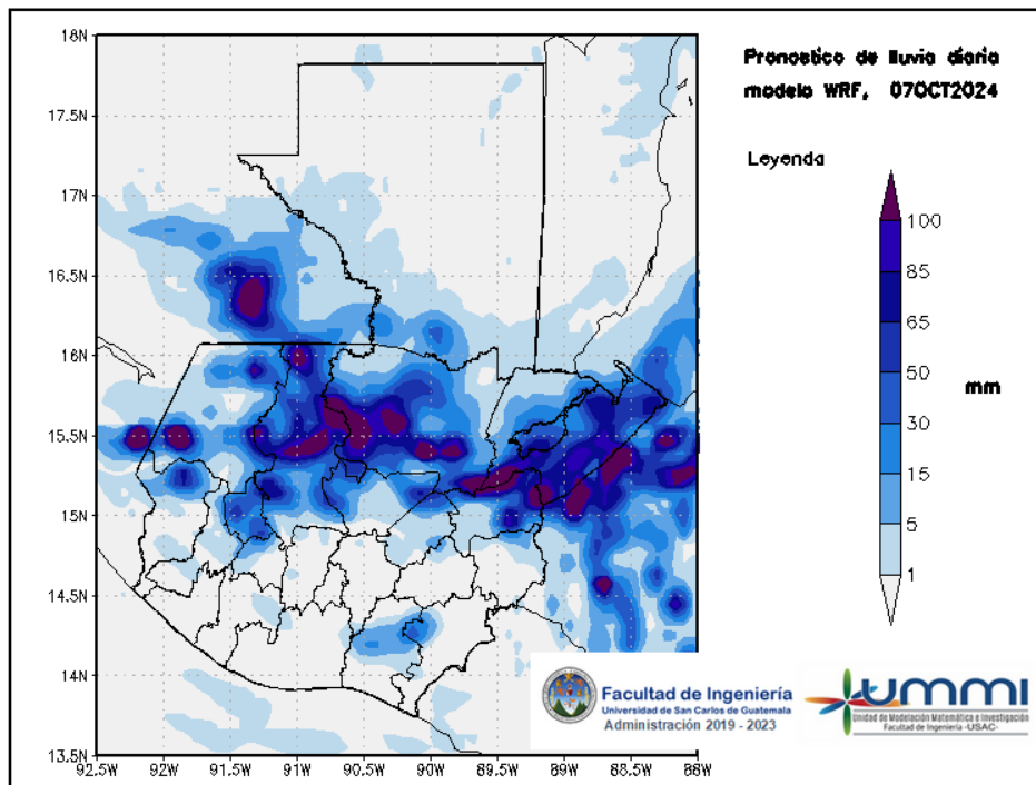
Figura 2: Pronóstico de lluvia diaria del 07 de October
