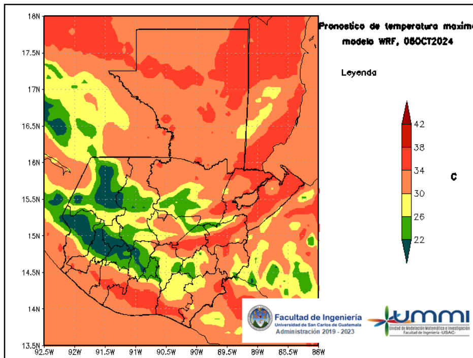
Figura 4: Pronóstico de temperatura máxima diaria del 06 de October
