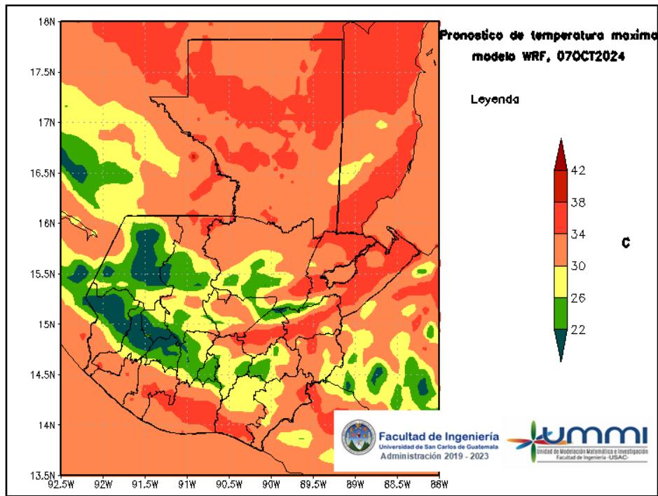
Figura 5: Pronóstico de temperatura máxima diaria del 07 de October
