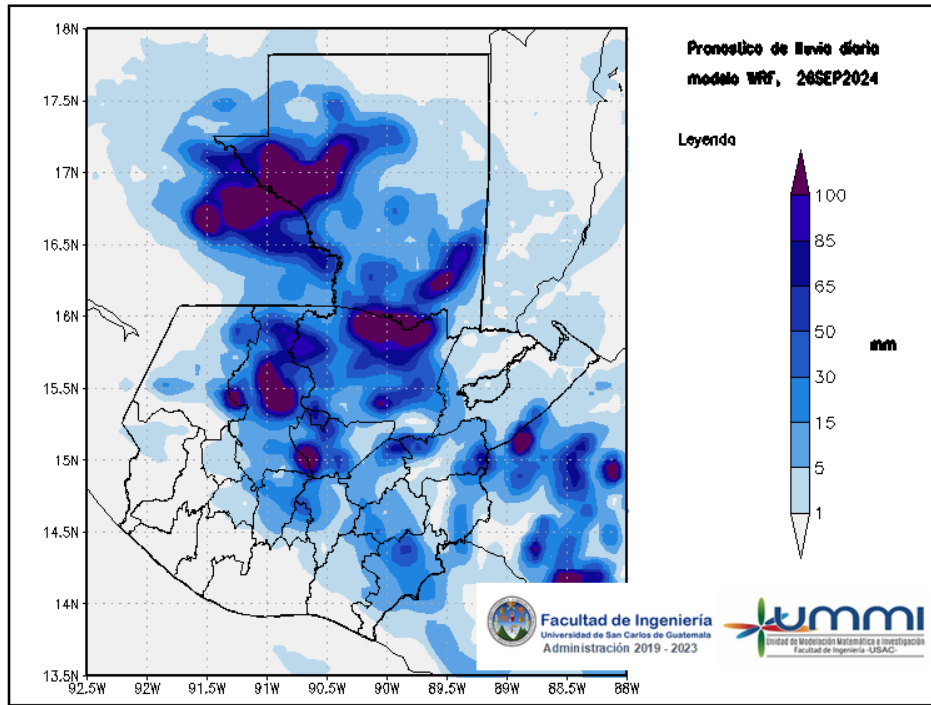
Figura 1: Pronóstico de lluvia diaria del 26 de September
