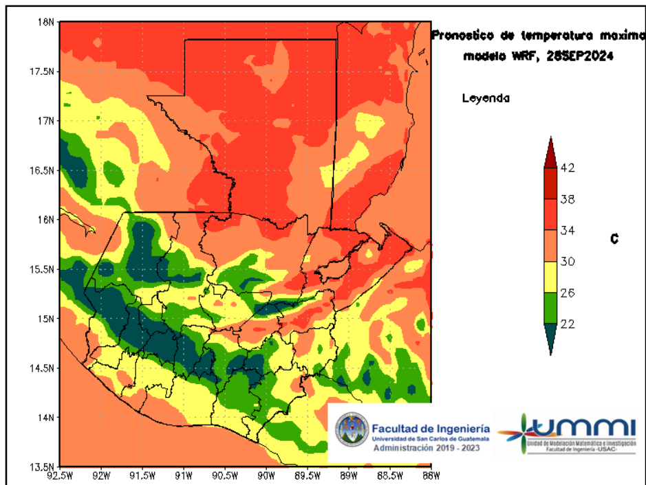
Figura 6: Pronóstico de temperatura máxima diaria del 28 de September
