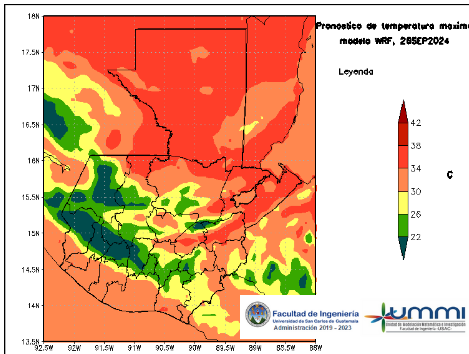
Figura 4: Pronóstico de temperatura máxima diaria del 26 de September
