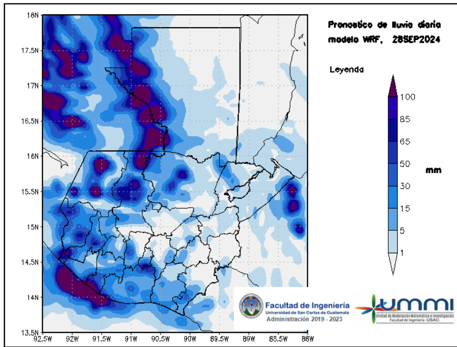
Figura 3: Pronóstico de lluvia diaria del 28 de September
