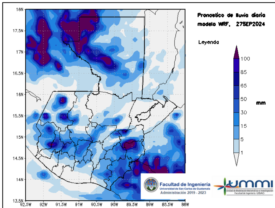
Figura 2: Pronóstico de lluvia diaria del 27 de September
