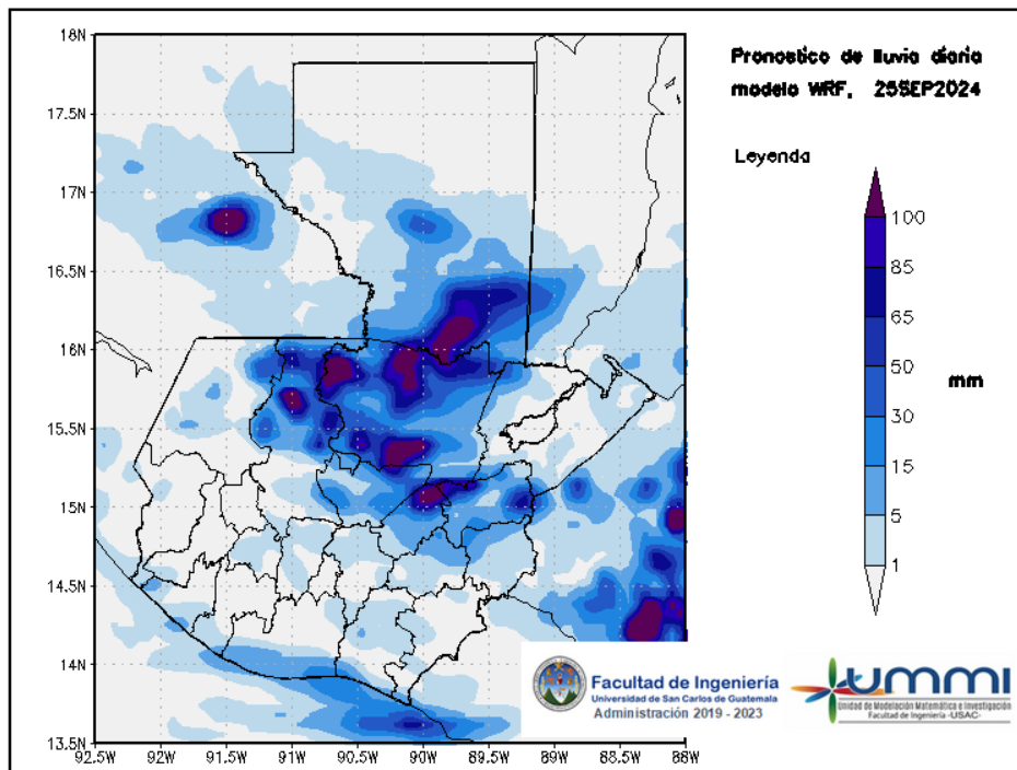
Figura 2: Pronóstico de lluvia diaria del 25 de September
