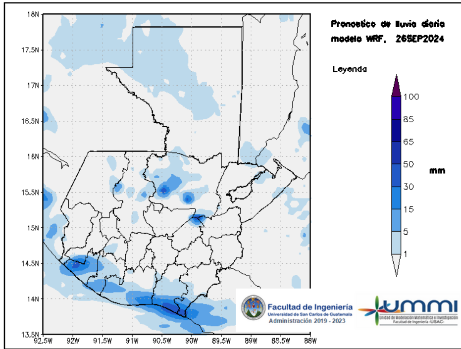
Figura 3: Pronóstico de lluvia diaria del 26 de September
