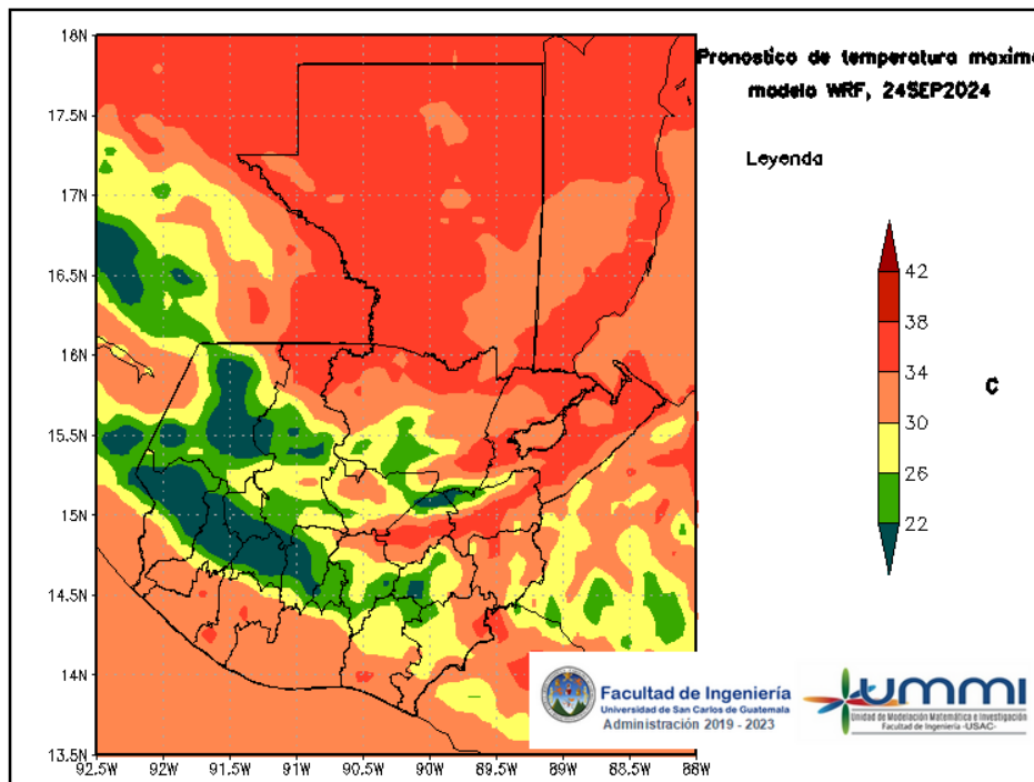
Figura 4: Pronóstico de temperatura máxima diaria del 24 de September
