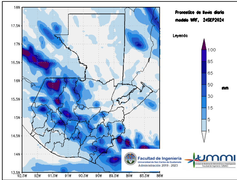
Figura 1: Pronóstico de lluvia diaria del 24 de September
