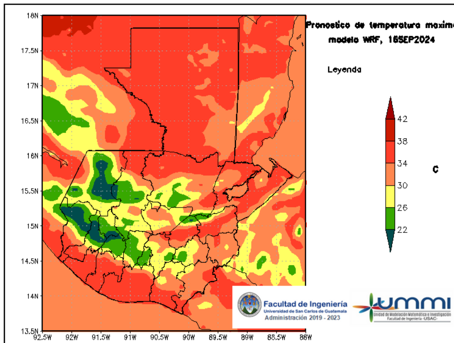
Figura 4: Pronóstico de temperatura máxima diaria del 16 de September
