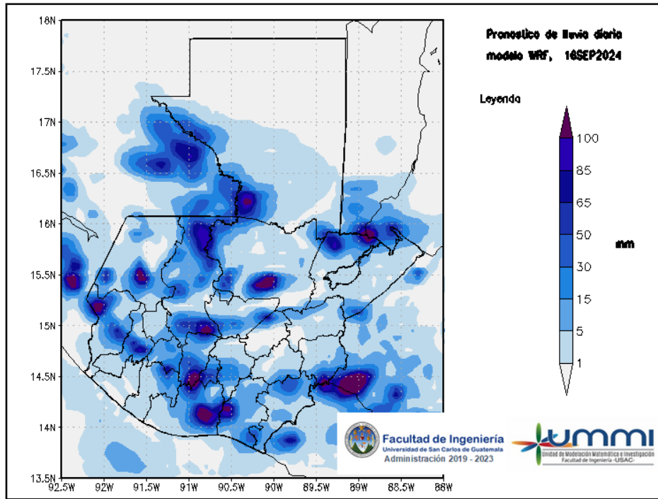
Figura 1: Pronóstico de lluvia diaria del 16 de September
