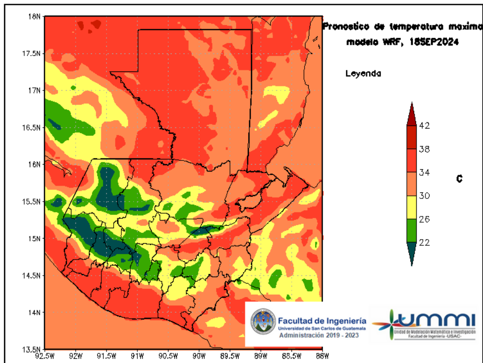
Figura 6: Pronóstico de temperatura máxima diaria del 18 de September
