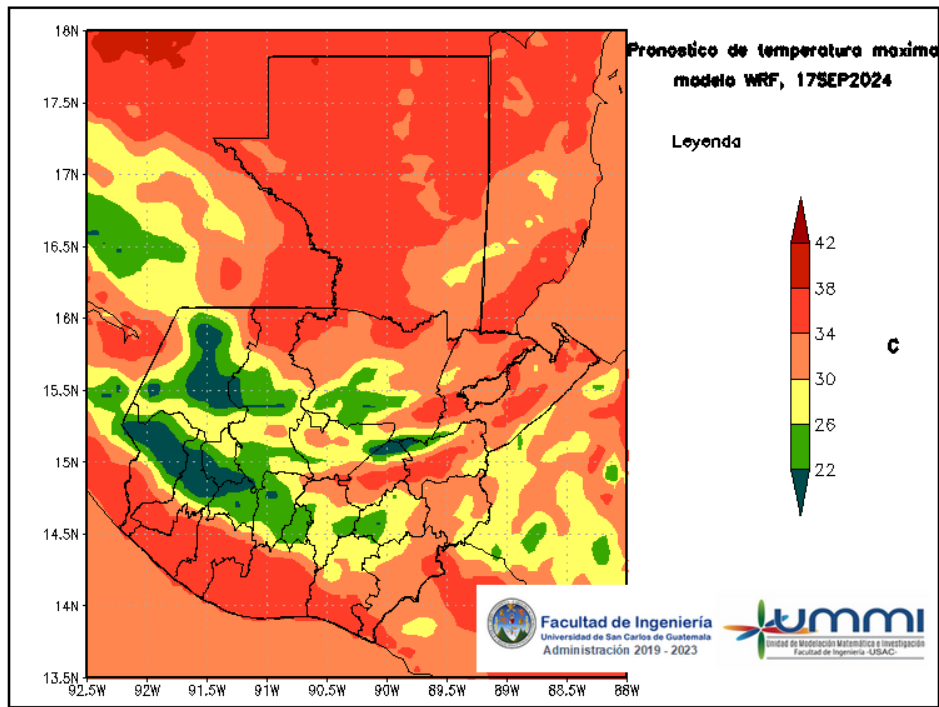
Figura 5: Pronóstico de temperatura máxima diaria del 17 de September
