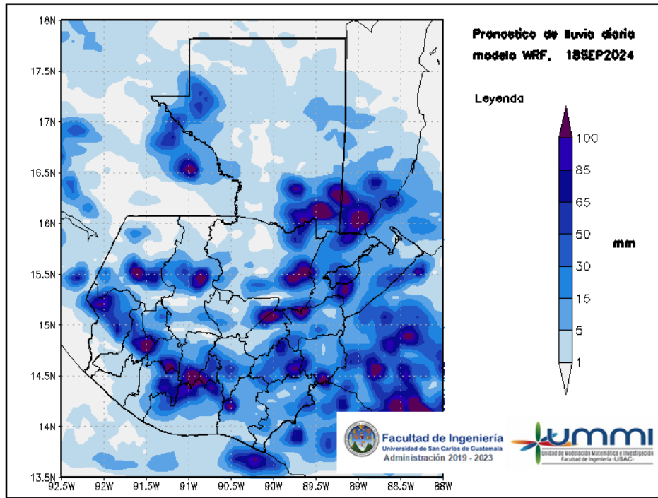
Figura 3: Pronóstico de lluvia diaria del 18 de September
