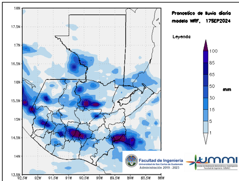
Figura 2: Pronóstico de lluvia diaria del 17 de September
