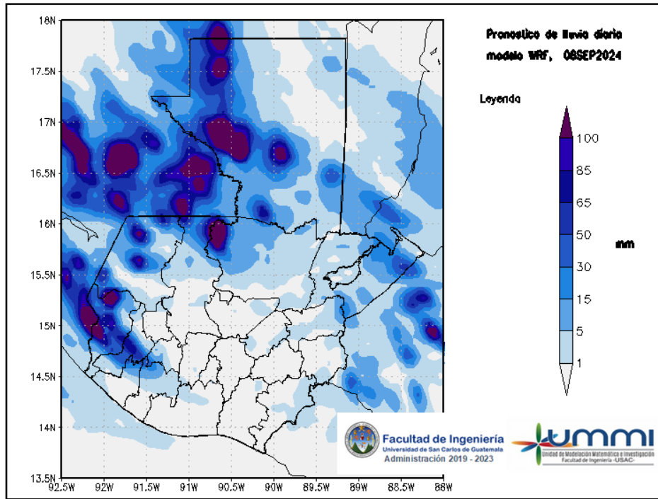
Figura 1: Pronóstico de lluvia diaria del 08 de September
