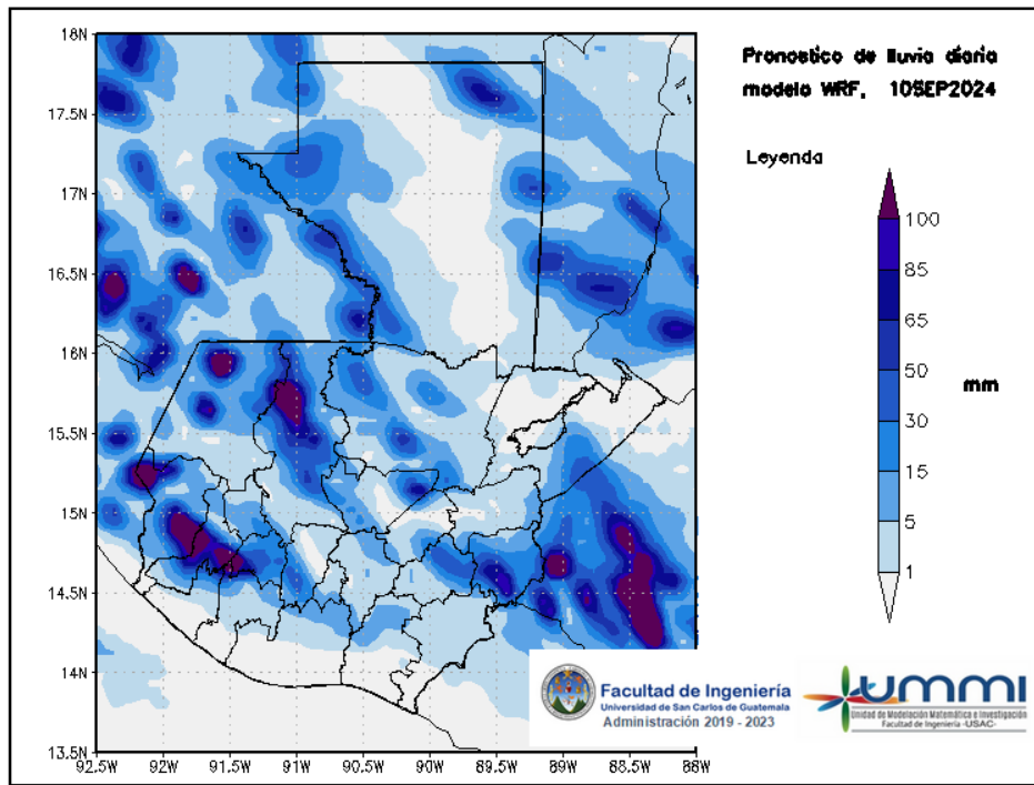
Figura 3: Pronóstico de lluvia diaria del 10 de September
