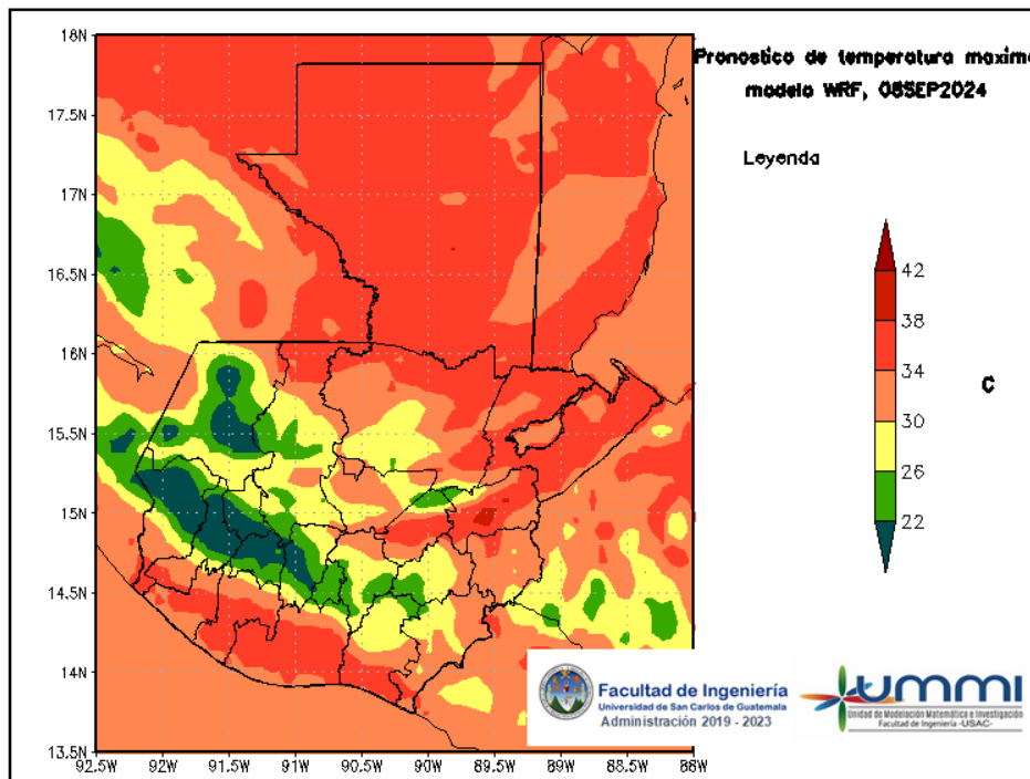
Figura 4: Pronóstico de temperatura máxima diaria del 08 de September
