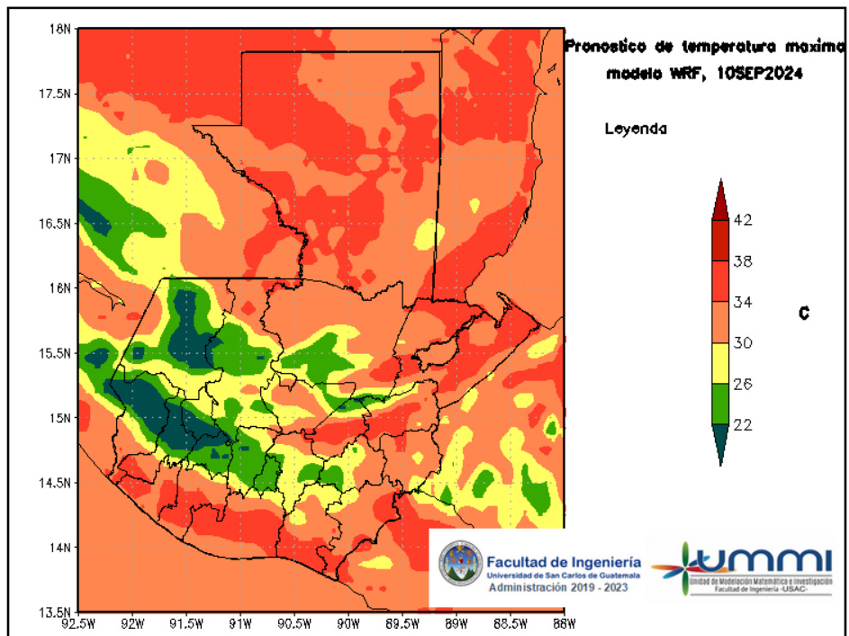
Figura 6: Pronóstico de temperatura máxima diaria del 10 de September
