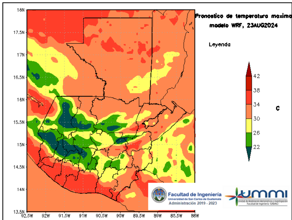
Figura 6: Pronóstico de temperatura máxima diaria del 23 de August
