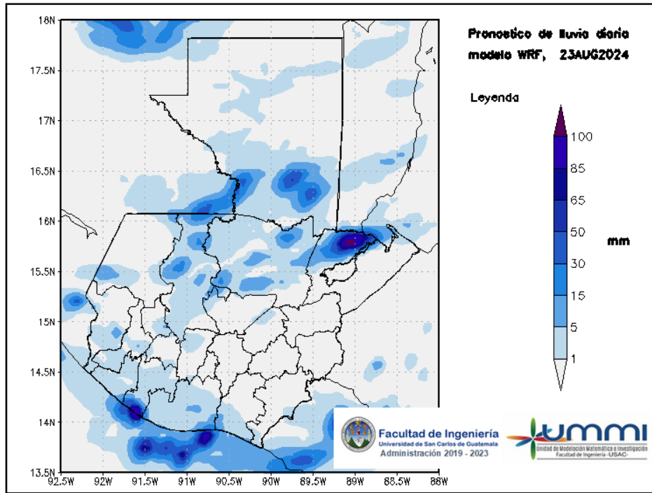
Figura 3: Pronóstico de lluvia diaria del 23 de August
