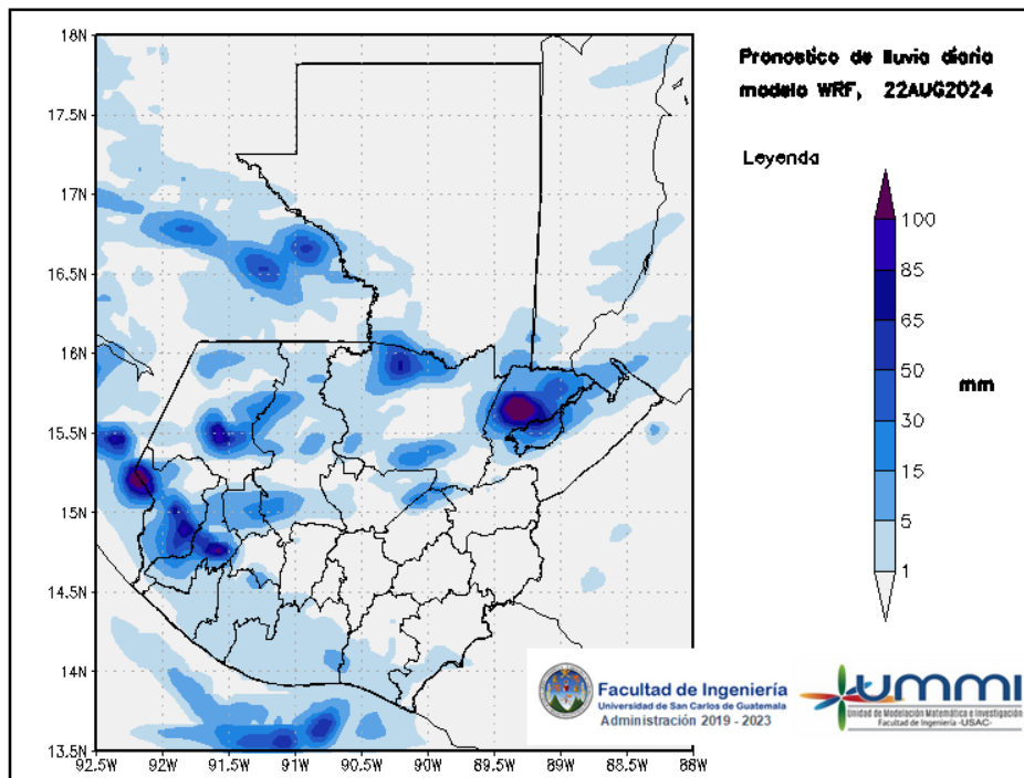
Figura 2: Pronóstico de lluvia diaria del 22 de August
