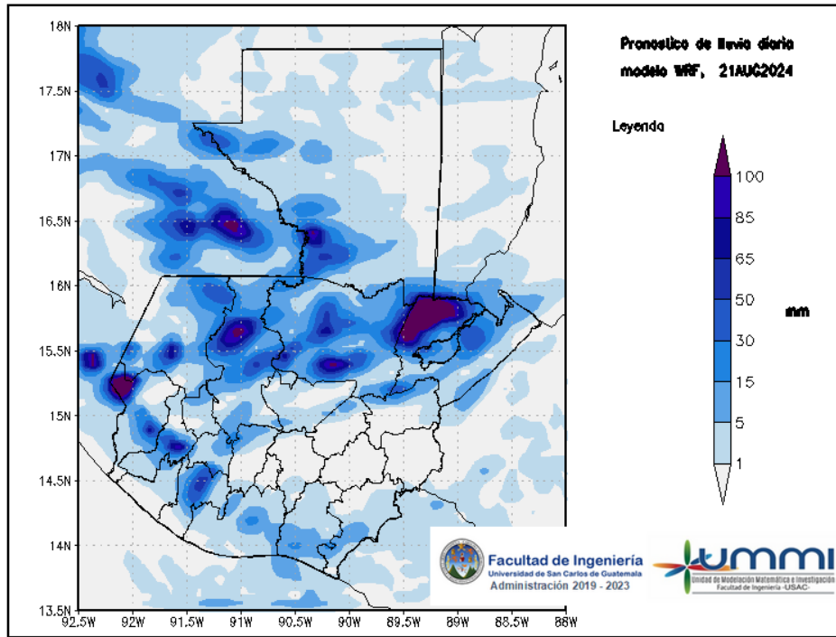
Figura 1: Pronóstico de lluvia diaria del 21 de August
