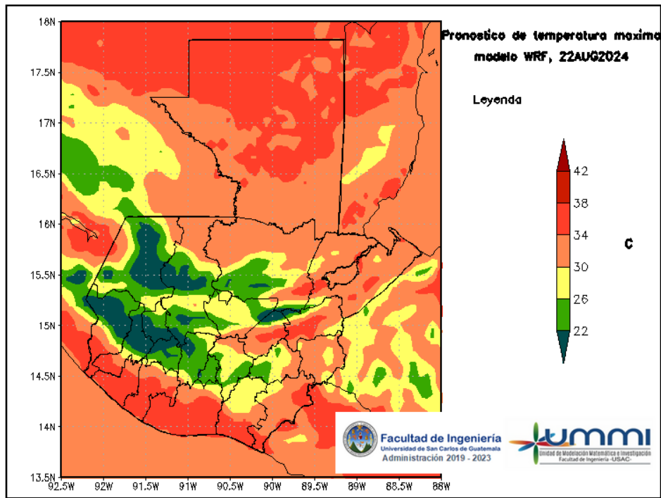
Figura 5: Pronóstico de temperatura máxima diaria del 22 de August
