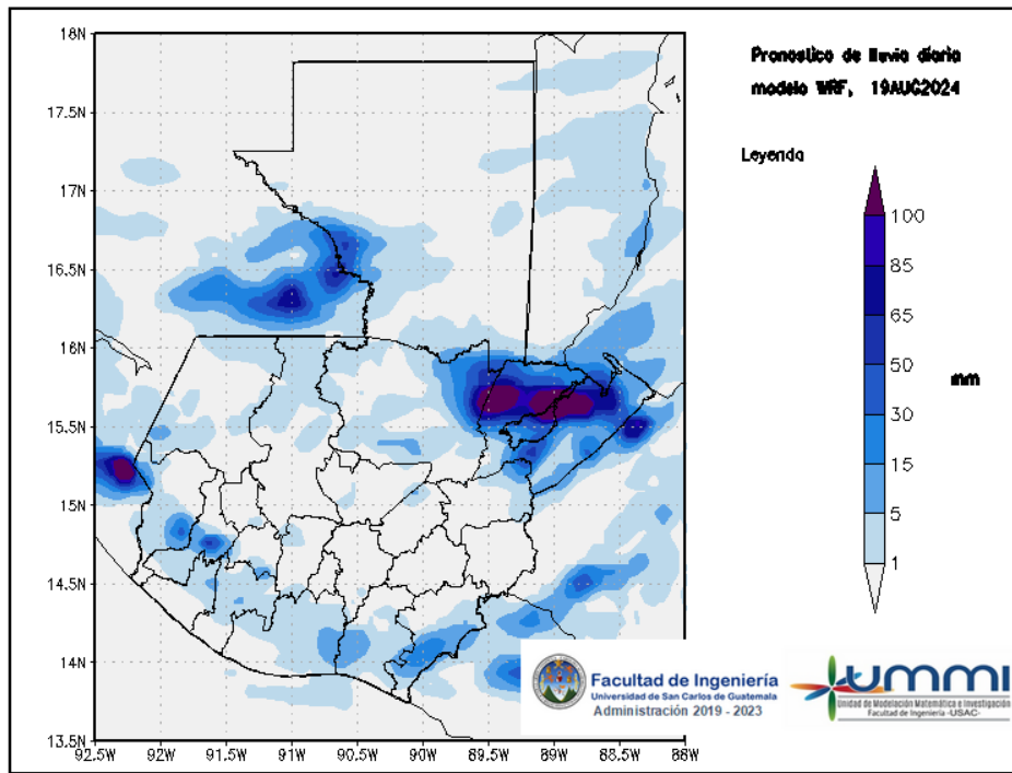
Figura 1: Pronóstico de lluvia diaria del 19 de August
