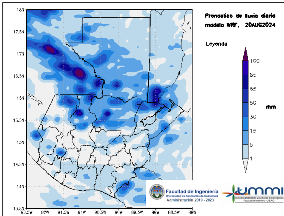
Figura 2: Pronóstico de lluvia diaria del 20 de August
