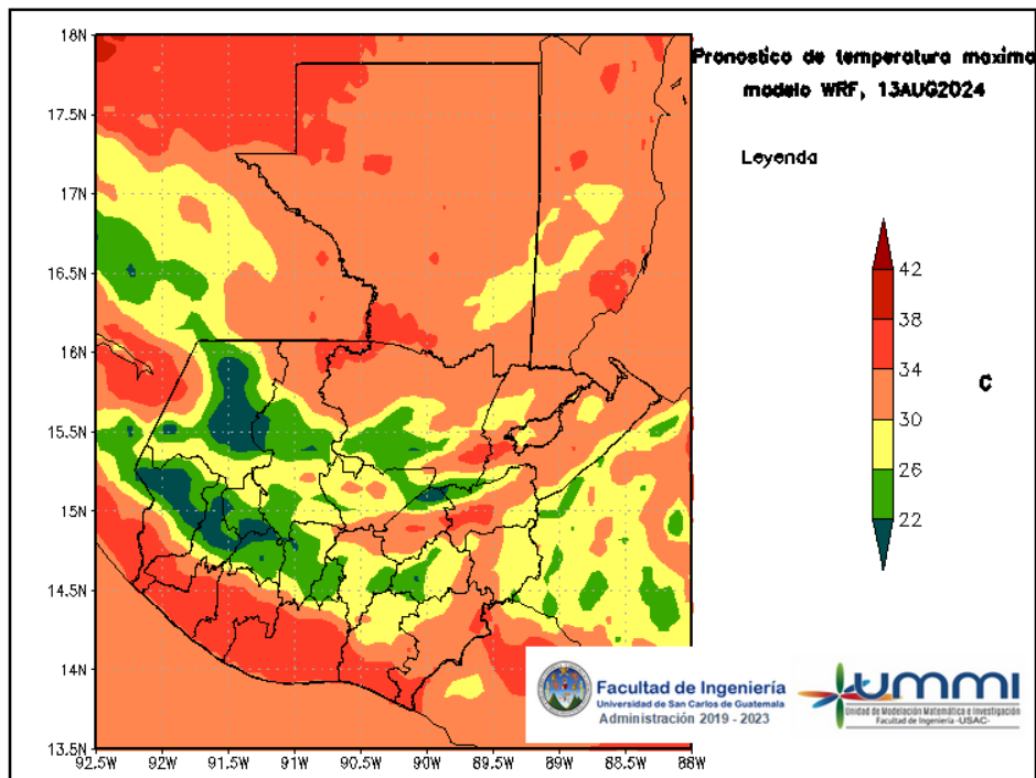
Figura 6: Pronóstico de temperatura máxima diaria del 13 de August
