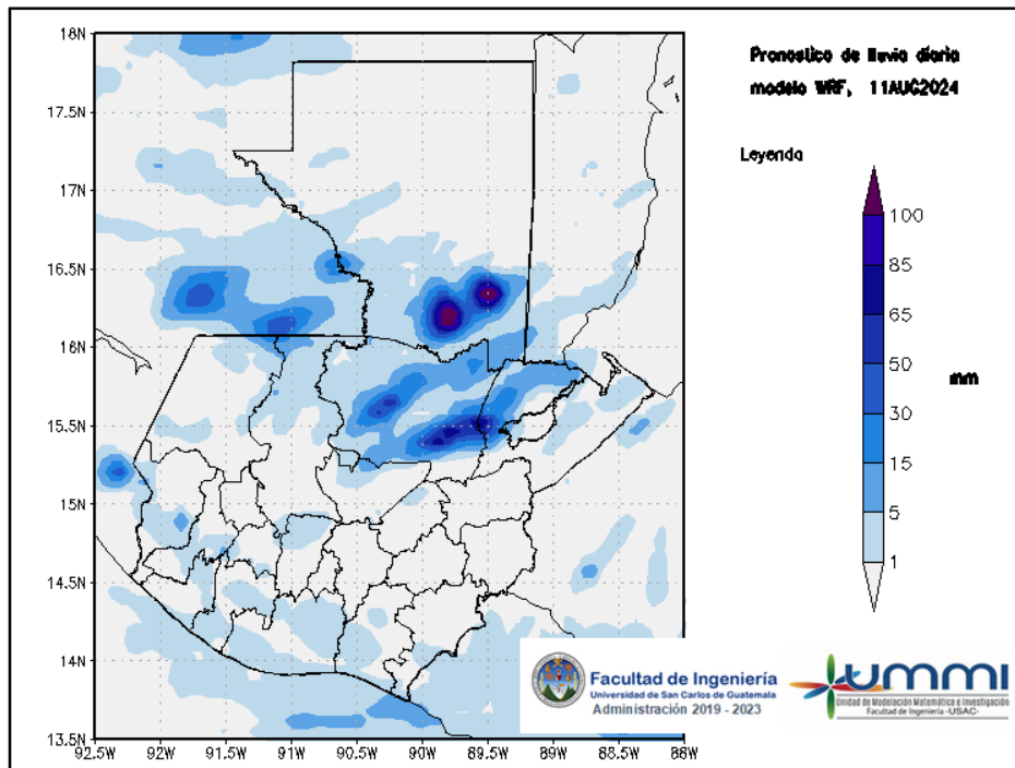
Figura 1: Pronóstico de lluvia diaria del 11 de August
