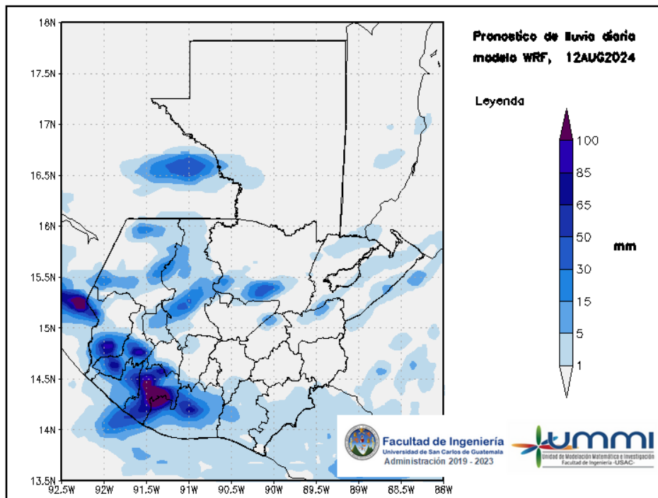
Figura 2: Pronóstico de lluvia diaria del 12 de August
