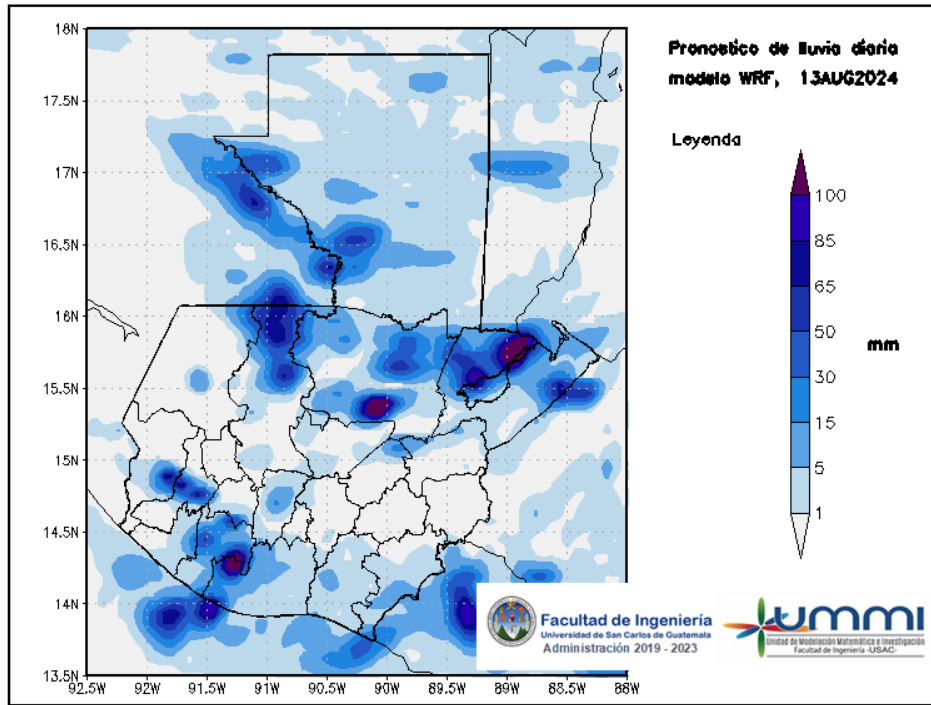
Figura 3: Pronóstico de lluvia diaria del 13 de August
