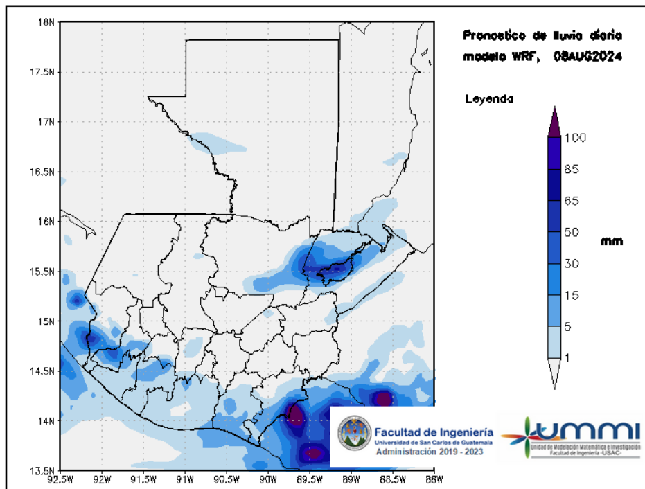
Figura 2: Pronóstico de lluvia diaria del 08 de August
