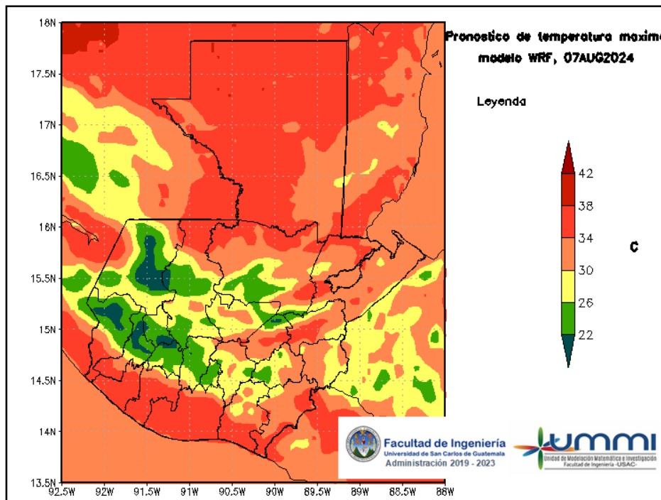
Figura 4: Pronóstico de temperatura máxima diaria del 07 de August
