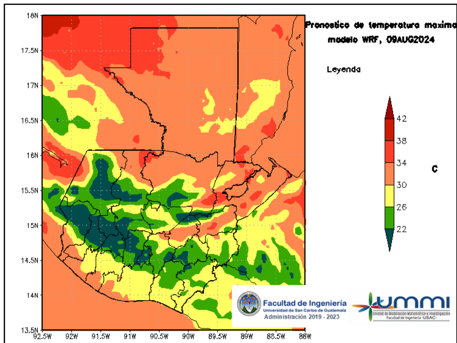
Figura 6: Pronóstico de temperatura máxima diaria del 09 de August
