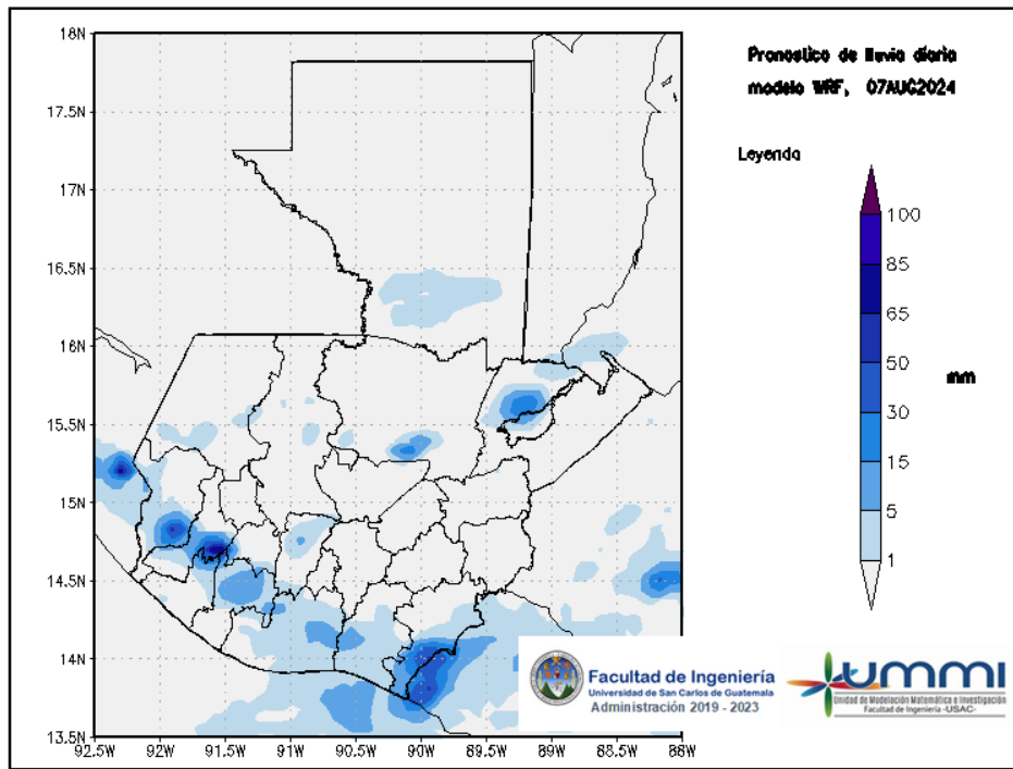
Figura 1: Pronóstico de lluvia diaria del 07 de August
