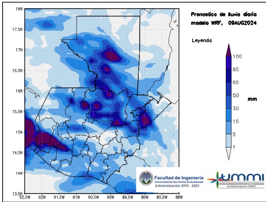
Figura 3: Pronóstico de lluvia diaria del 09 de August
