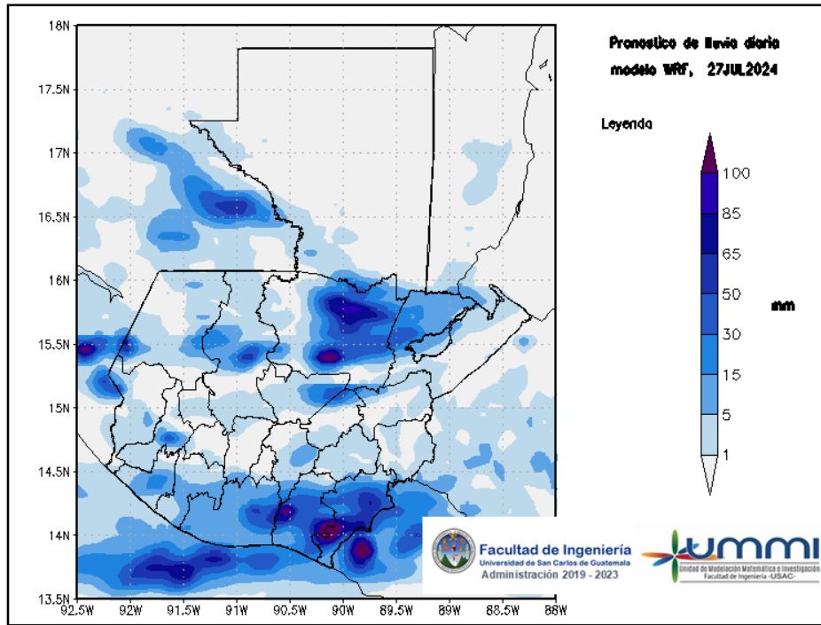
Figura 1: Pronóstico de lluvia diaria del 27 de July
