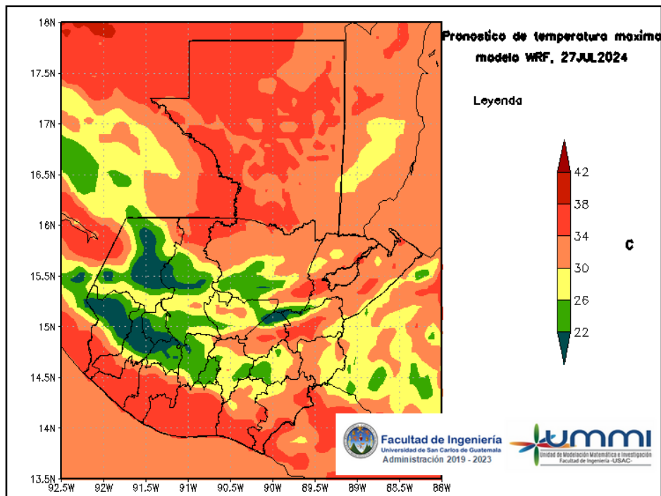
Figura 4: Pronóstico de temperatura máxima diaria del 27 de July
