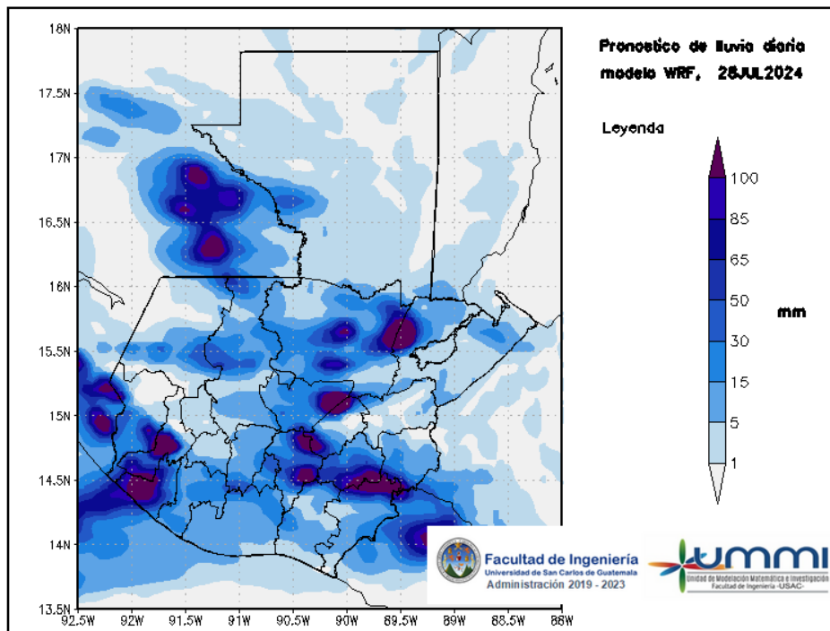
Figura 2: Pronóstico de lluvia diaria del 28 de July
