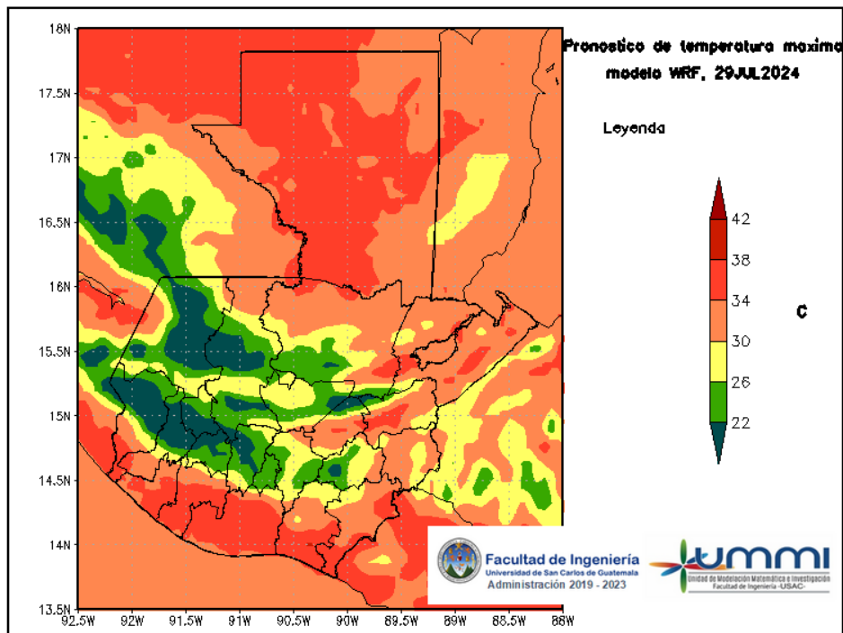
Figura 6: Pronóstico de temperatura máxima diaria del 29 de July
