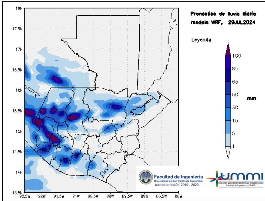
Figura 3: Pronóstico de lluvia diaria del 29 de July
