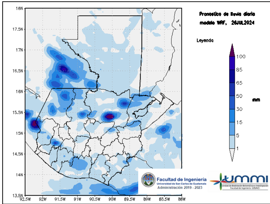
Figura 1: Pronóstico de lluvia diaria del 26 de July
