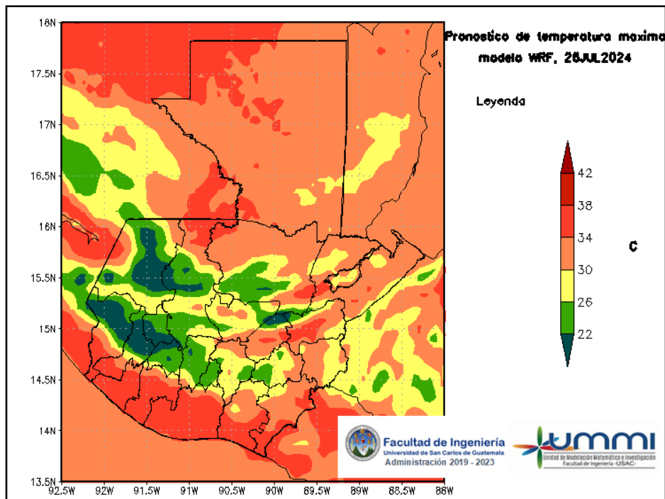
Figura 4: Pronóstico de temperatura máxima diaria del 26 de July
