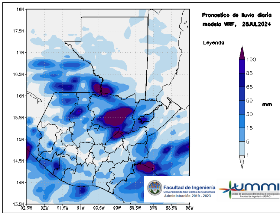
Figura 3: Pronóstico de lluvia diaria del 28 de July
