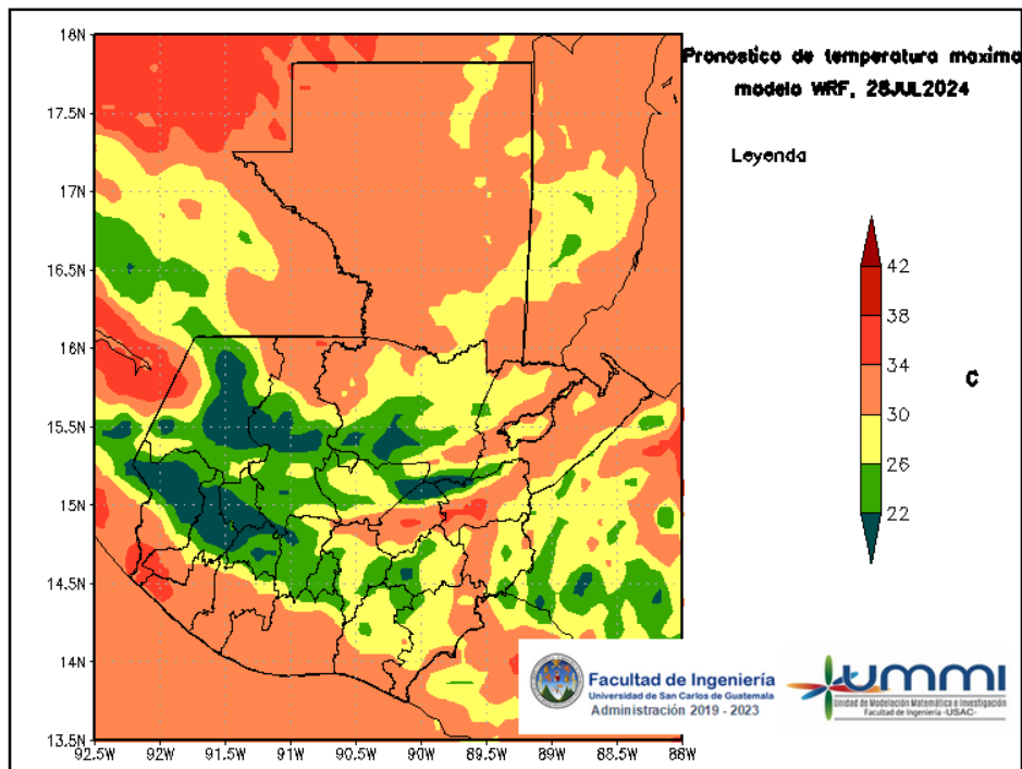
Figura 6: Pronóstico de temperatura máxima diaria del 28 de July
