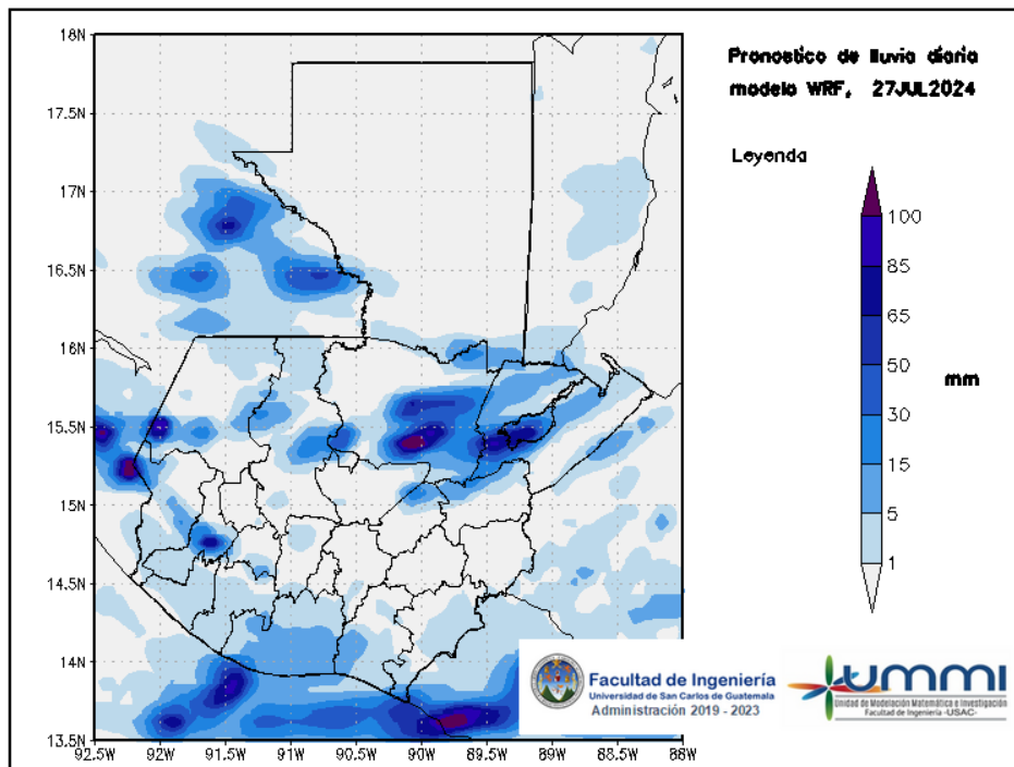
Figura 2: Pronóstico de lluvia diaria del 27 de July
